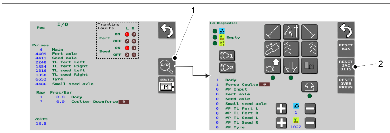
Bild. 7.9.4.1 - 343. Återställning av felminnet för körspårskopplingen
