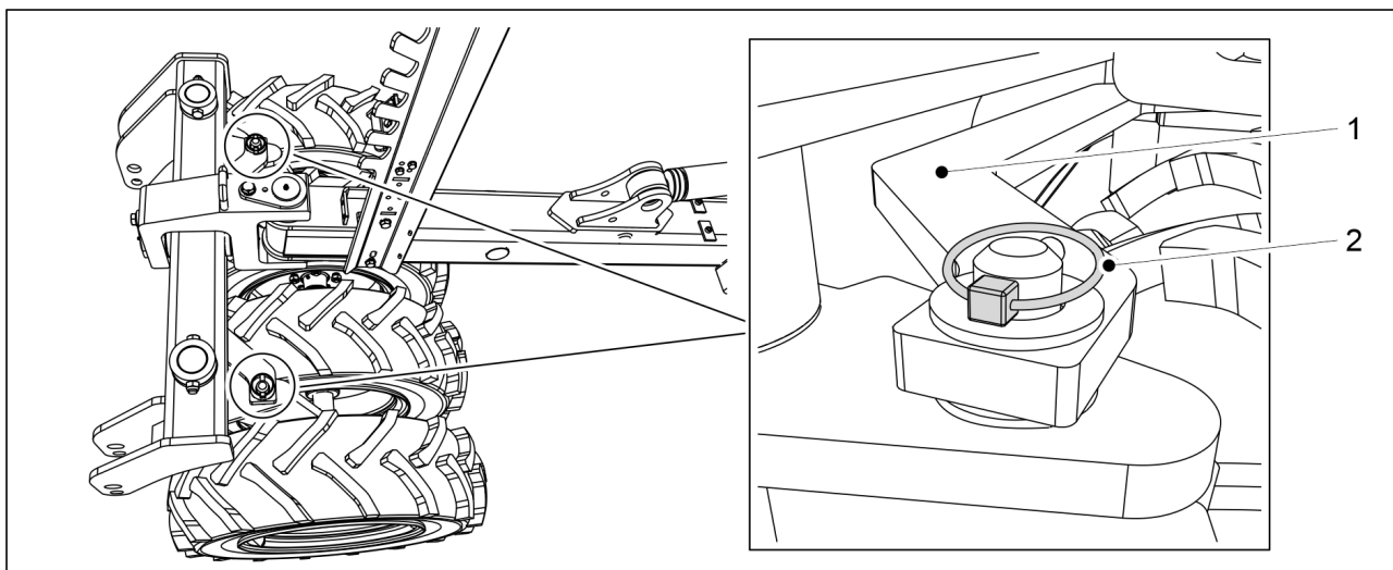
Bild. 7.1.2.3 - 256. Hjulpackarens stång
