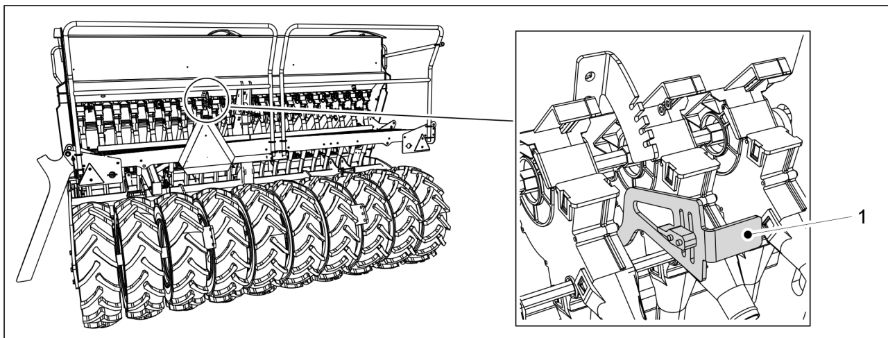
Bild. 6.24.2 - 249. Öppna bottenfliken till småfröbehållaren
