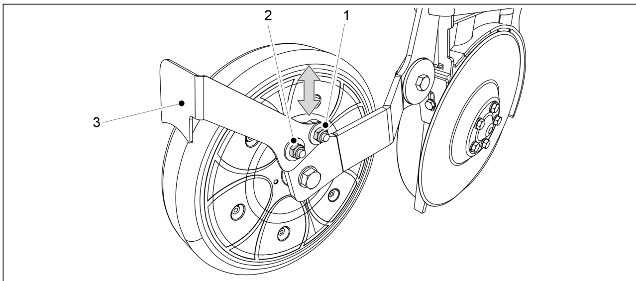
Bild. 7.8.5.2 - 334. Täckhjulets skrapa
