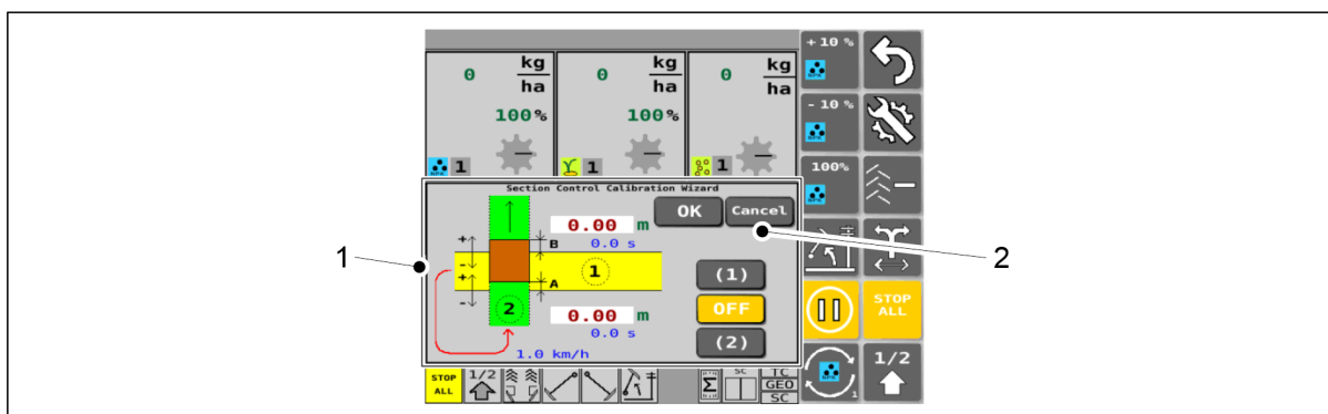
Bild. 6.11.2.1 - 216. Section Control Calibration Wizard och knappen CANCEL
