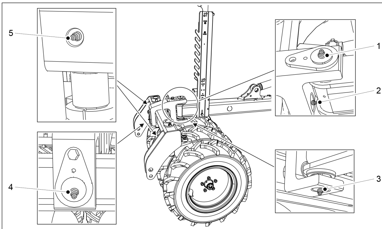
Bild. 7.2.10 - 280. Hjulpackarens stift
