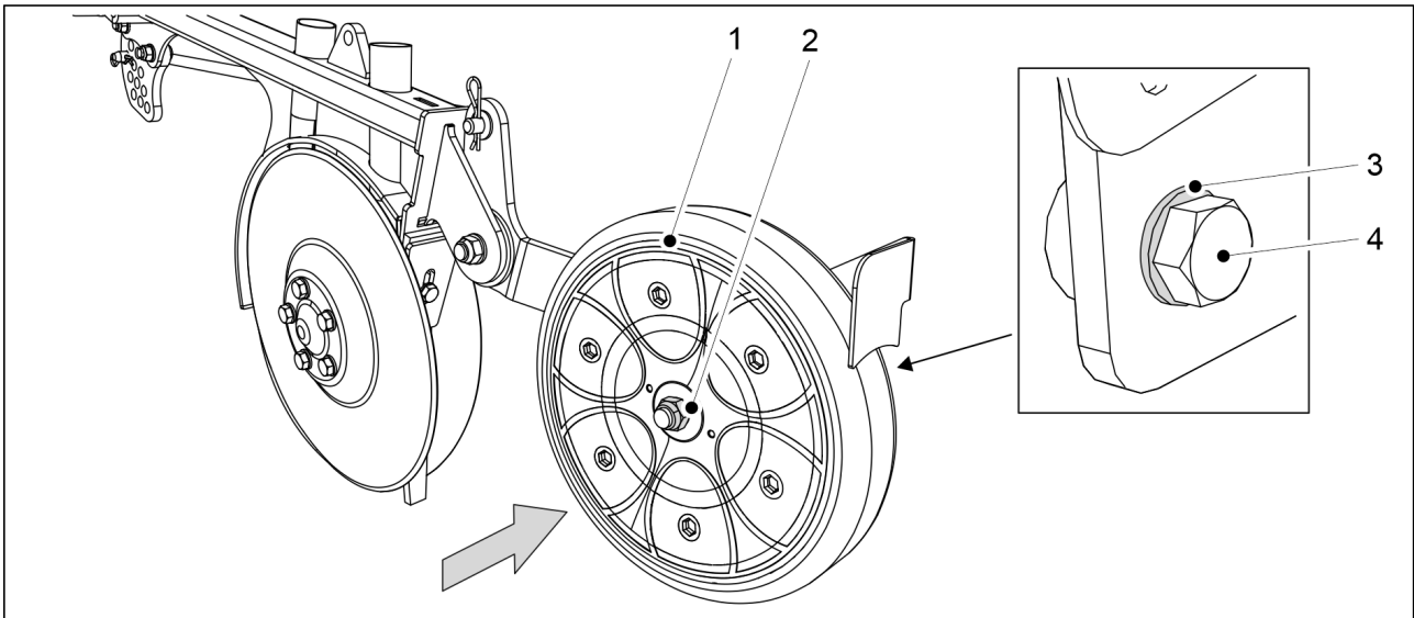
Bild. 7.8.4.2 - 332. Montering av täckhjulet
