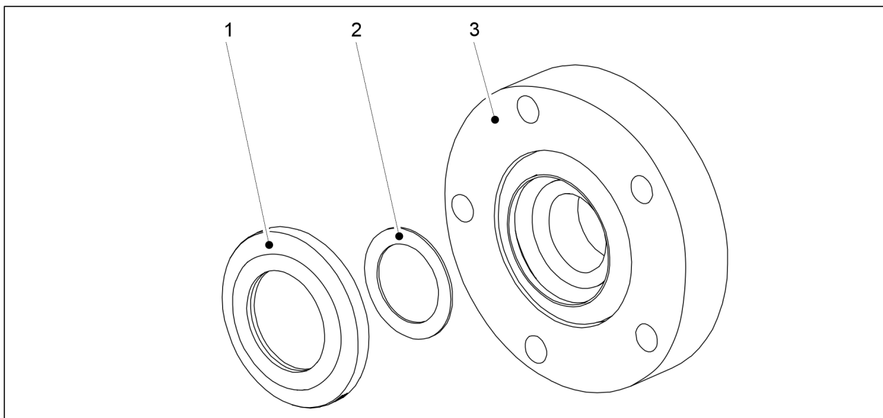
Bild. 7.8.3.1 - 327. Lagertätning och lagerring
