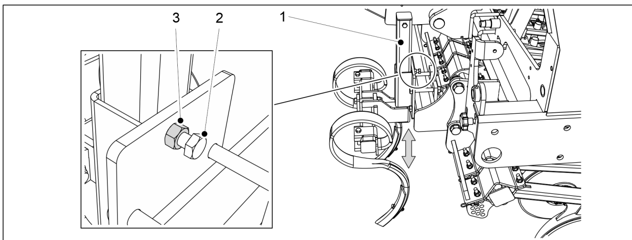
Bild. 6.18.1 - 237. Justering av spårborttagarens höjd
