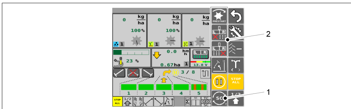
Bild. 6.10 - 209. Aktivering av knapparna för AVSTÄNGNING AV HALVA MASKINEN
