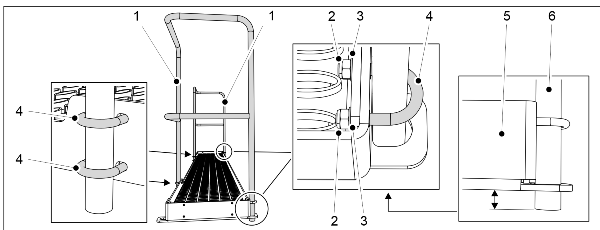
Bild. 5.1.15 - 94. Montering av räcken på en eCEREX 400-maskin
