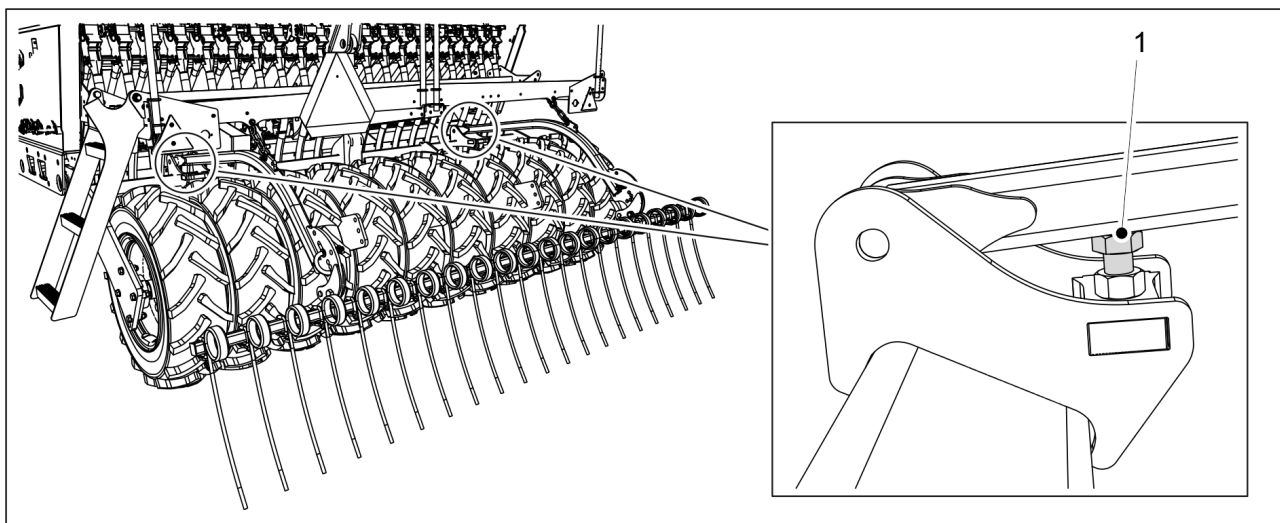
Bild. 6.14 - 228. Justering av efterharvens höjd
