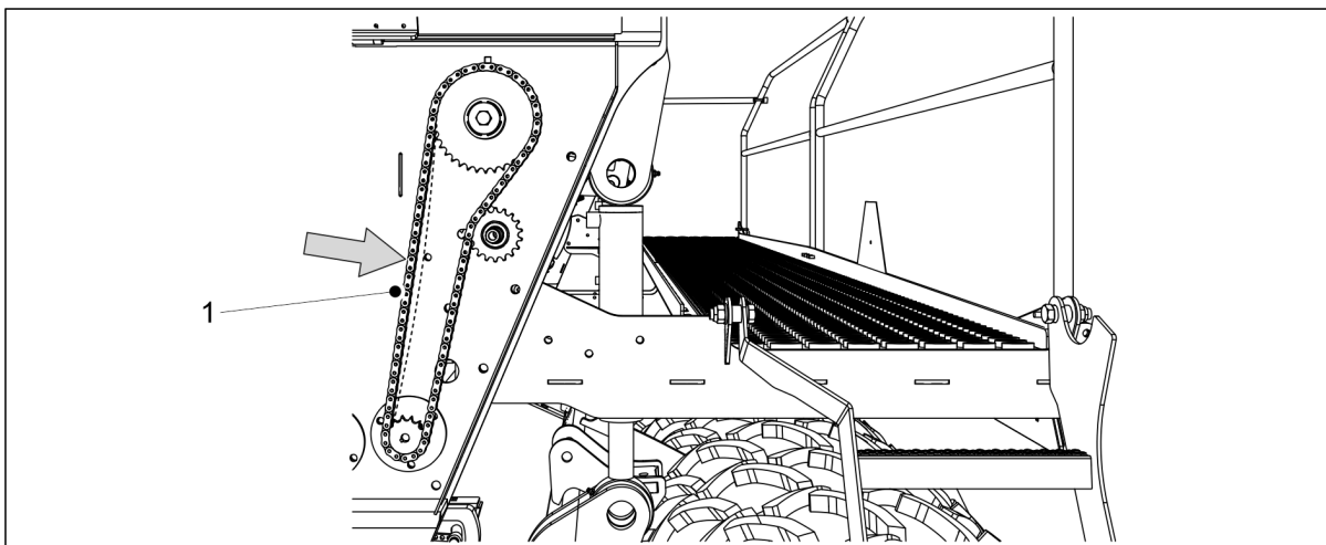
Bild. 7.1.5.2 - 266. Kontroll av kedjespänning, överföring av småfrön
