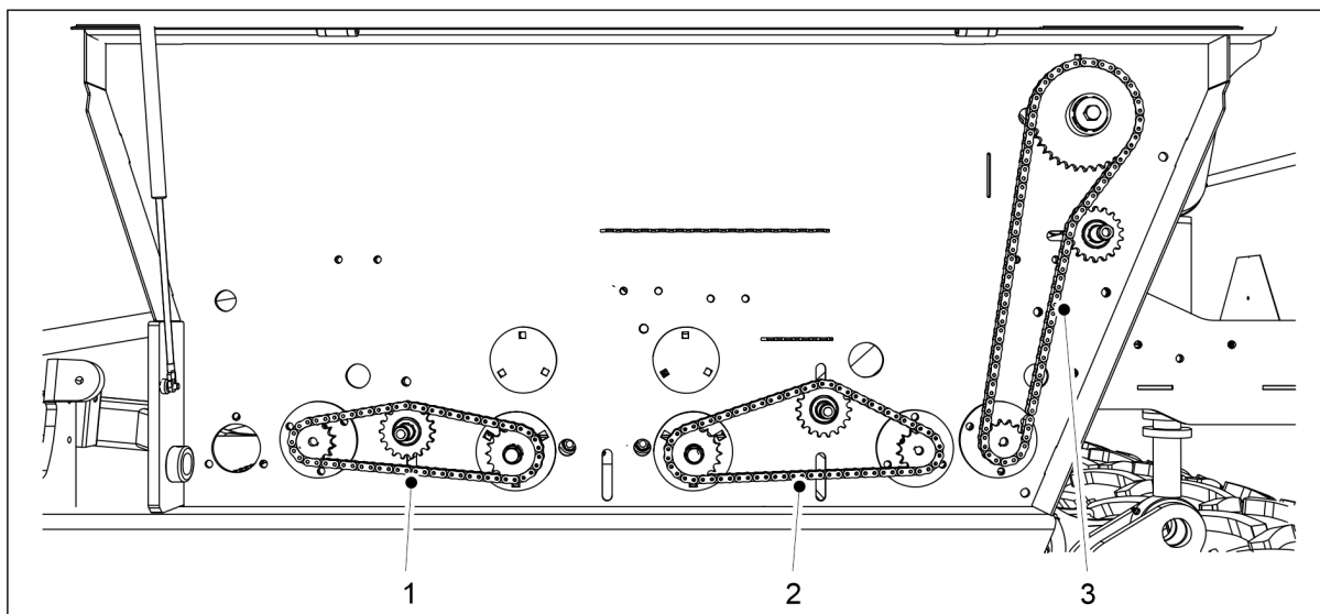
Bild. 7.2.2 - 273. Smörjning av transmissionskedjor
