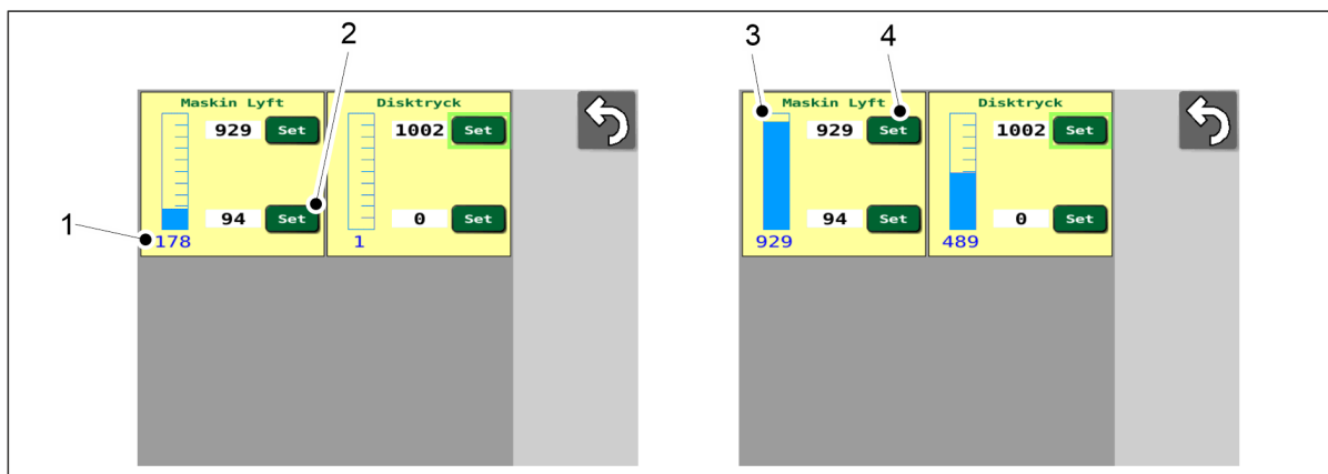
Bild. 7.9.1.1 - 335. Kalibrering av maskinens sålågessensor
