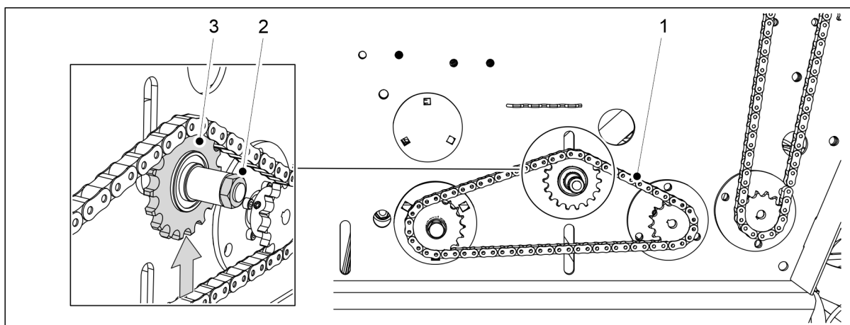
Bild. 7.5.1 - 310. Dra åt kedjan hos fröbehållaren
