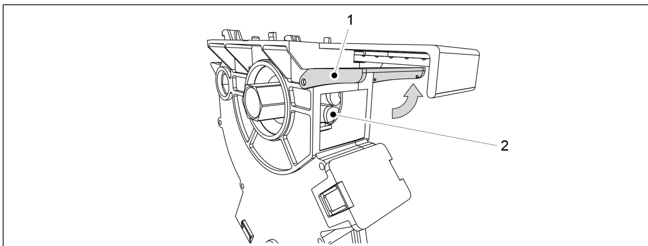
Bild. 7.3.5 - 294. Rengöring av matarenheter
