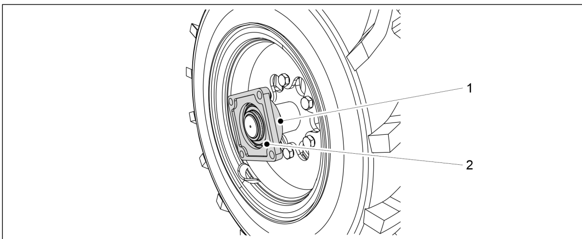
Bild. 7.4.3 - 307. Fästa lagret
