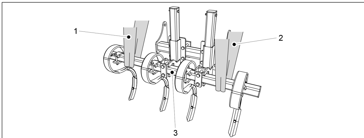
Bild. 5.1.7 - 70. Lyfta en spårborttagare
