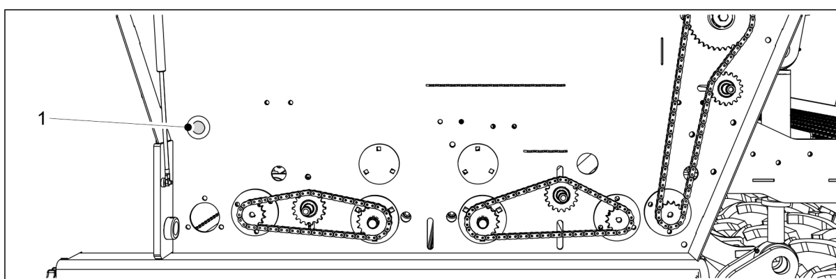
Bild. 6.8.3 - 203. Knapp
