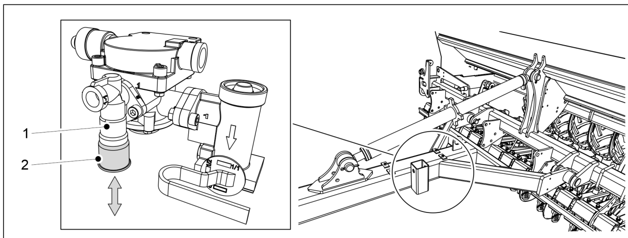
Bild. 6.22.2 - 243. Bromsfrigöringsventil
