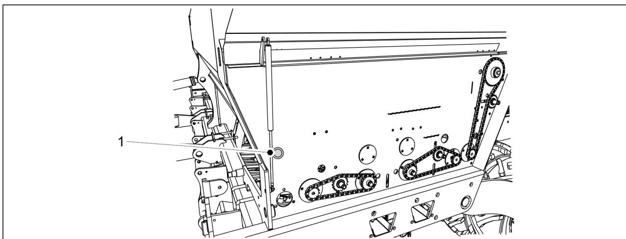
Bild. 4.1.1.10 - 24. Knapp
