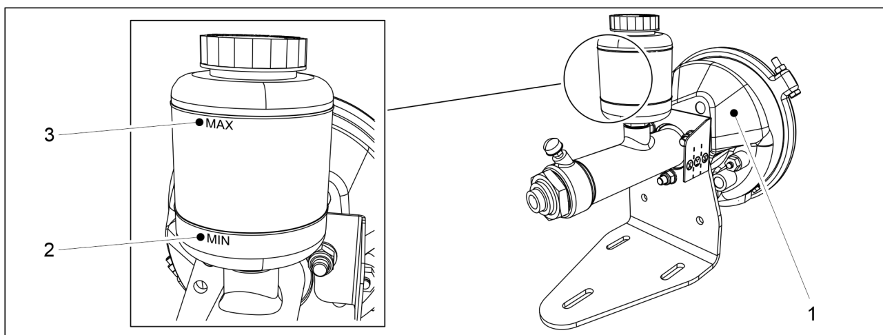
Bild. 7.1.10.3 - 272. Kontroll av oljenivån i den pneumatisk-hydrauliska omvandlaren
