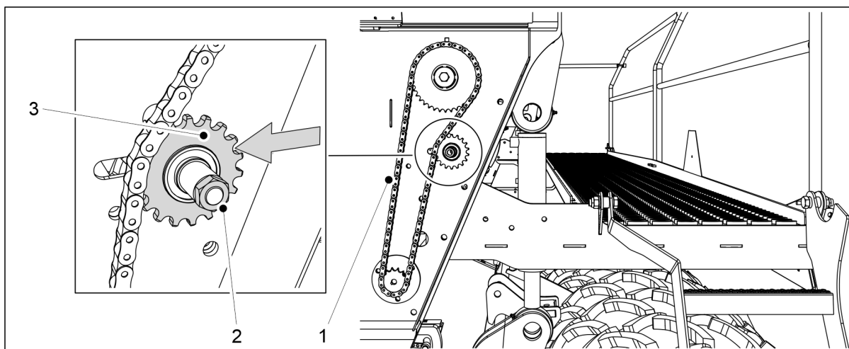
Bild. 7.5.2 - 311. Dra åt kedjan hos småfröbehållaren
