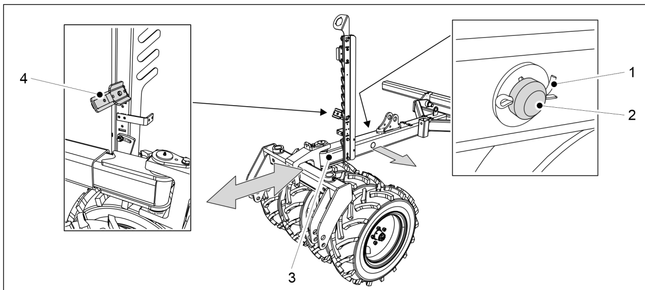
Bild. 5.3.1 - 115. Justering av bommens längd
