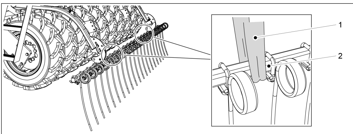
Bild. 5.1.13 - 84. Lyfta efterharven
