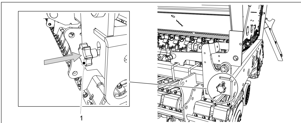
Bild. 6.8.3 - 205. Sätta in kalibreringsprovets justerstång
