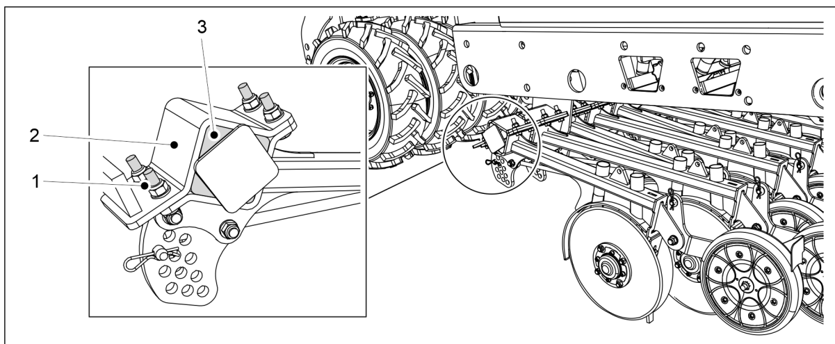
Bild. 7.8.1.1 - 320. Demontering av en såbill
