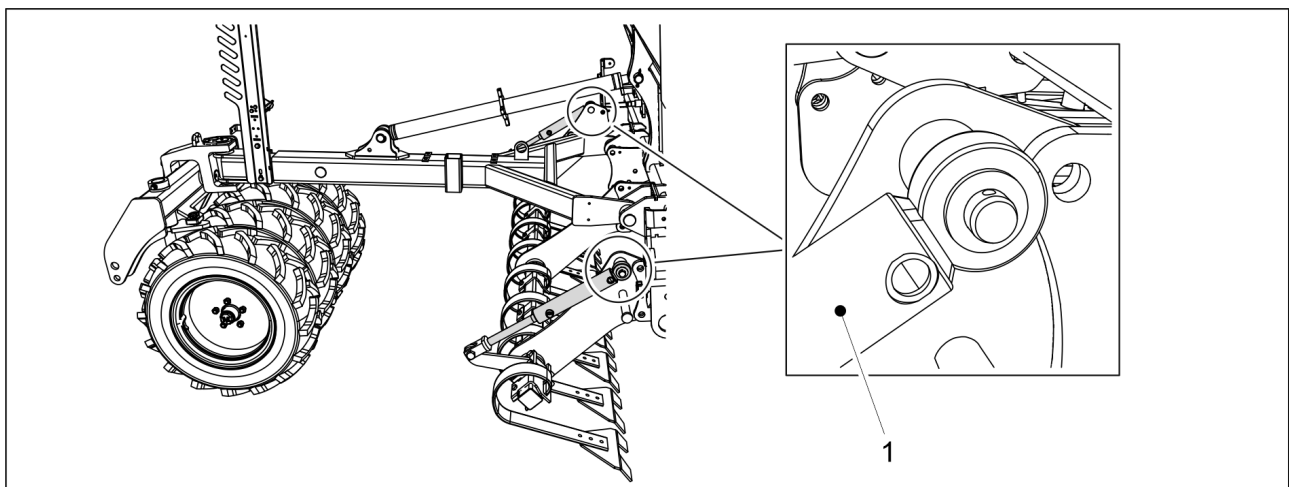
Bild. 7.2.11 - 283. Cylindrar hos den främre utjämningsharven
