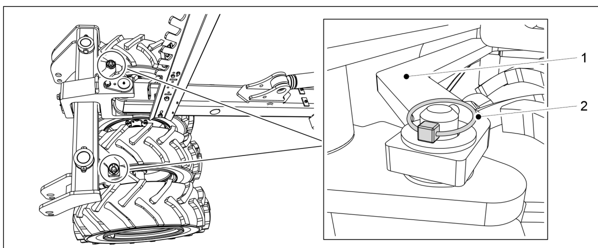
Bild. 7.2.10 - 281. Avlägsnande av hjulpackarens stång
