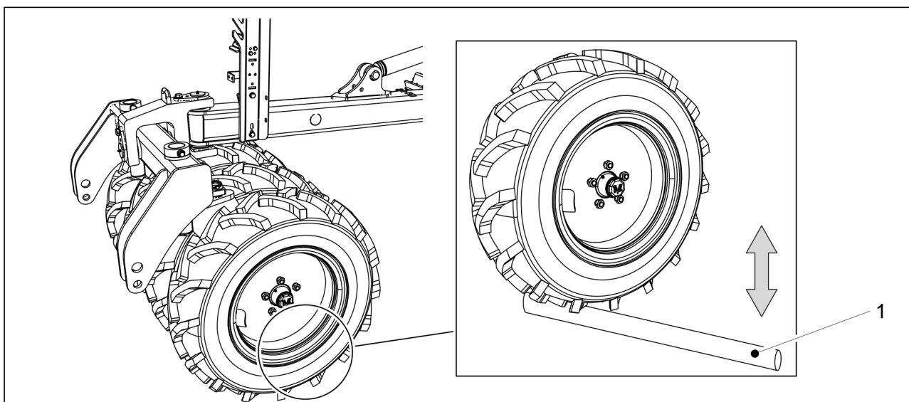
Bild. 7.1.4 - 264. Kontroll av lagers spelrum i hjulpackarens nav
