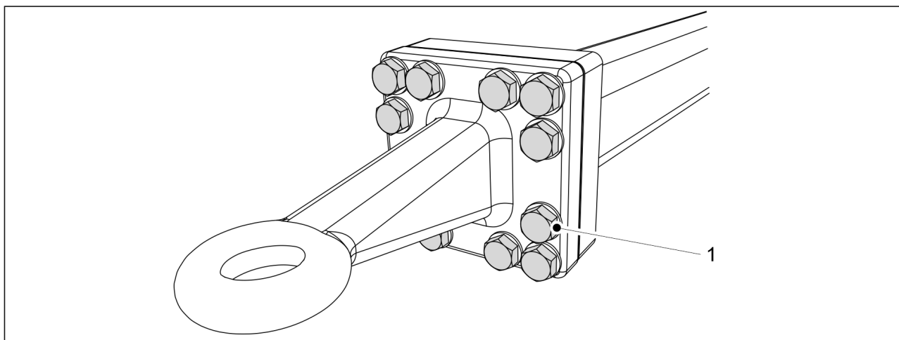
Bild. 7.1.2.6 - 263. Dragöglans skruvar
