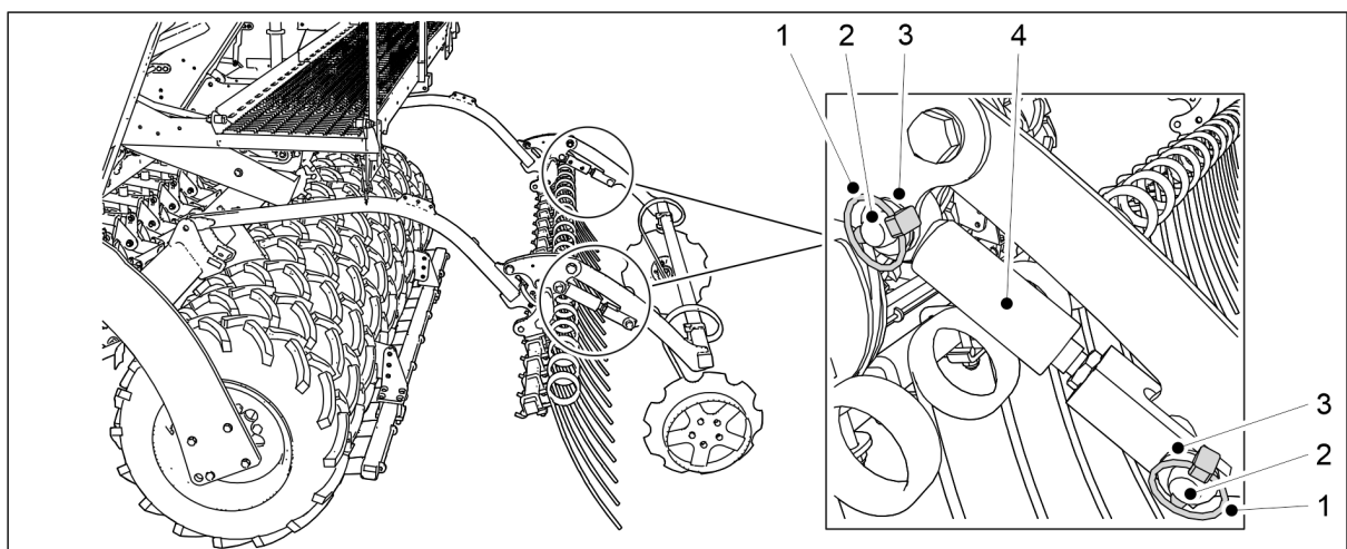
Bild. 7.4.1 - 297. Borttagning av de bakre markör cylindrarna
