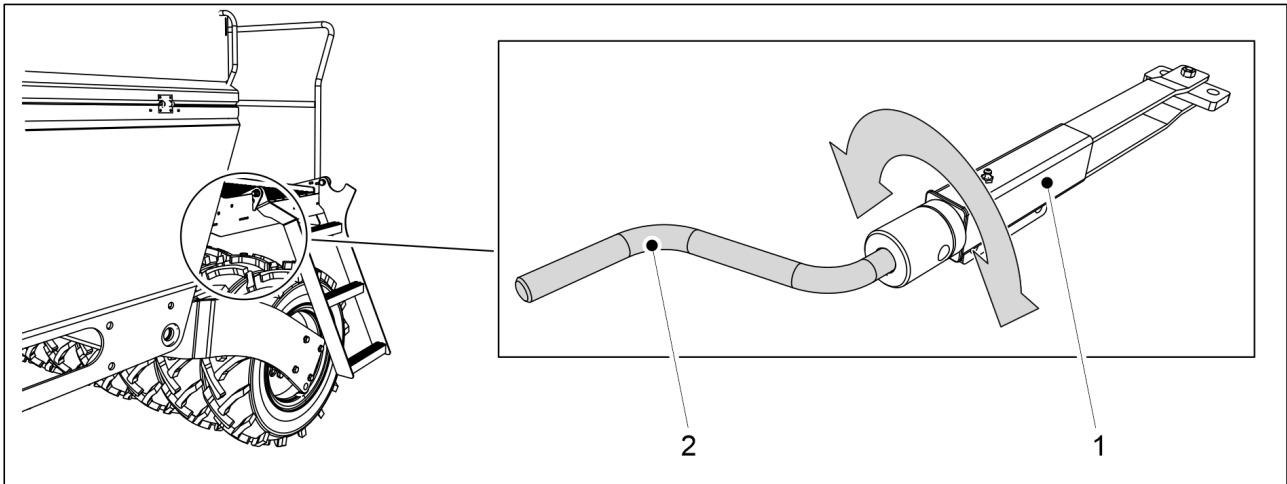
Bild. 6.22.1 - 242. Parkeringsbroms
