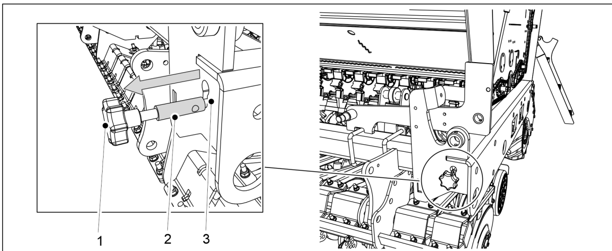
Bild. 6.8.2 - 188. Dra ut kalibreringsprovets justerstång
