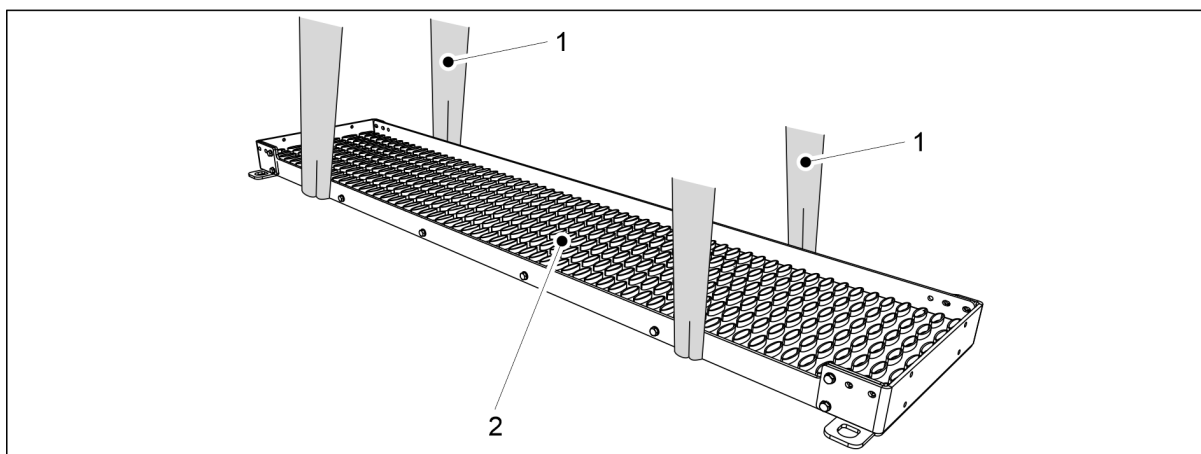
Bild. 5.1.16 - 97. Lyfta gångvägen
