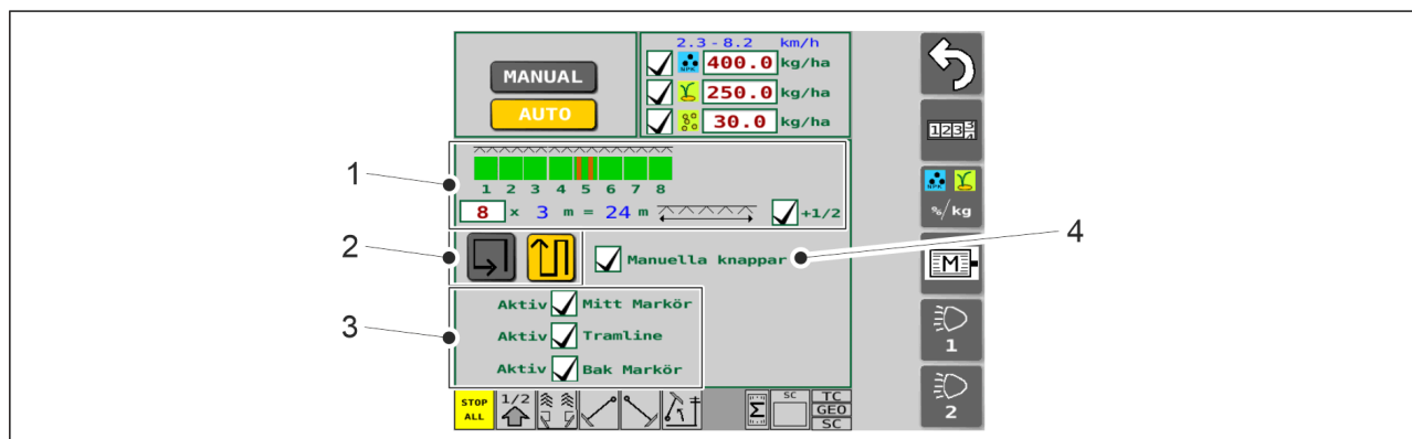
Bild. 4.1.3.1 - 42. Skärmbild från SeedPilot-kontrollsystemet som visar inställningar för utsäde, mitten
