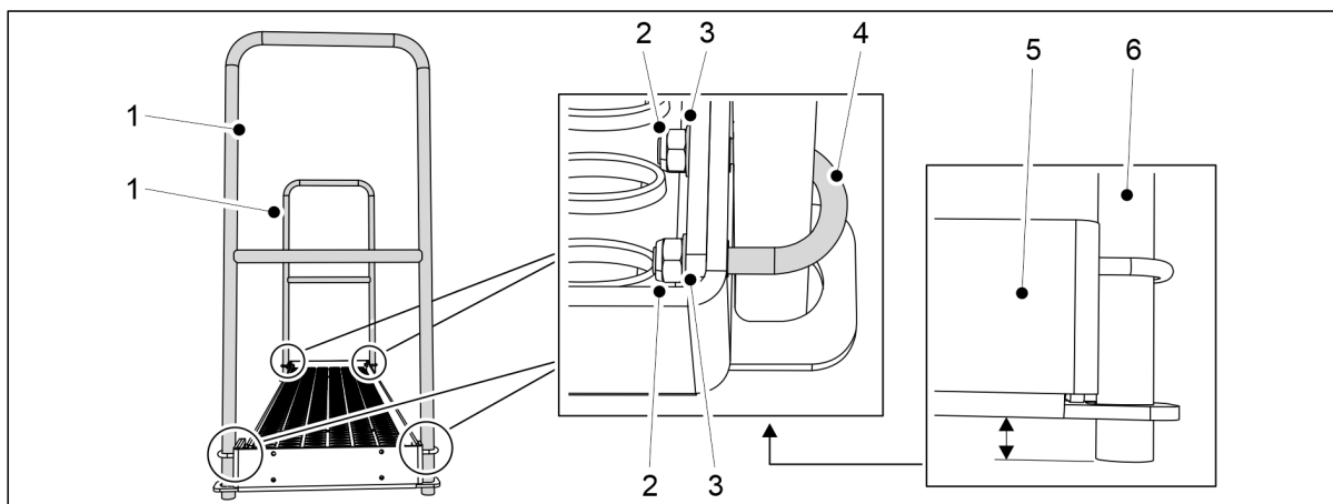
Bild. 5.1.16 - 100. Montering av räcken på en 300-maskin
