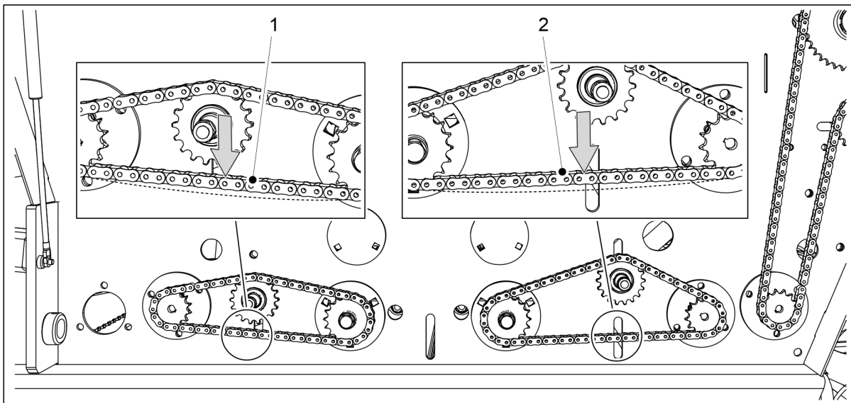
Bild. 7.1.5.1 - 265. Kontroll av kedjespänning, överföring av gödningsmedel och utsäde
