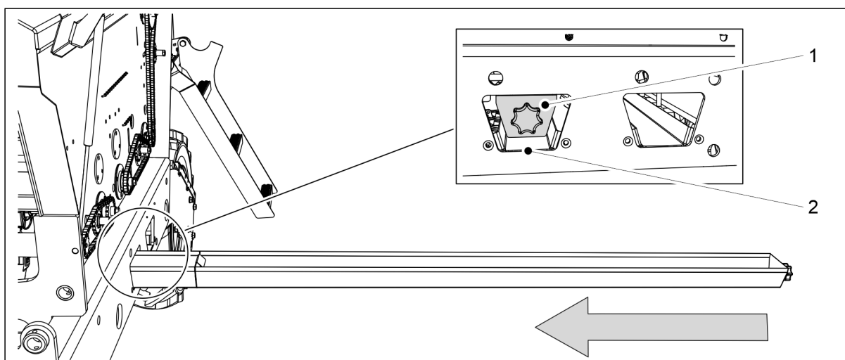
Bild. 6.8.1 - 180. Montera kalibreringsbrickorna
