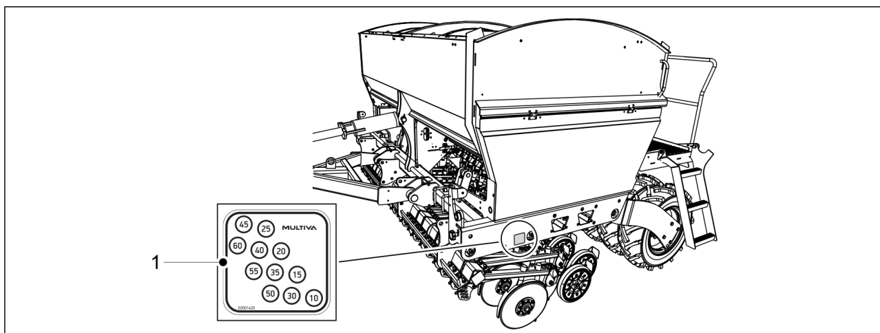
Bild. 6.12 - 225. Sådjup
