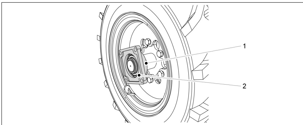
Bild. 7.4.2 - 304. Avlägsna ett flänslager
