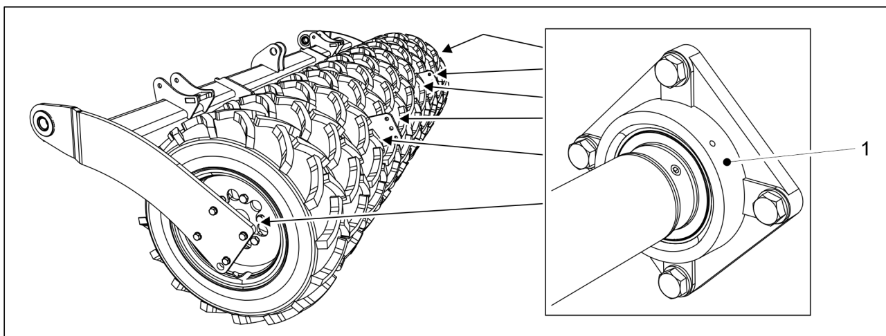
Bild. 7.2.5 - 275. Hjulaxelns kullager
