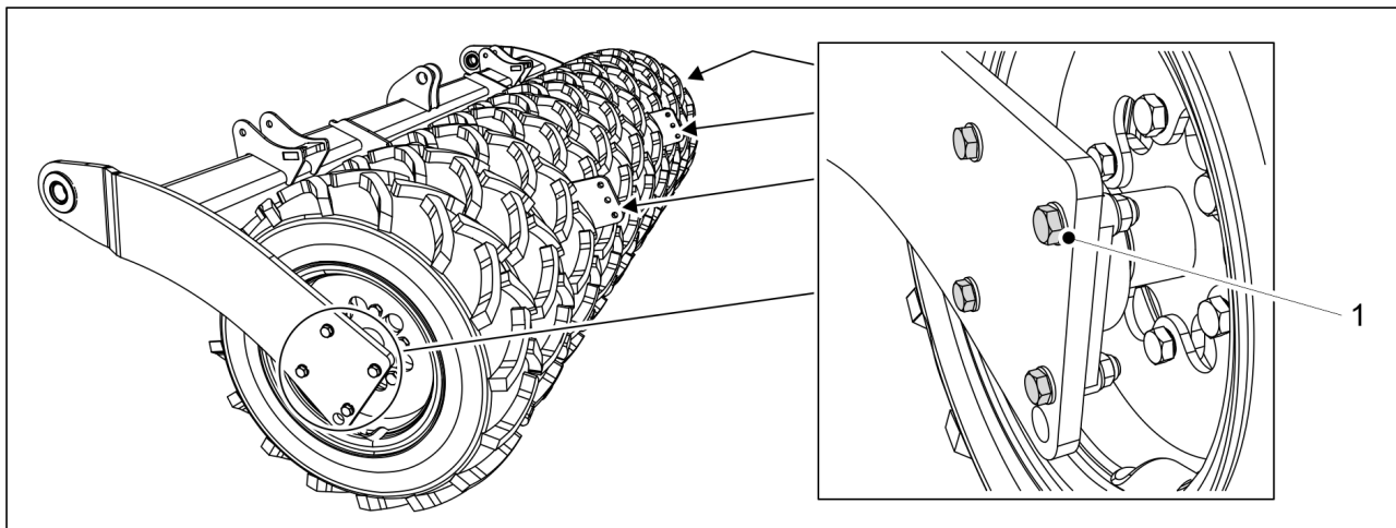
Bild. 7.1.2.2 - 255. Skruvarna i transporthjulens flänslager
