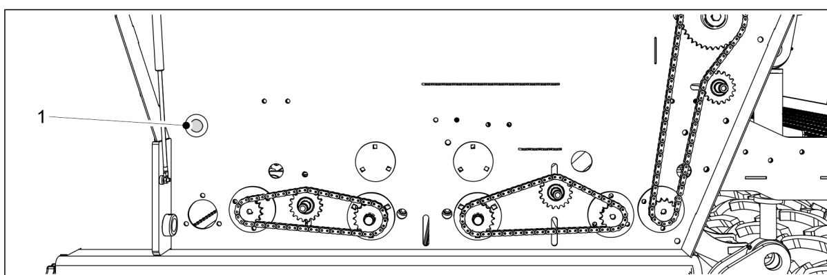
Bild. 6.8.1 - 185. Knapp
