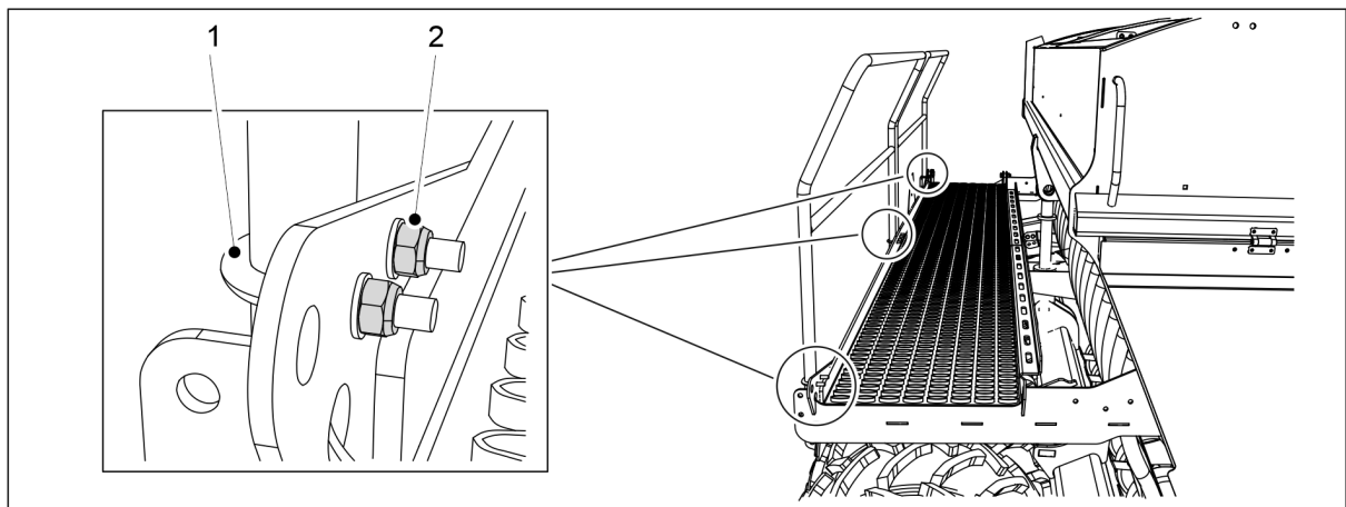
Bild. 7.1.2.5 - 262. Arbetsplattformens U-skrivar
