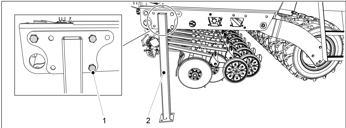
Bild. 7.4.1 - 300. Transportstöd
