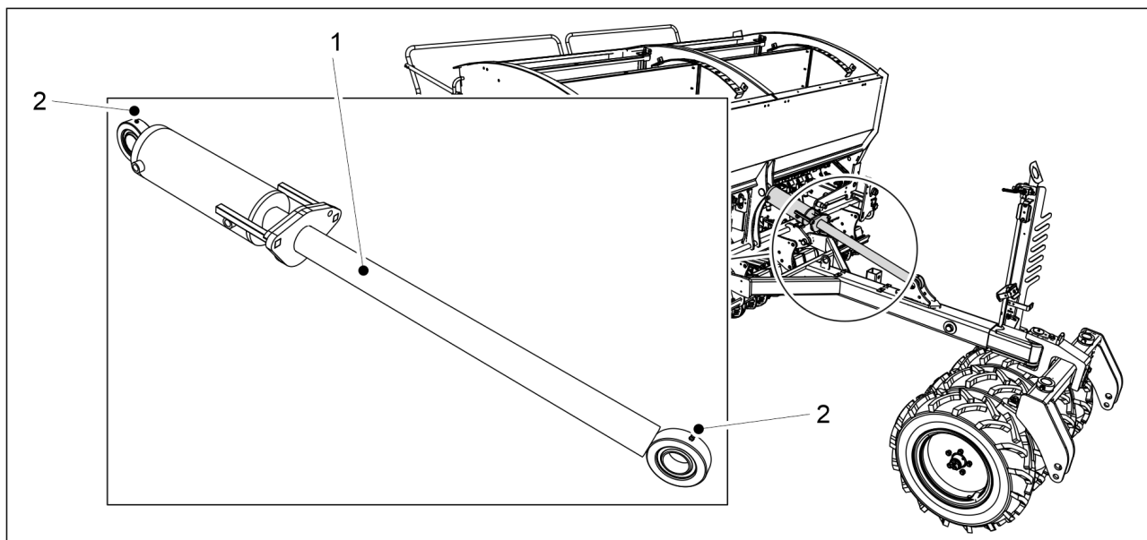
Bild. 7.2.14 - 286. Dragstångscylinde
