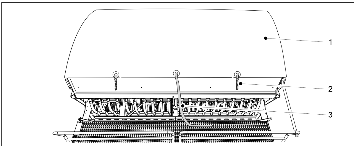
Bild. 6.7 - 177. Presenning för behållare
