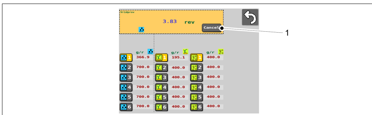
Bild. 6.8.3 - 201. Avbrytande av rotationsräkningen
