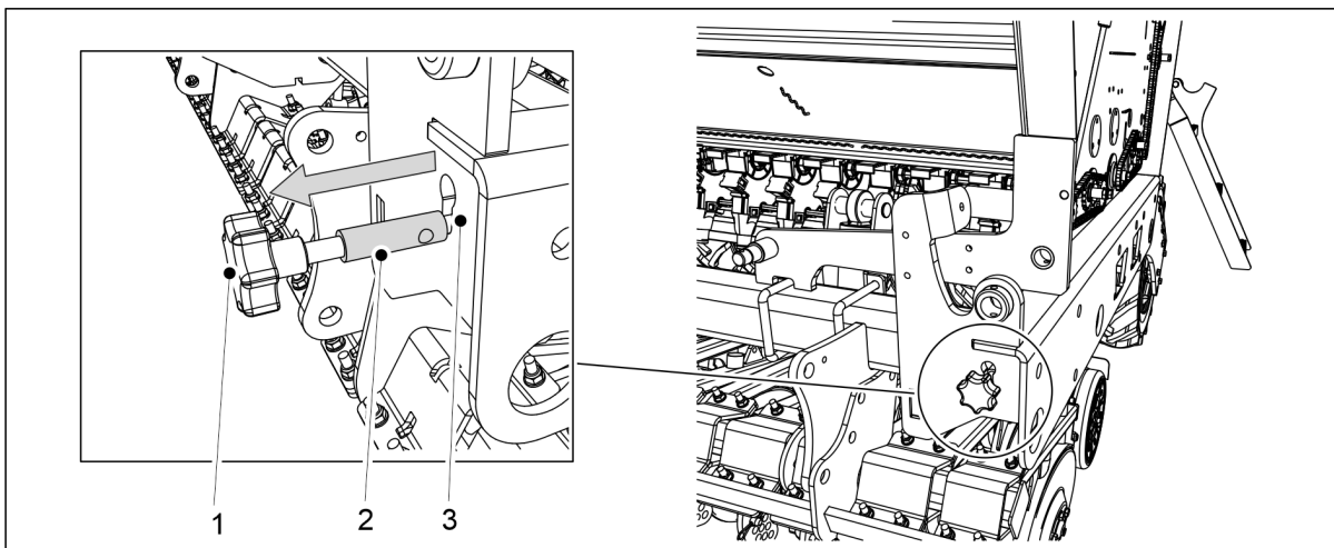
Bild. 6.8.3 - 197. Dra ut kalibreringsprovets justerstång
