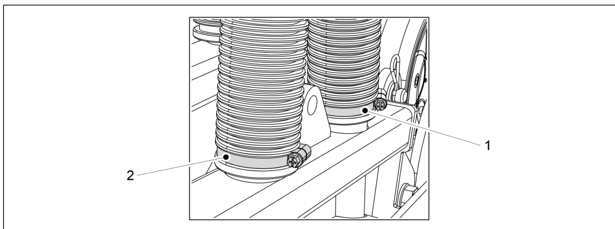
Bild. 5.1.10 - 75. Fästa utsädes- och gödningsmedelsröret till såbilen
