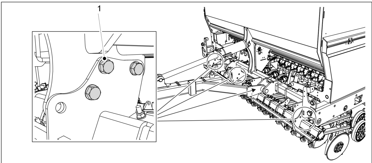
Bild. 7.1.2.4 - 258. Såbillens sexkantskruvar
