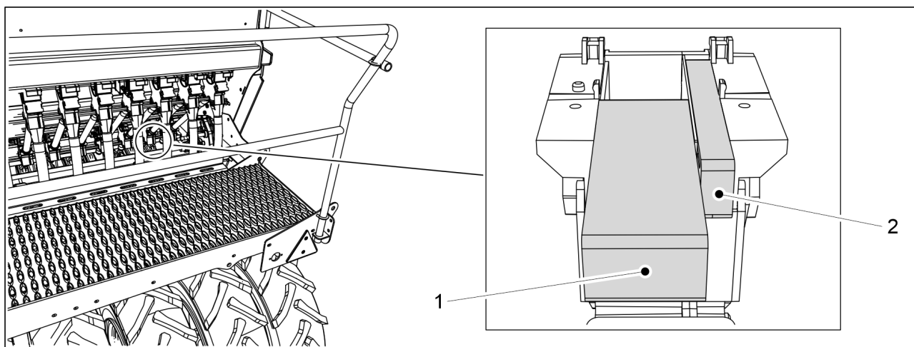
Bild. 6.6.7.2 - 166. Avstängningsplattans positioner
