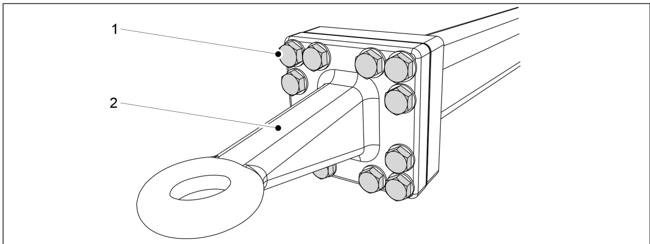
Bild. 7.7.1.2 - 317. Dragögla
