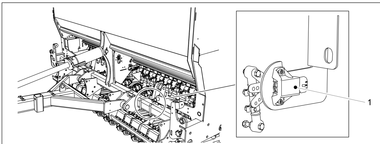
Bild. 4.1.1.9 - 23. Såbillstrycksensor
