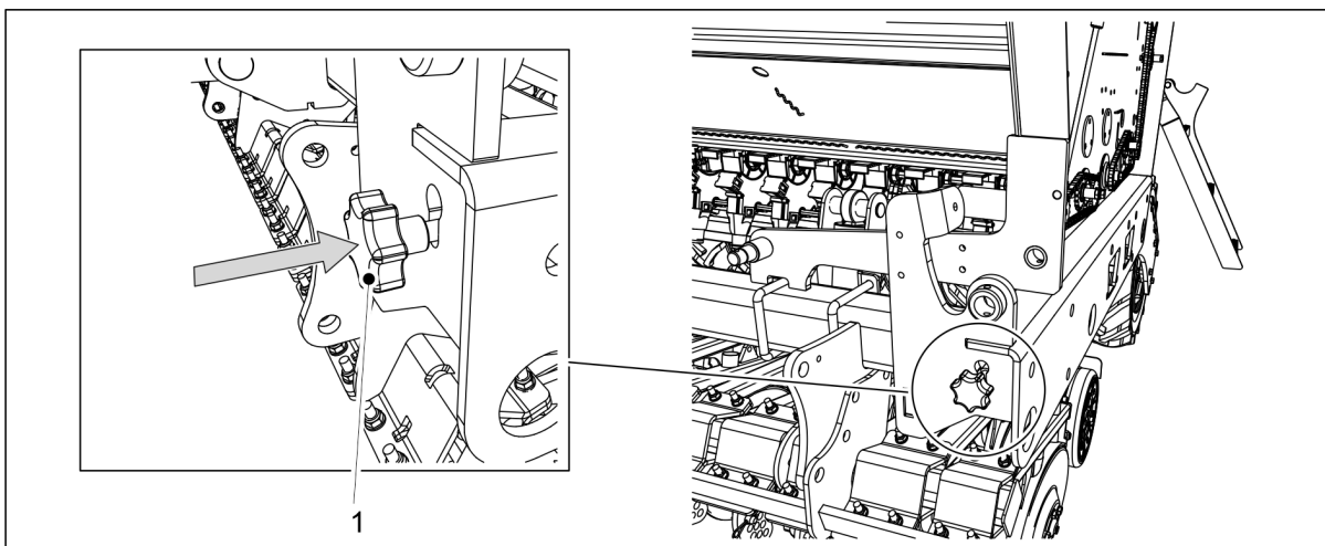
Bild. 6.8.2 - 196. Sätta in kalibreringsprovets justerstång
