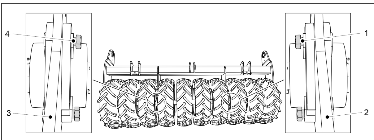
Bild. 7.4.1 - 302. Vrida skruvarna
