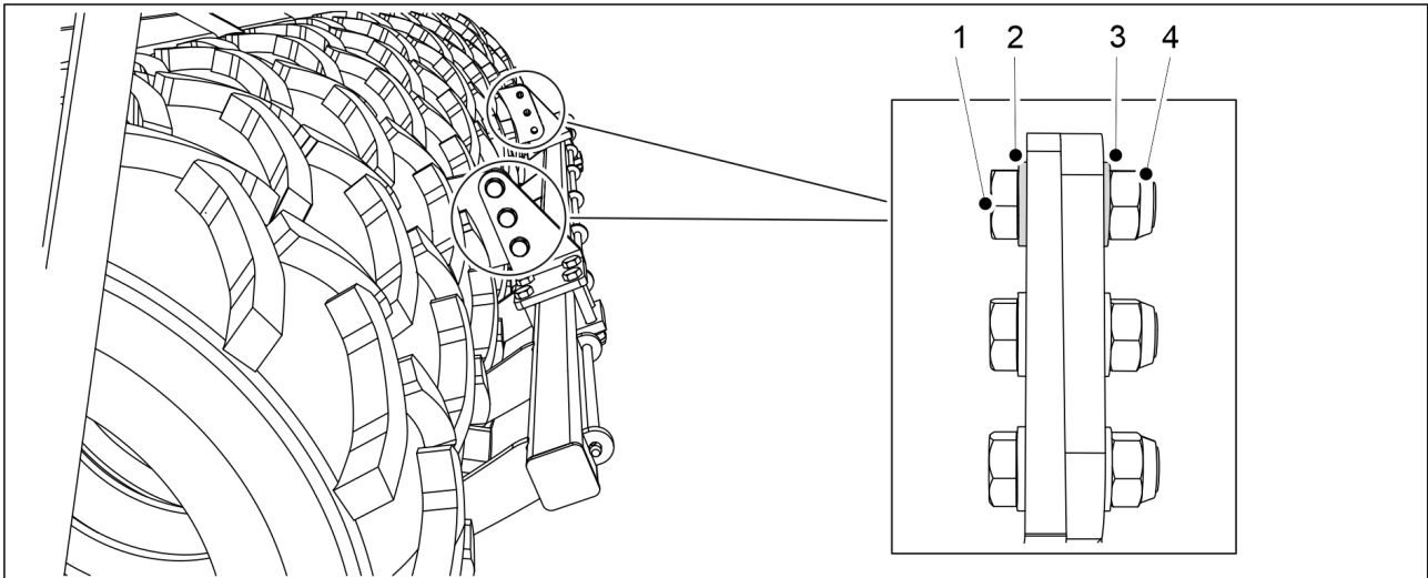
Bild. 7.4.1 - 296. Demontering av skrapan
