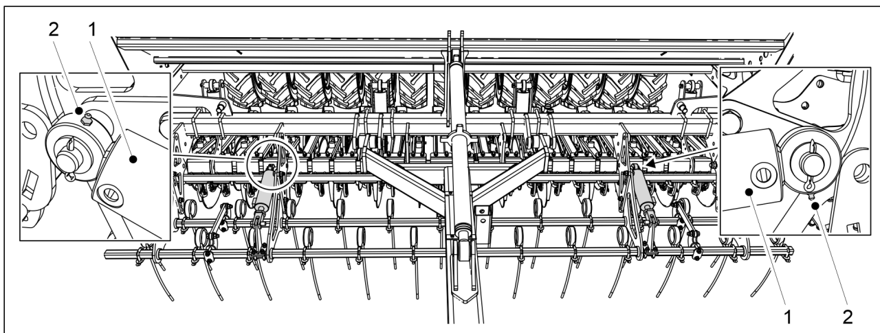
Bild. 7.2.12 - 284. Cylindrar hos den främre harven
