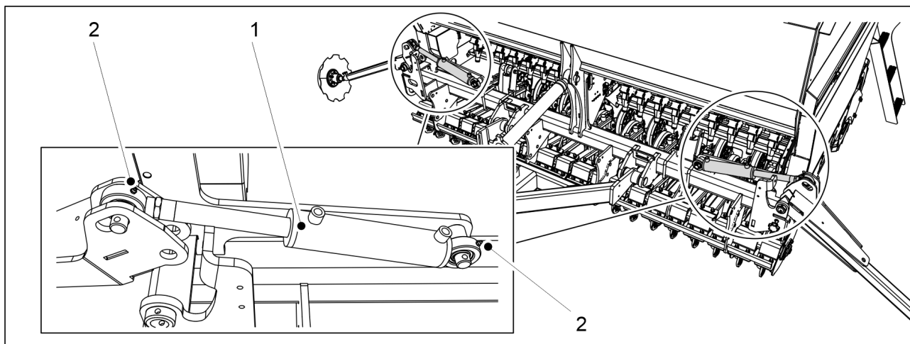
Bild. 7.2.8 - 278. Cylindrar hos de mellersta markörerna.
