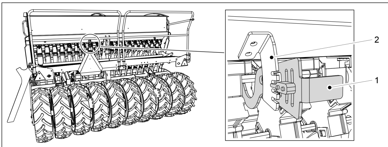
Bild. 6.6.8.1 - 170. Reglerspak för matarnas bottenflikar, småfröbehållare
