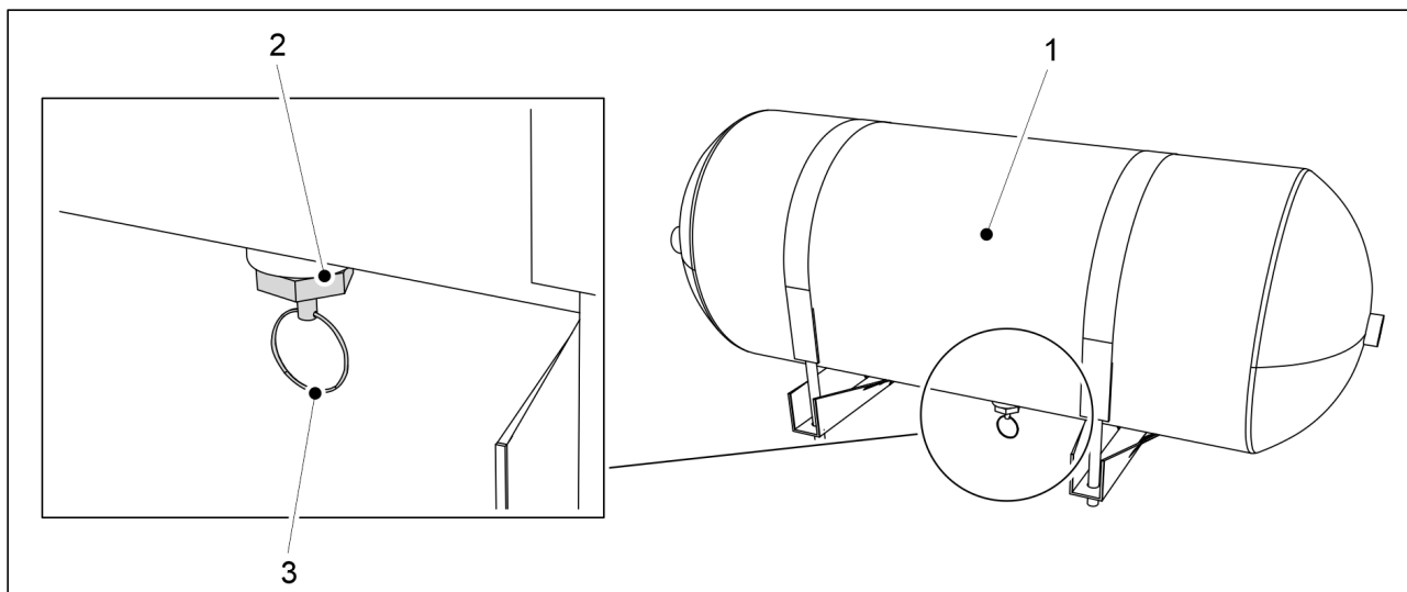
Bild. 7.1.10.2 - 271. Tömning av vatten från den pneumatiska tanken
