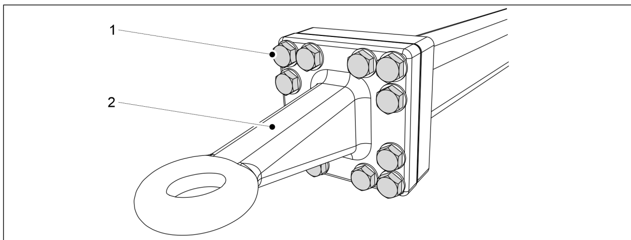
Bild. 7.7.1.1 - 316. Dragögla
