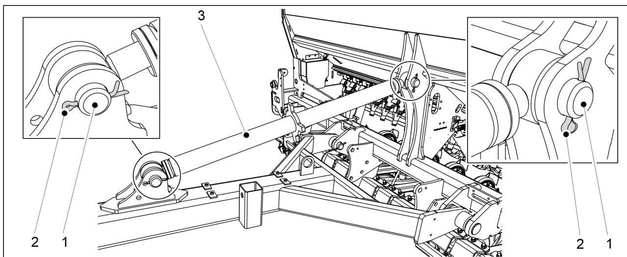
Bild. 5.1.3 - 58. Vantskruv
