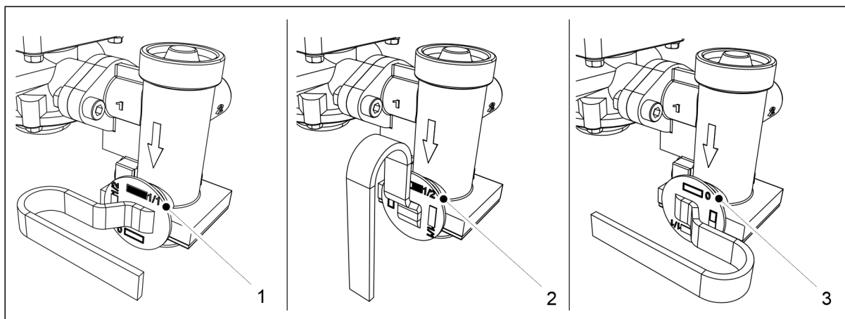
Bild. 6.22.3 - 245. Lägen för bromskraftsregleringsventillen
