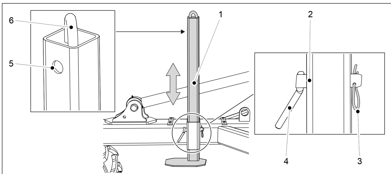
Bild. 5.3.2 - 116. Markutrustning
