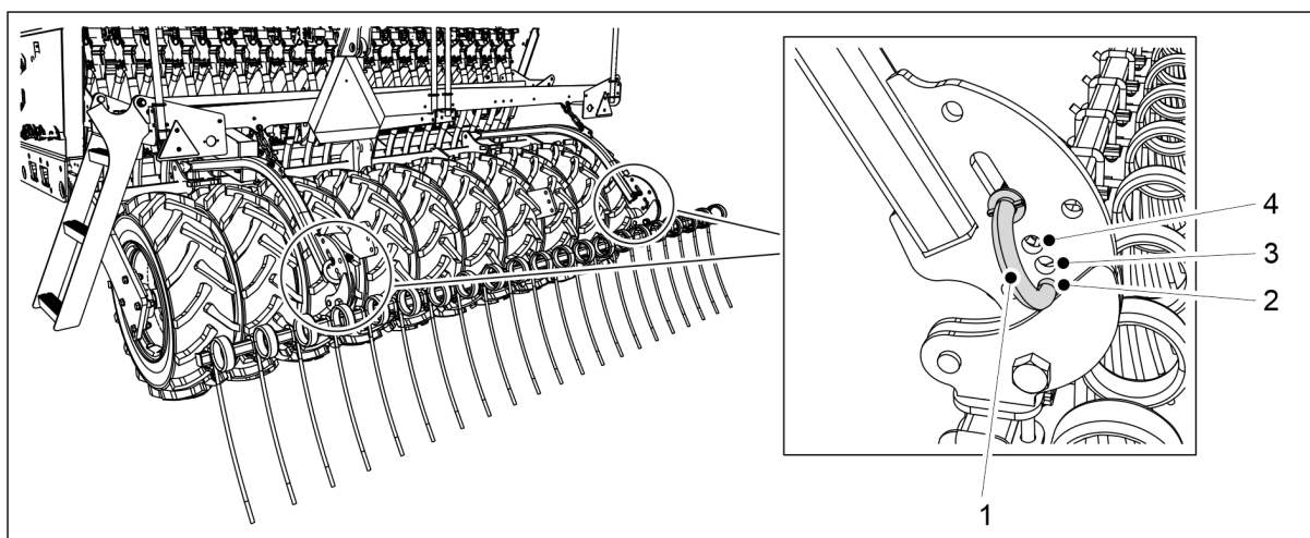
Bild. 6.14 - 229. Justering av efterharvens vinkel
