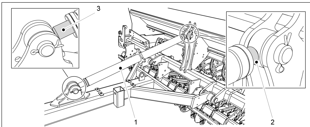
Bild. 7.2.15 - 287. Vantskruv
