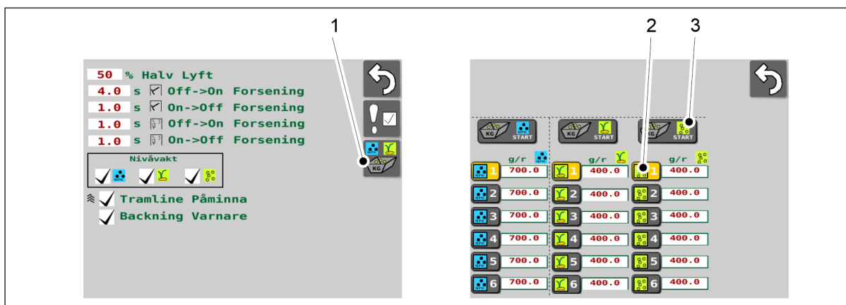
Bild. 6.8.3 - 199. Starta kalibreringsprovet
