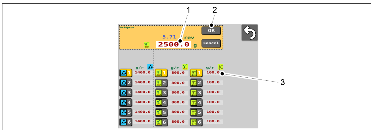
Bild. 6.8.3 - 204. Skriva in vägningsresultatet
