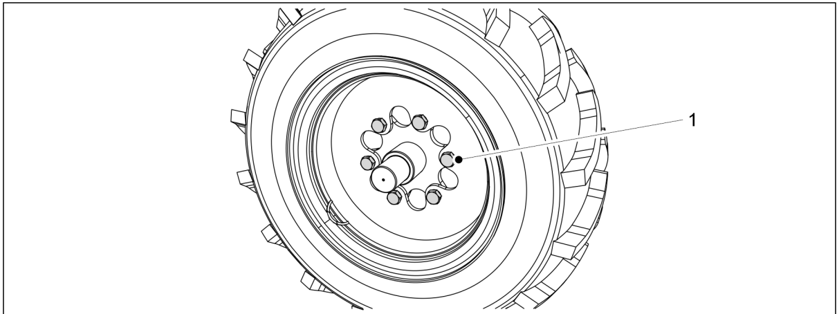
Bild. 7.4.2 - 305. Lossa skruvarna
