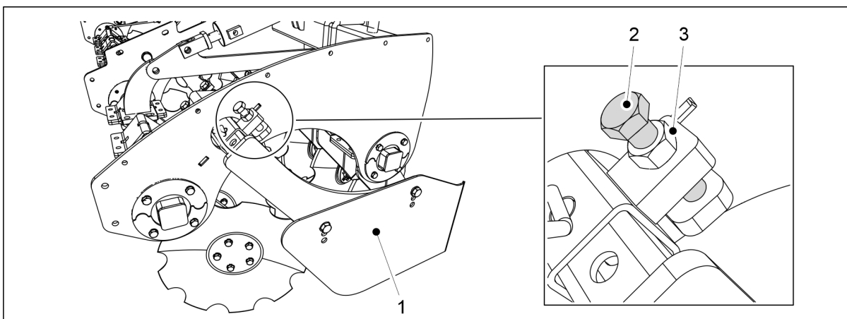
Bild. 6.17 - 234. Justering av det nedre läget för sidobegränsare
