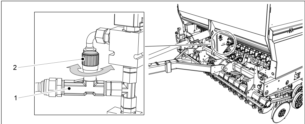
Bild. 5.3.7 - 125. Justera mittmarkörernas lyfthastighet
