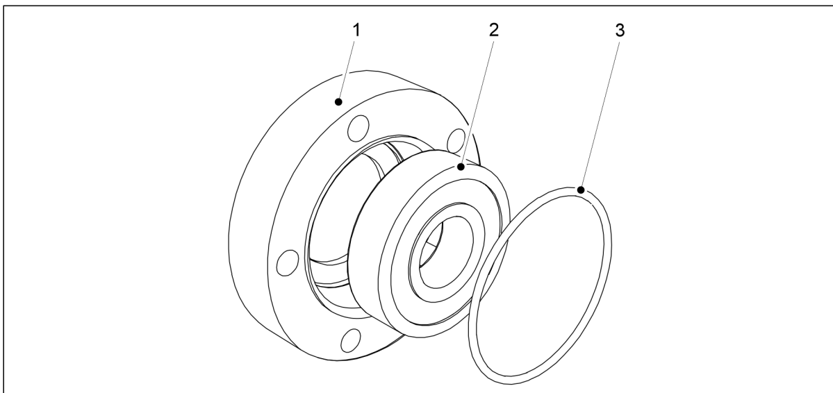
Bild. 7.8.3.1 - 328. Borttagning av lagret och O-ringen
