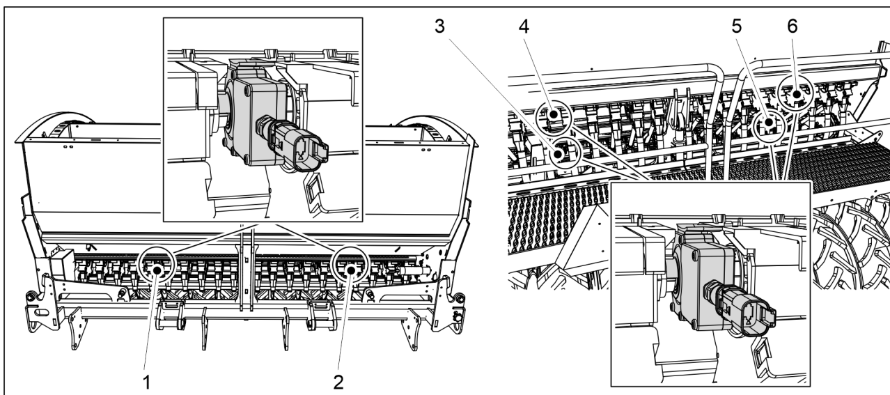
Bild. 4.1.1.7 - 20. Position hos körspårskopplingar
