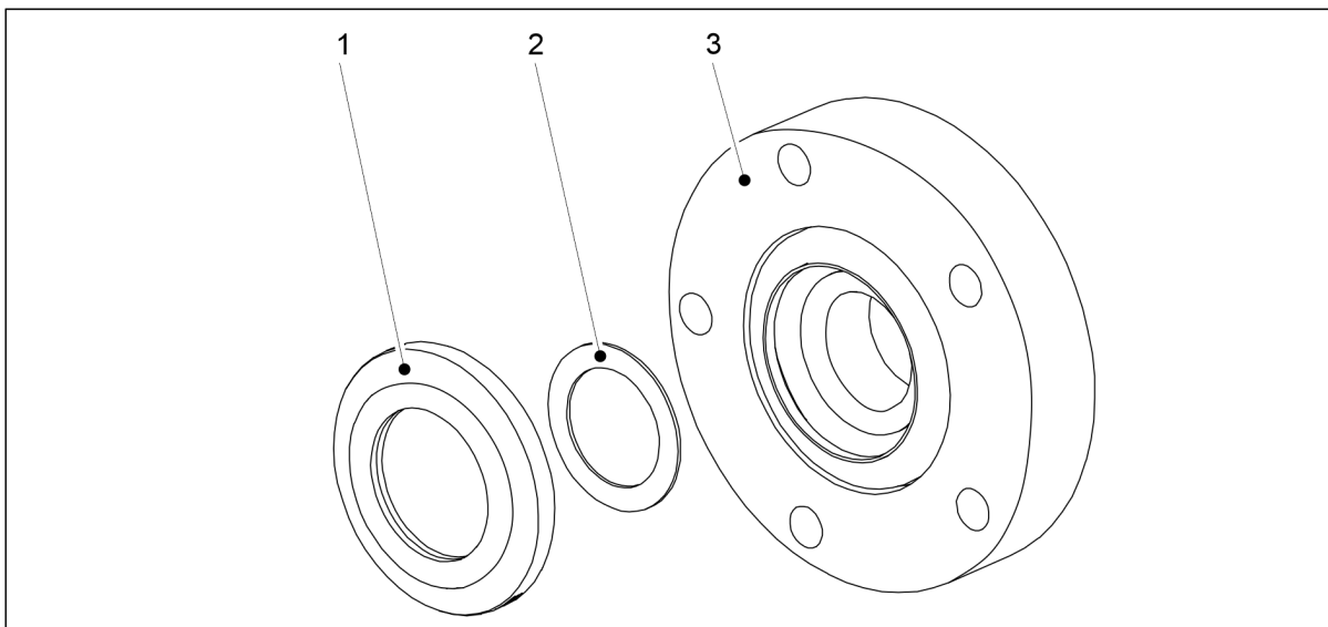
Bild. 7.8.3.2 - 330. Lagertätning och lagerring
