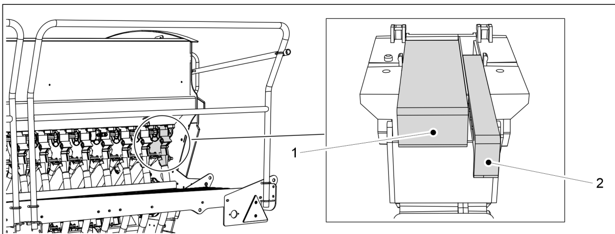
Bild. 6.6.8.2 - 172. Avstängningsplattans positioner
