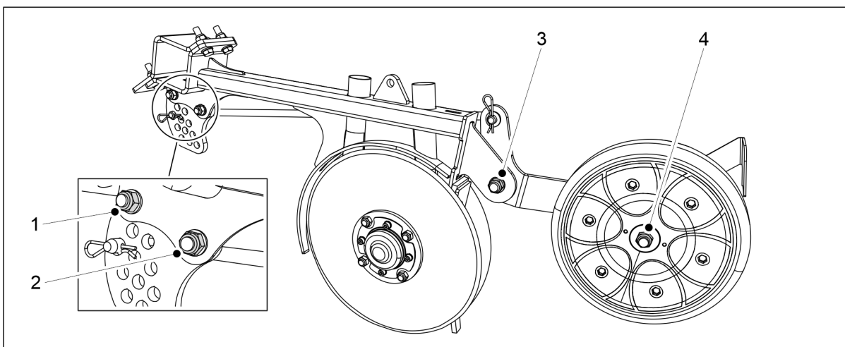
Bild. 7.1.2.4 - 260. Skruvar hos såbillstäckhjulet och djupjustering
