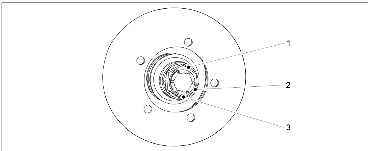
Bild. 7.6.1 - 315. Åtdragning av hjulpackarens lager
