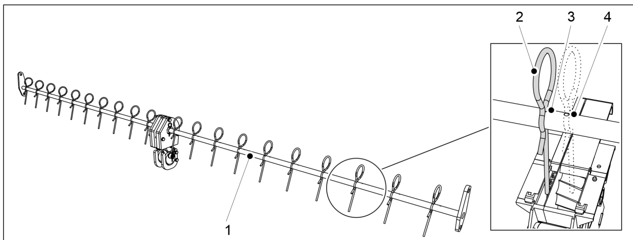
Bild. 6.19.3 - 241. Pendelspridare för småfrön
