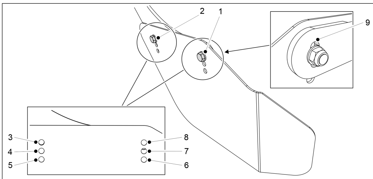
Bild. 6.17 - 235. Justering av sidobegränsarnas höjd och vinkel
