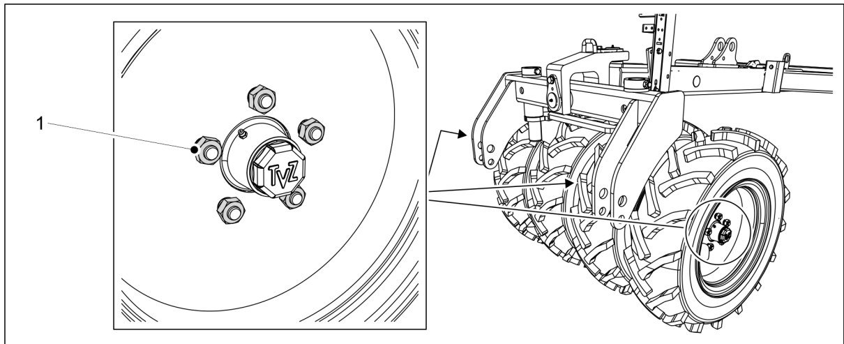
Bild. 7.1.2.3 - 257. Hjulpackarens skruvar
