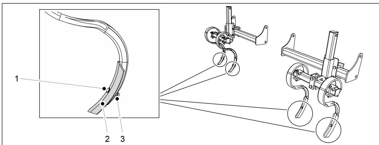
Bild. 6.18.2 - 238. Byta ut en S-pinnspets
