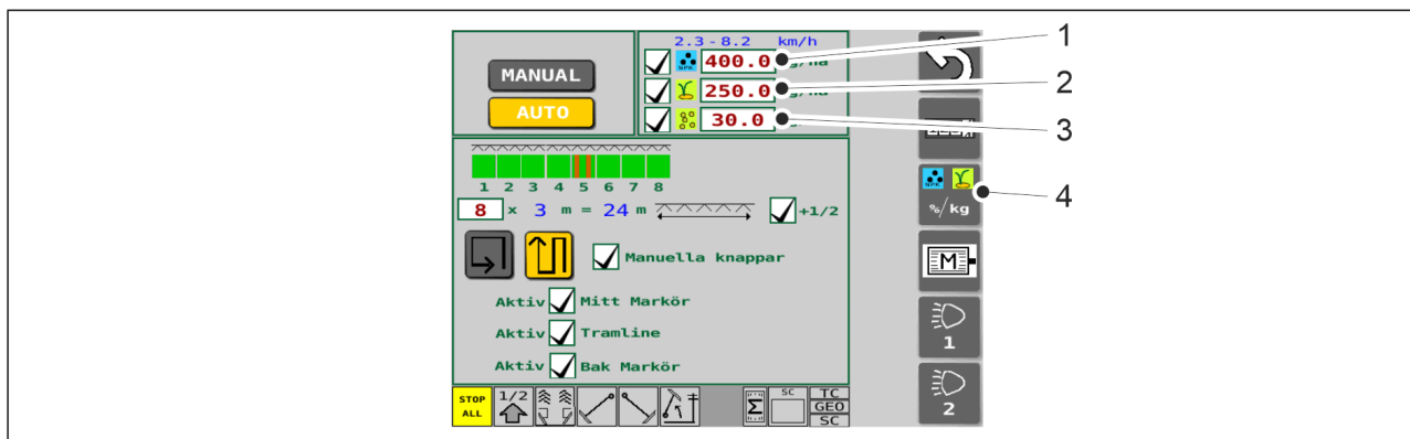
Bild. 6.3.4 - 133. Målhastigheter
