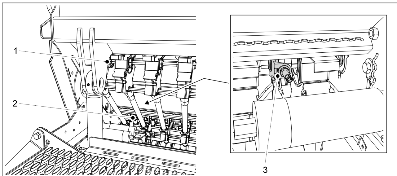
Bild. 4.1.1.5 - 17. Placering av en drivaxels rotationsvakter
