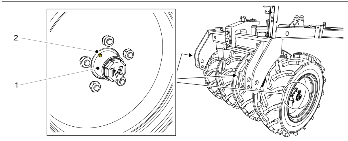
Bild. 7.2.10 - 282. Hjulpackarens hjulnav
