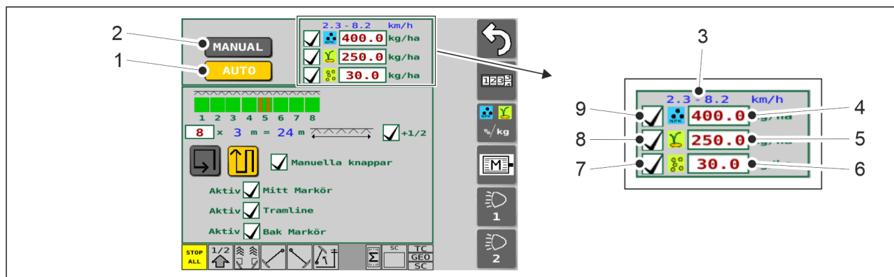
Bild. 4.1.3.1 - 41. Skärmbild för inställningar för utsäde, överst
