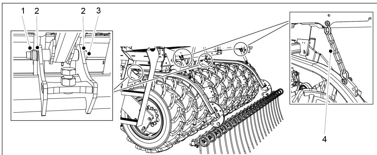
Bild. 7.4.1 - 298. Demontering av efterharven
