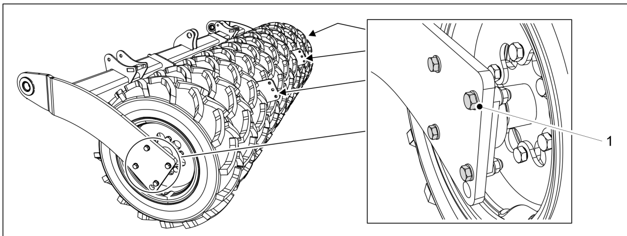
Bild. 7.4.4 - 308. Montering av hjulet
