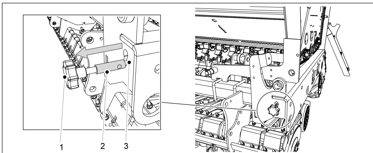
Bild. 6.8.1 - 179. Dra ut kalibreringsprovets justerstång
