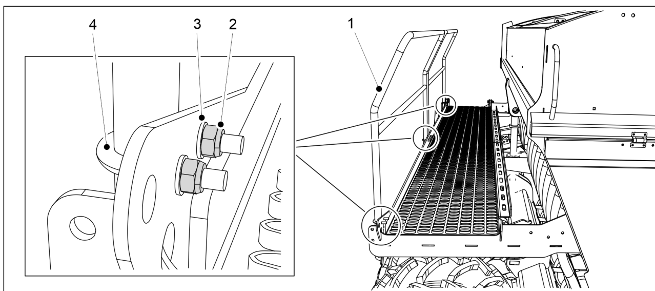
Bild. 5.1.17 - 103. Vända arbetsplattformens bakre räcke
