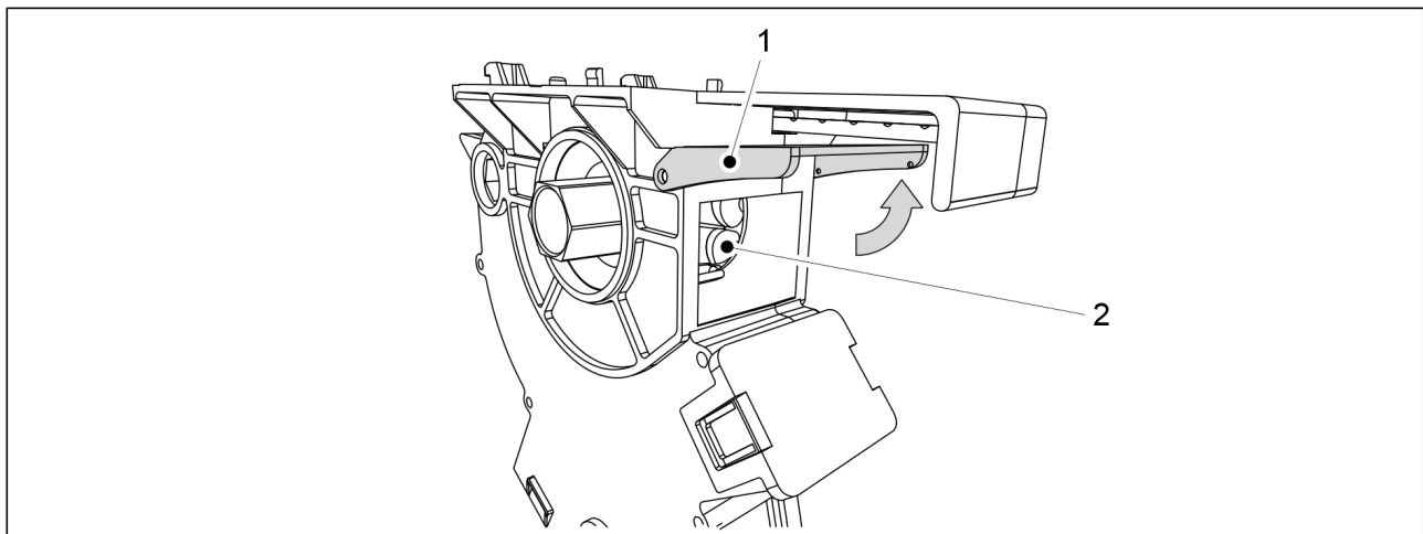
Bild. 7.3.6 - 295. Rengöring av matarenheterna i småfröbehållaren
