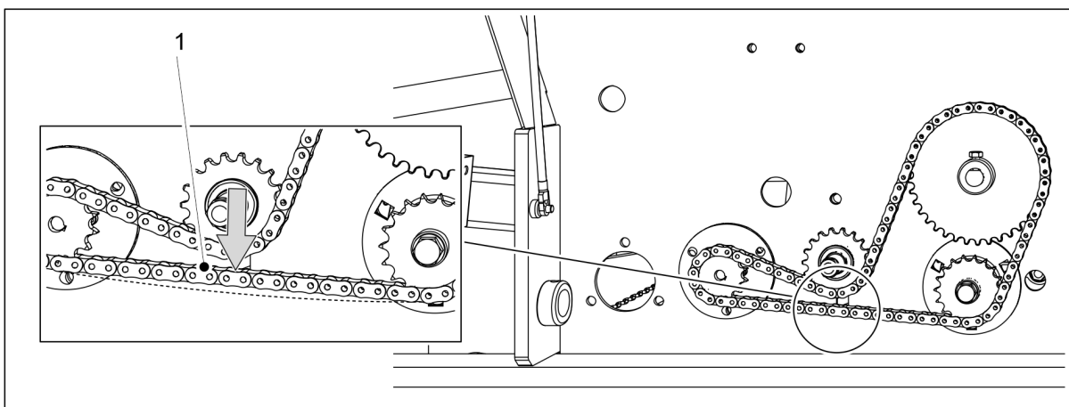
Bild. 7.1.5.3 - 267. Kontrollera kedjespänningen, transmission hos gödningsmedlets spridaraxel
