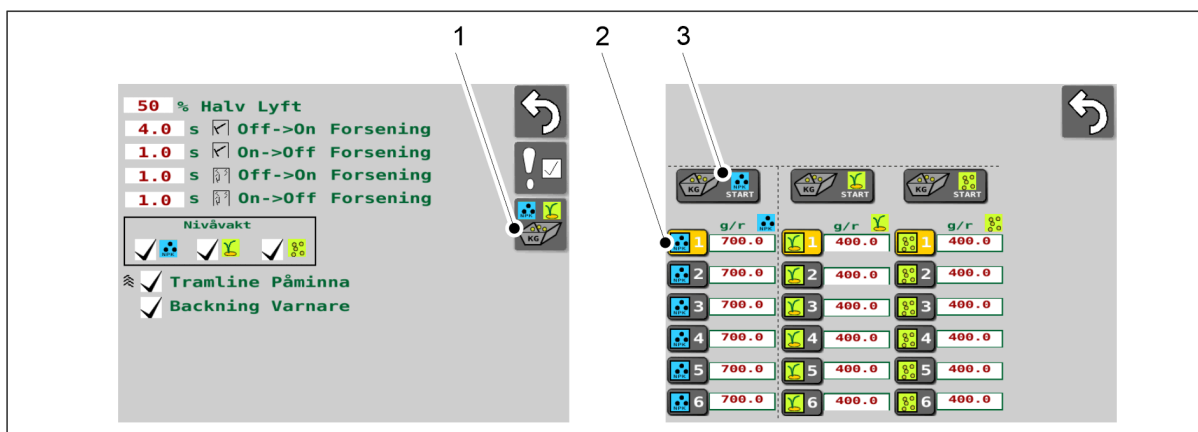
Bild. 6.8.1 - 181. Starta kalibreringsprovet
