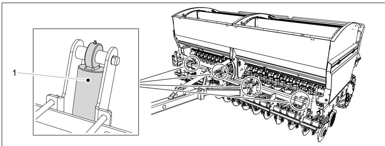
Bild. 7.2.3 - 274. Smörjning av såbillstryckcylindern
