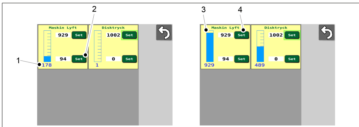
Bild. 7.9.1.2 - 336. Kalibrering av såbillstrycksensorn
