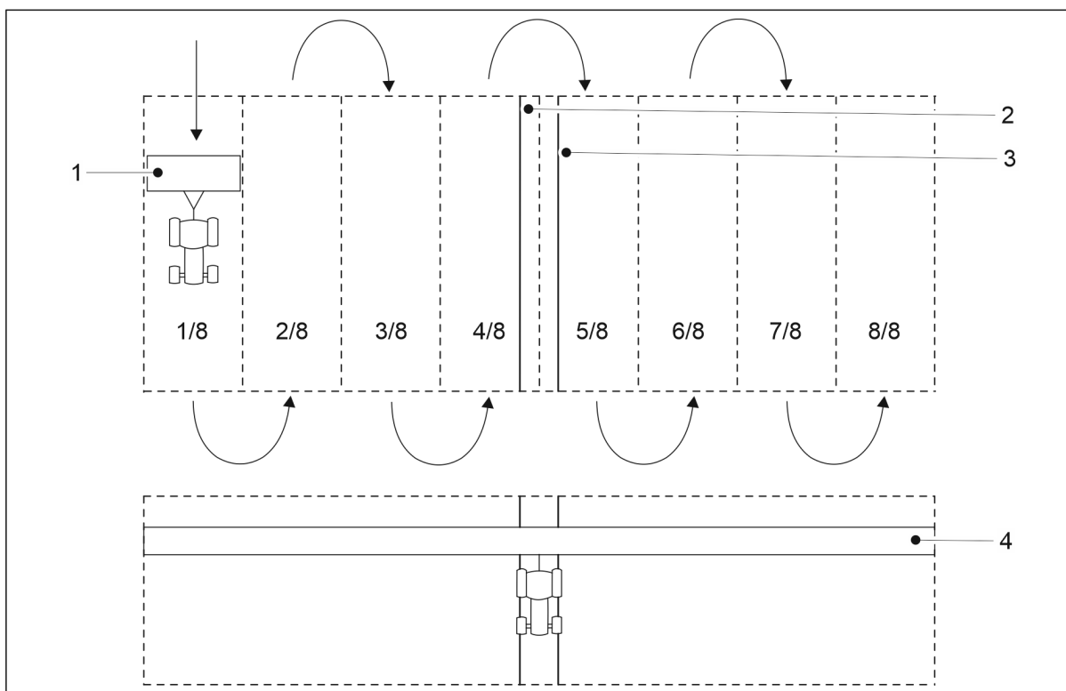
Bild. 5.2.1.1 - 106. Asymmetriska körspår
