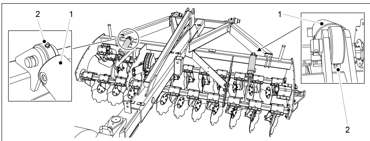
Bild. 7.2.13 - 285. Cylindrar hos den främre tallrikskultivatorn
