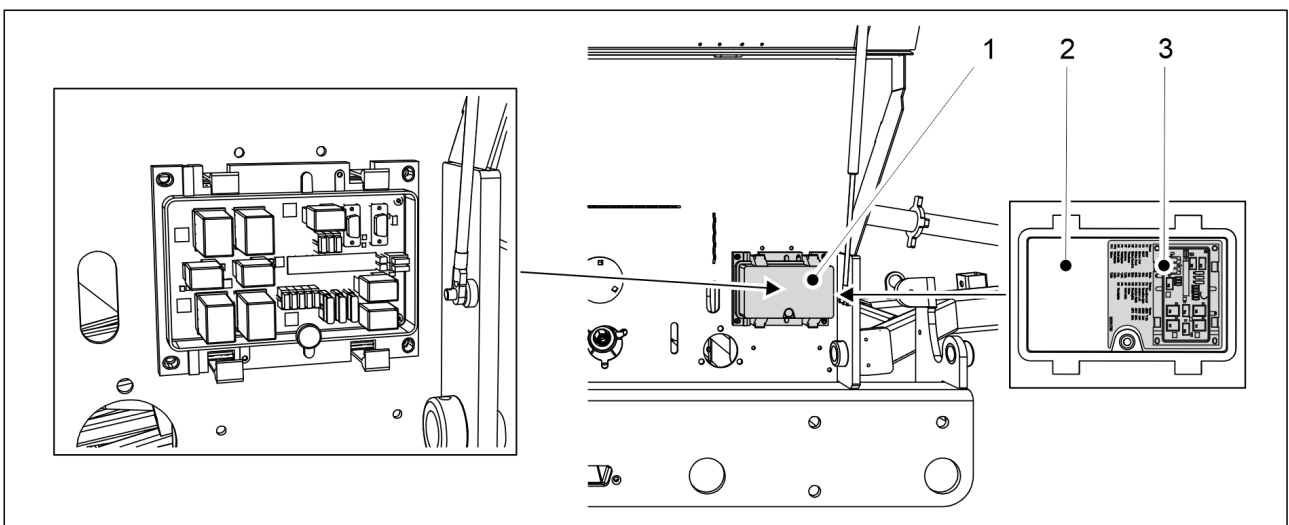
Bild. 4.1.1.2 - 14. Säkring och relädosor
