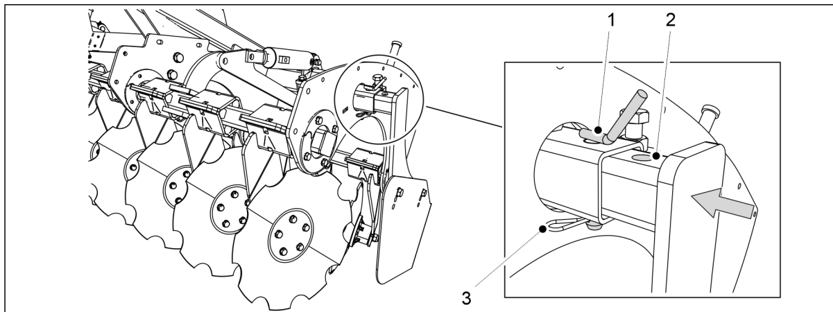
Bild. 6.17 - 236. Justering av den främre tallrikskultivatorns sidobegränsare för transport
