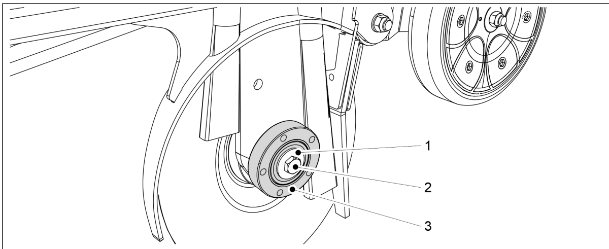
Bild. 7.8.2.1 - 324. Demontering av lagerhuset
