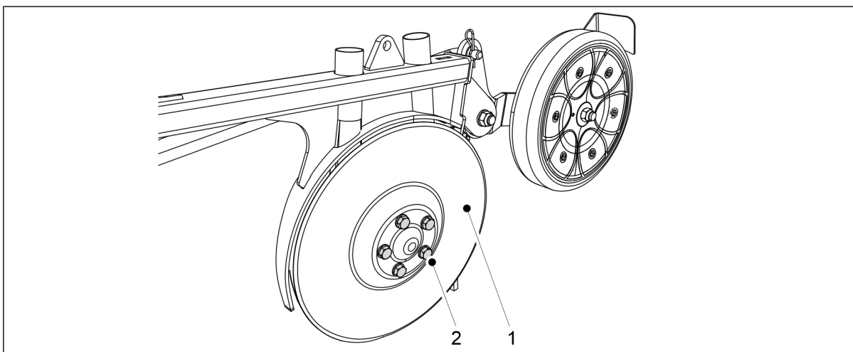
Bild. 7.8.2.2 - 326. Montera en skiva
