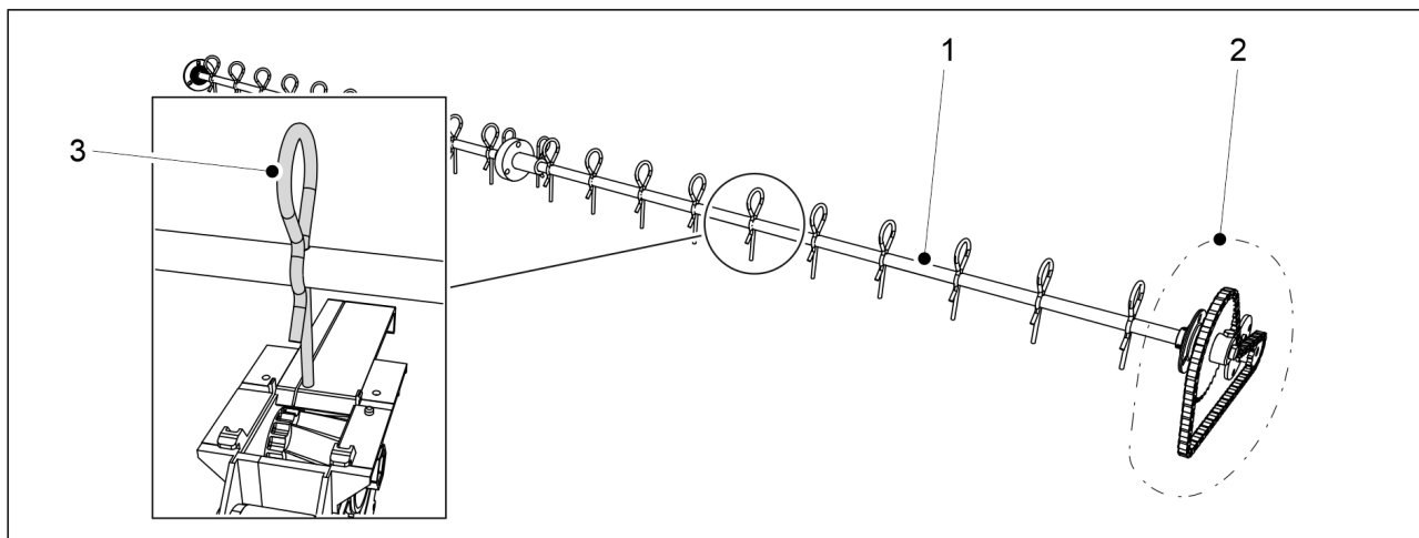
Bild. 6.19.2 - 240. Utsädets spridaraxel
