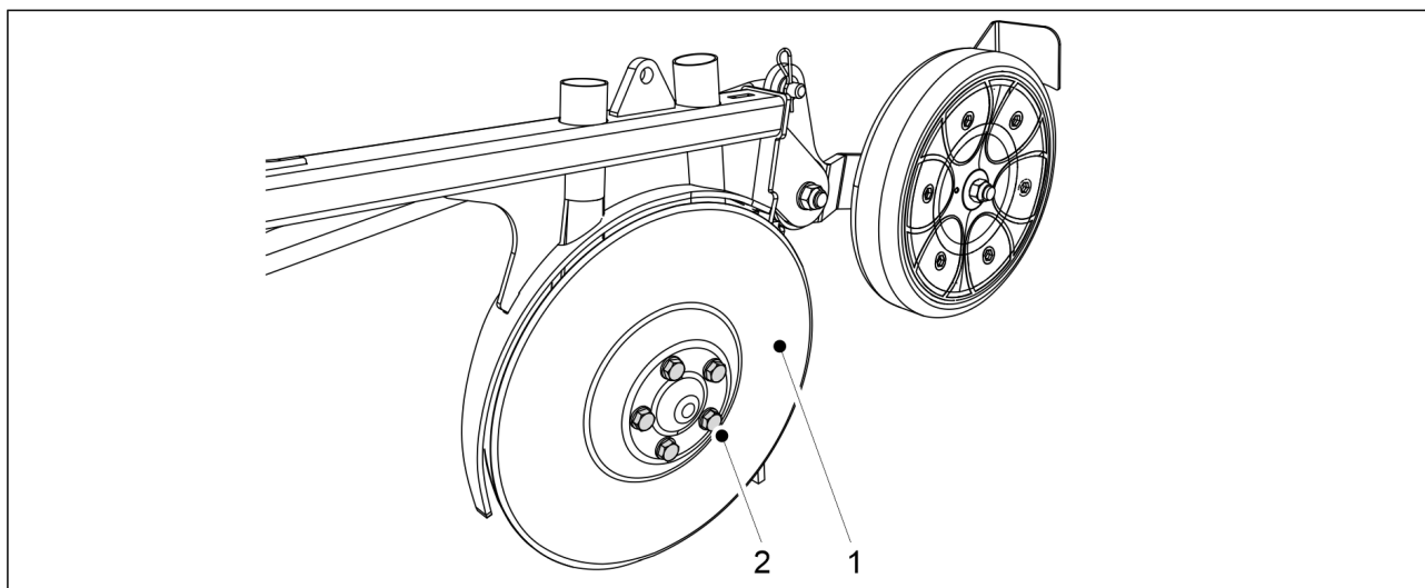
Bild. 7.8.2.1 - 323. Lossa en skiva
