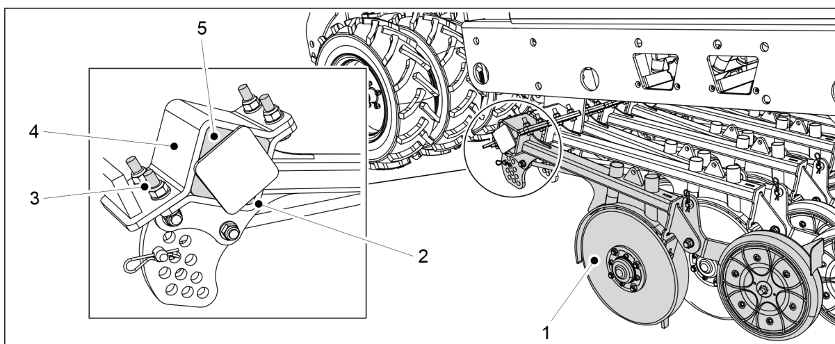
Bild. 7.8.1.2 - 321. Fästa såbillen
