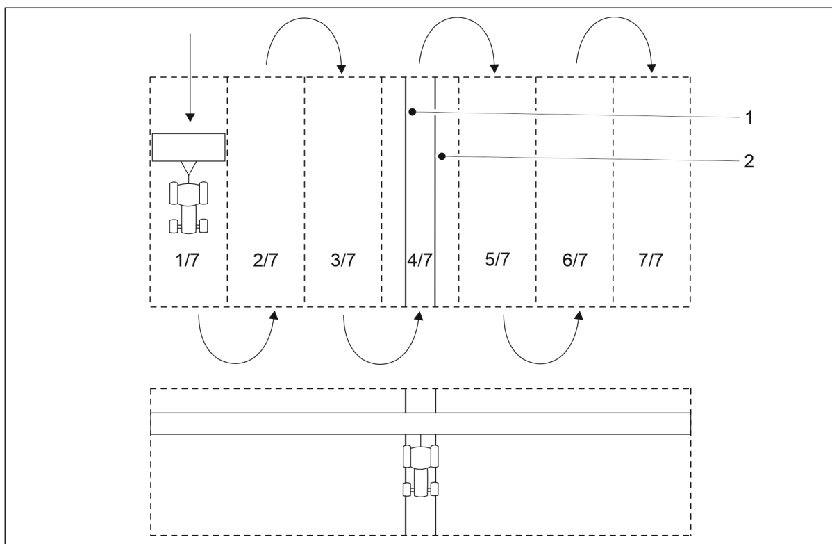
Bild. 5.2.1.2 - 110. Symmetriska körspår
