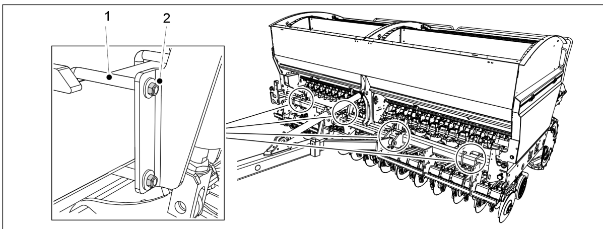
Bild. 7.1.2.4 - 259. Skruvar för såbillstryck
