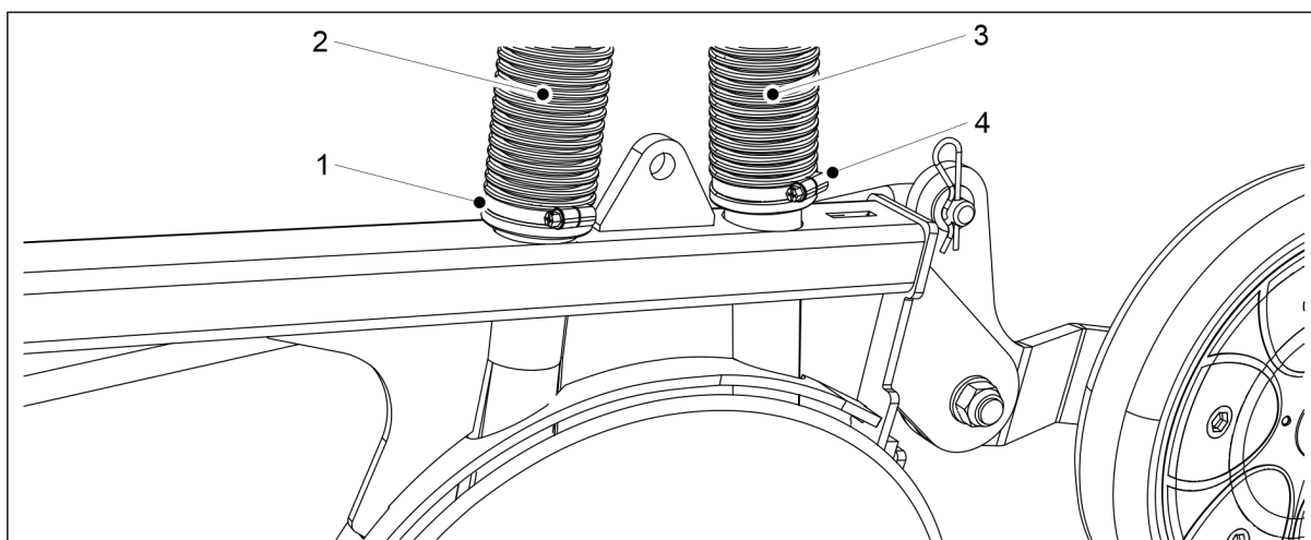
Bild. 7.8.1.1 - 319. Koppla från såbillsslanger
