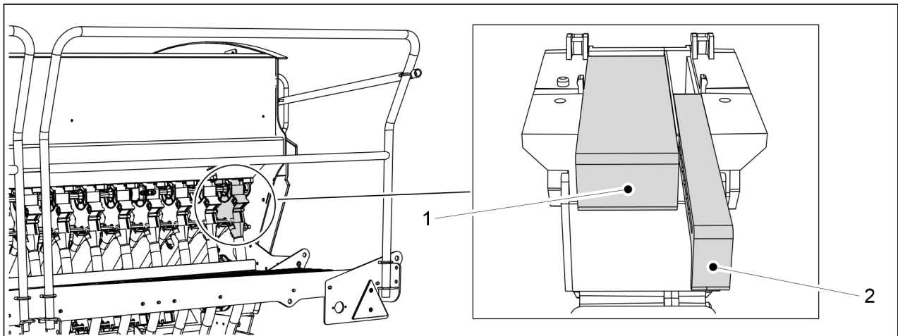
Bild. 6.6.8.2 - 173. Avstängningsplattans positioner
