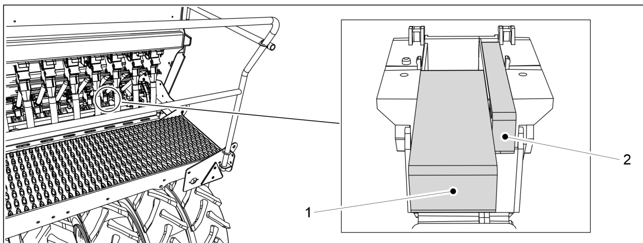
Bild. 6.6.7.2 - 167. Avstängningsplattans positioner
