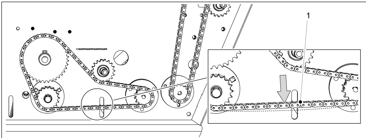
Bild. 7.1.5.4 - 268. Kontroll av kedjespänning, transmission hos utsädens spridaraxel
