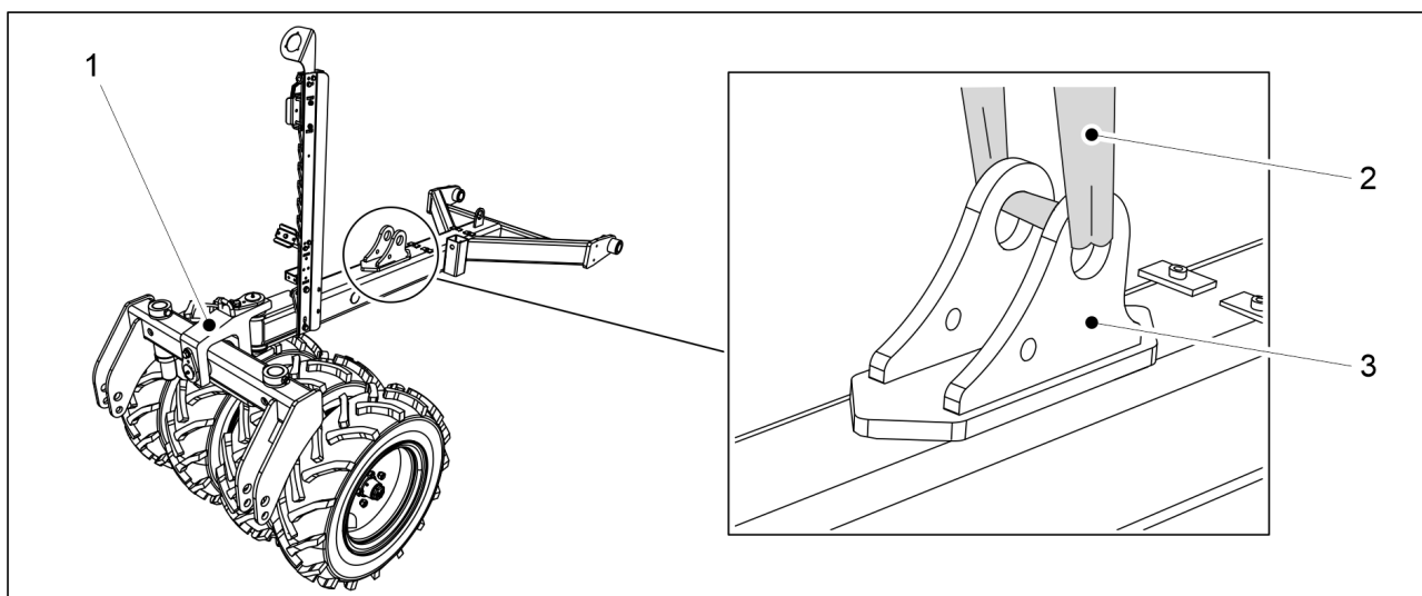
Bild. 5.1.1 - 53. Lyfta hjulpackaren
