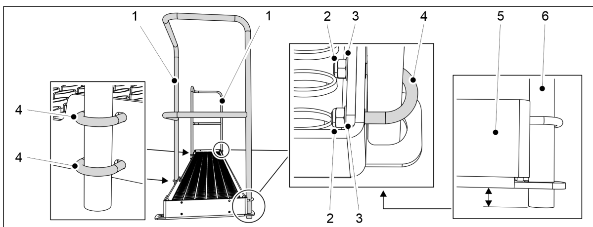
Bild. 5.1.16 - 101. Montering av räcken på en 400-maskin
