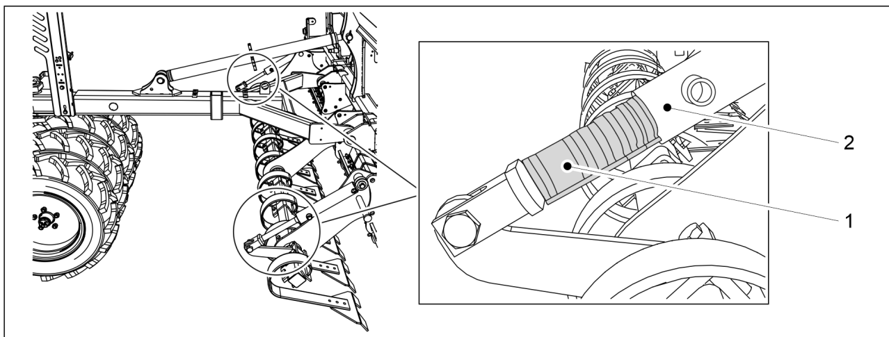
Bild. 6.15 - 230. Justering av den främre utjämningsharven
