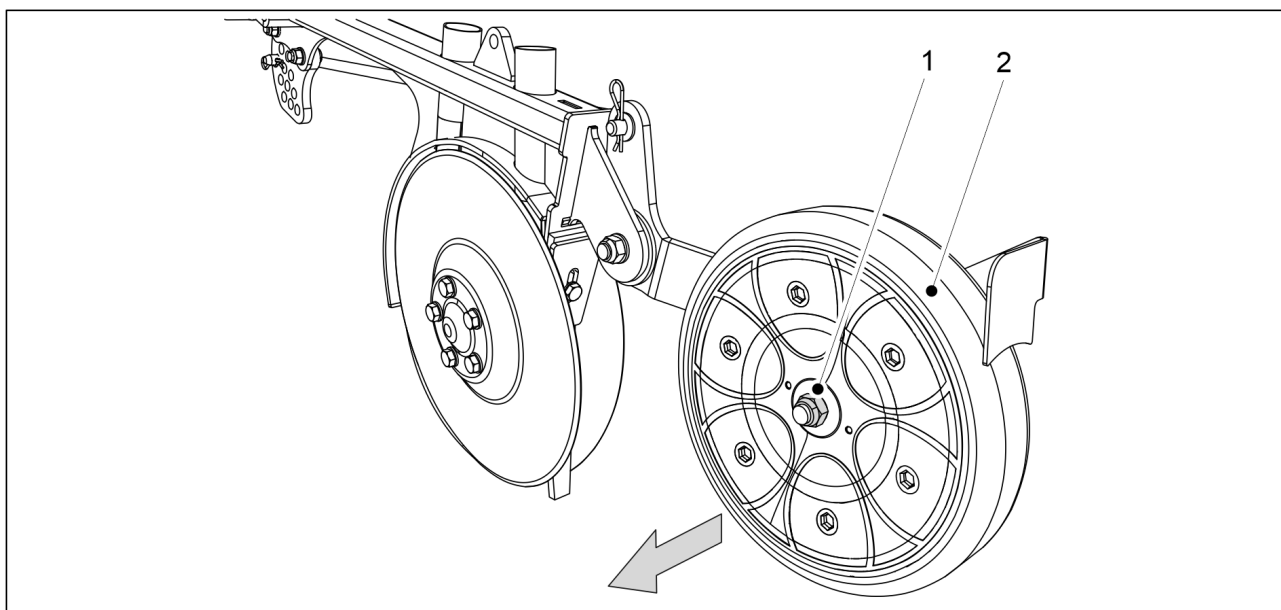
Bild. 7.8.4.1 - 331. Demontering av täckhjulet
