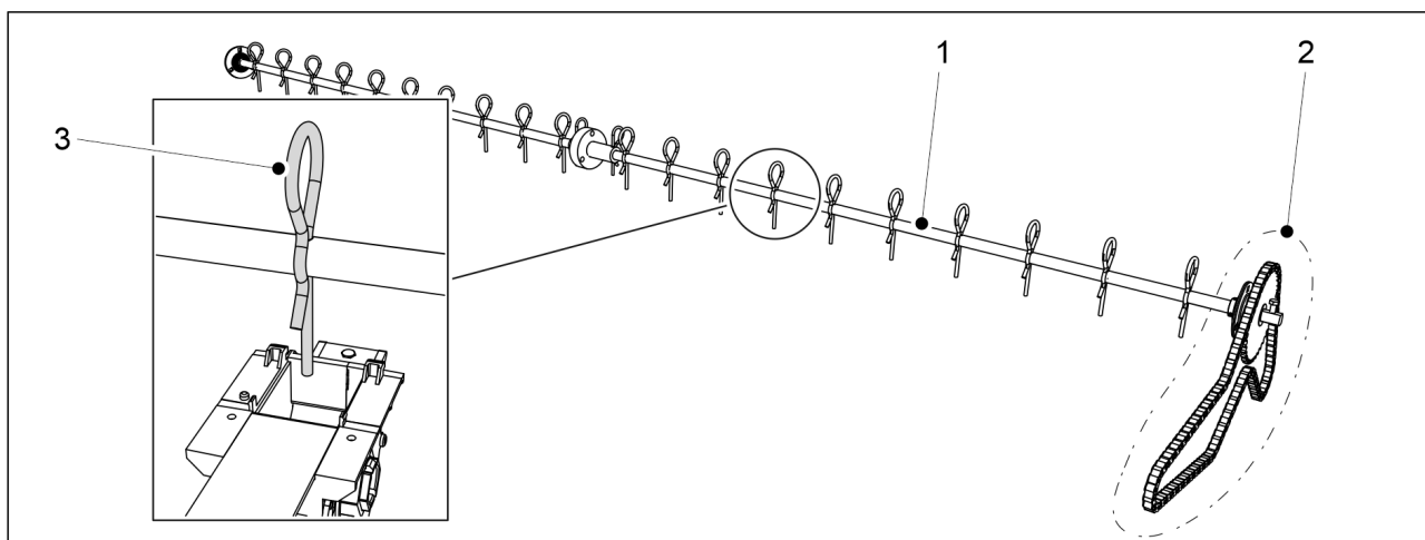
Bild. 6.19.1 - 239. Gödningsmedlets spridaraxel
