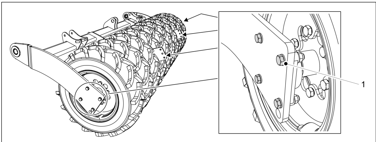
Bild. 7.4.1 - 301. Demontering av hjulet
