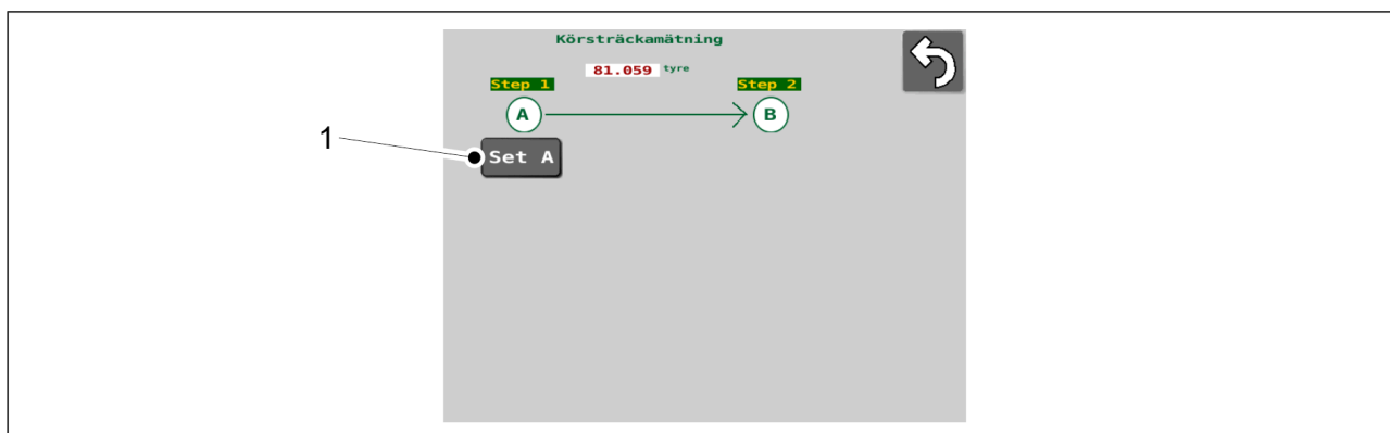
Bild. 7.9.2.1 - 337. Kör kalibrering 1
