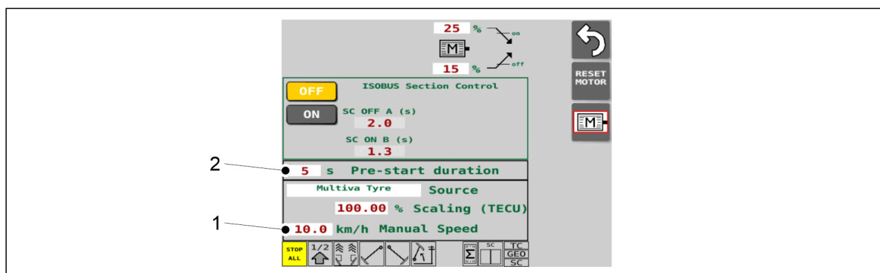
Bild. 6.9 - 206. Inställningar för funktionen PRESTART
