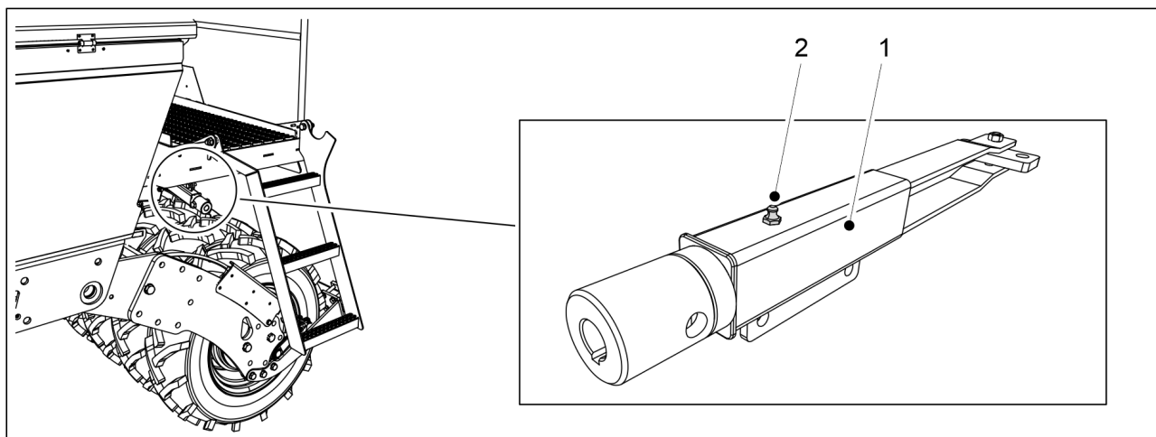
Bild. 7.2.17 - 289. Parkeringsbromsvev
