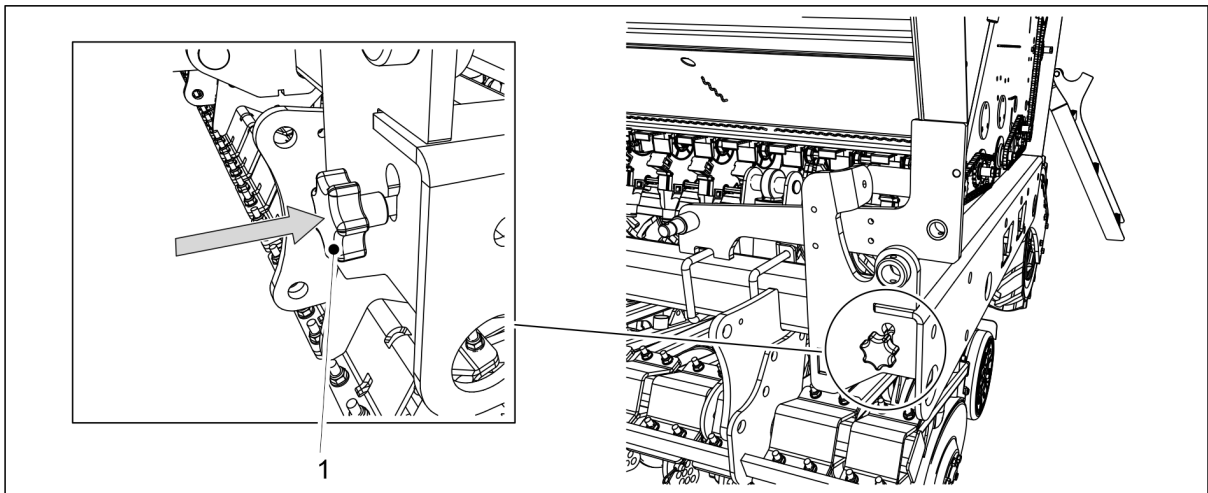
Bild. 6.8.1 - 187. Sätta in kalibreringsprovets justerstång
