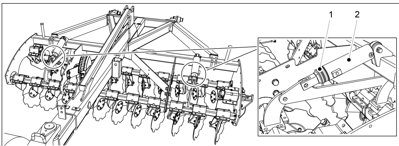
Bild. 6.17 - 233. Justering av den främre tallrikskultivatorns jordbearbetningsdjup
