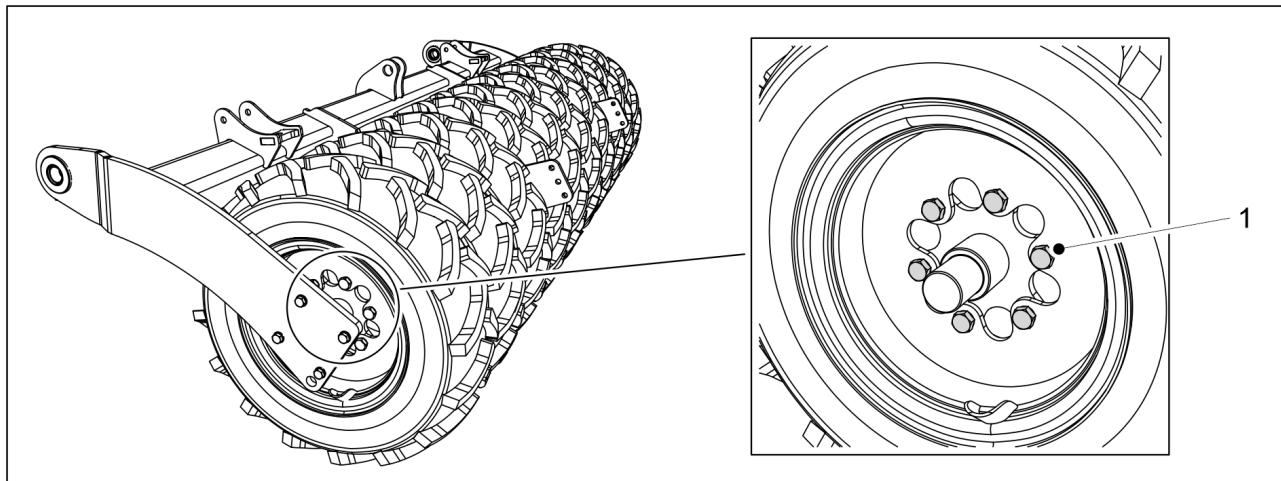
Bild. 7.1.2.1 - 254. Transporthjulens skruvar
