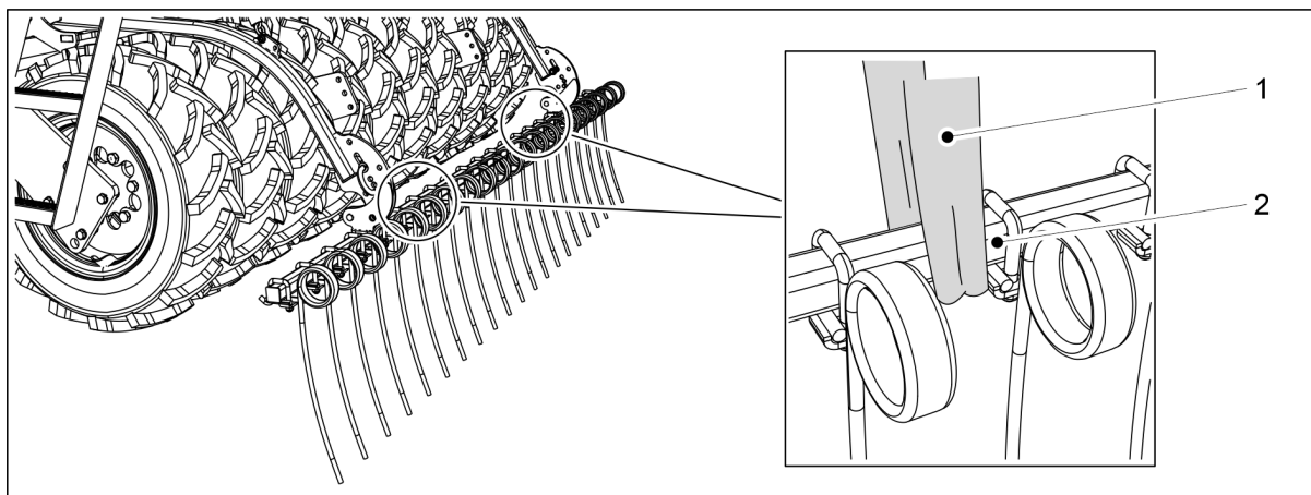
Bild. 7.4.1 - 299. Lyfta efterharven
