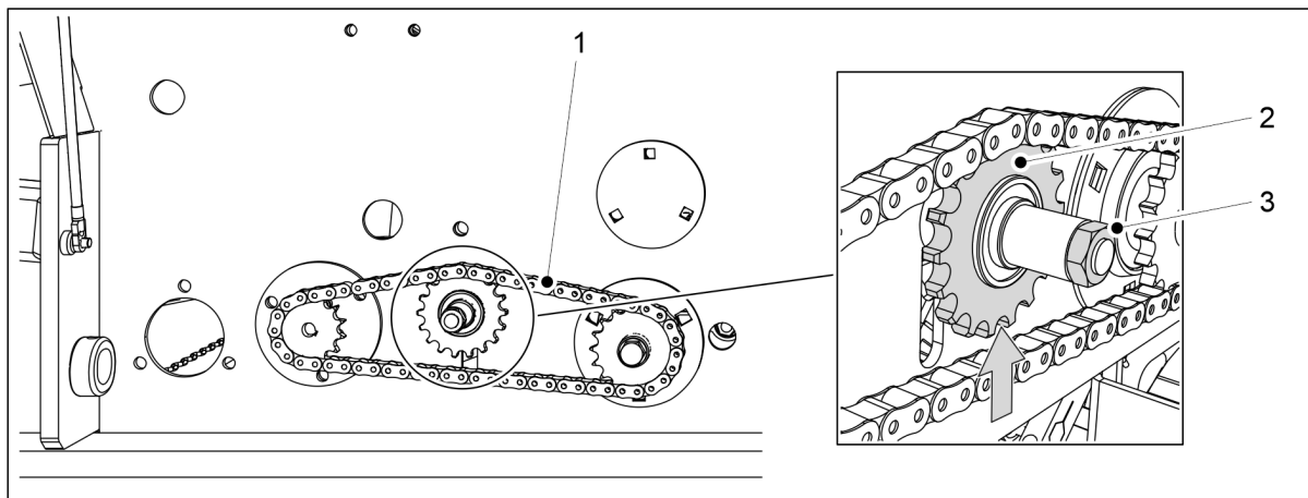
Bild. 7.5.1 - 309. Spänning av gödningsmedelsbehållarens kedja
