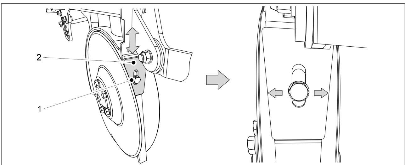
Bild. 7.8.5.1 - 333. Skivskrapa
