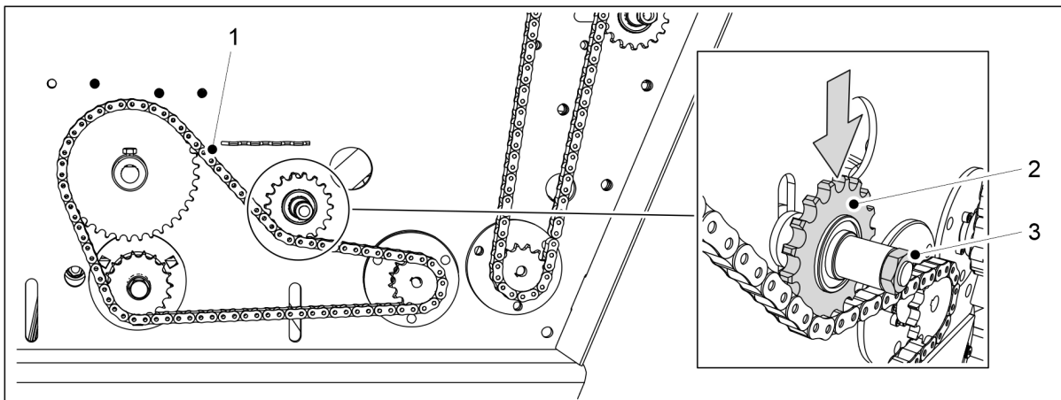
Bild. 7.5.4 - 313. Spänna kedjan hos utsädens spridaraxel
