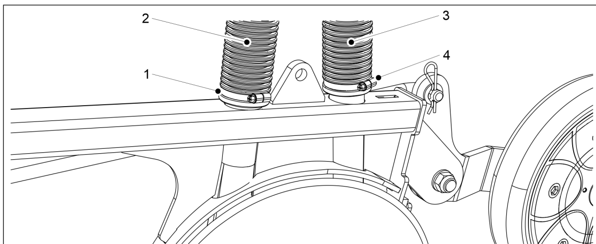
Bild. 7.8.1.2 - 322. Anslutning av såbillsslangar
