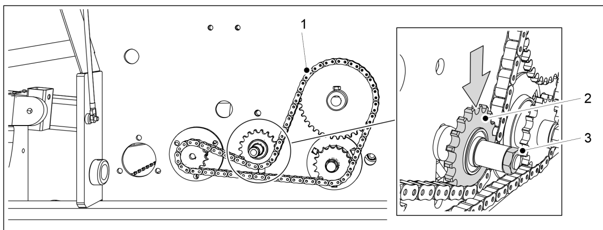
Bild. 7.5.3 - 312. Spänna kedjan på gödningsmedlets spridaraxel
