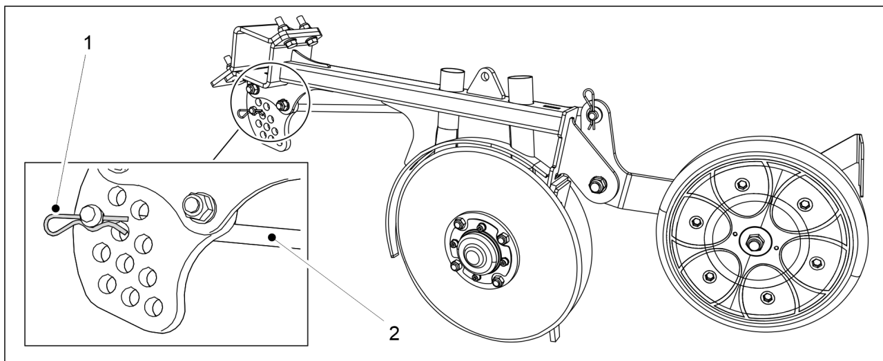
Bild. 6.12 - 226. Justering av såbillens sådjup
