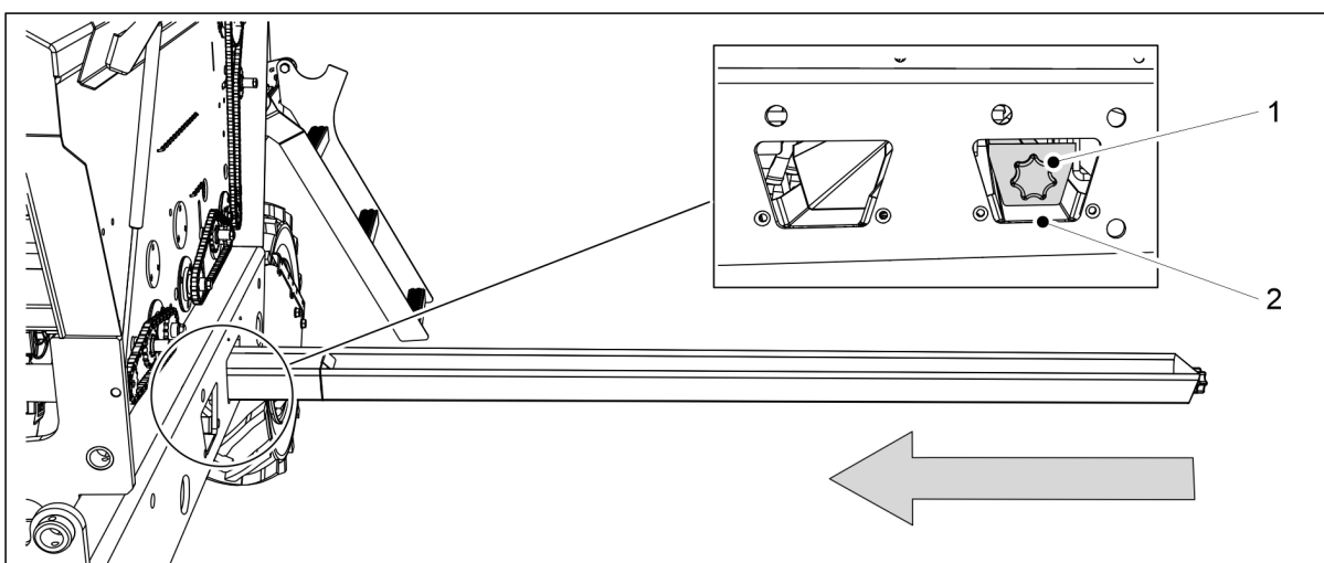
Bild. 6.8.2 - 189. Montera kalibreringsbrickorna
