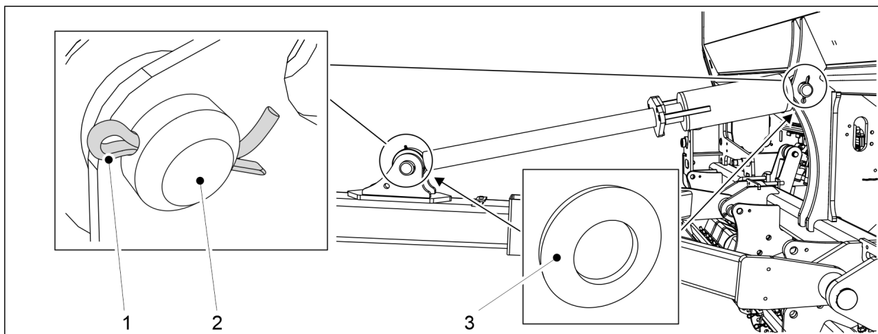
Bild. 5.1.2 - 57. Dragstångscylinder
