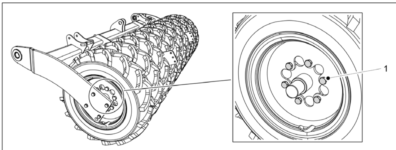
Bild. 7.1.2.1 - 252. Transporthjulens skruvar
