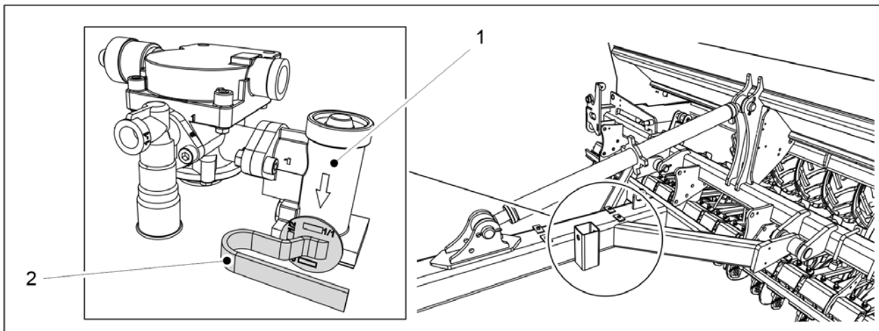
Bild. 6.22.3 - 242. Bromskraftsreglerventil
