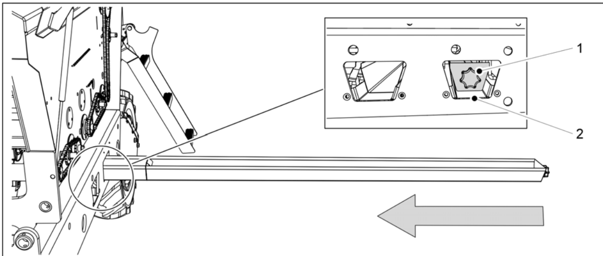
Bild. 6.8.2 - 186. Montera kalibreringsbrickorna
