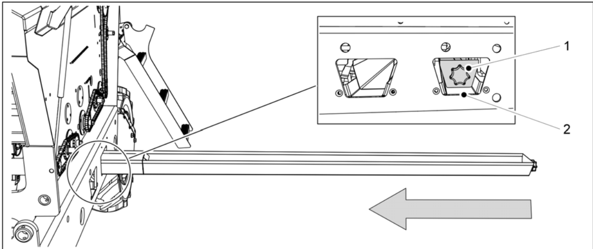
Bild. 6.8.3 - 195. Montera kalibreringsbrickorna
