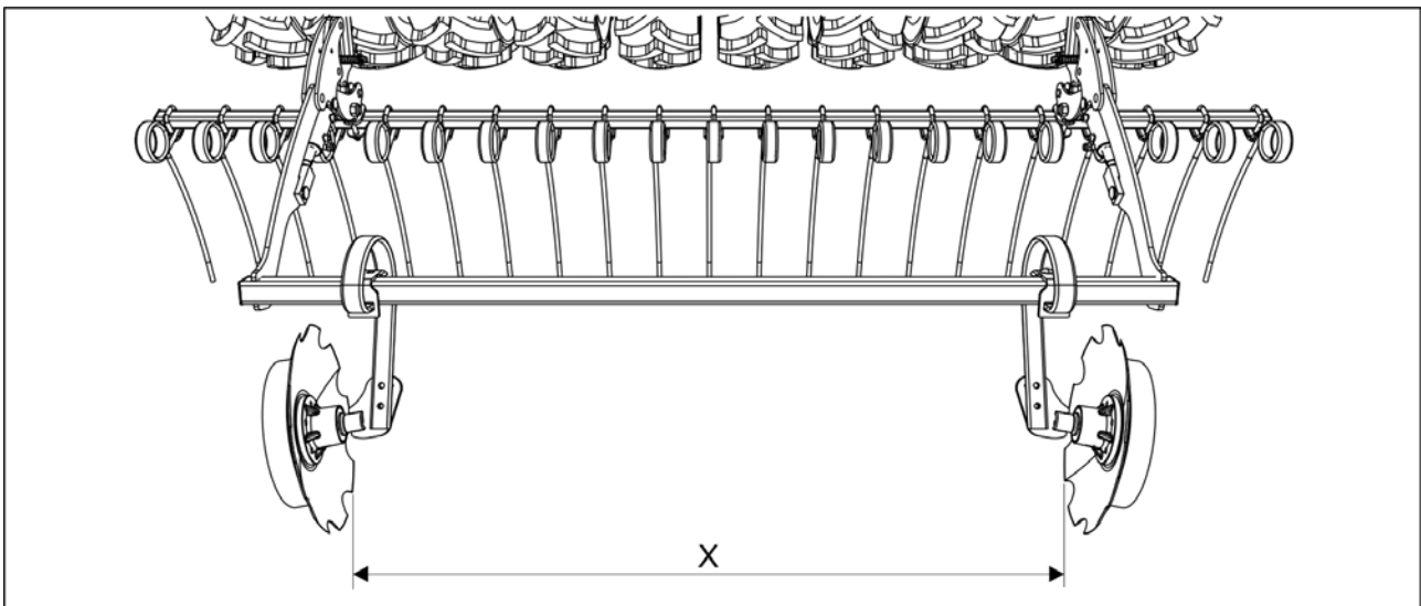
Bild. 5.3.8 - 128. Justering av bredden hos de bakre matarna
