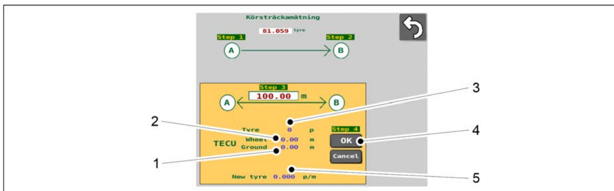
Bild. 7.9.2.1 - 335. Kör kalibrering 3
