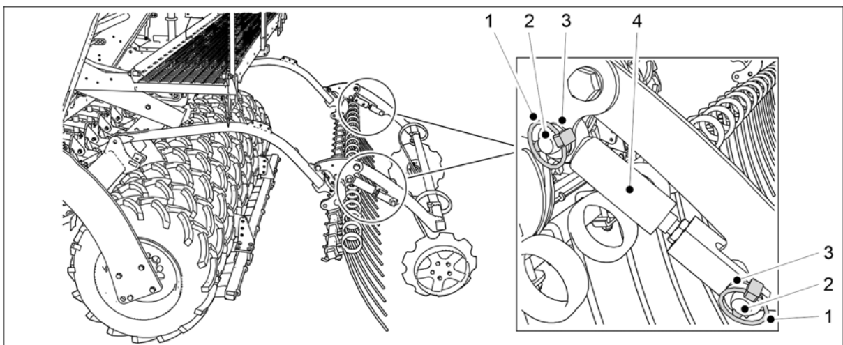
Bild. 7.4.1 - 293. Borttagning av de bakre markör cylindrarna
