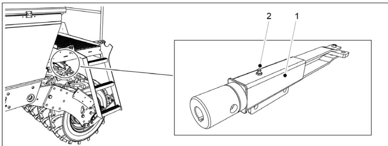
Bild. 7.2.16 - 285. Parkeringsbromsvev
