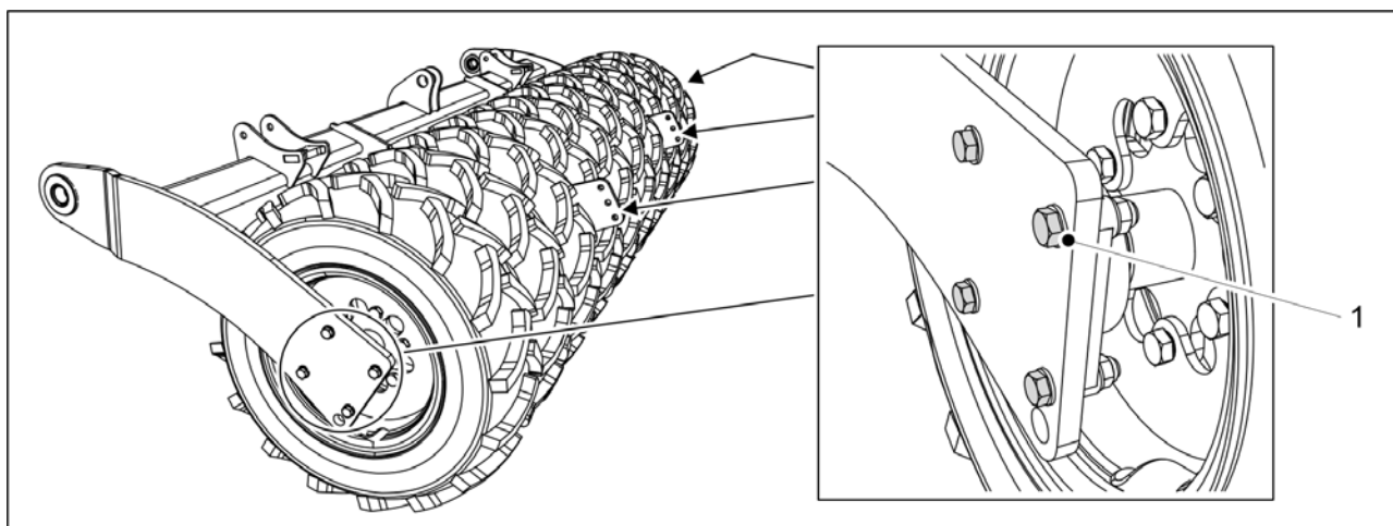
Bild. 7.4.4 - 304. Montering av hjulet
