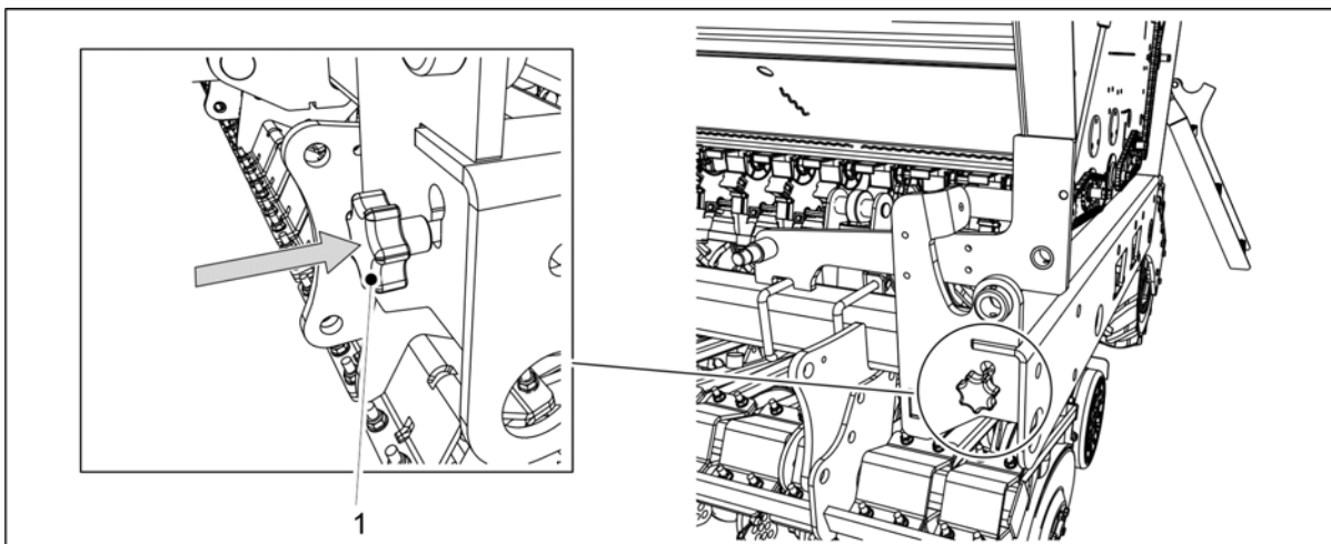
Bild. 6.8.3 - 202. Sätta in kalibreringsprovets justerstång
