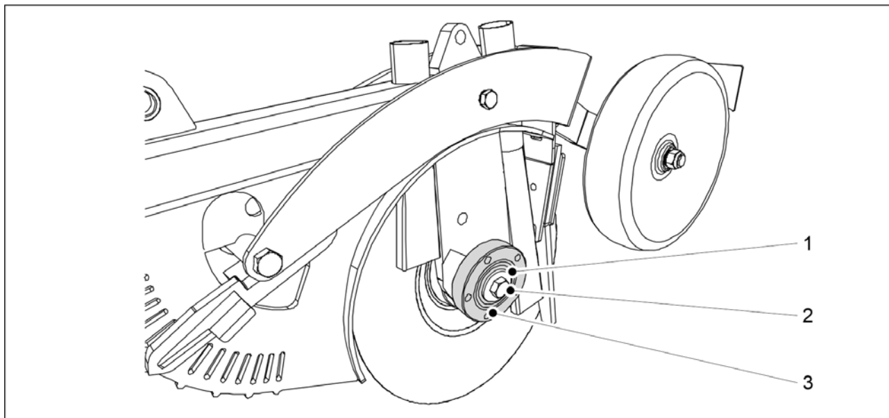
Bild. 7.8.2.2 - 322. Montering av lagerhuset
