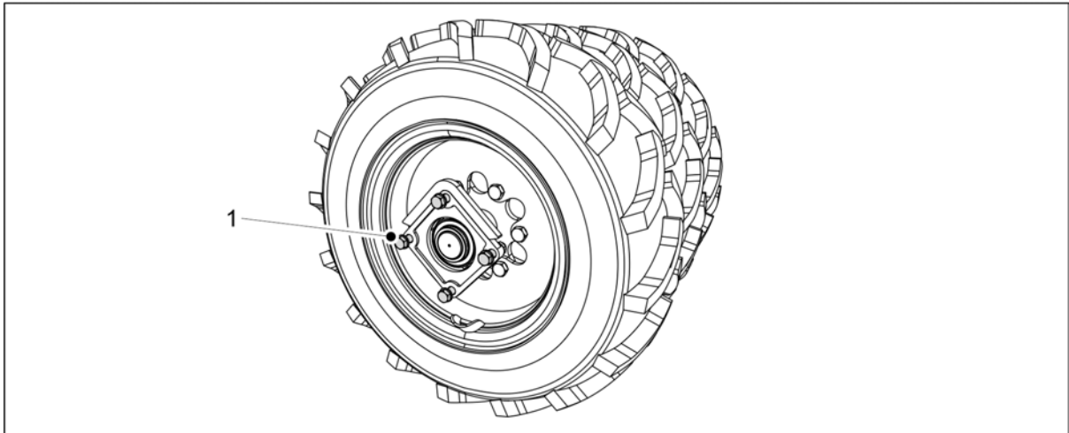
Bild. 7.4.1 - 299. Hjulet stöds av skruvar
