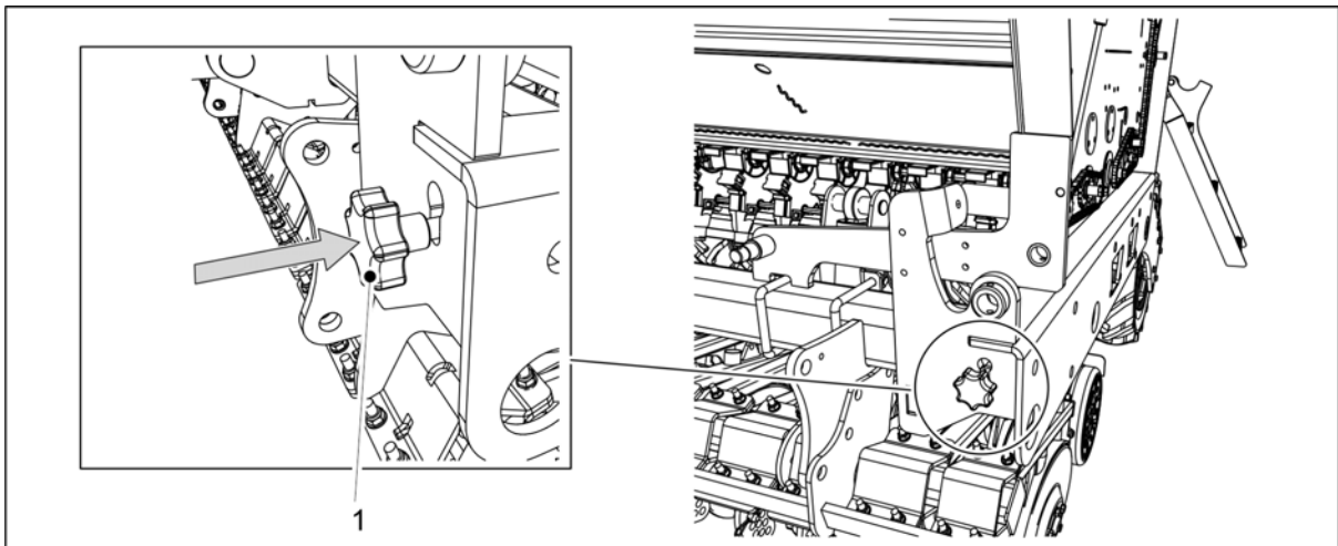
Bild. 6.8.1 - 184. Sätta in kalibreringsprovets justerstång
