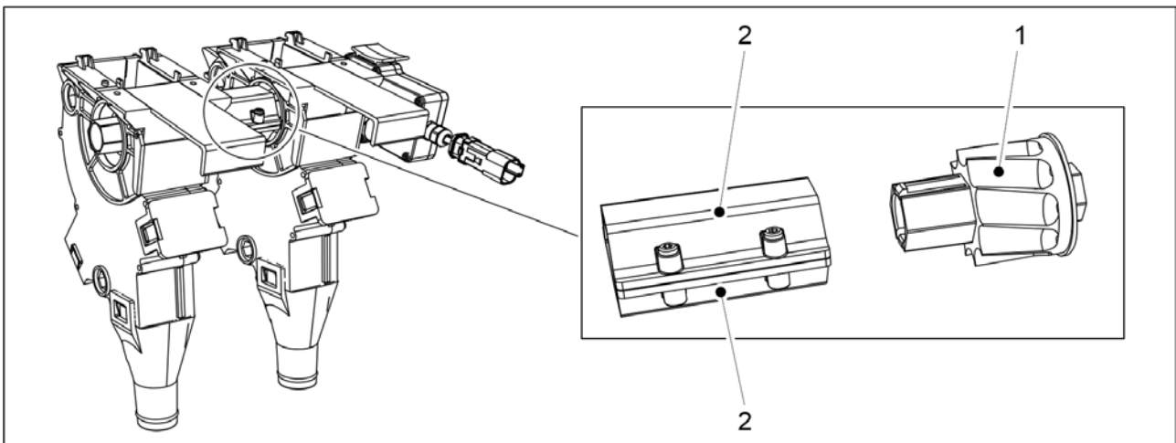
Bild. 4.1.1.8 - 23. Körspårförlängningar
