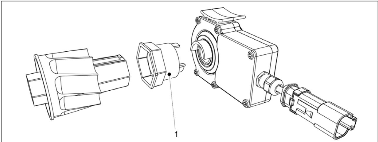
Bild. 4.1.1.7 - 22. Anslutningsbussning
