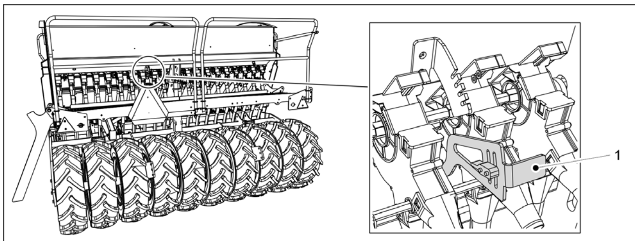
Bild. 7.3.2 - 288. Bottenflik öppen
