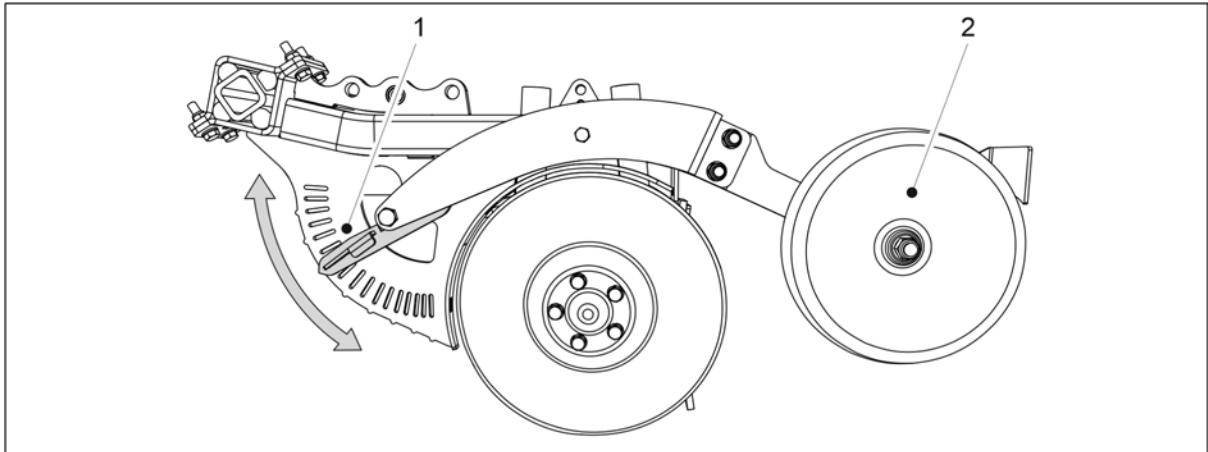
Bild. 6.12 - 223. Justering av såbillens sådjup
