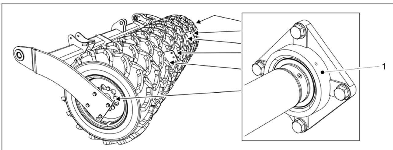
Bild. 7.2.4 - 271. Hjulaxelns kullager
