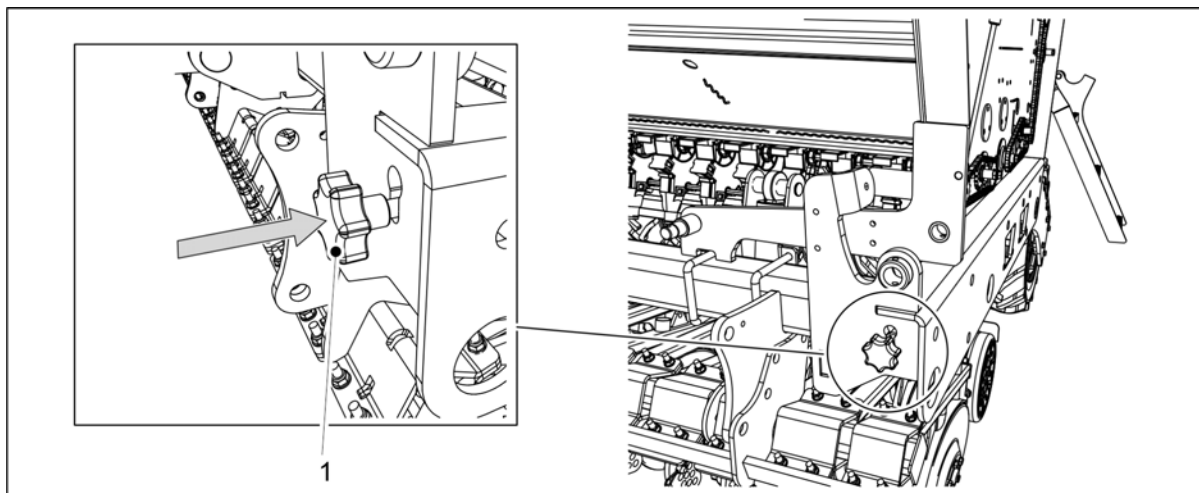
Bild. 6.8.2 - 193. Sätta in kalibreringsprovets justerstång
