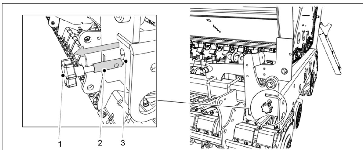
Bild. 6.8.3 - 194. Dra ut kalibreringsprovets justerstång
