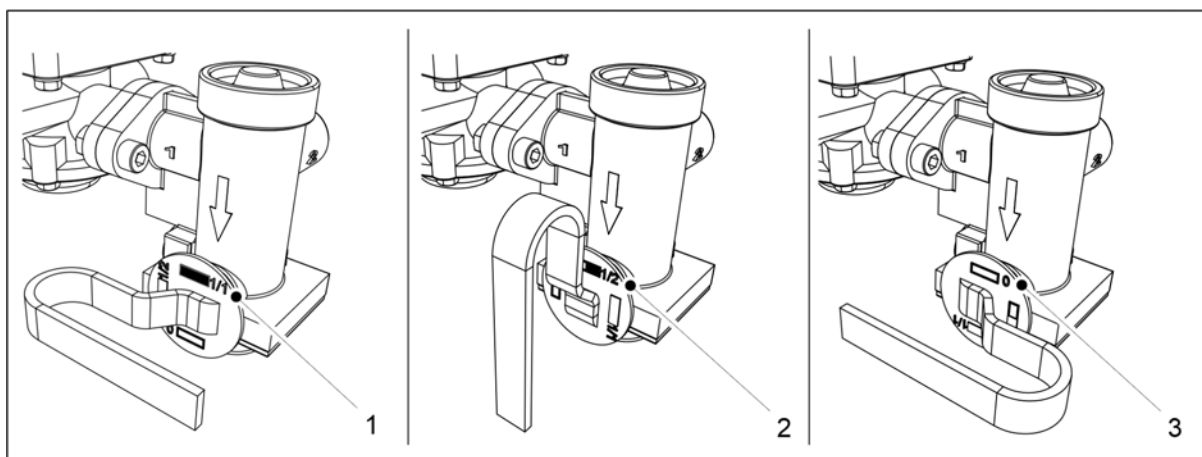
Bild. 6.22.3 - 243. Lägen för bromskraftsregleringsventillen
