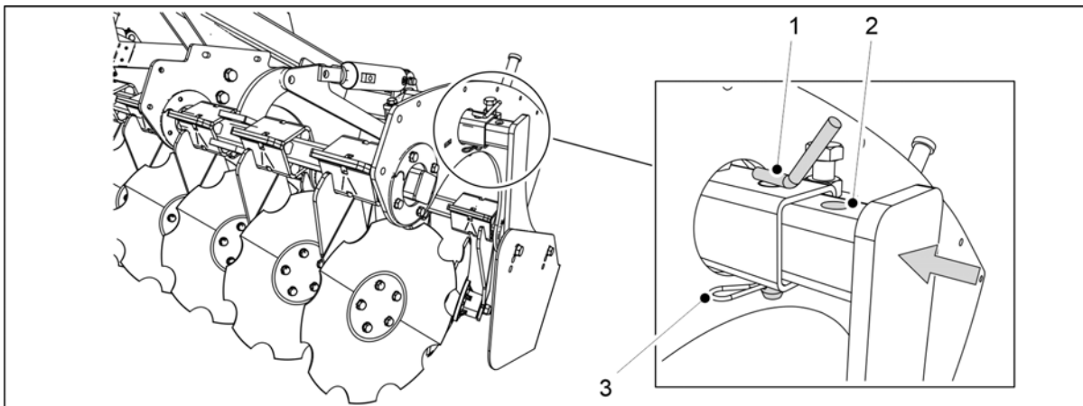
Bild. 6.17 - 234. Justering av den främre tallrikskultivatorns sidobegränsare för transport
