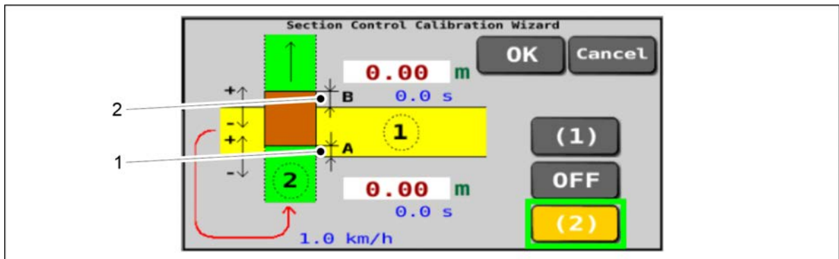
Bild. 6.11.2.1 - 215. Kalibreringssteg 2
