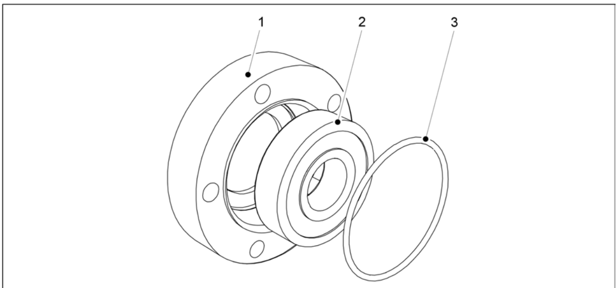
Bild. 7.8.3.1 - 325. Borttagning av lagret och O-ringen
