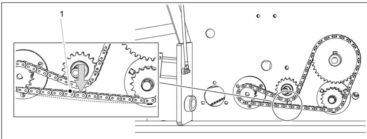
Bild. 7.1.5.3 - 264. Kontrollera kedjespänningen, transmission hos gödningsmedlets spridaraxel
