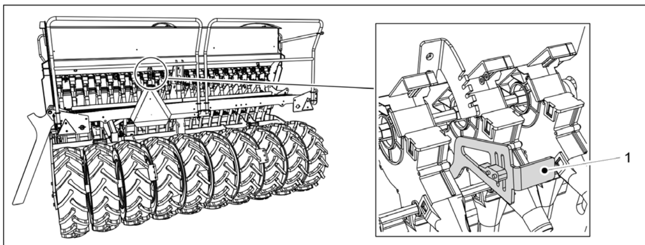
Bild. 6.24.2 - 247. Öppna bottenfliken till småfröbehållaren
