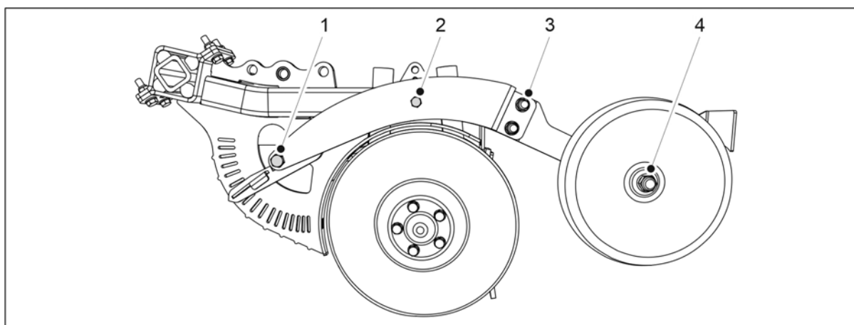
Bild. 7.1.2.4 - 257. Skruvar hos såbillstäckhjulet och djupjustering
