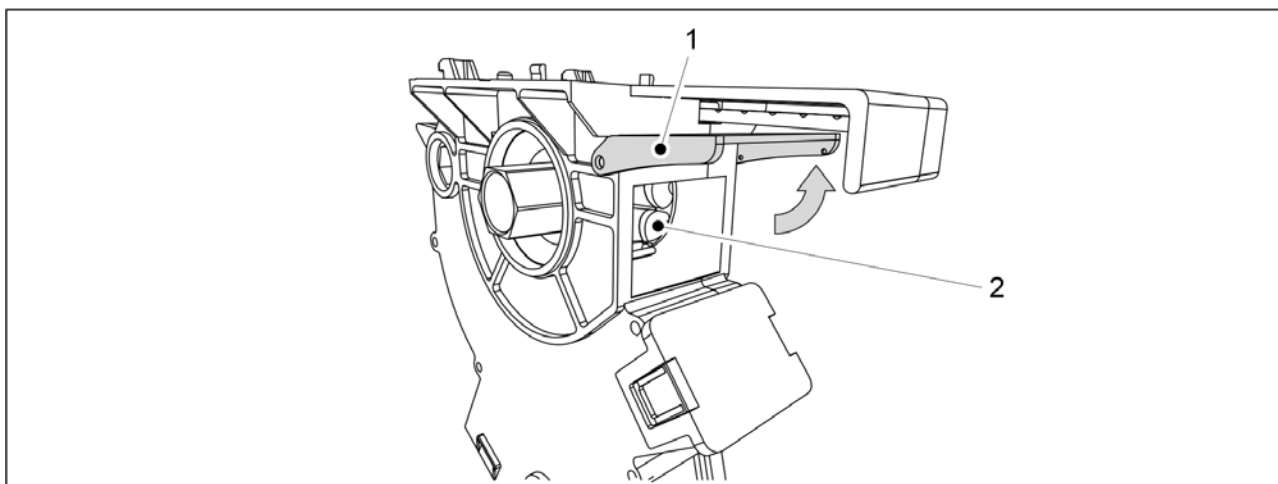
Bild. 7.3.6 - 291. Rengöring av matarenheterna i småfröbehållaren
