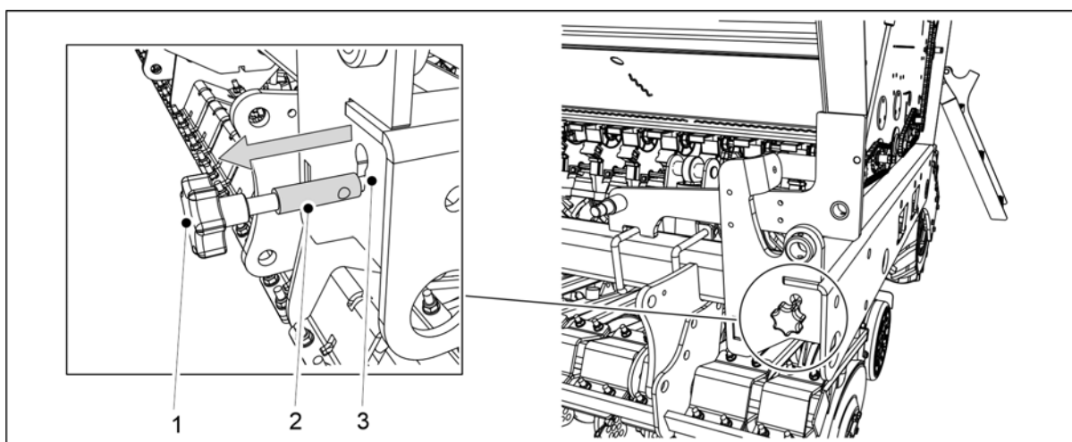
Bild. 6.8.1 - 176. Dra ut kalibreringsprovets justerstång
