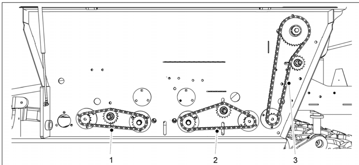
Bild. 7.2.2 - 270. Smörjning av transmissionskedjor
