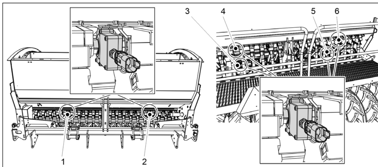
Bild. 4.1.1.7 - 21. Position hos körspårkopplingar
