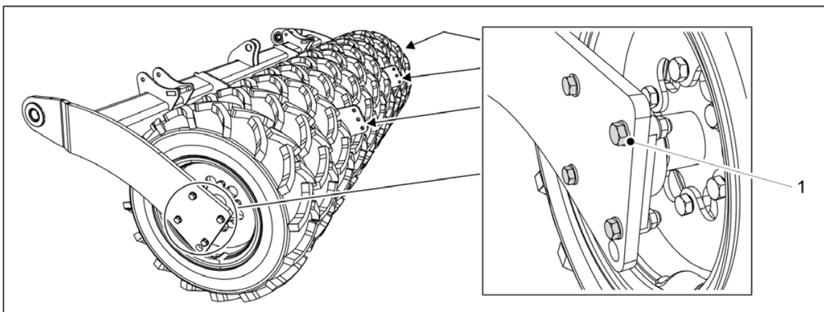
Bild. 7.4.1 - 297. Demontering av hjulet
