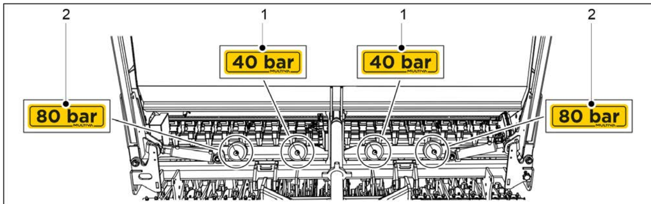
Bild. 3.3 - 9. Tryckackumulatoretiketter
