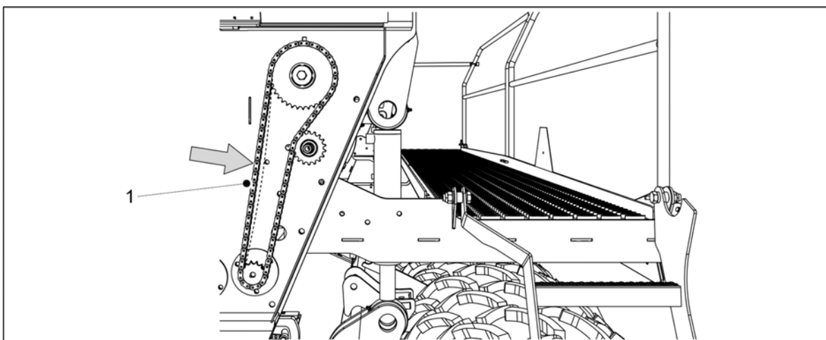
Bild. 7.1.5.2 - 263. Kontroll av kedjespänning, överföring av småfrön
