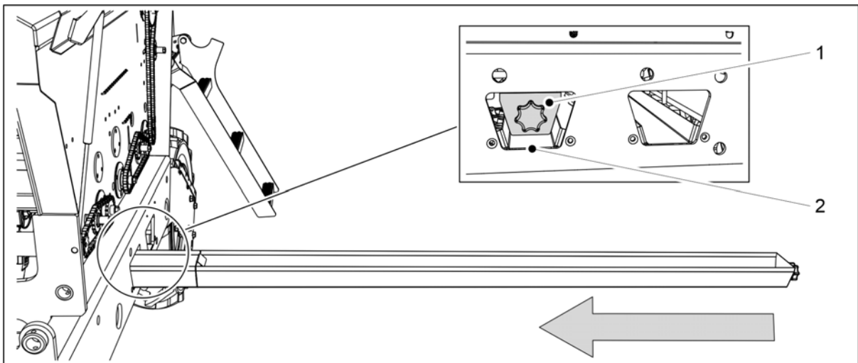
Bild. 6.8.1 - 177. Montera kalibreringsbrickorna
