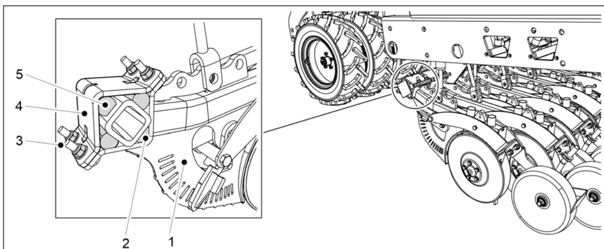
Bild. 7.8.1.2 - 317. Fästa såbillen
