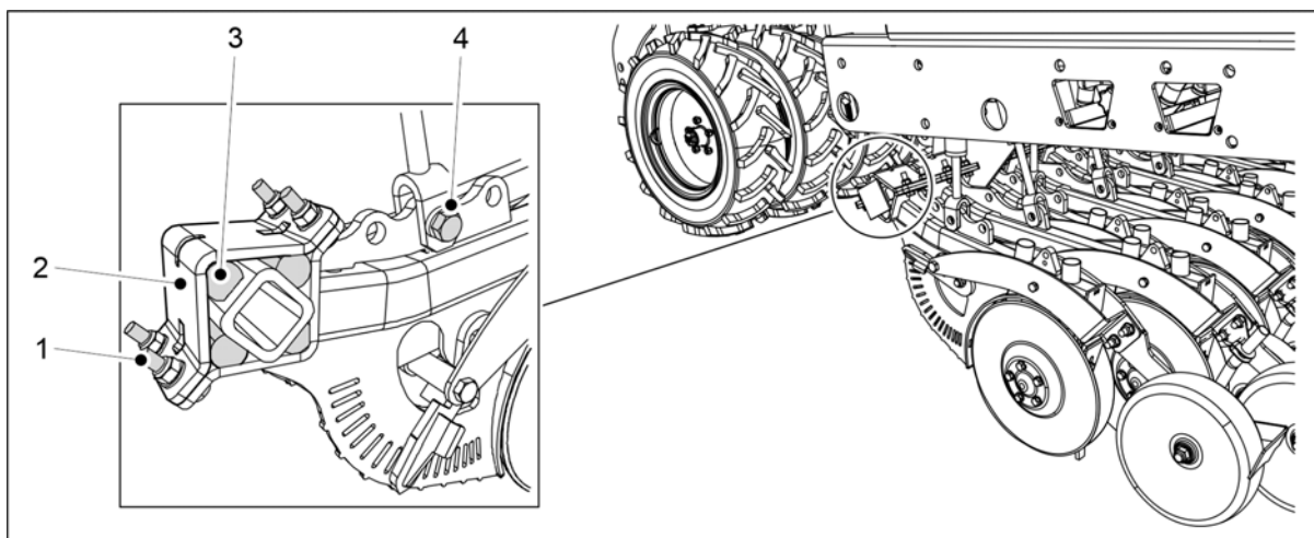
Bild. 7.8.1.1 - 316. Demontering av en såbill
