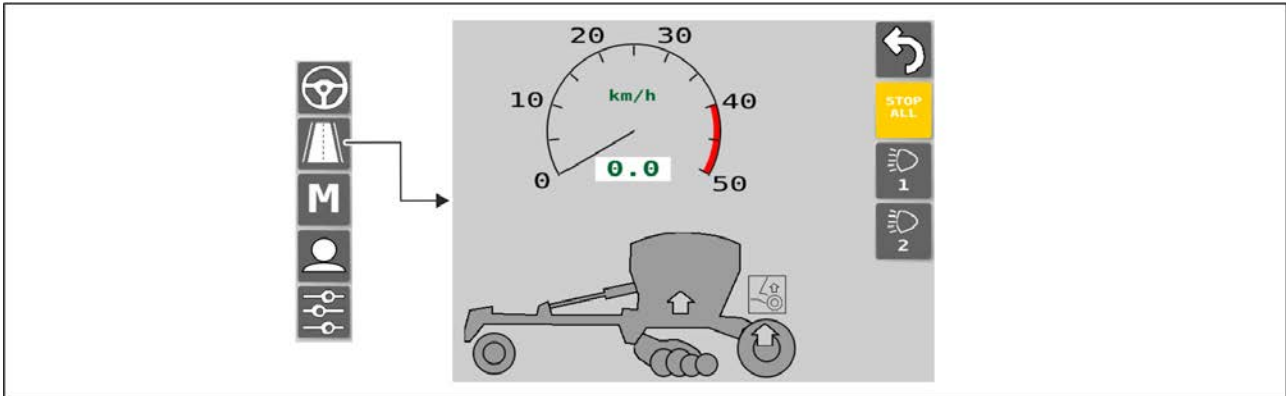
Bild. 4.1.2 - 33. Transportdrift
