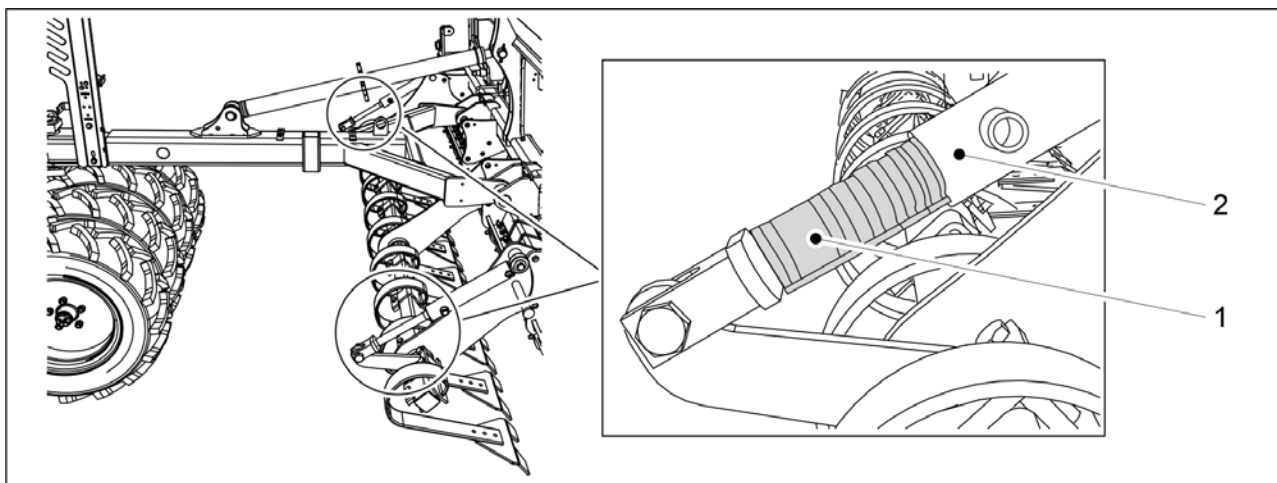
Bild. 6.15 - 228. Justering av den främre utjämningsharven
