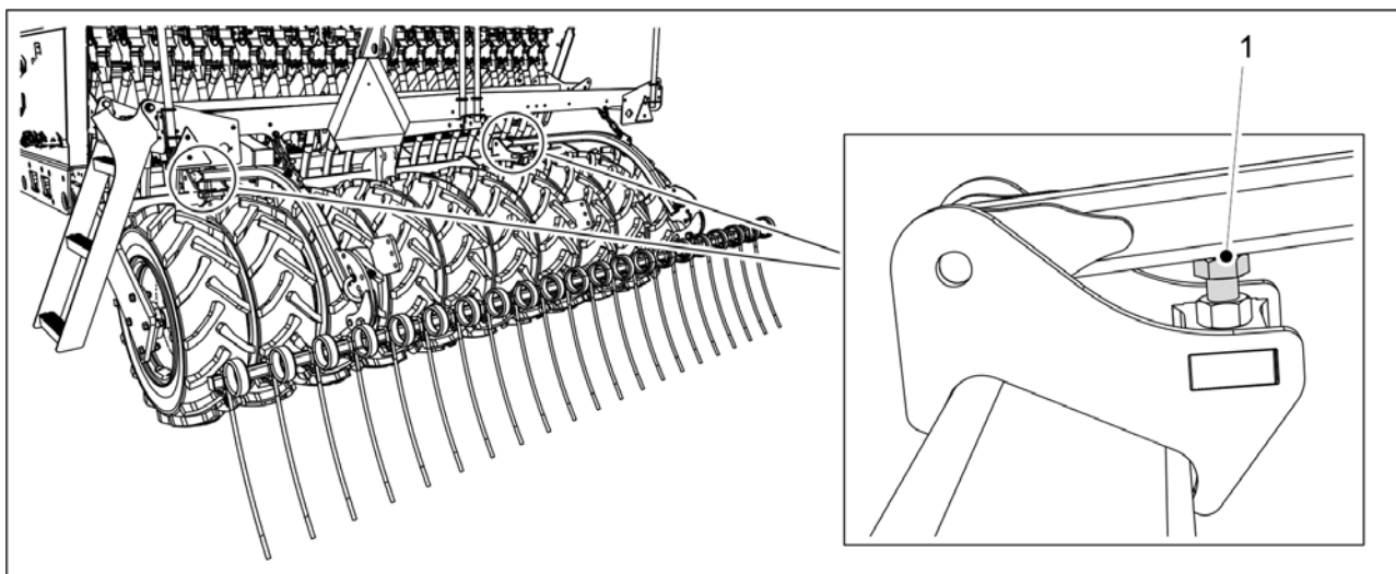
Bild. 6.14 - 226. Justering av efterharvens höjd
