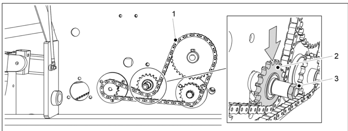
Bild. 7.5.3 - 308. Spänna kedjan på gödningsmedlets spridaraxel
