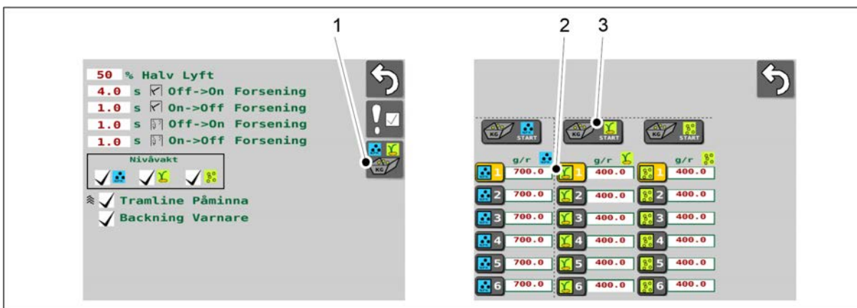
Bild. 6.8.2 - 187. Starta kalibreringsprovet
