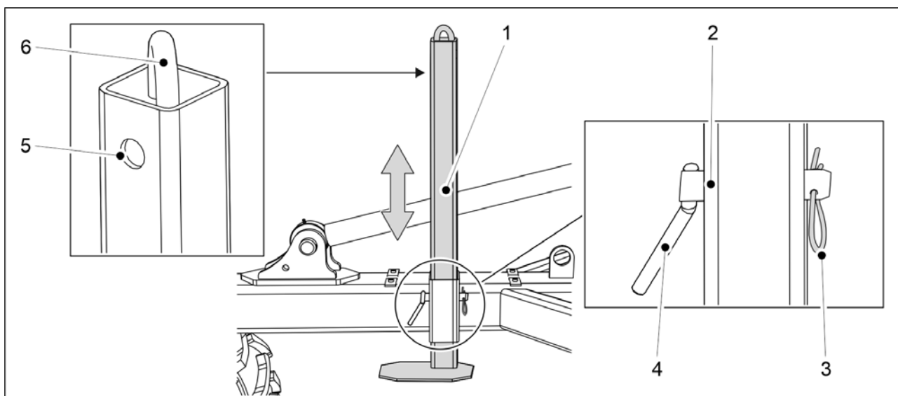
Bild. 5.3.2 - 118. Markutrustning
