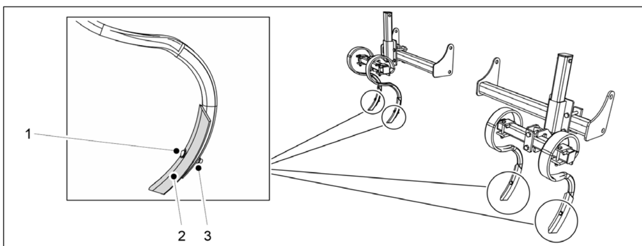
Bild. 6.18.2 - 236. Byta ut en S-pinnspets
