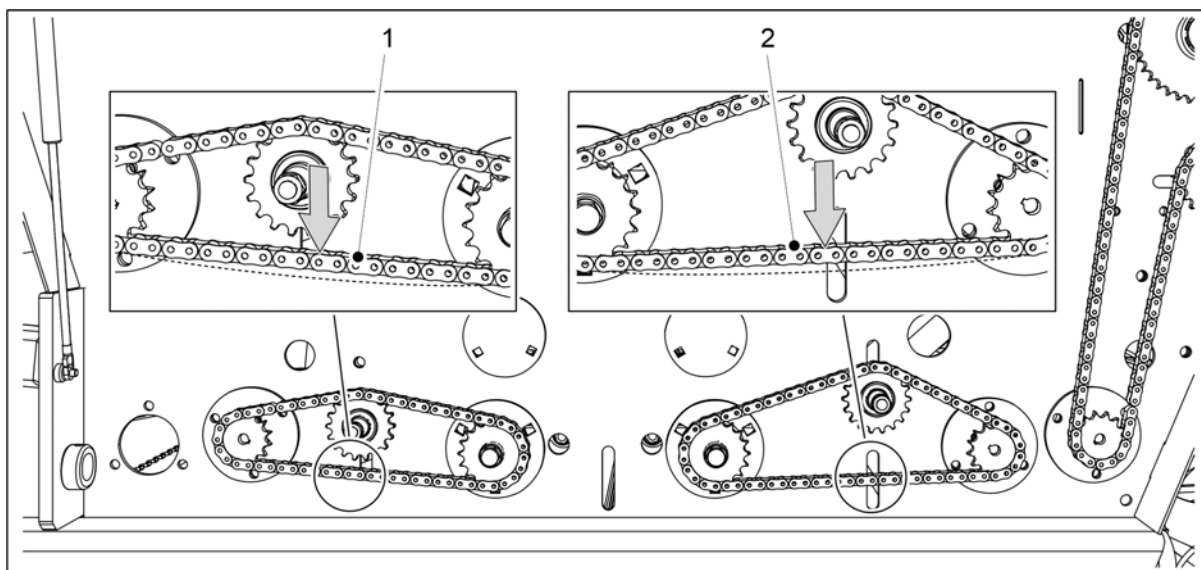
Bild. 7.1.5.1 - 262. Kontroll av kedjespänning, överföring av gödningsmedel och utsäde
