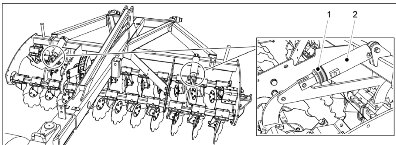
Bild. 6.17 - 231. Justering av den främre tallrikskultivatorns jordbearbetningsdjup
