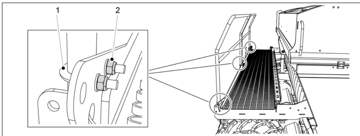
Bild. 7.1.2.5 - 259. Arbetsplattformens U-skrivar
