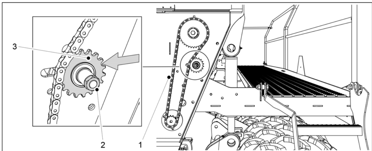
Bild. 7.5.2 - 307. Dra åt kedjan hos småfröbehållaren
