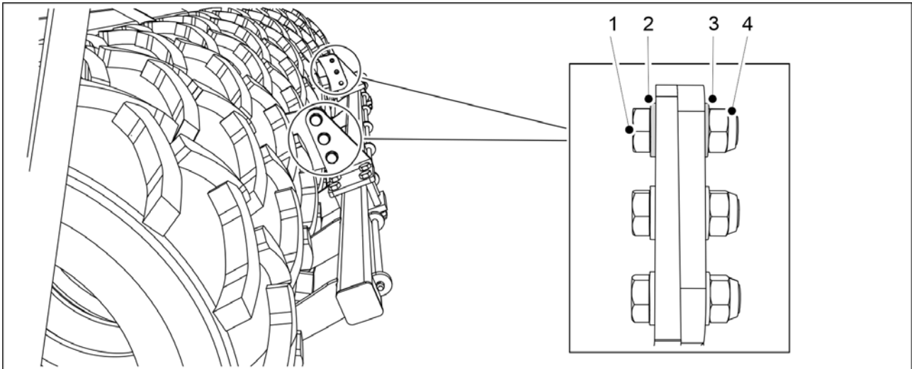
Bild. 7.4.1 - 292. Demontering av skrapan
