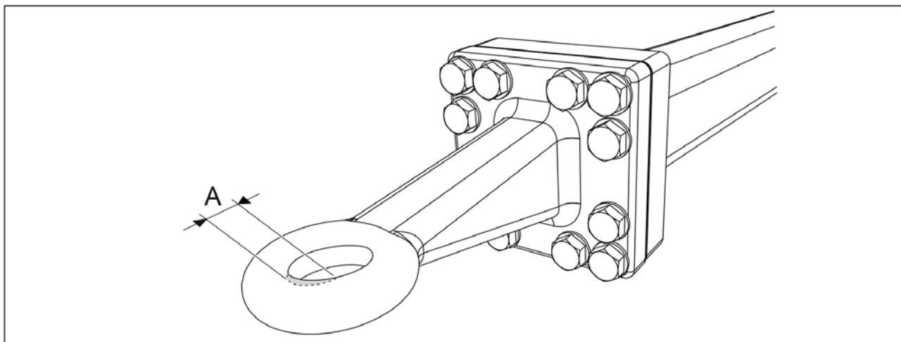
Bild. 7.1.8 - 266. Slitage på dragöglan
