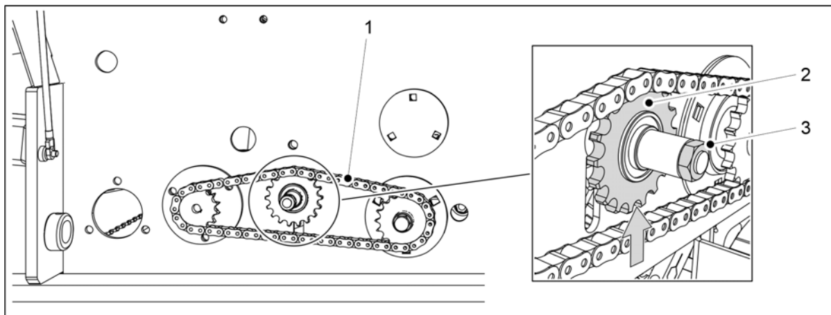
Bild. 7.5.1 - 305. Spänning av gödningsmedelsbehållarens kedja
