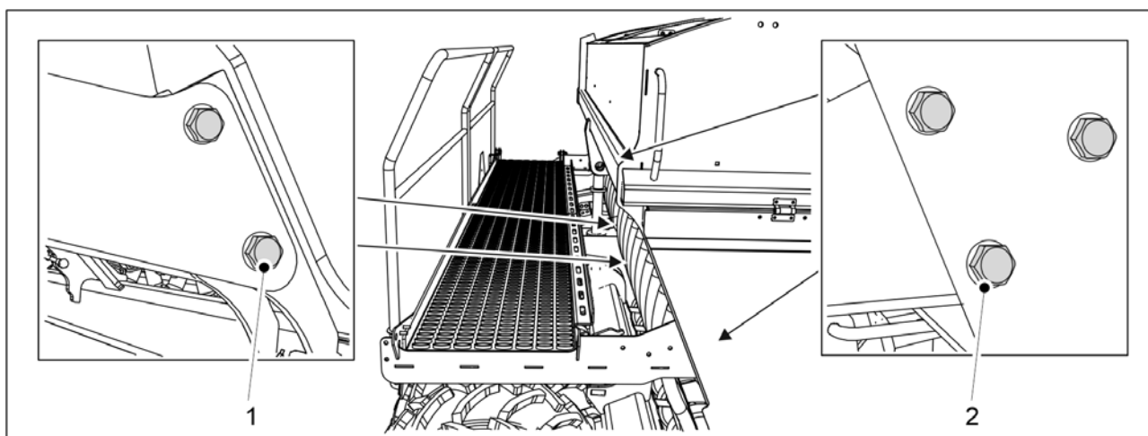
Bild. 7.1.2.5 - 258. Arbetsplattformens skruvar
