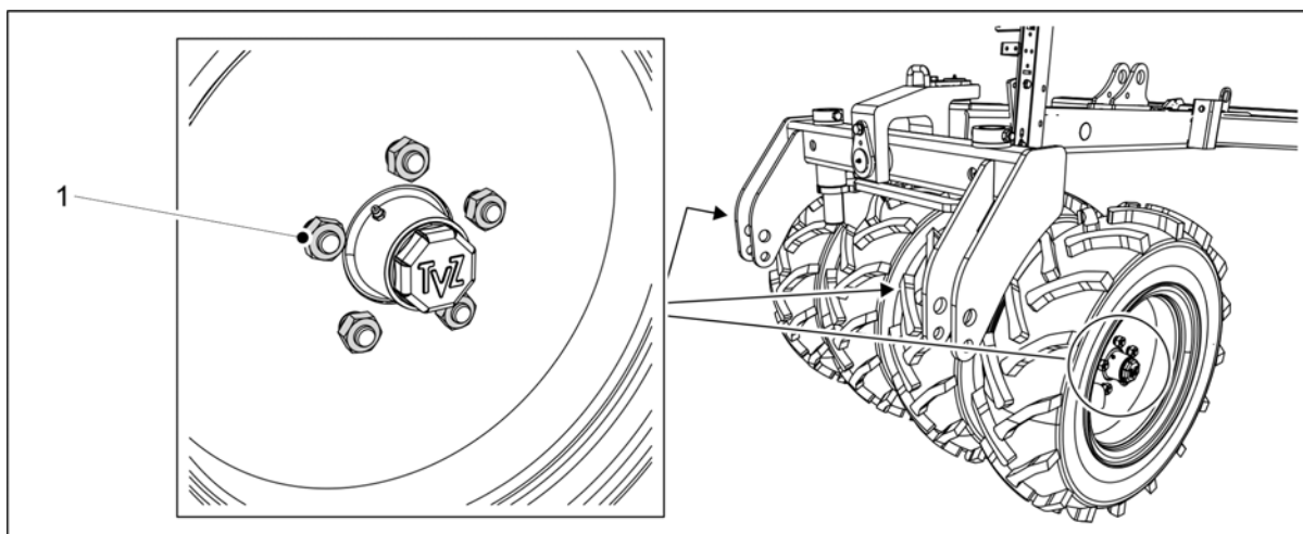
Bild. 7.1.2.3 - 255. Hjulpackarens skruvar
