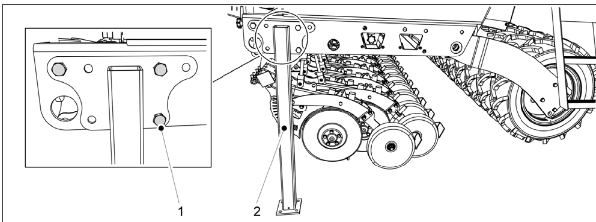
Bild. 7.4.1 - 296. Transportstöd
