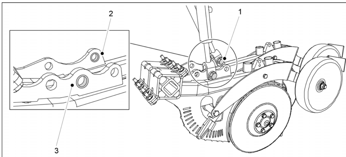
Bild. 7.8.1.2 - 318. Montering av cylinder till såbill
