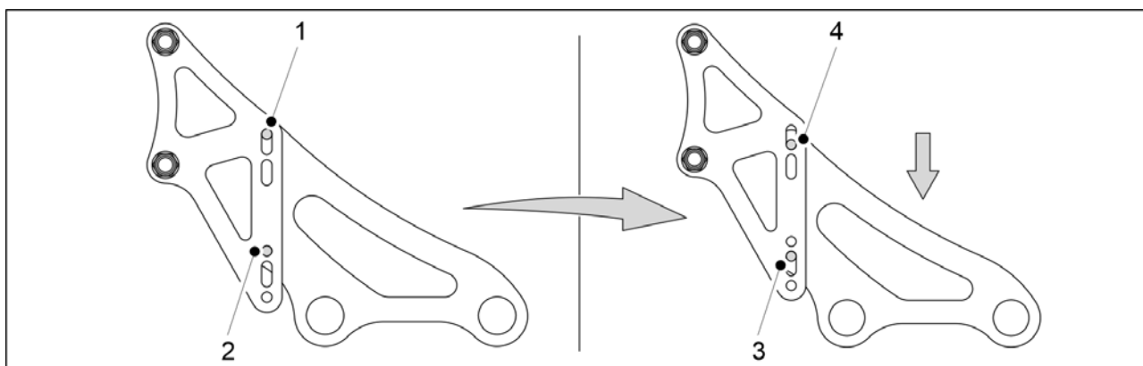
Bild. 6.16 - 230. Justering av främre harvens höjd
