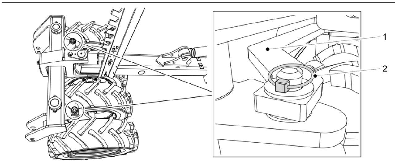
Bild. 7.1.2.3 - 254. Hjulpackarens stång
