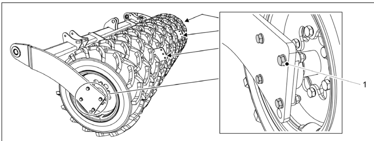
Bild. 7.1.2.2 - 253. Skruvarna i transporthjulens flänslager
