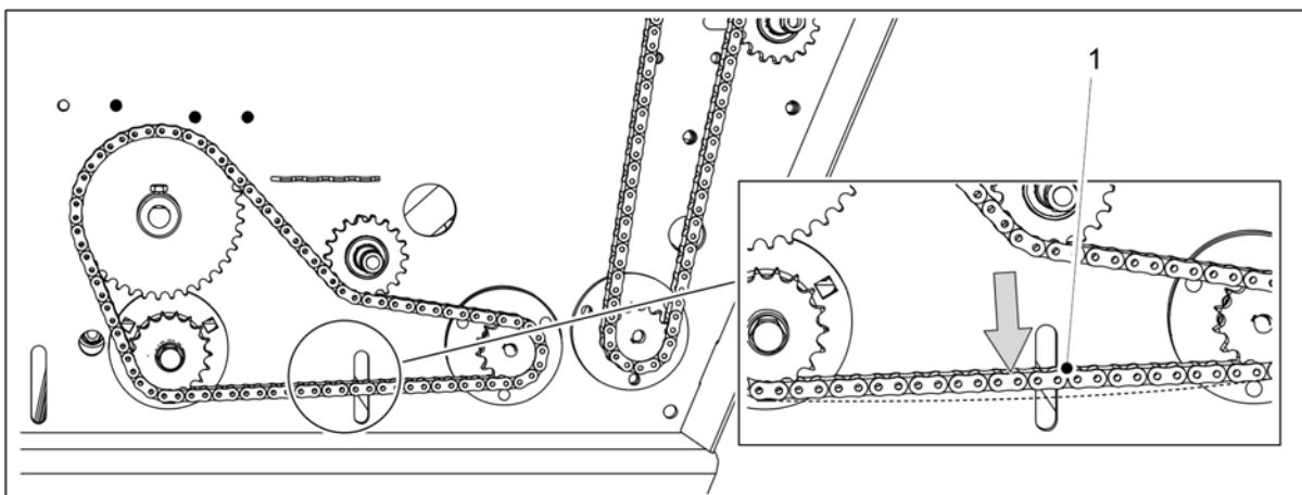
Bild. 7.1.5.4 - 265. Kontroll av kedjespänning, transmission hos utsädens spridaraxel
