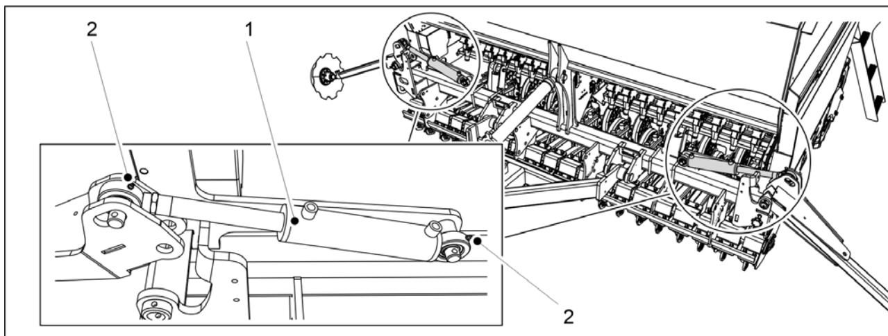
Bild. 7.2.7 - 274. Cylindrar hos de mellersta markörerna.
