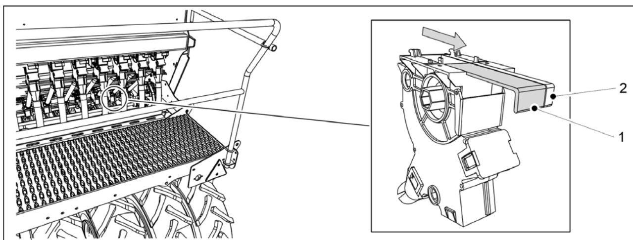
Bild. 6.6.7.2 - 168. Avstängningsplattor på utsädesmataren
