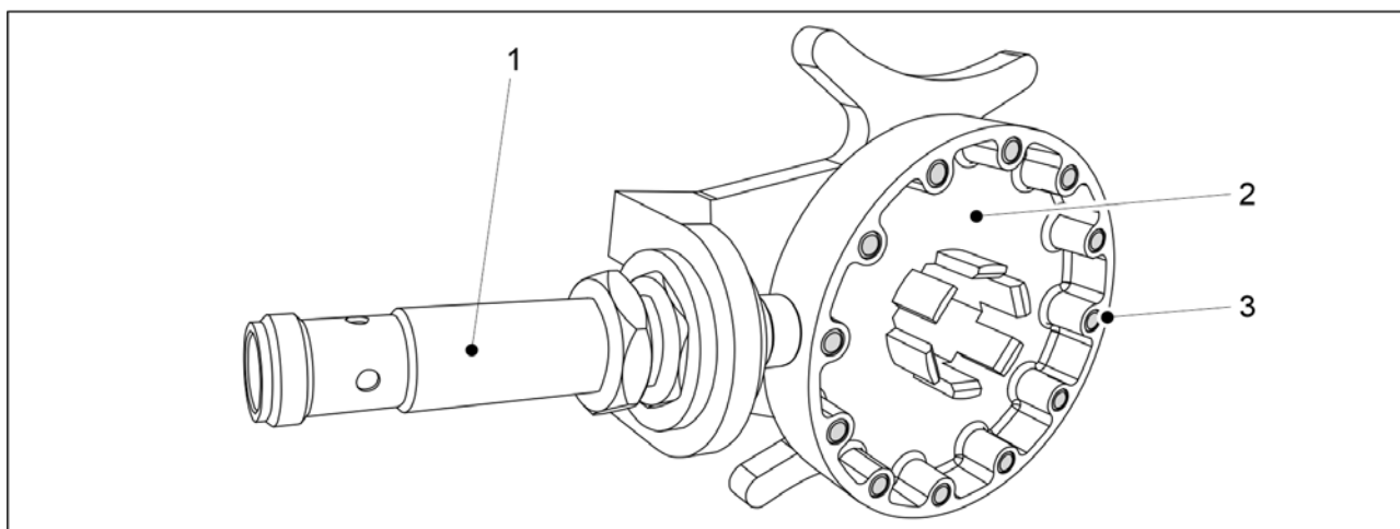
Bild. 4.1.1.5 - 19. Drivaxelns rotationsvakt
