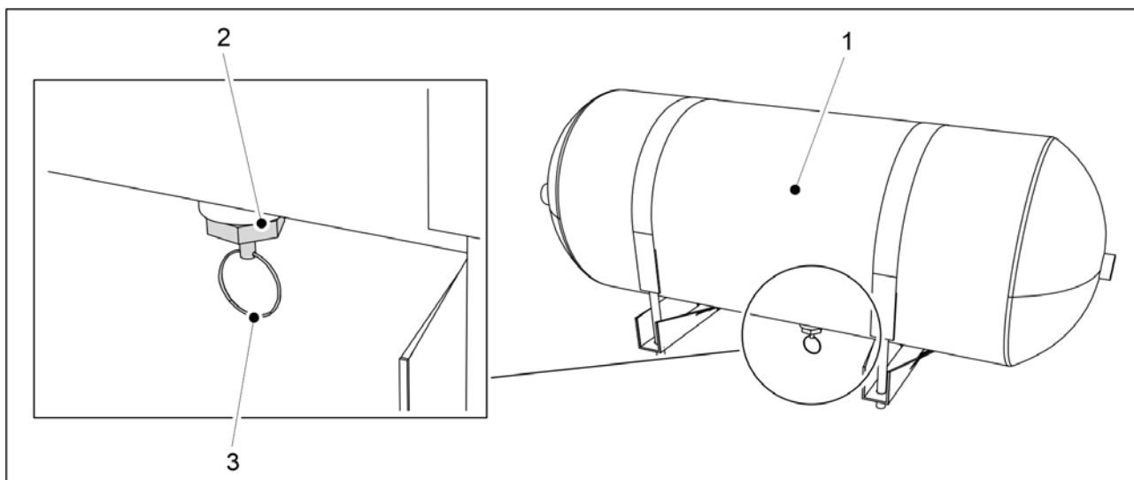
Bild. 7.1.10.2 - 268. Tömning av vatten från den pneumatiska tanken
