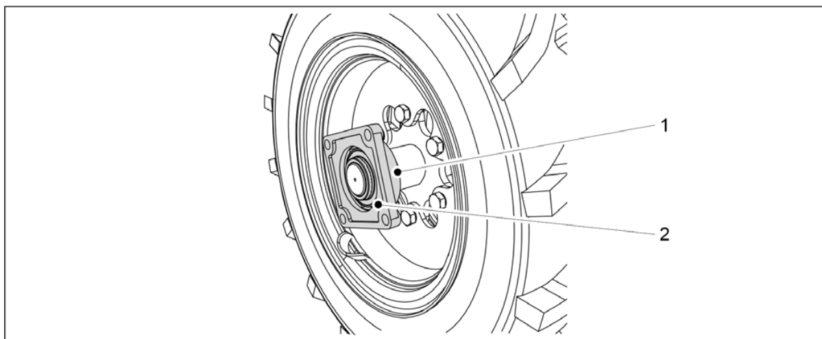
Bild. 7.4.3 - 303. Fästa lagret
