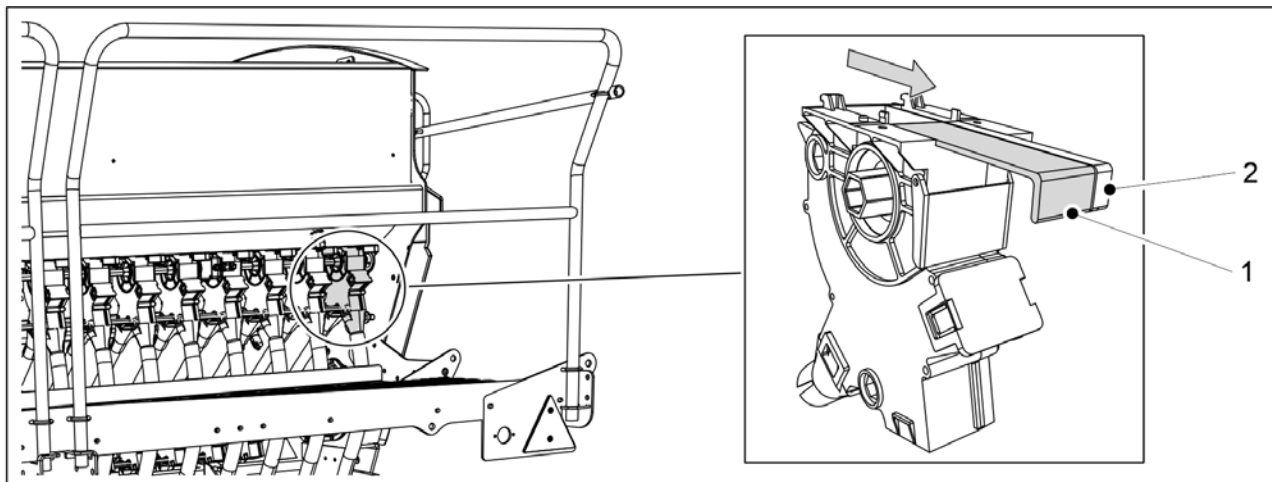
Bild. 6.6.8.2 - 171. Avstängningsplattor på småfrömataren
