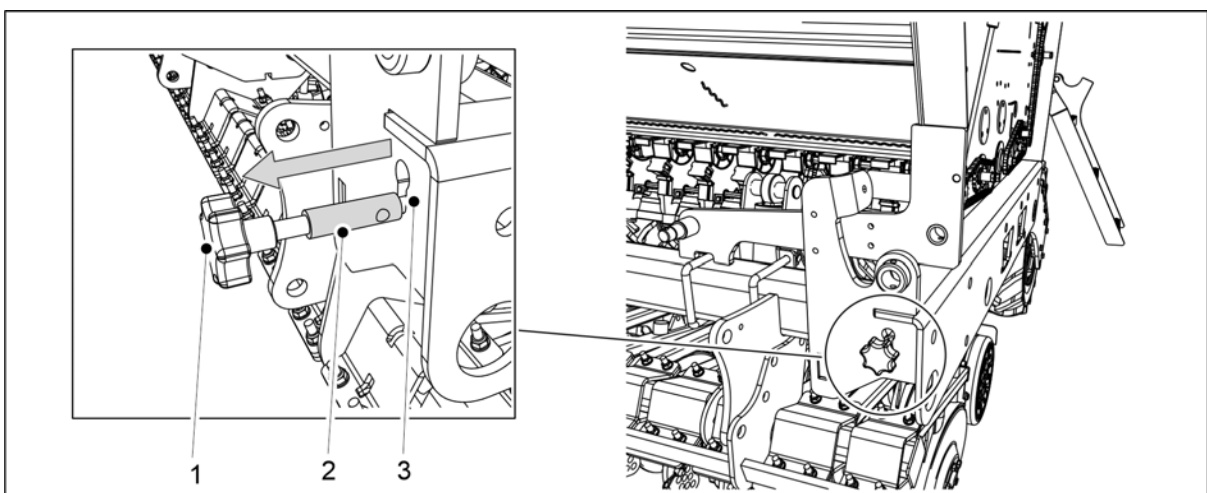
Bild. 6.8.2 - 185. Dra ut kalibreringsprovets justerstång
