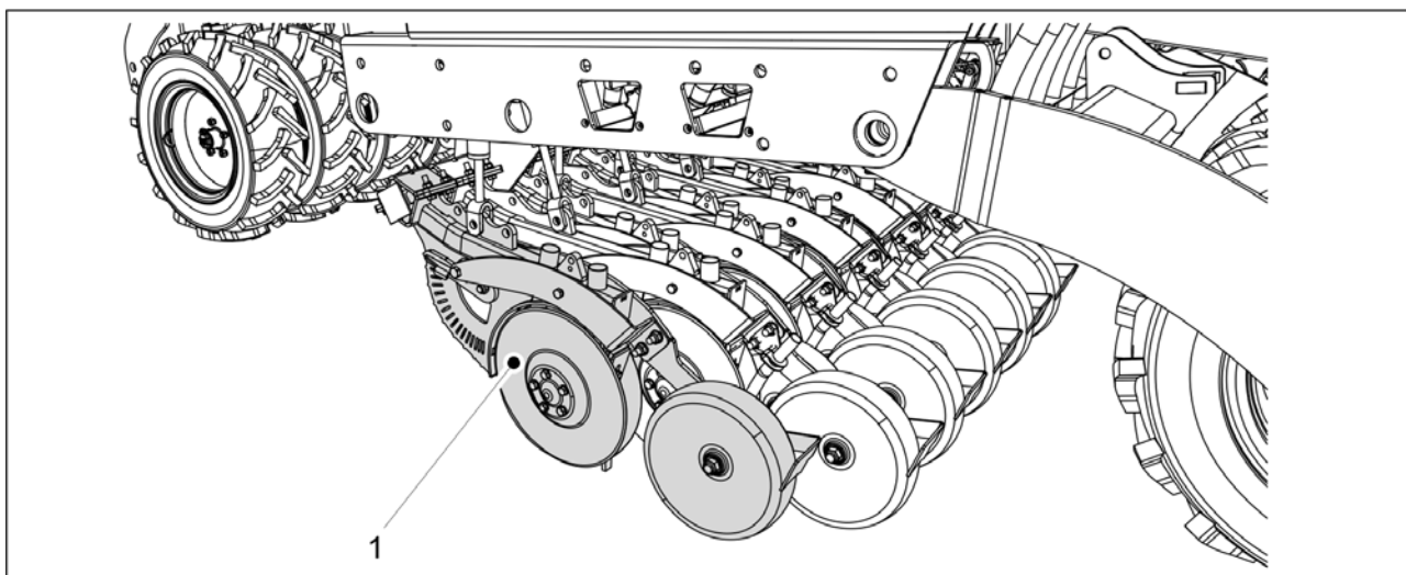
Bild. 7.8.1.1 - 314. Sänka såbillen till marken
