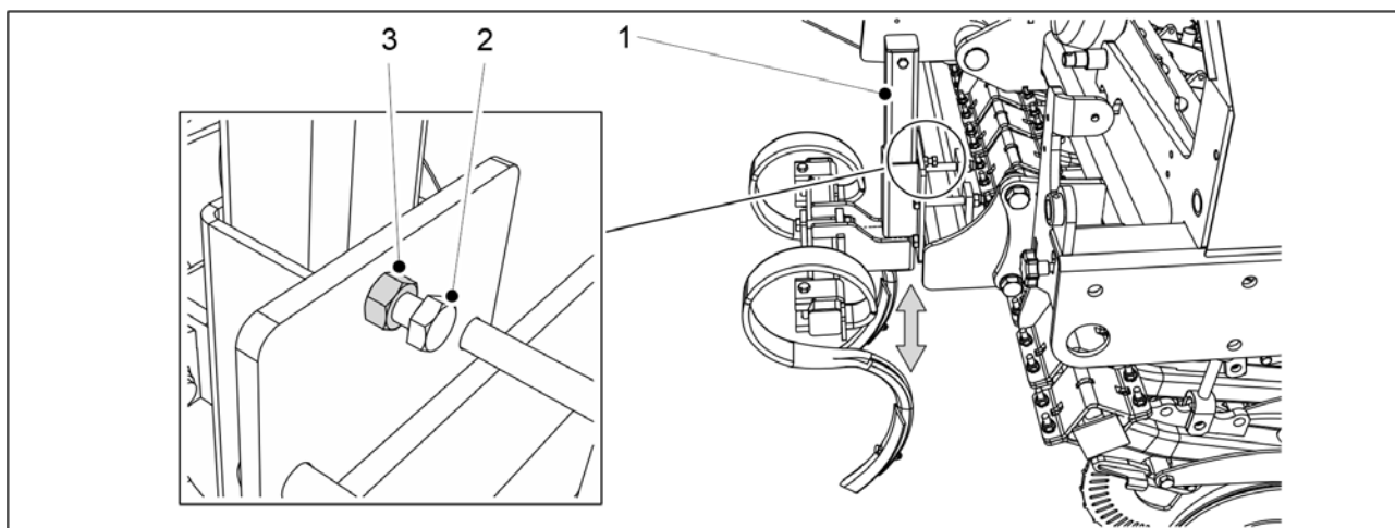
Bild. 6.18.1 - 235. Justering av spårborttagarens höjd
