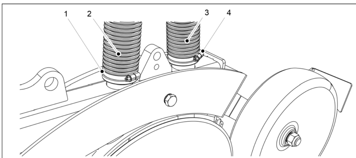
Bild. 7.8.1.2 - 319. Anslutning av såbillsslanger
