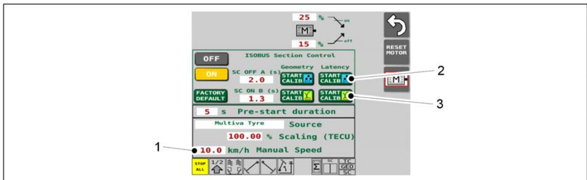
Bild. 6.11.2.2 - 217. Startar fördröjningskalibreringen
