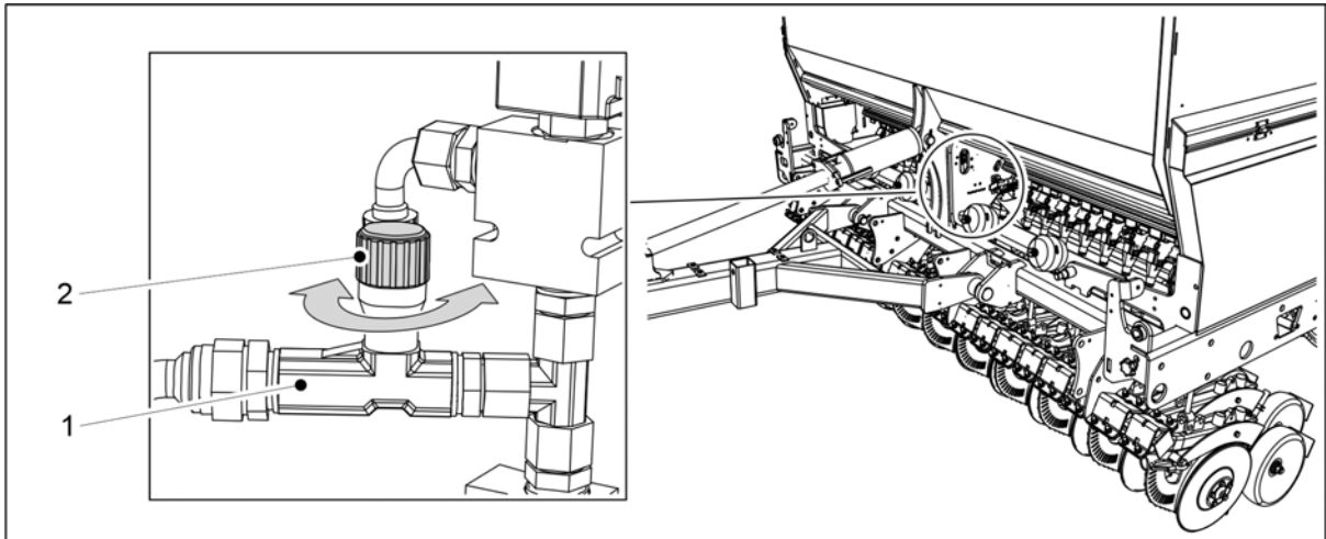
Bild. 5.3.7 - 127. Justera mittmarkörernas lyfthastighet
