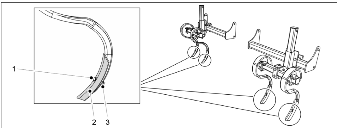
Billede. 6.18.2 - 236. Bytte en S-tindespiss
