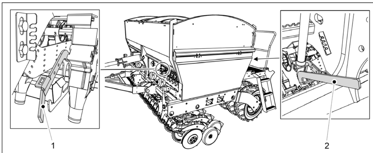
Billede. 7.3.1 - 286. Bunnklaffer åpne
