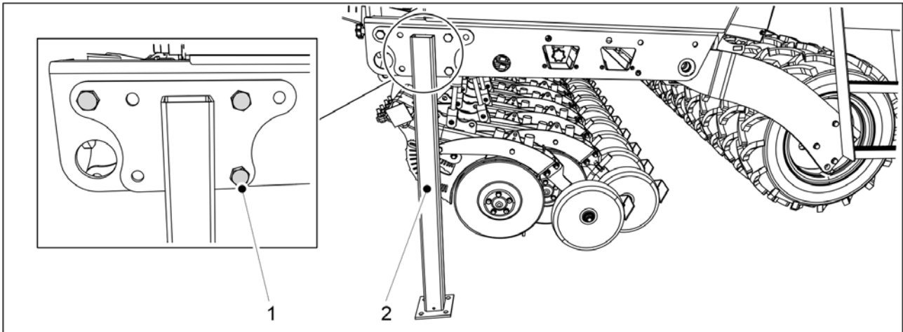
Billede. 5.1.9 - 74. Transportstøtte
