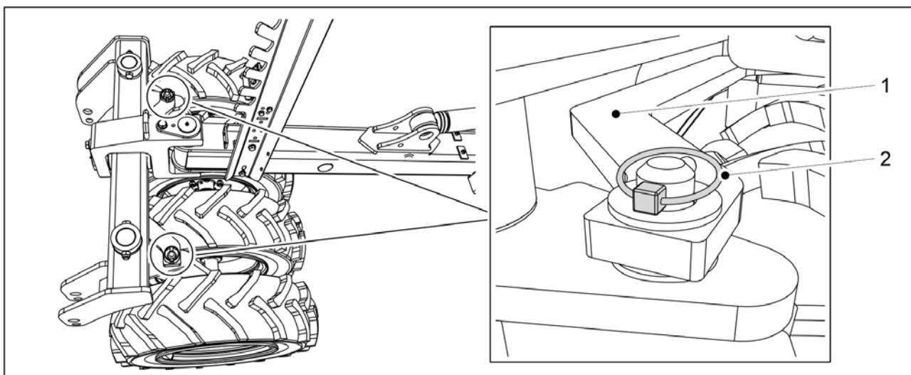
Billede. 7.1.2.3 - 254. Hjulpakkerstang
