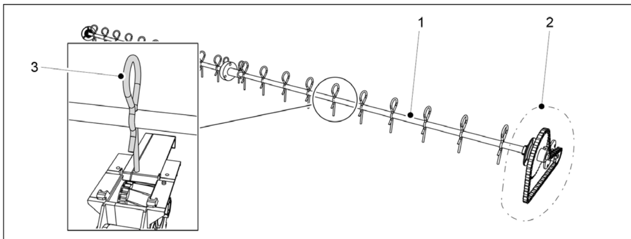
Billede. 6.19.2 - 238. Frøspredningsaksel
