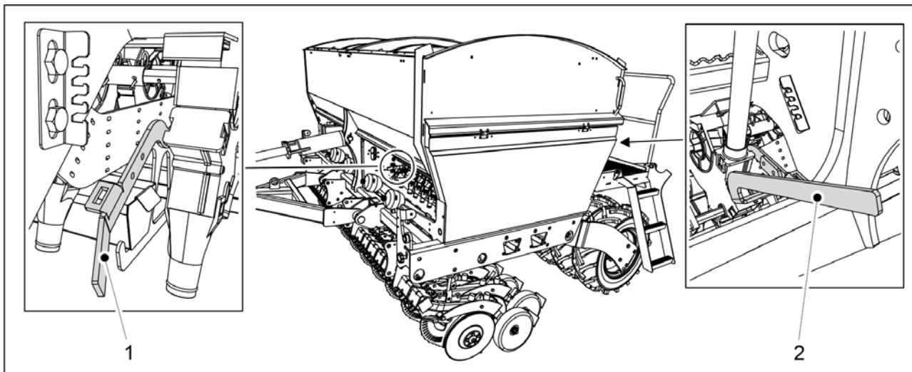
Billede. 6.23.2 - 244. Åpne traktens bunnsklaff
