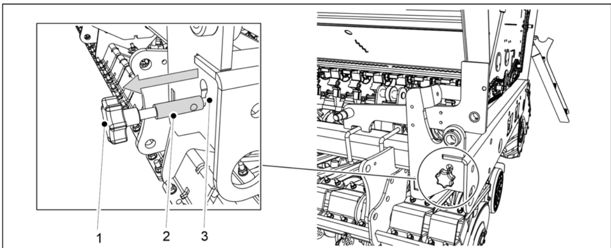
Billede. 6.8.1 - 176. Trekke ut kalibreringstestens justeringsstang
