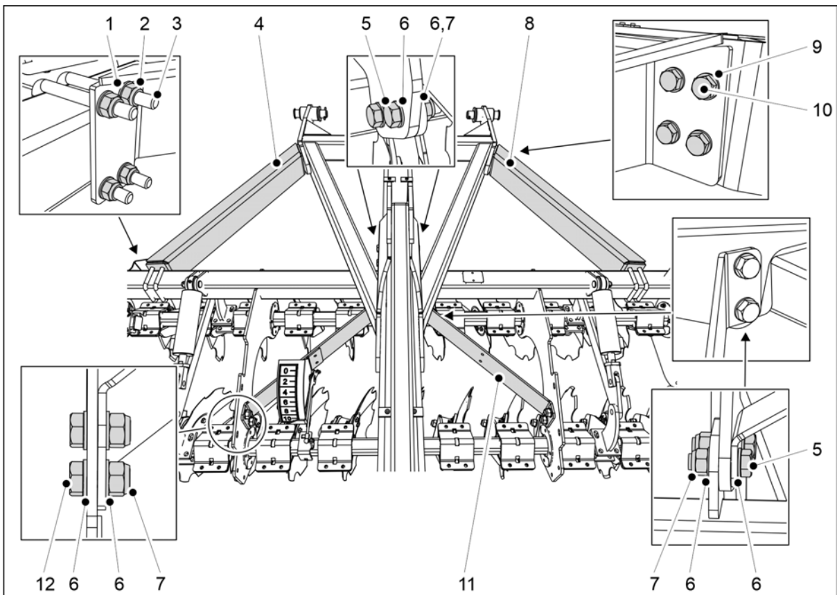
Billede. 5.1.6 - 67. Feste den fremre skivekultivatoren til trekkstangen
