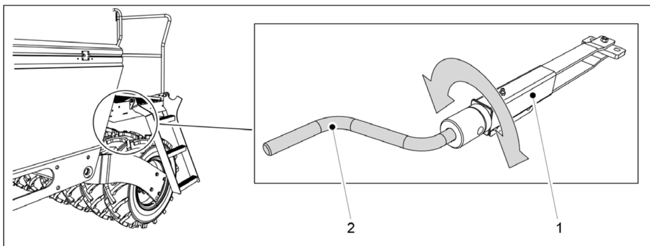
Billede. 6.22.1 - 240. Parkeringsbrems
