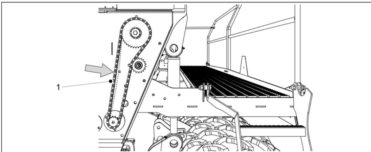
Billede. 7.1.5.2 - 263. Kontrollere kjedespenning, kraftoverføring for småfrø
