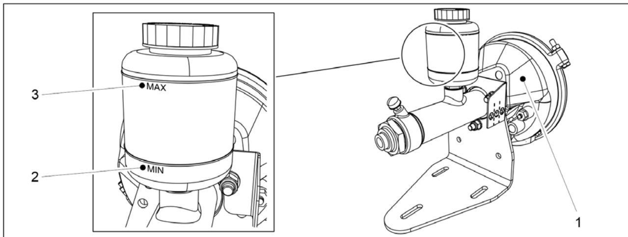
Billede. 7.1.10.3 - 269. Kontrollerer oljenivået i trykkluft-hydraulikk-omformeren
