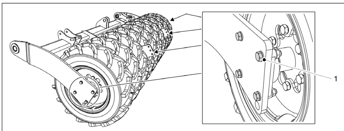
Billede. 7.4.1 - 297. Demontere hjulmontasjen
