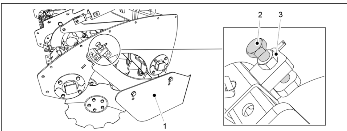
Billede. 6.17 - 232. Justere den nedre posisjonen til sidesperrene
