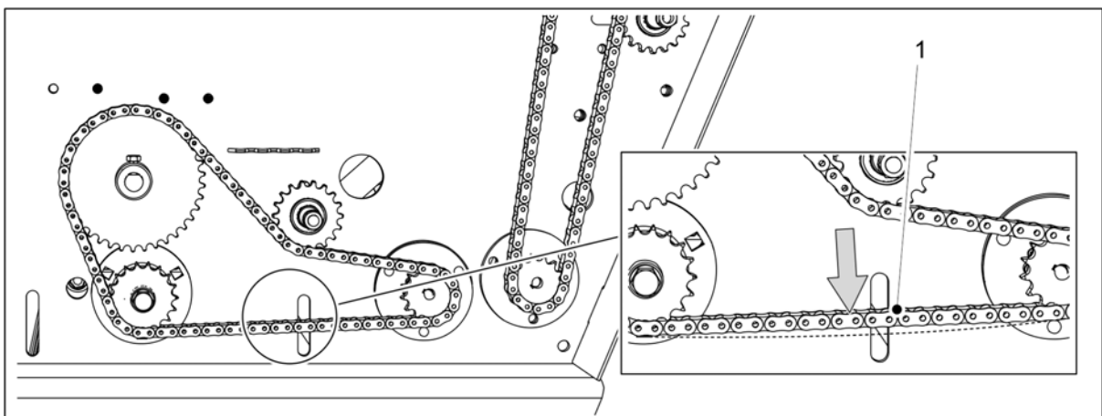
Billede. 7.1.5.4 - 265. Kontrollere kjedespennning, kraftoverføring for frøspredningsaksel
