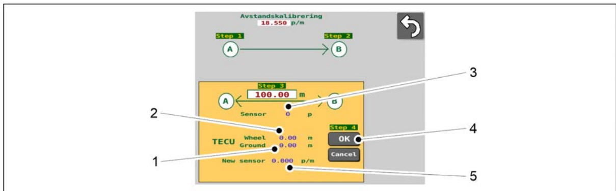
Billede. 7.9.2.1 - 335. Kjørekalibrering 3
