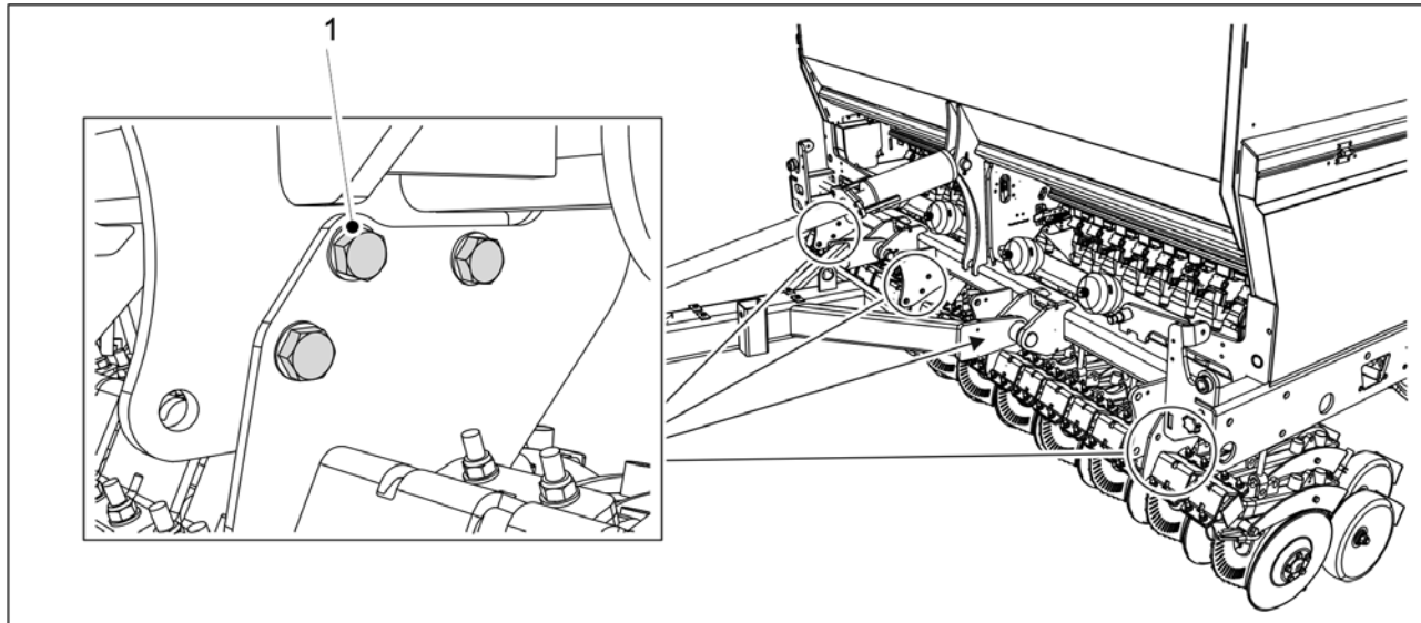
Billede. 7.1.2.4 - 256. Ristelraftbolter
