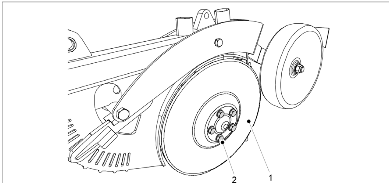
Billede. 7.8.2.1 - 320. Ta av en skive
