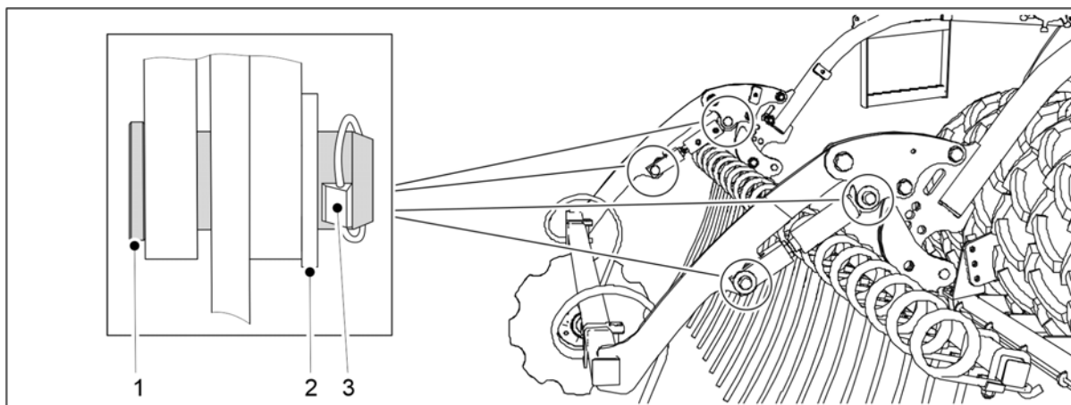
Billede. 5.1.14 - 90. Montere bakmarkørsynderne
