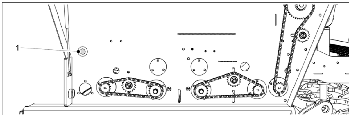
Billede. 6.8.2 - 188. Trykknapp
