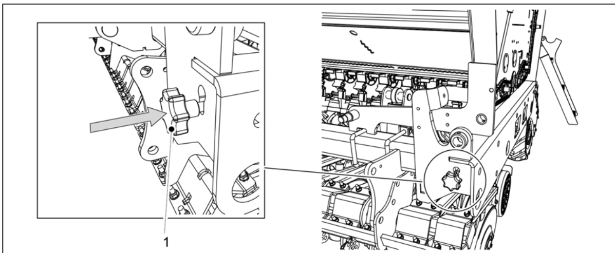
Billede. 6.8.2 - 193. Sette inn kalibreringstestens justeringsstang
