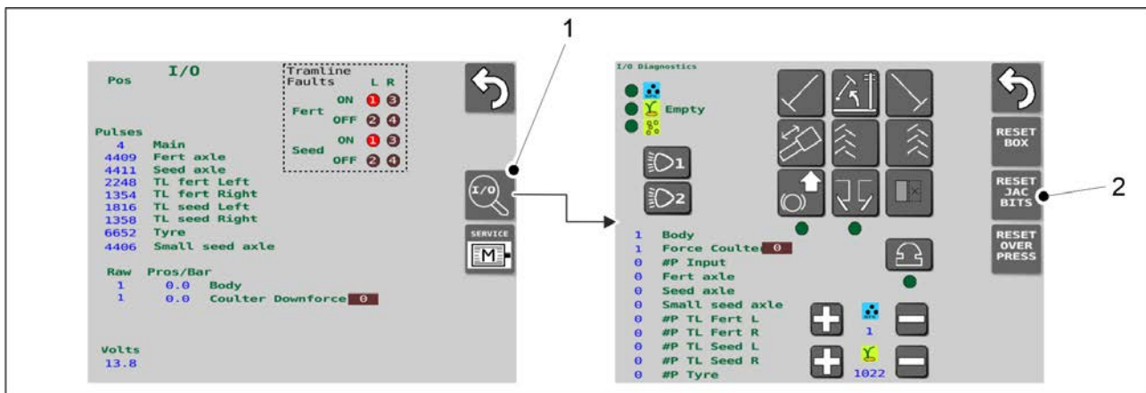
Billede. 7.9.4.1 - 339. Nullstilling av feilminnet for trikkeskinnclutchen
