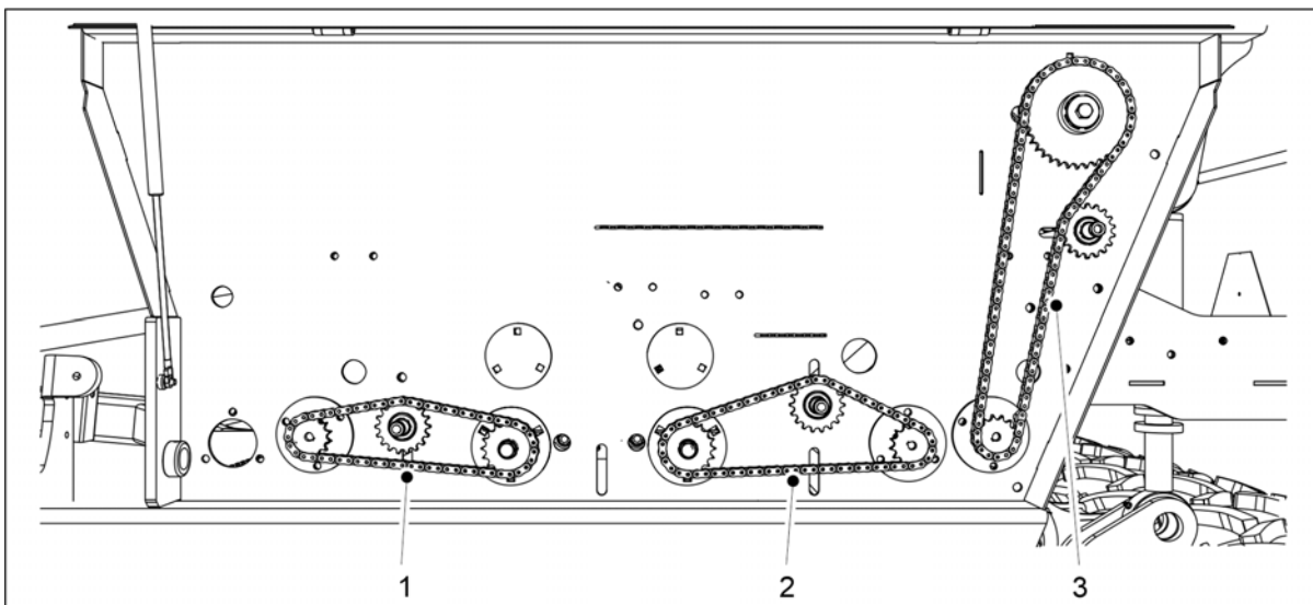
Billede. 7.2.2 - 270. Smøre kraftoverføringskjedene
