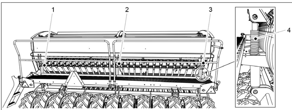
Billede. 6.26 - 250. Sylindersperrer
