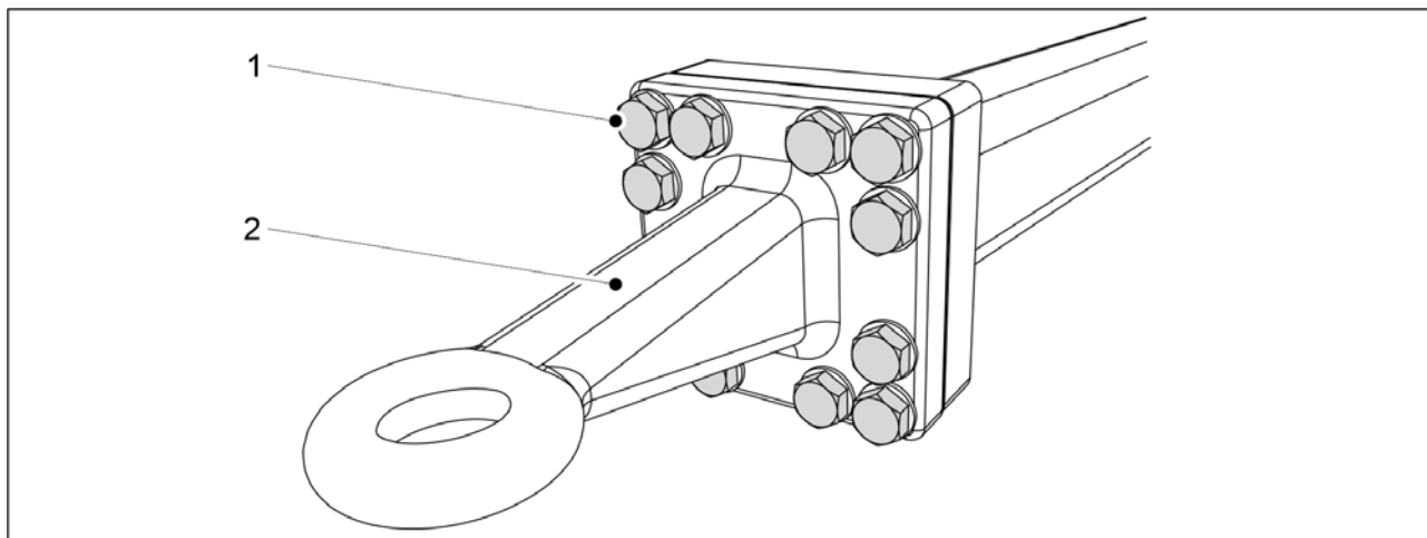
Billede. 7.7.1.1 - 312. Tauemalje
