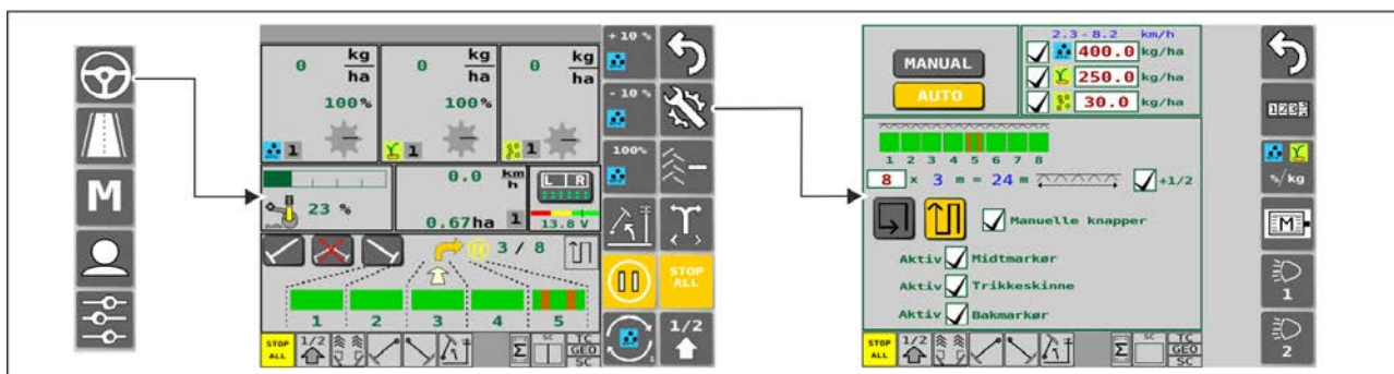
Billede. 4.1.2 - 29. Kjøreskjermbilde og såinnstillinger (automatisk)
