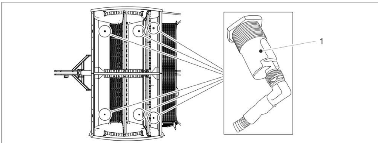
Billede. 4.1.1.6 - 20. Traktnivåsensorer
