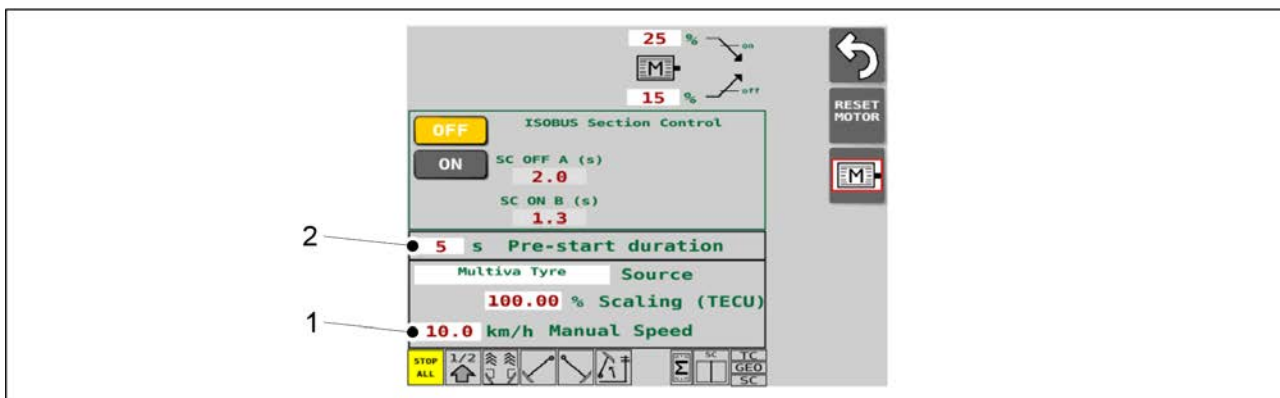
Billede. 6.9 - 203. Innstillinger for PRESTART-funksjonen
