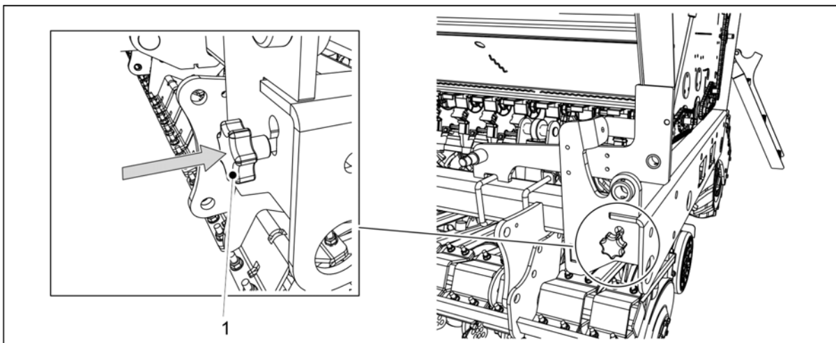
Billede. 6.8.3 - 202. Sette inn kalibreringstestens justeringsstang
