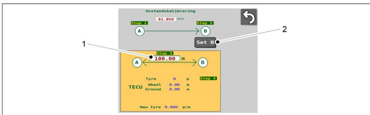
Billede. 7.9.2.1 - 334. Kjørekalibrering 2
