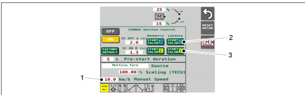
Billede. 6.11.2.2 - 217. Starte forsinkelseskalibreringen
