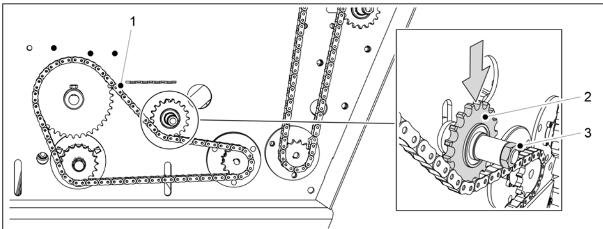
Billede. 7.5.4 - 309. Stramme kjedet for frøspredningsakselen
