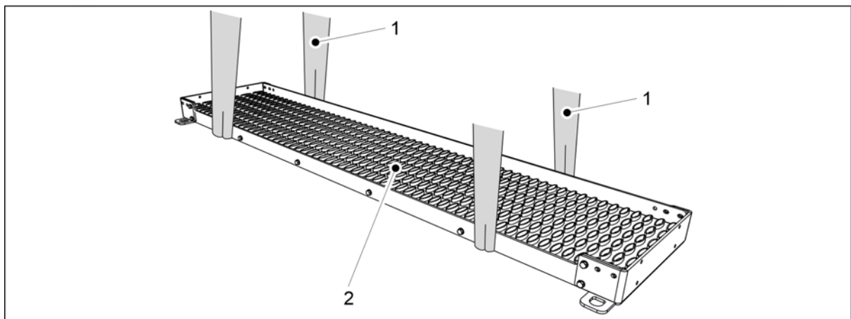
Kuva. 5.1.16 - 97. Kävelytason nostaminen
