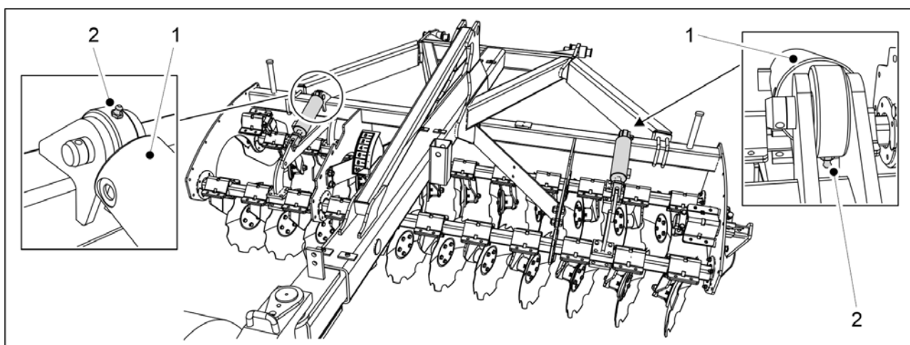
Kuva. 7.2.13 - 280. Etukiekkomuokkaimen sylinterit
