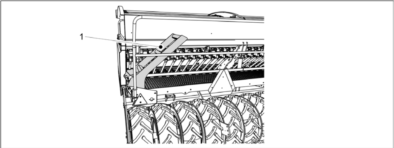
Kuva. 6.7 - 171. Hoitotason rappuset
