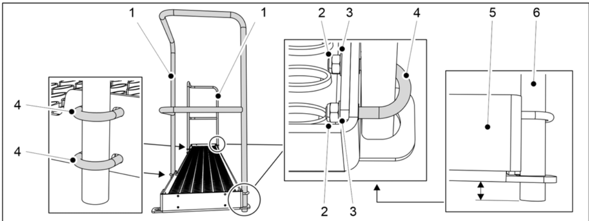
Kuva. 5.1.15 - 94. Kaiteiden kiinnittäminen eCEREX 400 -koneessa
