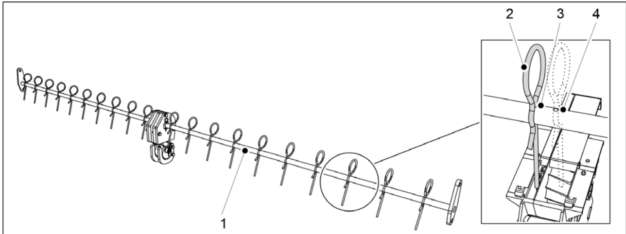
Kuva. 6.19.3 - 236. Piensiemenen heilurisekoitin
