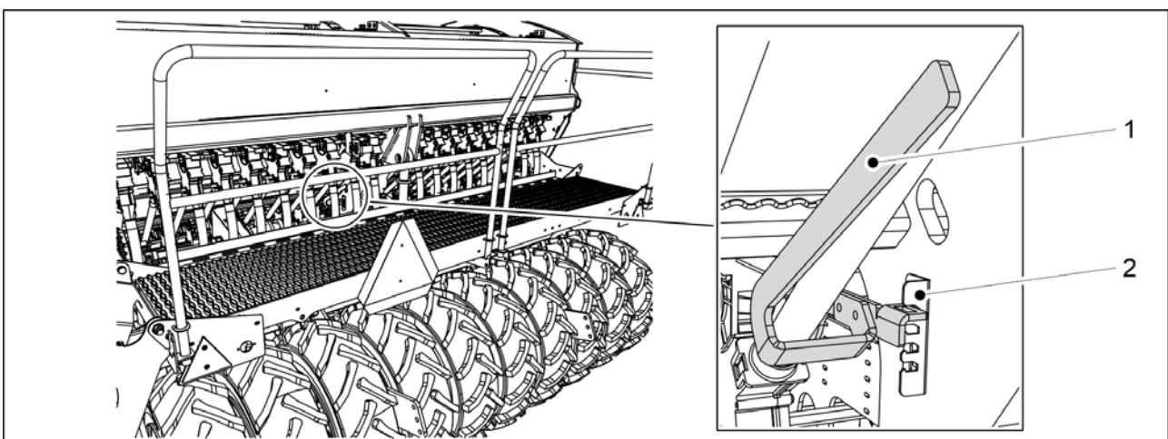
Kuva. 6.6.7.1 - 164. Syöttöyksiköiden pohjaläppien säätövipu, siemensäiliö
