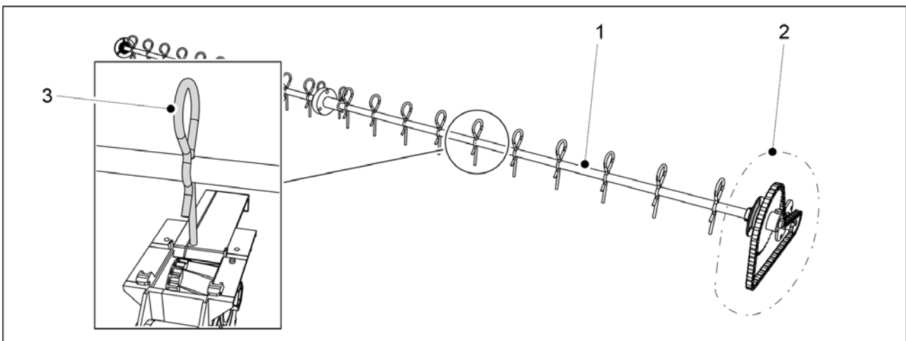
Kuva. 6.19.2 - 235. Siemenen karistaja-akseli
