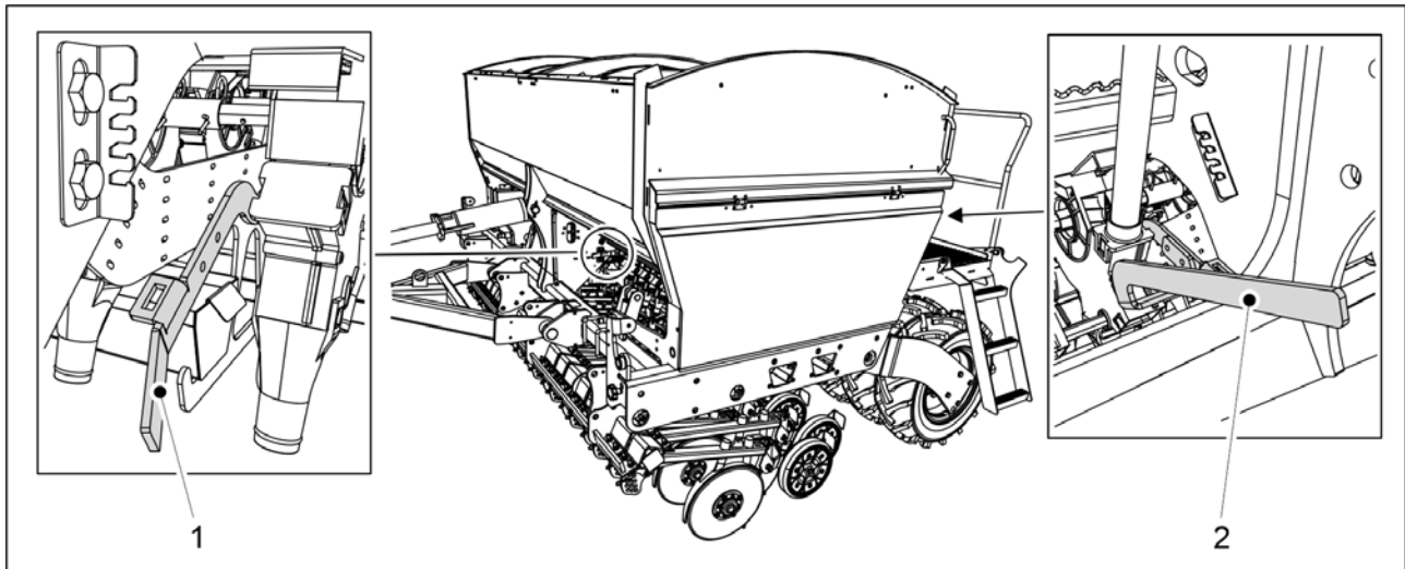
Kuva. 6.23.2 - 241. Säiliöiden pohjaläpän avaaminen
