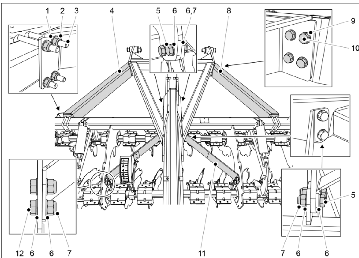
Kuva. 5.1.6 - 66. Etukiekkomuokkaimen kiinnittäminen vetopuomiin
