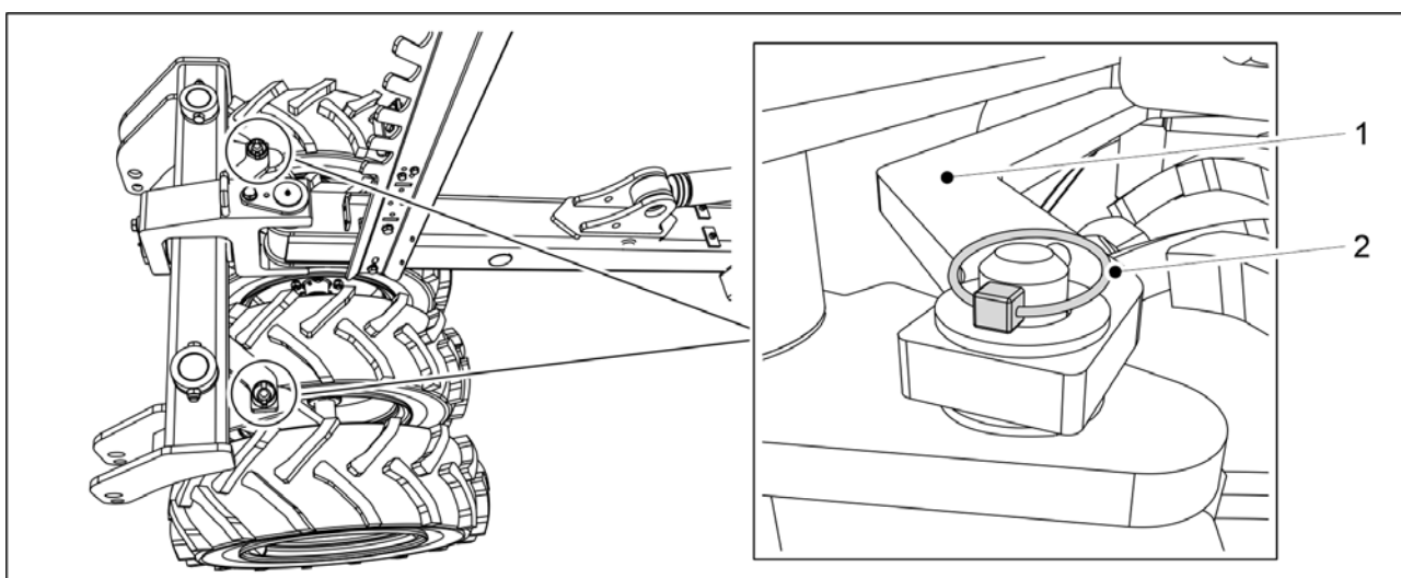
Kuva. 7.1.2.3 - 251. Pyöränvälilyrjän tanko
