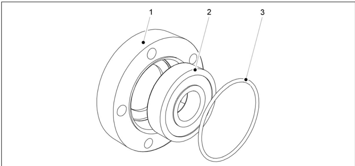
Kuva. 7.8.3.1 - 323. Laakerin ja O-renkaan irrottaminen
