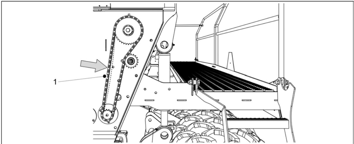
Kuva. 7.1.5.2 - 261. Ketjujen kireyden tarkastus, piensiemenen voimansiirto
