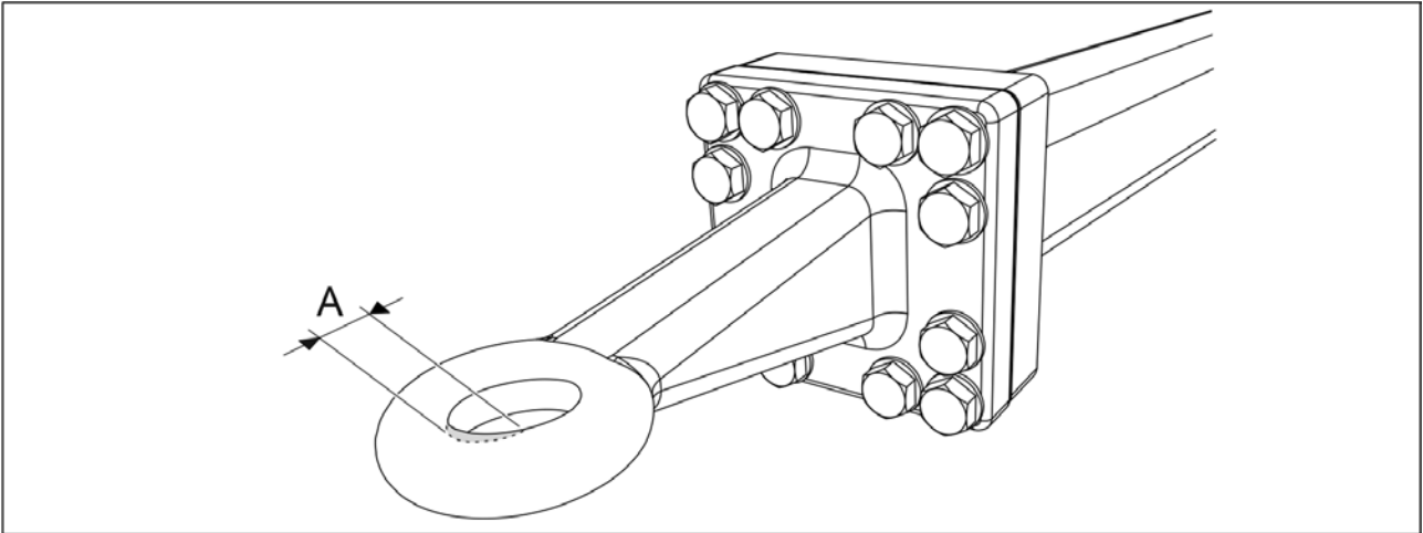
Kuva. 7.1.8 - 264. Vetolenkin kuluma
