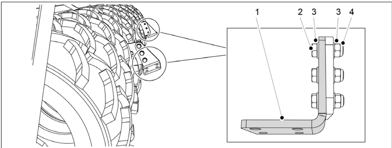
Kuva. 5.1.11 - 76. Kiviraapan ripustuslevyjen kiinnittäminen
