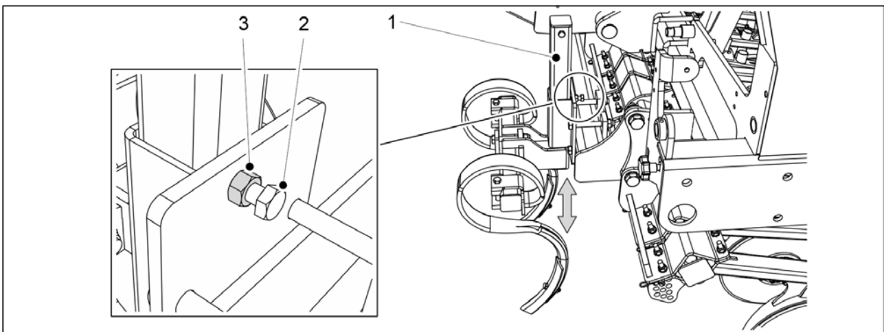
Kuva. 6.18.1 - 232. Ajourakuohkeuttimen korkeuden säätäminen
