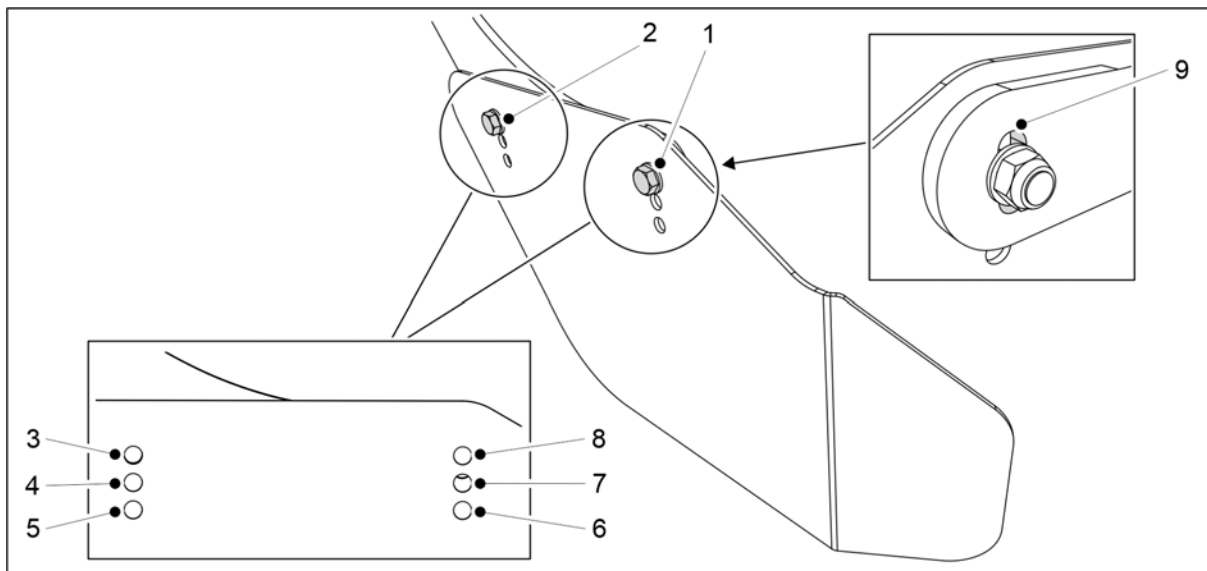
Kuva. 6.17 - 230. Sivurajoittimen korkeuden ja kulman säätäminen
