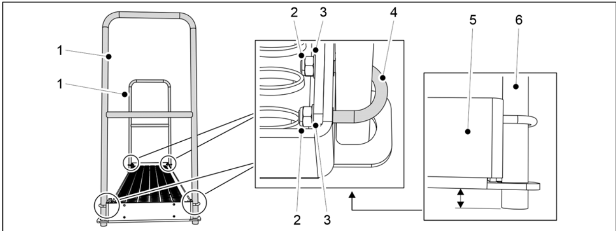
Kuva. 5.1.15 - 93. Kaiteiden kiinnittäminen eCEREX 300 -koneessa
