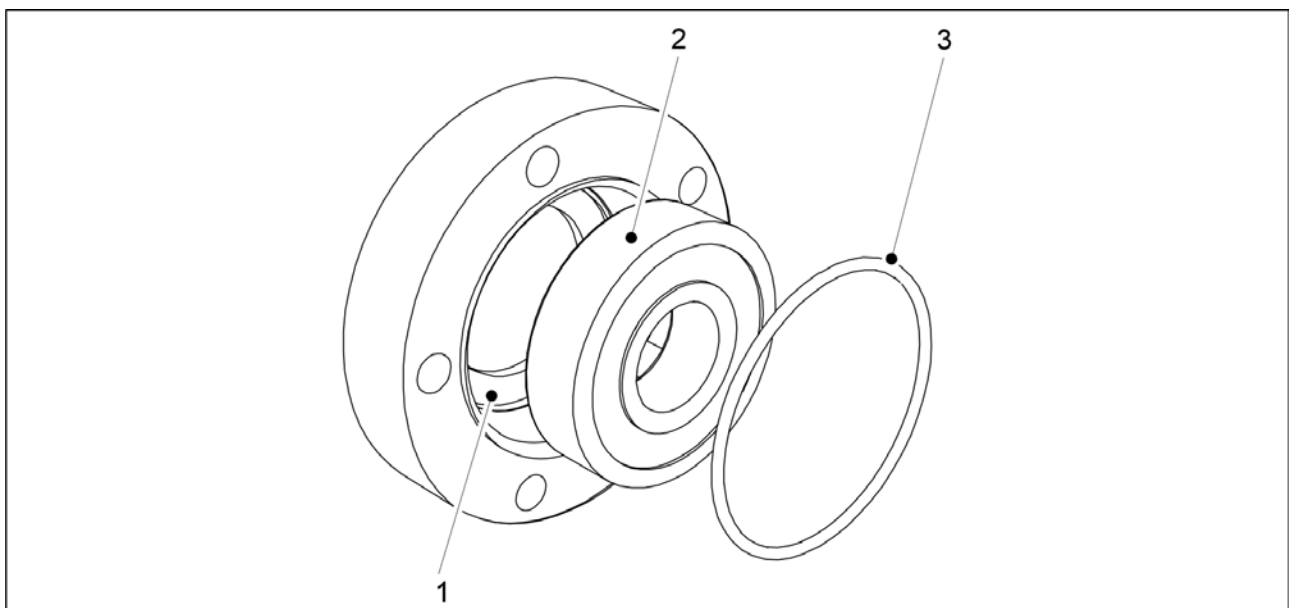
Kuva. 7.8.3.2 - 324. Laakerin asennus
