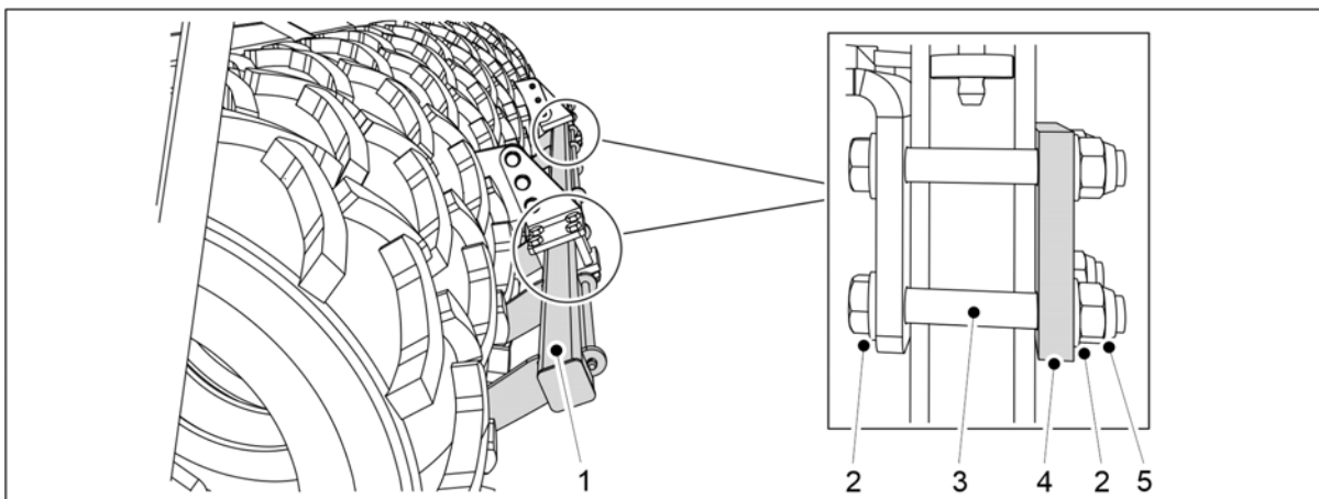
Kuva. 5.1.11 - 77. Kiviraapan kiinnittäminen
