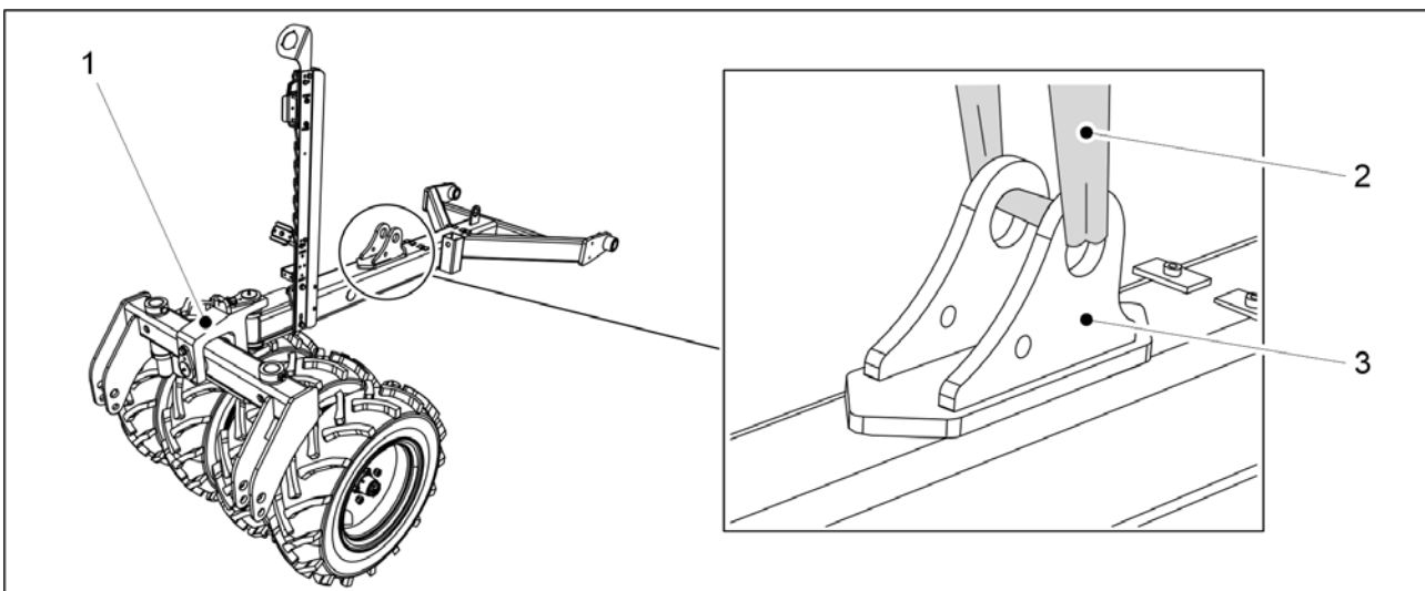
Kuva. 5.1.1 - 53. Pyöränvälijyrän nostaminen
