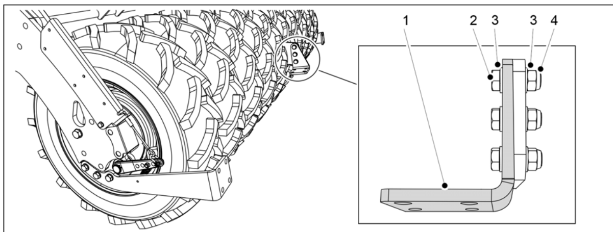
Kuva. 5.1.12 - 80. Kiviraapan ripustuslevyn kiinnittäminen
