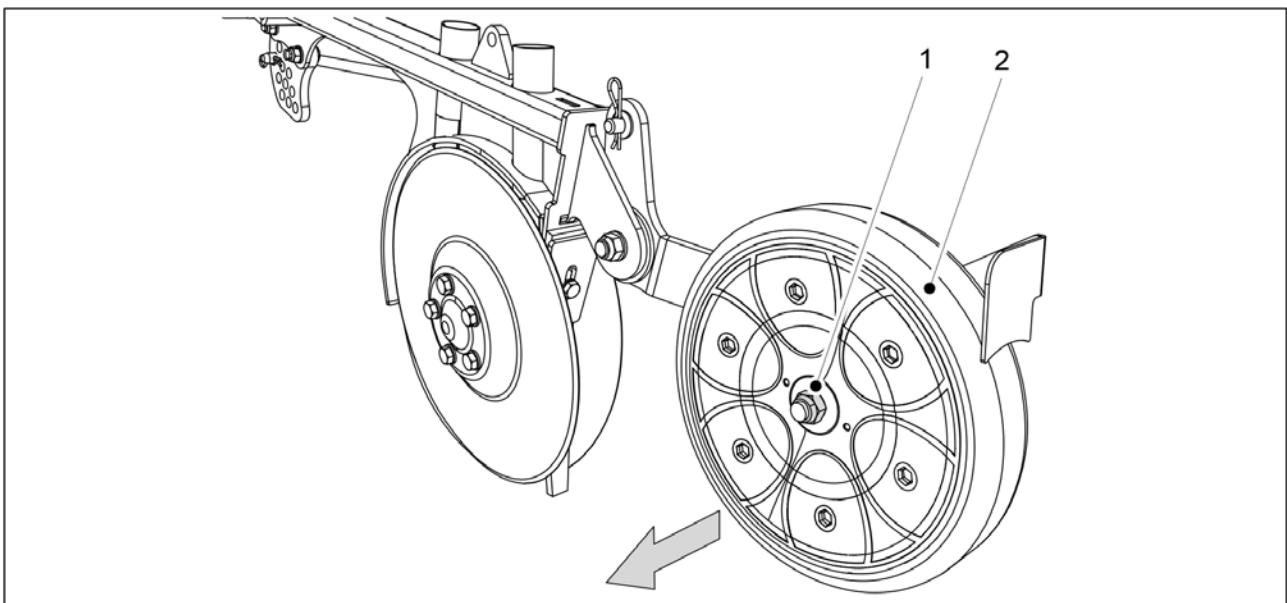
Kuva. 7.8.4.1 - 326. Peittopyörän irrotus
