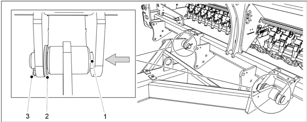
Kuva. 5.1.1 - 54. Pyöränvälijyrän kiinnittäminen
