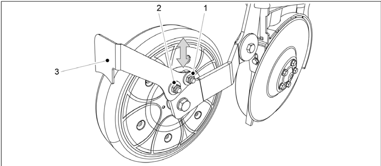
Kuva. 7.8.5.2 - 329. Peittopyörän raappalevy
