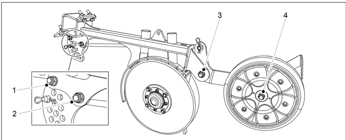
Kuva. 7.1.2.4 - 255. Vantaan peittopyörän ja syvyysäädön pultit
