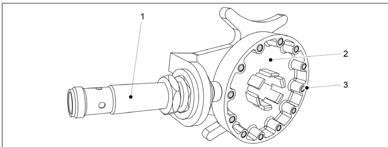
Kuva. 4.1.1.5 - 18. Pyörintävähti
