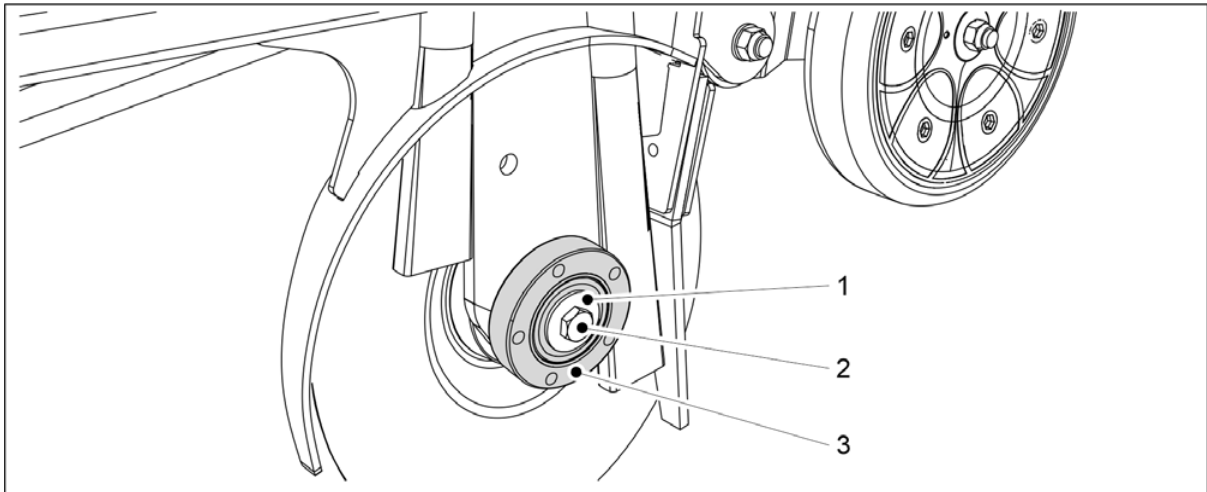
Kuva. 7.8.2.1 - 319. Laakeripesän irrotus
