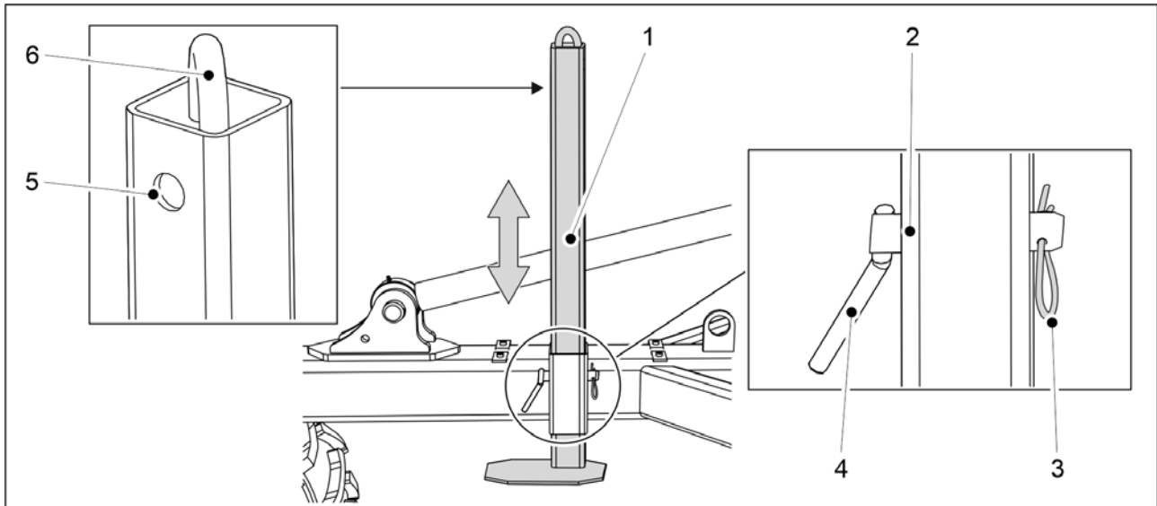
Kuva. 5.3.2 - 116. Maatuki
