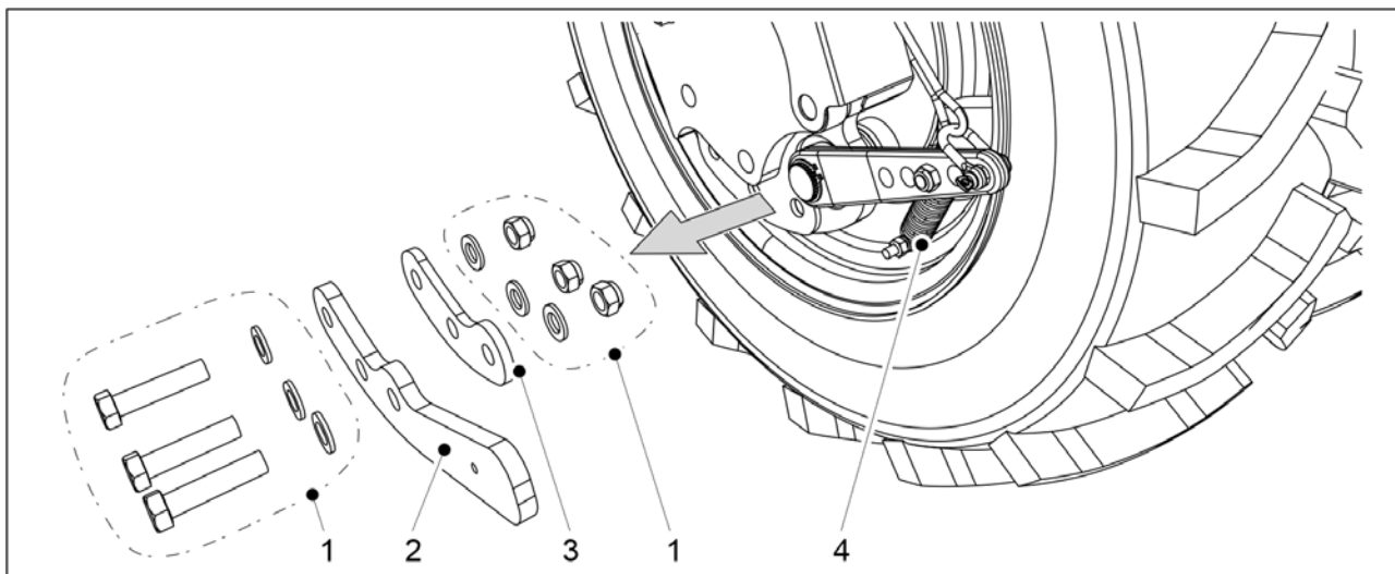
Kuva. 5.1.12 - 78. Vivun ja välilevyn irrotus
