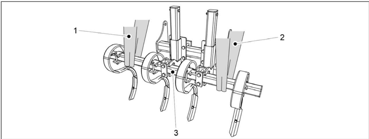
Kuva. 5.1.7 - 70. Ajourakuohkeuttimen nostaminen
