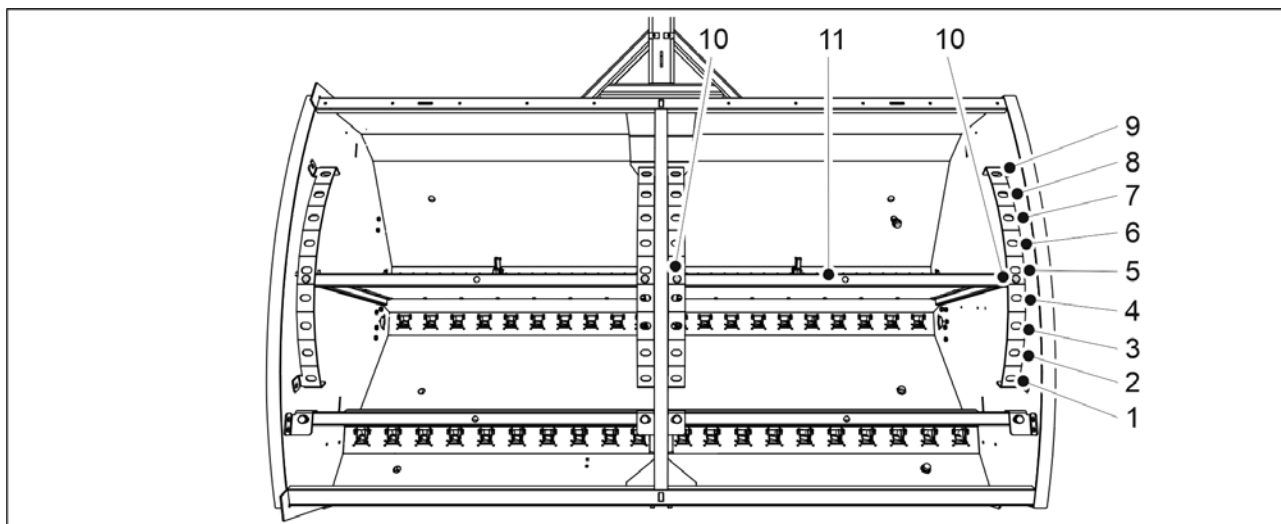
Kuva. 6.6.4 - 158. Säiliön väliseinän säätäminen
