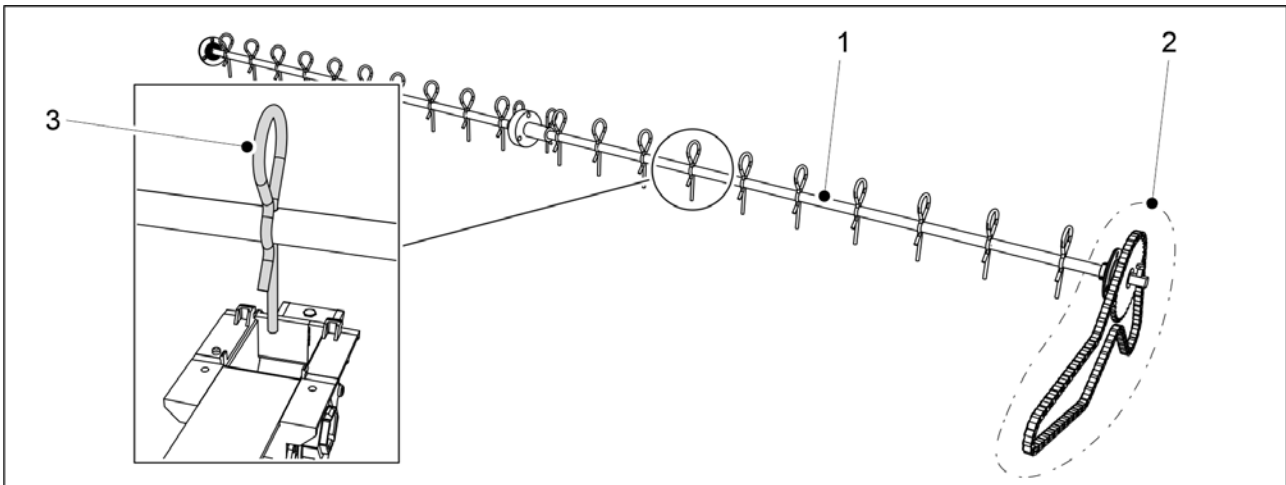
Kuva. 6.19.1 - 234. Lannoitteen karistaja-akseli
