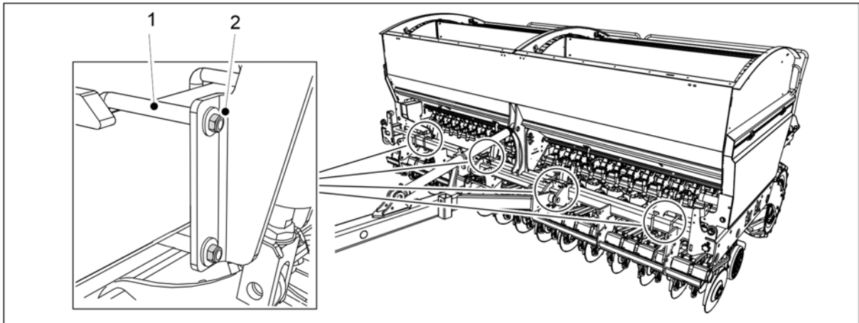
Kuva. 7.1.2.4 - 254. Vannaspainatuksen pultit
