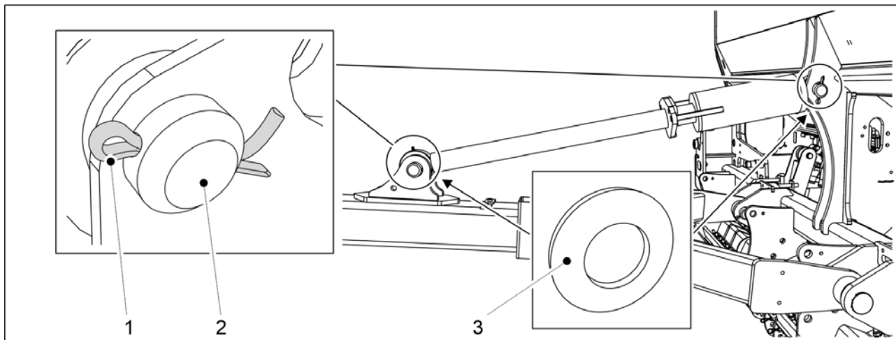
Kuva. 5.1.2 - 57. Aisasynteri
