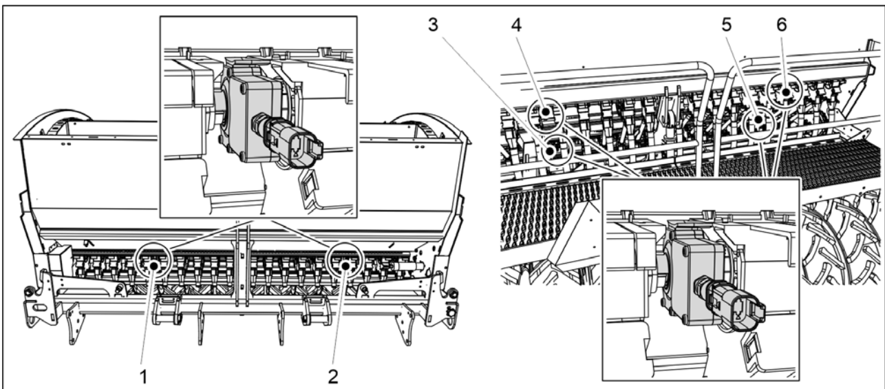
Kuva. 4.1.1.7 - 20. Ajourakytkimien sijainti
