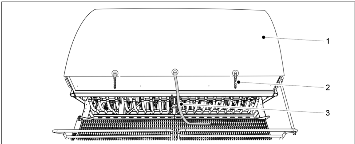
Kuva. 6.7 - 172. Säiliön pressu
