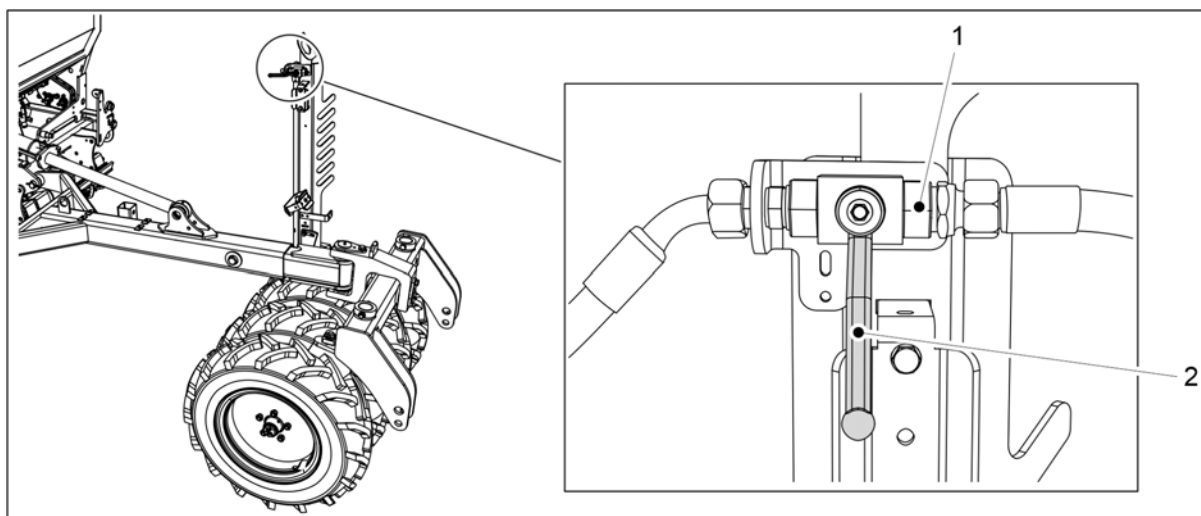
Kuva. 5.3.5 - 122. Nostopiirin sulkuhanan sulkeminen
