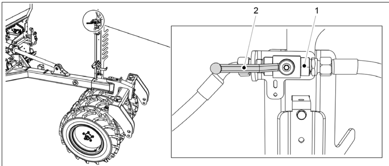
Kuva. 5.3.5 - 121. Nostopiirin sulkuhanan avaaminen
