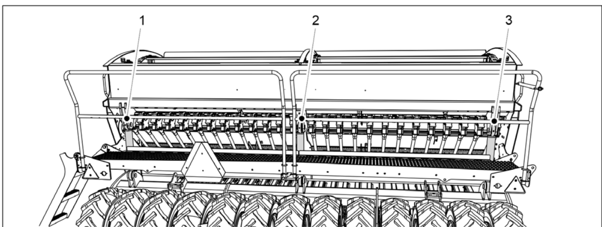
Kuva. 6.2 - 129. Nostosylinteri
