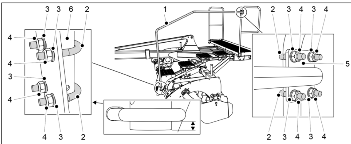
Kuva. 5.1.16 - 102. Porraskaiteen kiinnittäminen
