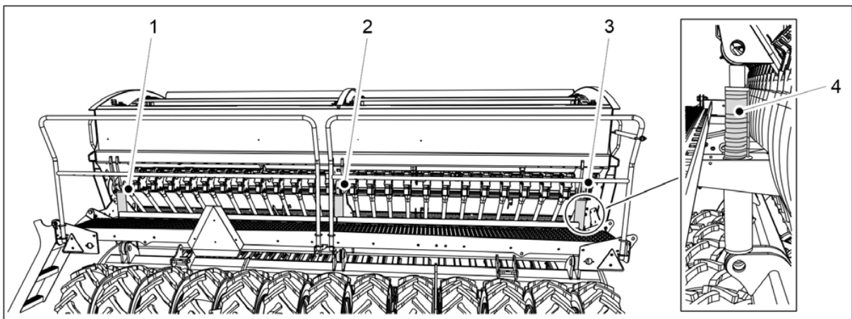
Kuva. 6.26 - 247. Sylinterin rajoitinpalat
