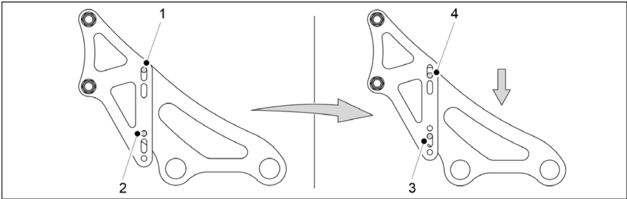
Kuva. 6.16 - 227. Etuharan korkeuden säätäminen
