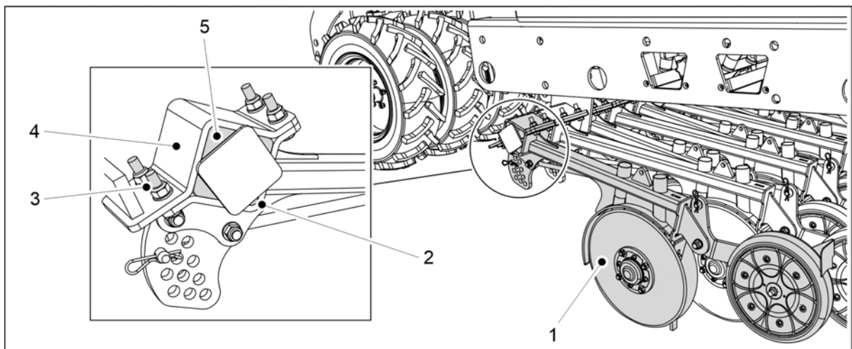
Kuva. 7.8.1.2 - 316. Vantaan kiinnitys
