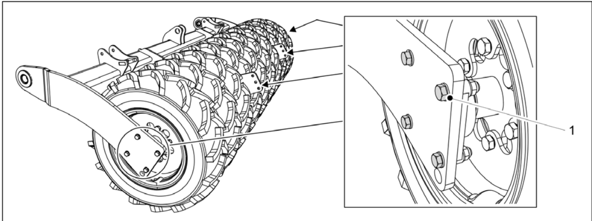
Kuva. 7.4.1 - 296. Rengaspaketin irrotus
