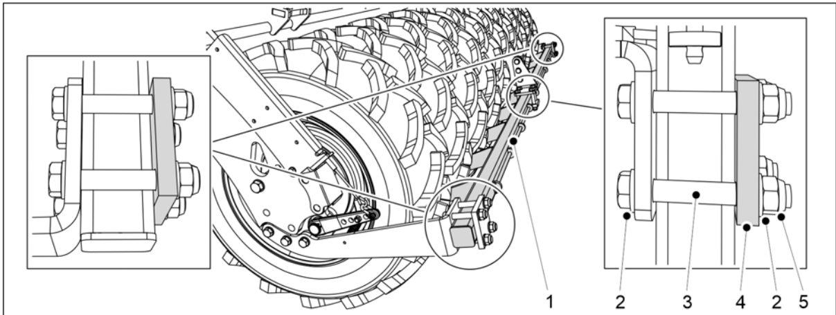
Kuva. 5.1.12 - 81. Kiviraapan kiinnittäminen
