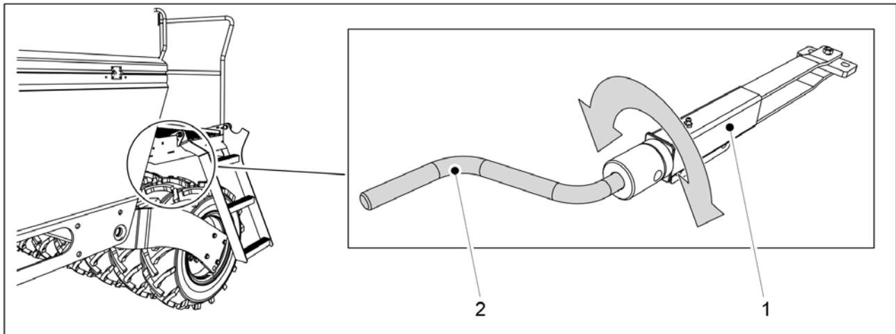
Kuva. 6.22.1 - 237. Seisontajarru
