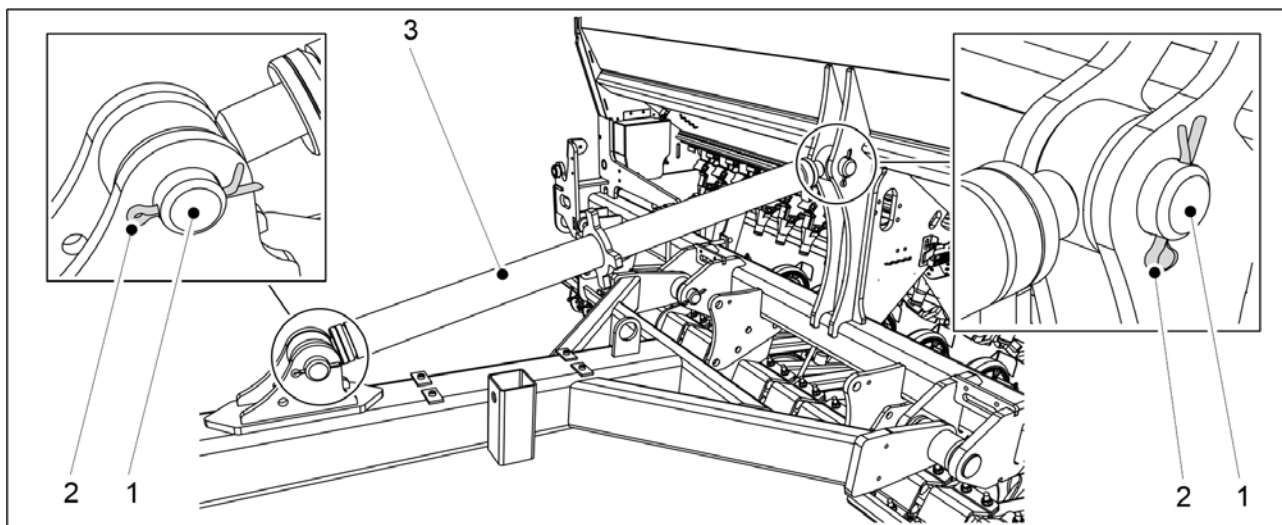
Kuva. 5.1.3 - 58. Vanttiruuvi
