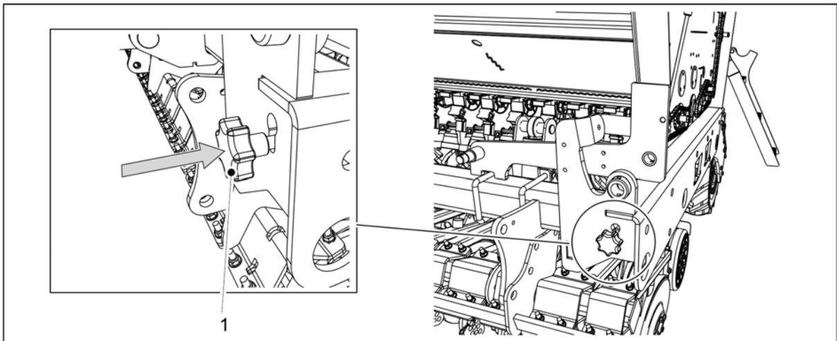
Kuva. 6.8.3 - 200. Kiertokokeen säätötangon sisääntyöntö
