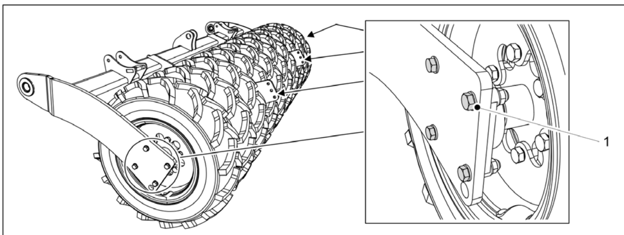
Kuva. 7.4.4 - 303. Rengaspaketin kiinnittäminen
