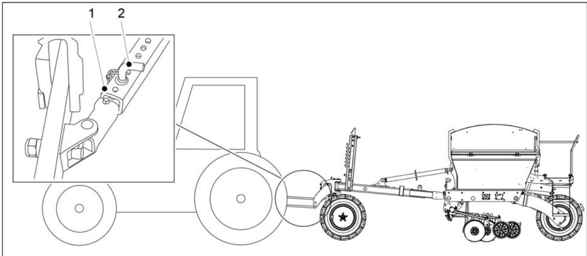
Kuva. 5.3 - 114. Traktorin vetovarsien sivurajoittimet
