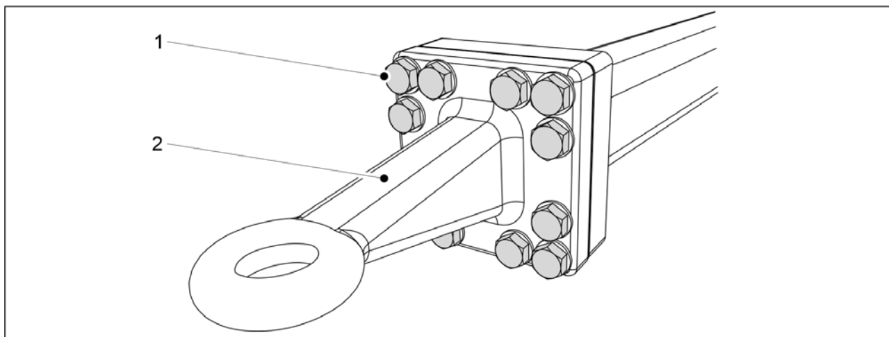
Kuva. 7.7.1.2 - 312. Vetolenkki
