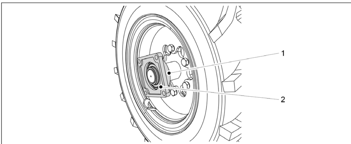
Kuva. 7.4.3 - 302. Laakerin kiinnittäminen
