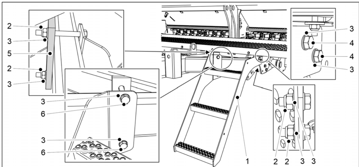
Kuva. 5.1.15 - 95. Rappusten kiinnittäminen
