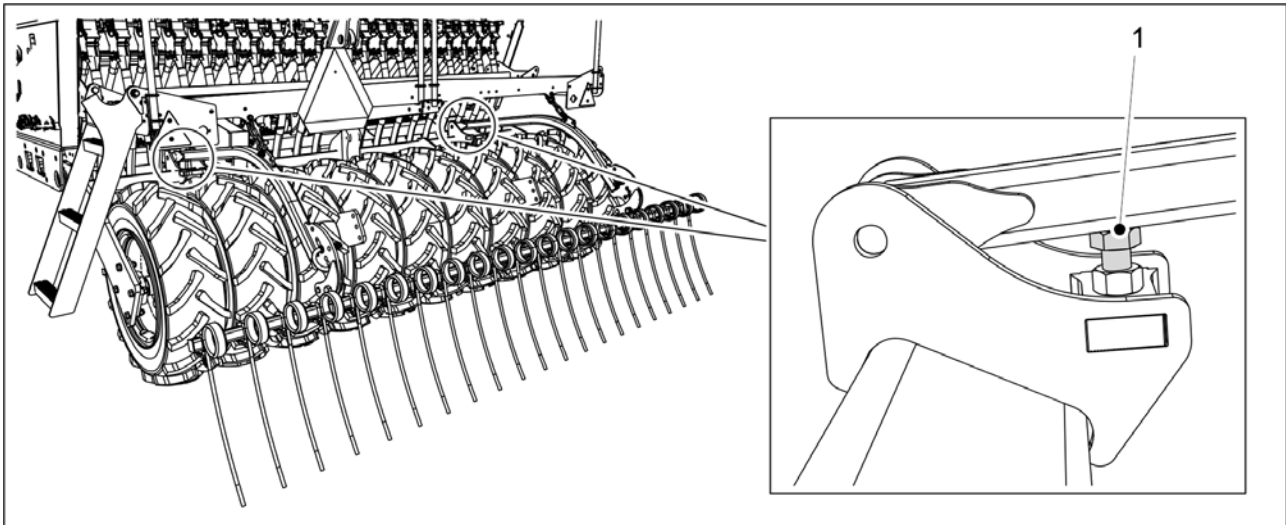
Kuva. 6.14 - 223. Jälkiharan korkeuden säätäminen
