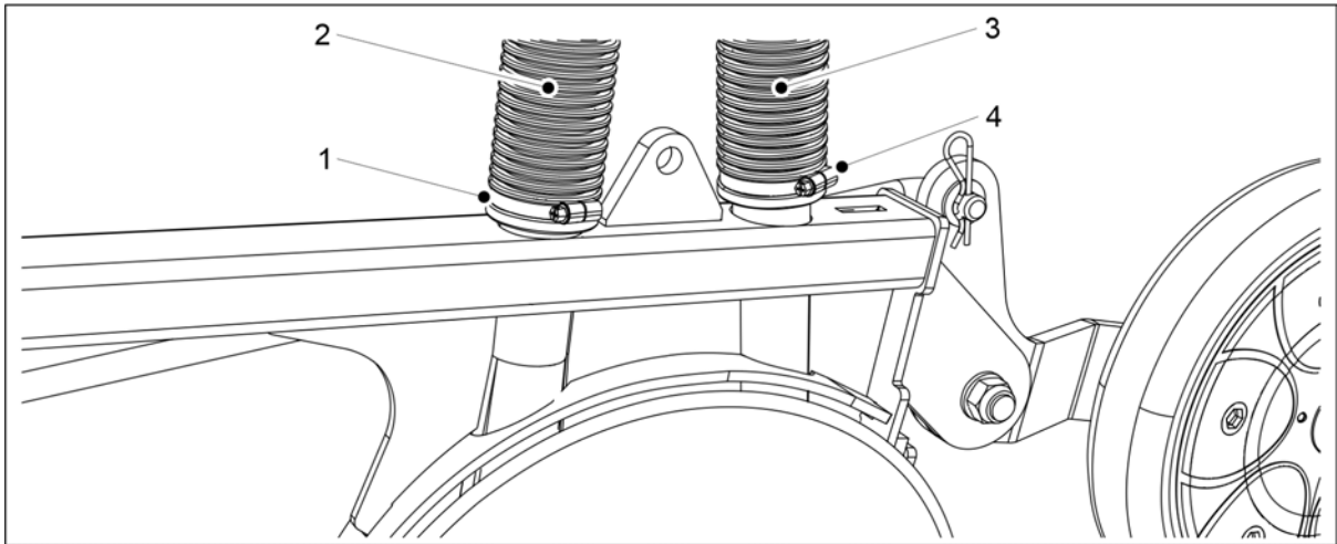
Kuva. 7.8.1.2 - 317. Vantaan letkujen asennus
