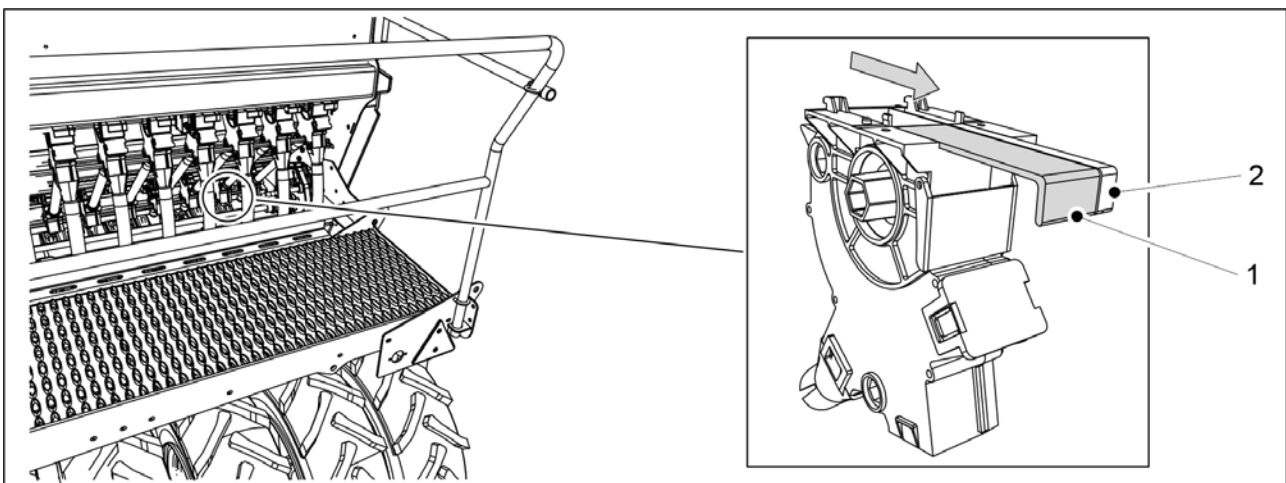
Kuva. 6.6.7.2 - 166. Sulkuluukut siemenen syöttöyksikössä
