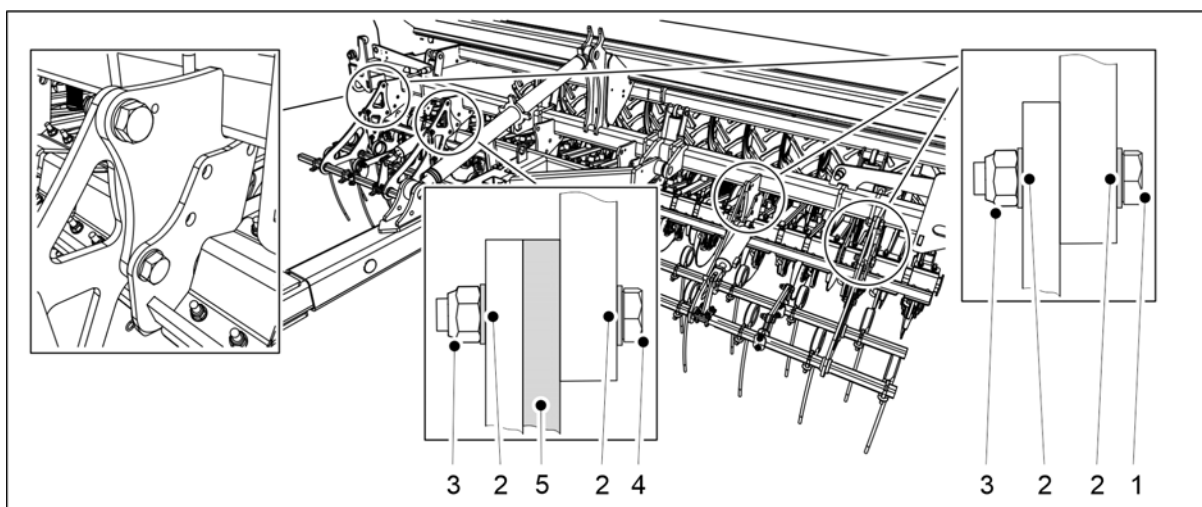
Kuva. 5.1.5 - 63. Etuharan kiinnittäminen
