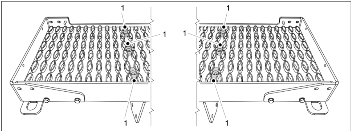
Kuva. 5.1.15 - 91. Kävelytason kiinnikkeet
