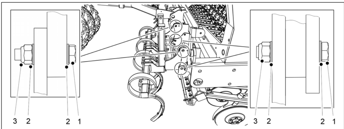
Kuva. 5.1.7 - 71. Ajourakuohkeuttimen kiinnittäminen
