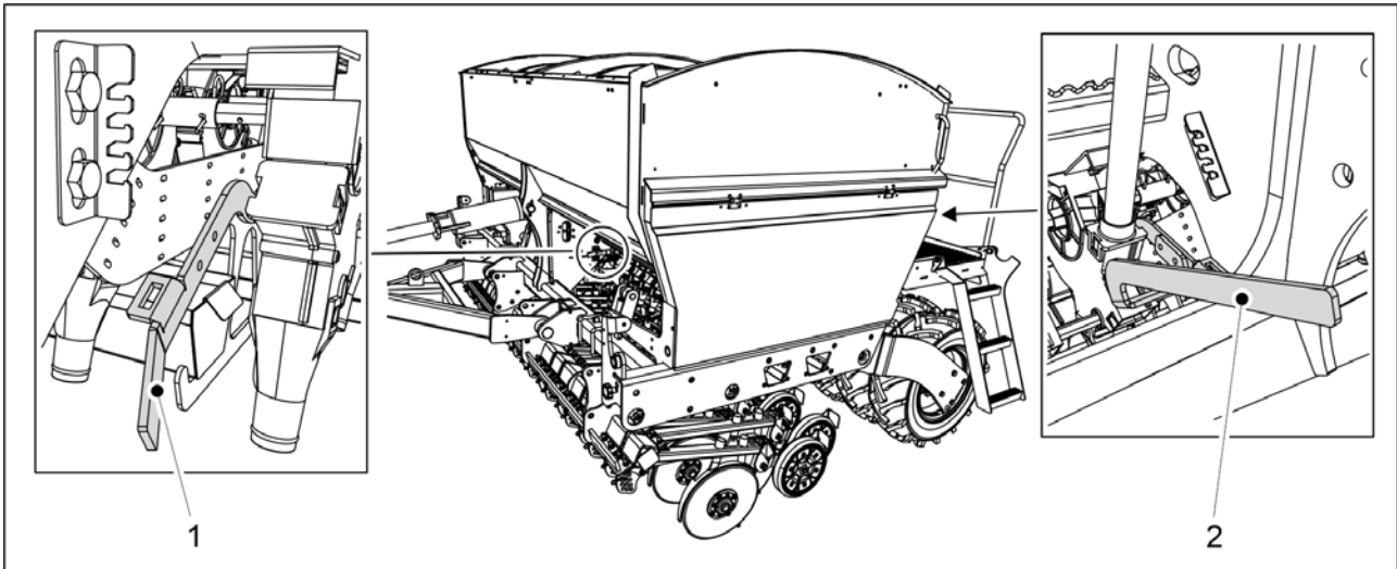
Kuva. 7.3.1 - 285. Pohjaläpät auki
