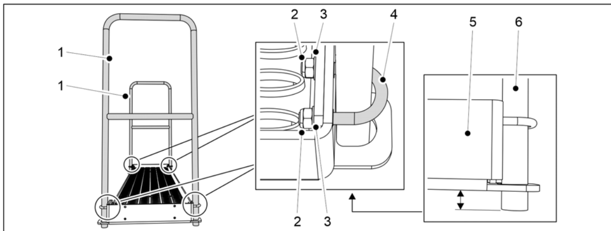
Kuva. 5.1.16 - 100. Kaiteiden kiinnittäminen 300-koneessa
