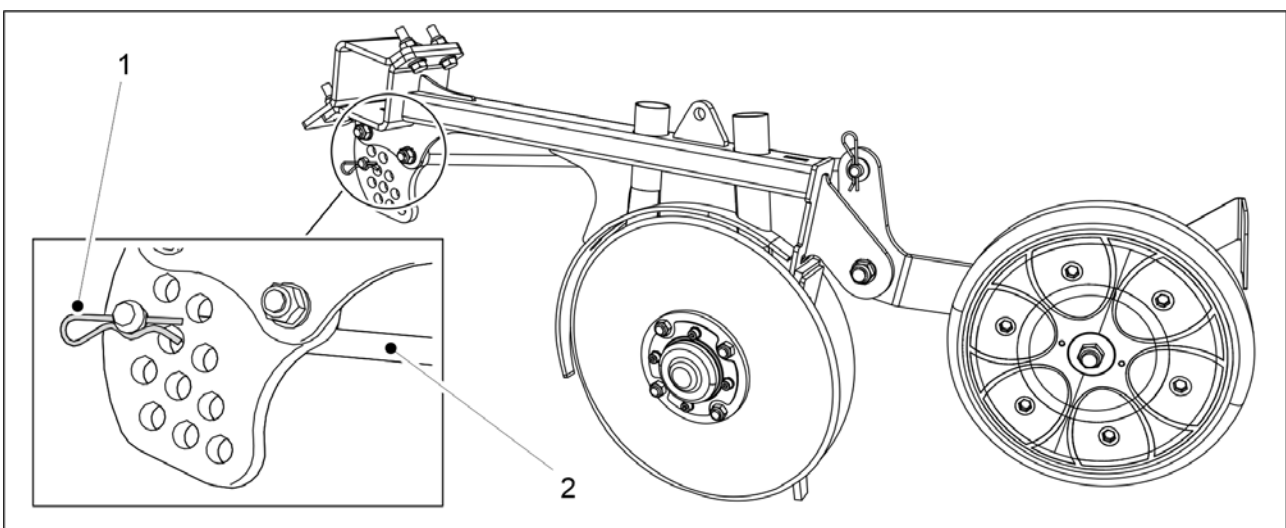
Kuva. 6.12 - 221. Vantaan kylvösyvyyden säätäminen
