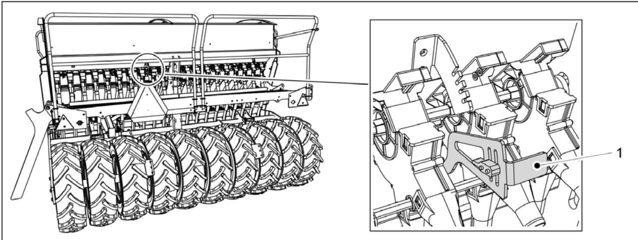
Kuva. 7.3.2 - 287. Pohjaläppä auki
