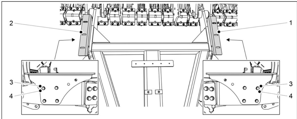
Kuva. 5.1.16 - 96. Kävelytason kannattimien kiinnittäminen
