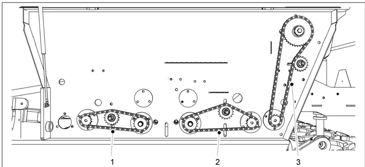
Kuva. 7.2.2 - 268. Voimansiirron ketjujen voitelu
