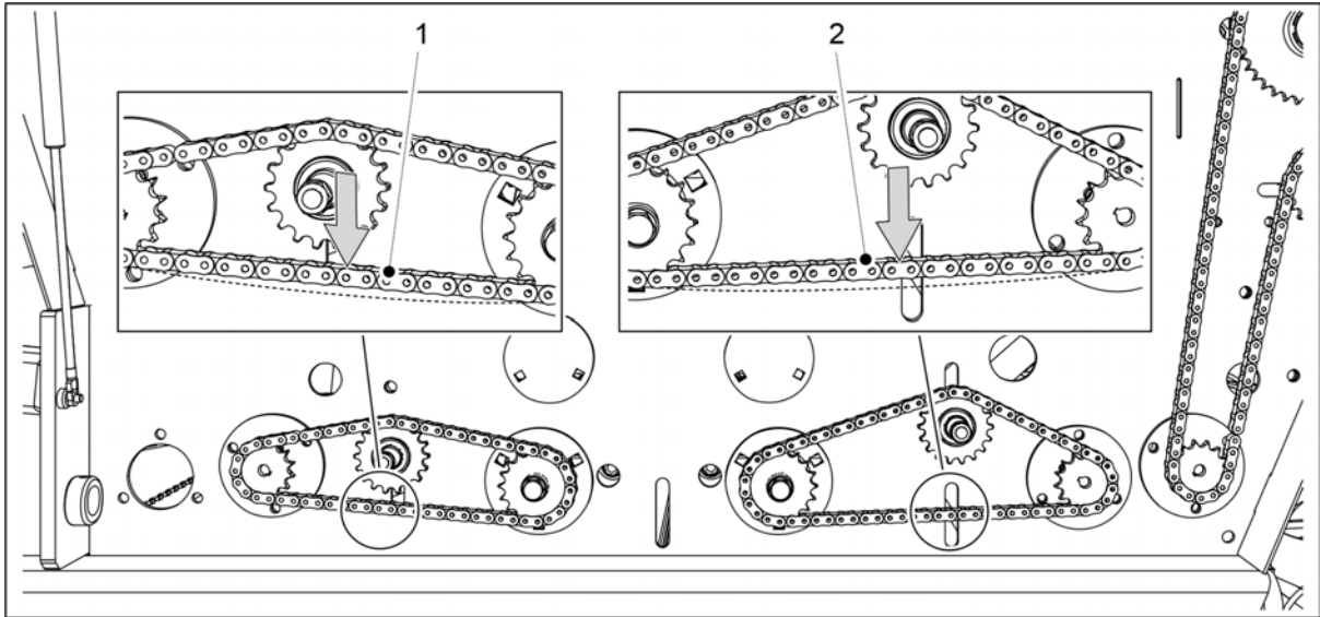
Kuva. 7.1.5.1 - 260. Ketjujen kireyden tarkastus, lannoitteen ja siemenen voimansiirto
