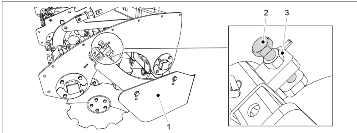
Kuva. 6.17 - 229. Sivurajoittimen ala-asennon säätäminen
