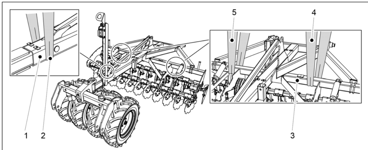
Kuva. 5.1.6 - 67. Vetopuomin ja etukiekkomuokkaimen nostaminen
