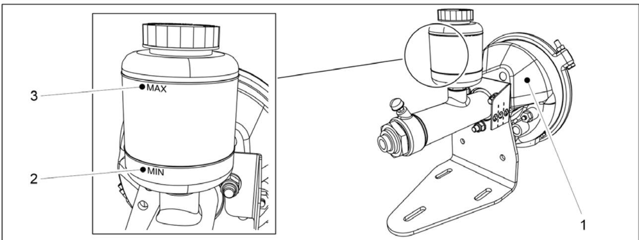
Kuva. 7.1.10.3 - 267. Paineilma-hydraulimuuntimen öljytason tarkastus
