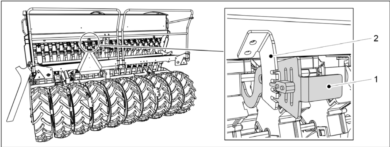
Kuva. 6.6.8.1 - 167. Syöttöyksiköiden pohjaläppien säätövipu, piensiemensäiliö
