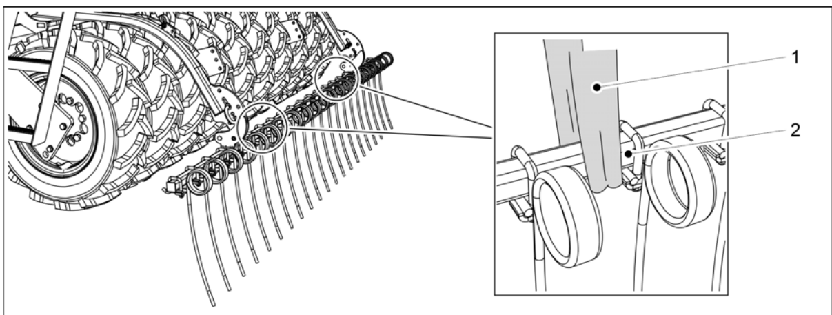
Kuva. 5.1.13 - 84. Jälkiharan nostaminen
