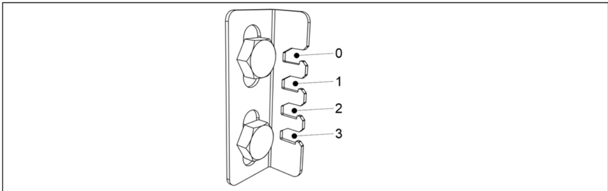
Kuva. 6.6.7.1 - 165. Säätövivun asennot / kylvettävä materiaali
