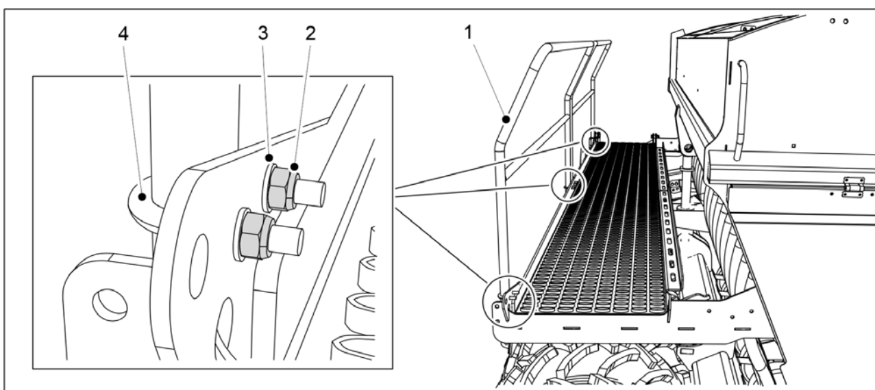
Kuva. 5.1.17 - 103. Hoitotason takakaiteen kääntäminen
