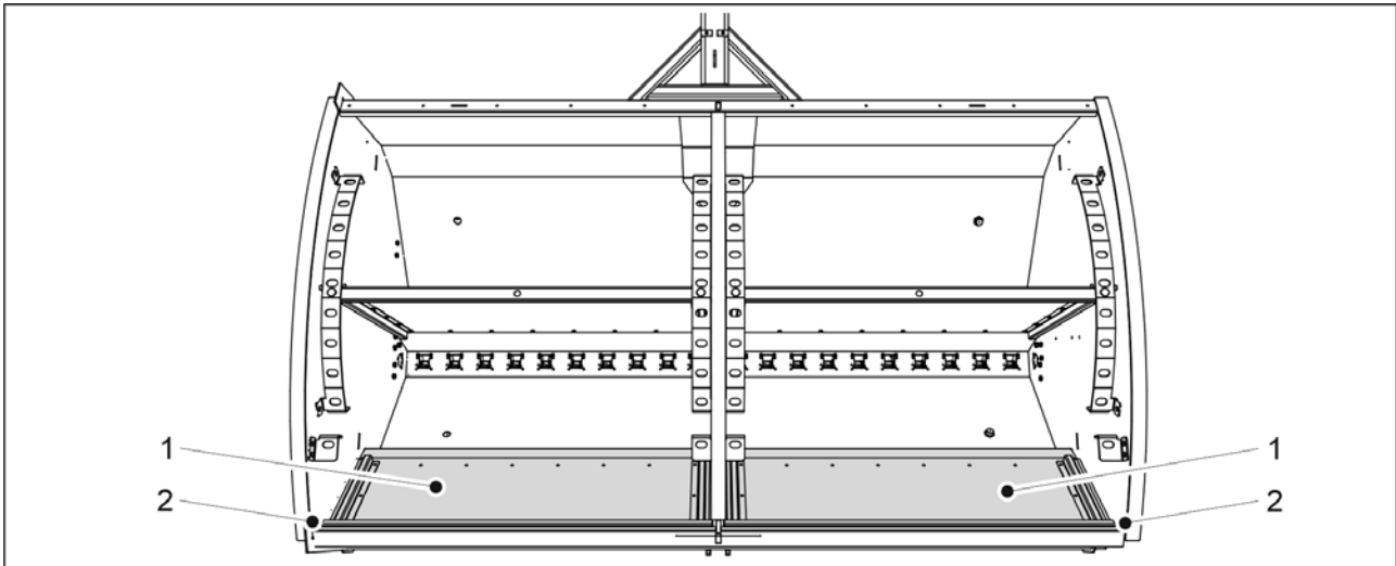
Kuva. 6.6.4.1 - 159. Piensiemensäiliön väliseinät käännettynä taakse
