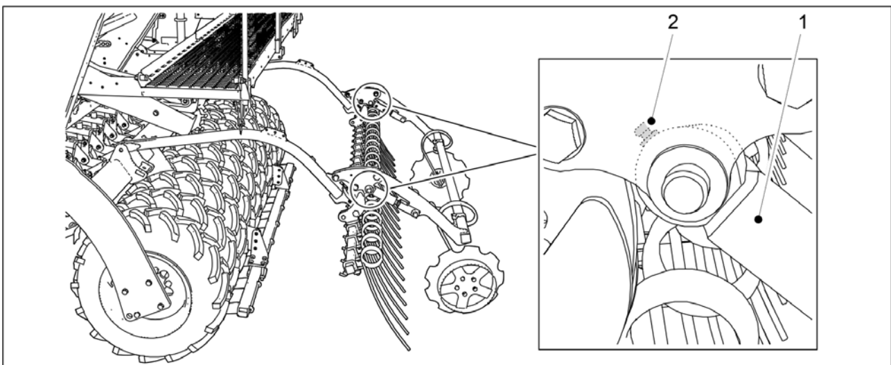
Kuva. 7.2.9 - 274. Takamerkkarisylinterit
