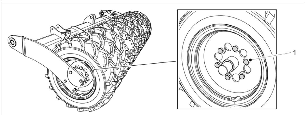
Kuva. 7.1.2.1 - 249. Kuljetuspyörien pyöränpultit
