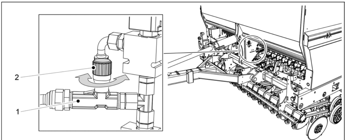
Kuva. 5.3.7 - 125. Keskimerkkarien nostonopeuden säätäminen
