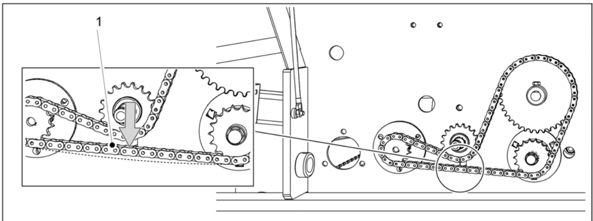
Kuva. 7.1.5.3 - 262. Ketjujen kireyden tarkastus, lannoitteen karistaja-akselin voimansiirto
