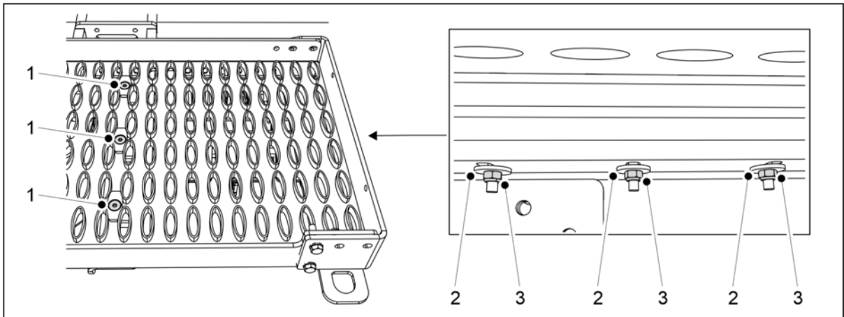
Kuva. 5.1.15 - 92. Kävelytason kiinnitys kannattimiin
