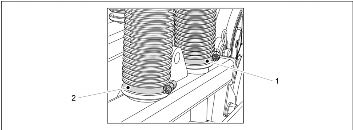
Kuva. 5.1.10 - 75. Siemen- ja lannoiteputken kiinnitys vantaalle
