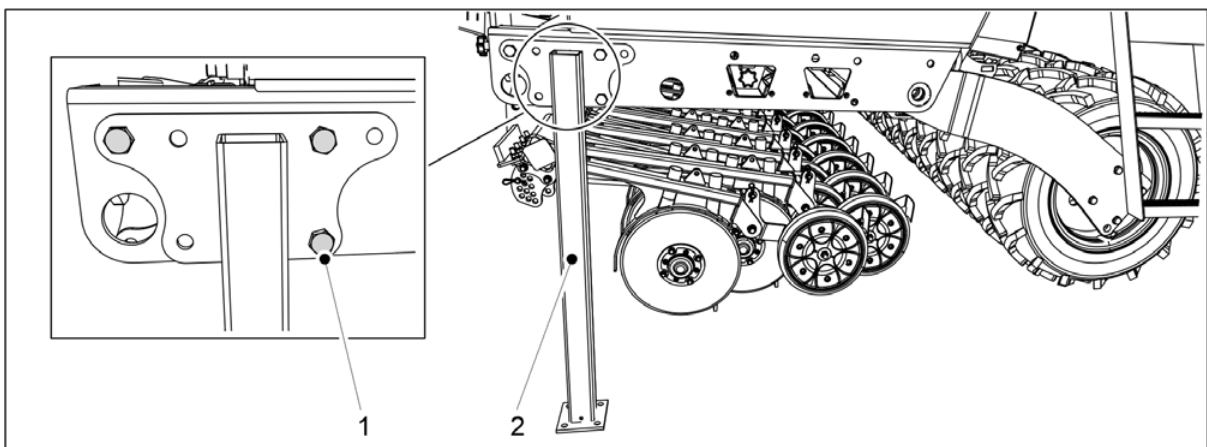
Kuva. 7.4.1 - 295. Kuljetustuet
