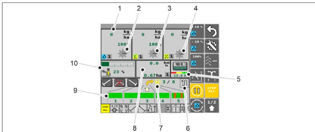
Kuva. 4.1.3.1 - 40. Ajonäyttö
