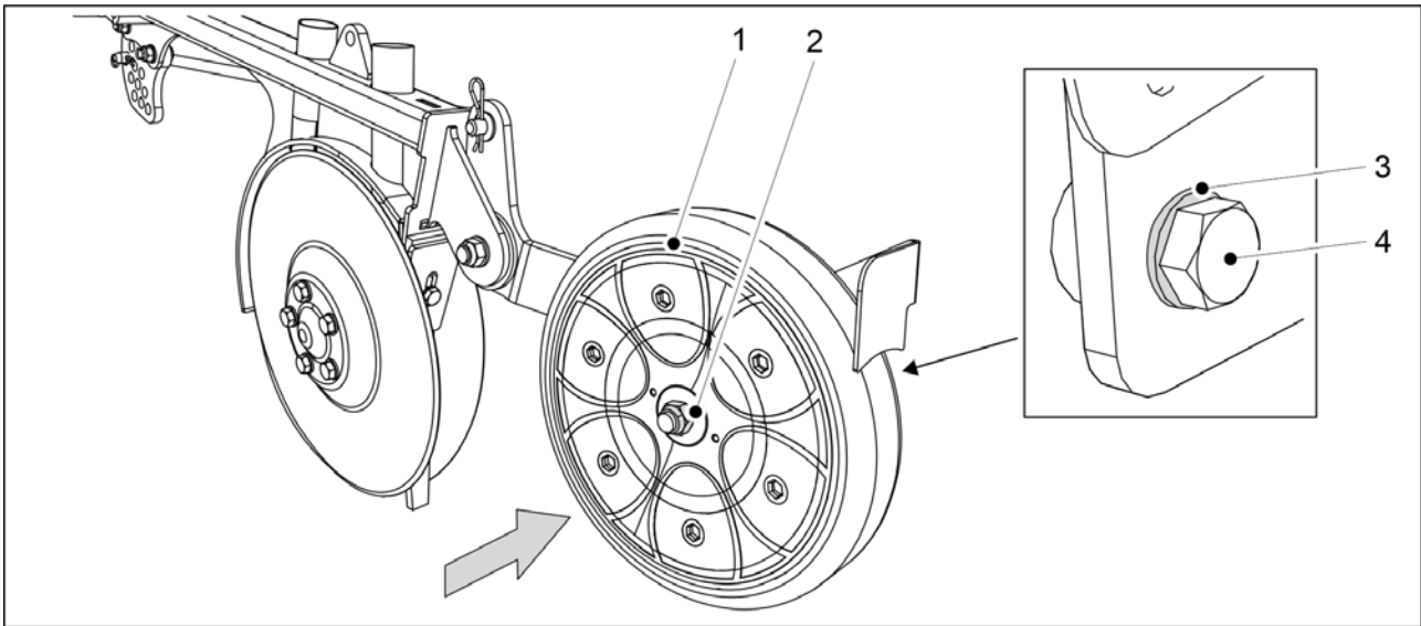
Kuva. 7.8.4.2 - 327. Peittopyörän asennus
