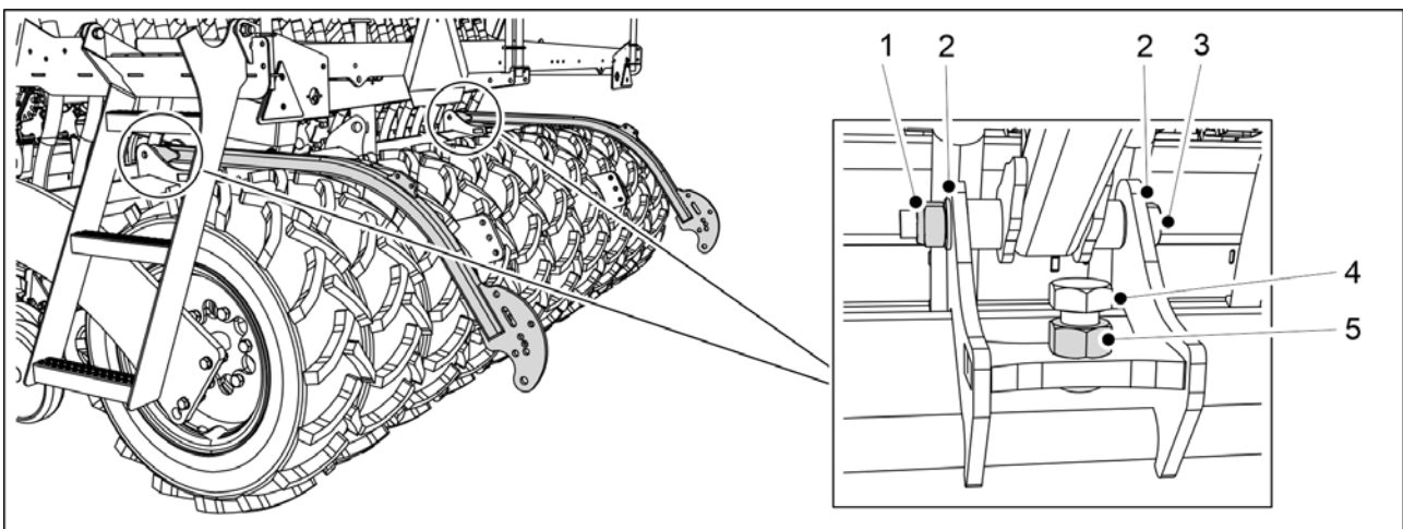
Kuva. 5.1.13 - 82. Jälkiharan varsien kiinnittäminen
