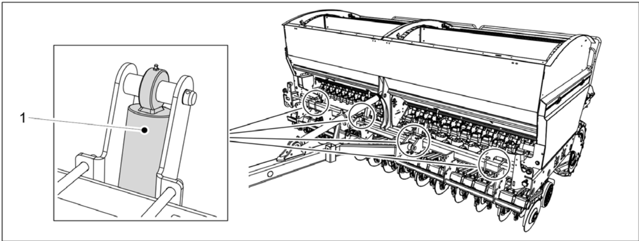
Kuva. 7.2.3 - 269. Vannaspainatussyinterien voitelu
