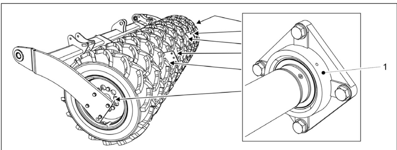
Kuva. 7.2.5 - 270. Pyöräakselien laakerit
