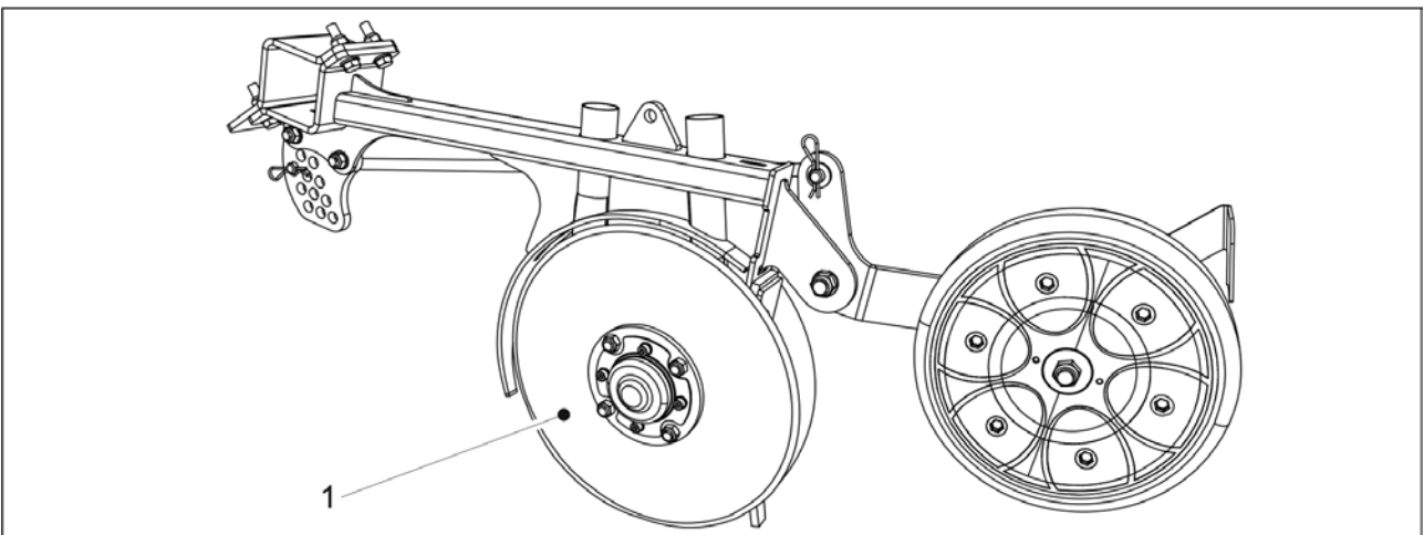
Kuva. 7.1.9 - 265. Vantaan kiekot
