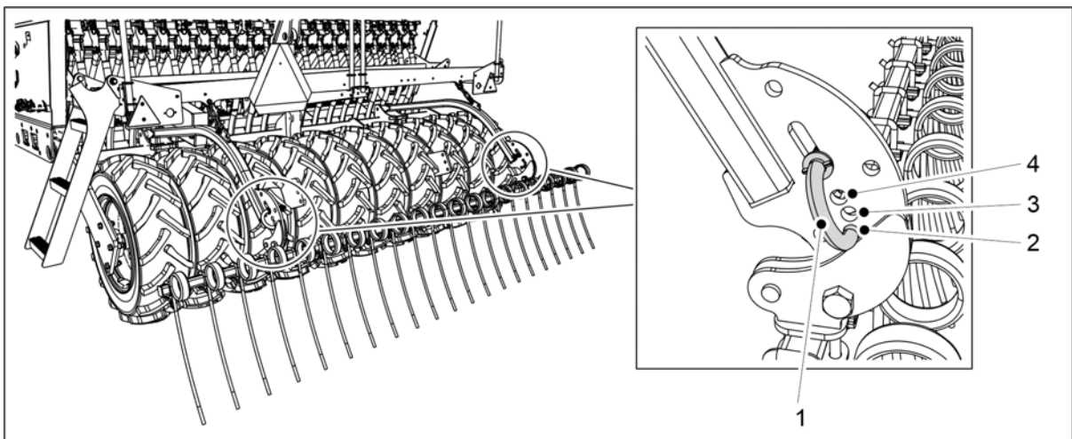
Kuva. 6.14 - 224. Jälkiharan kulman säätäminen
