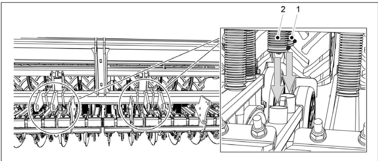
Kuva. 5.1.10 - 74. Siemen- ja lannoiteputken alaveto
