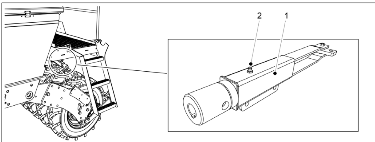
Kuva. 7.2.17 - 284. Seisontajarruveivi
