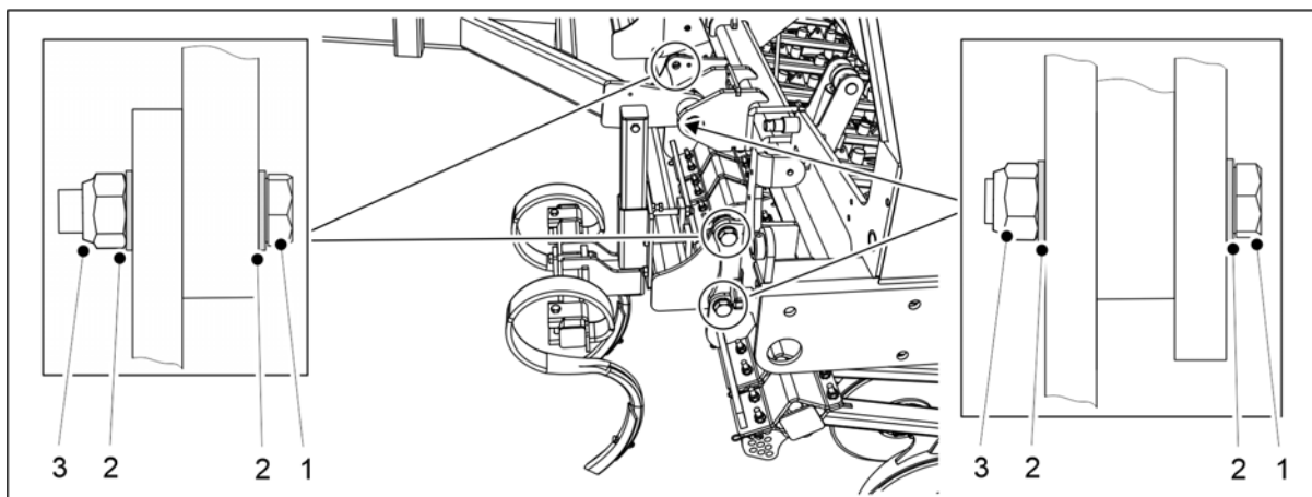
Kuva. 5.1.7 - 69. Ajourakuohkeuttimen kiinnittäminen
