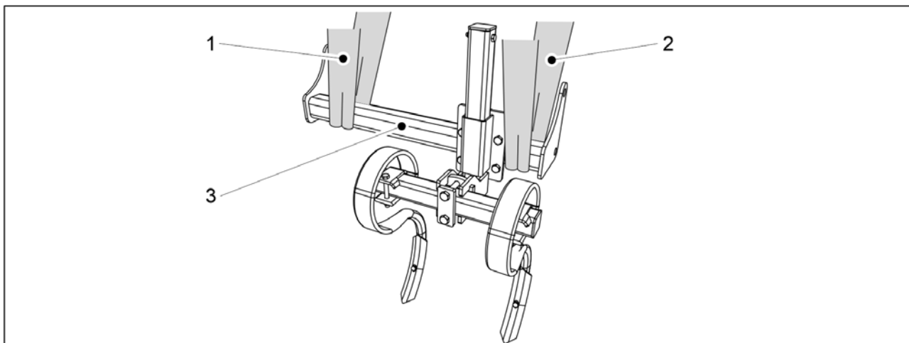
Kuva. 5.1.7 - 68. Ajourakuohkeuttimen nostaminen
