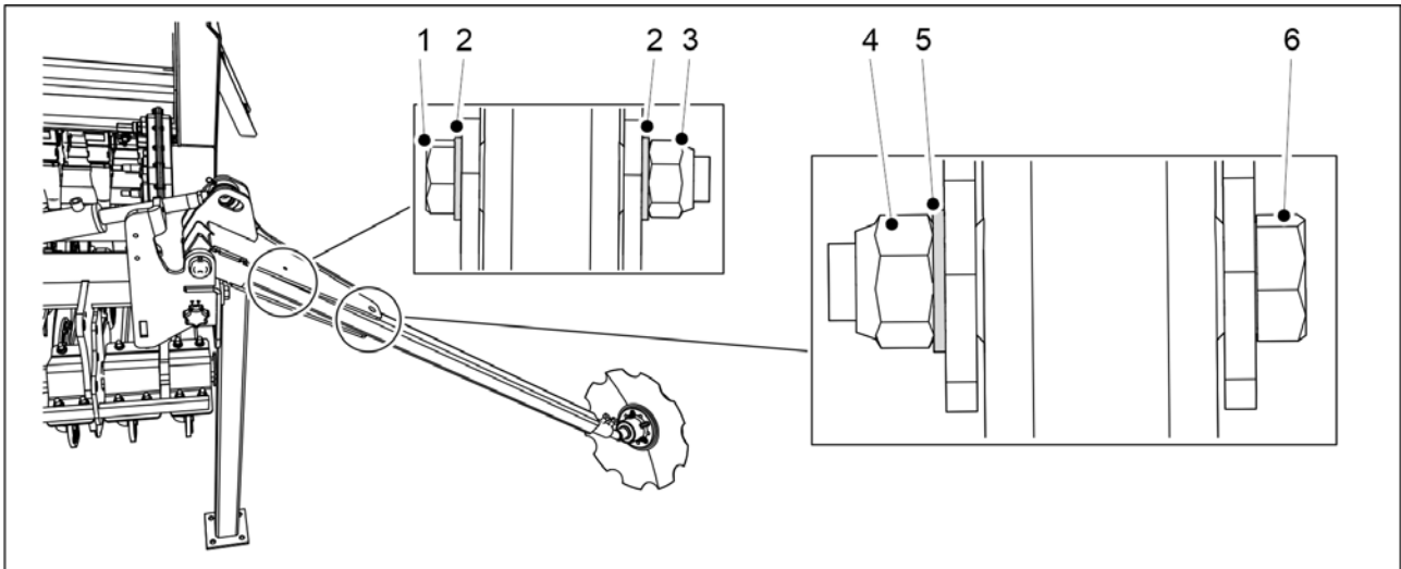
Kuva. 5.1.8 - 72. Keskimerkkarien kiinnittäminen
