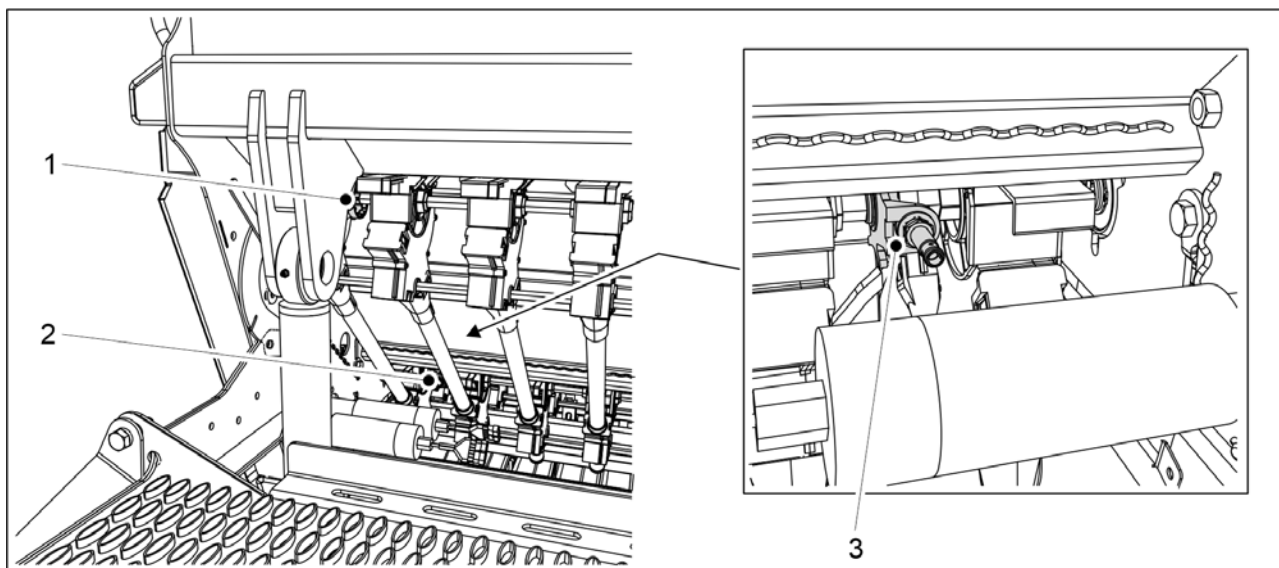
Kuva. 4.1.1.5 - 17. Pyörintävahtien sijainti
