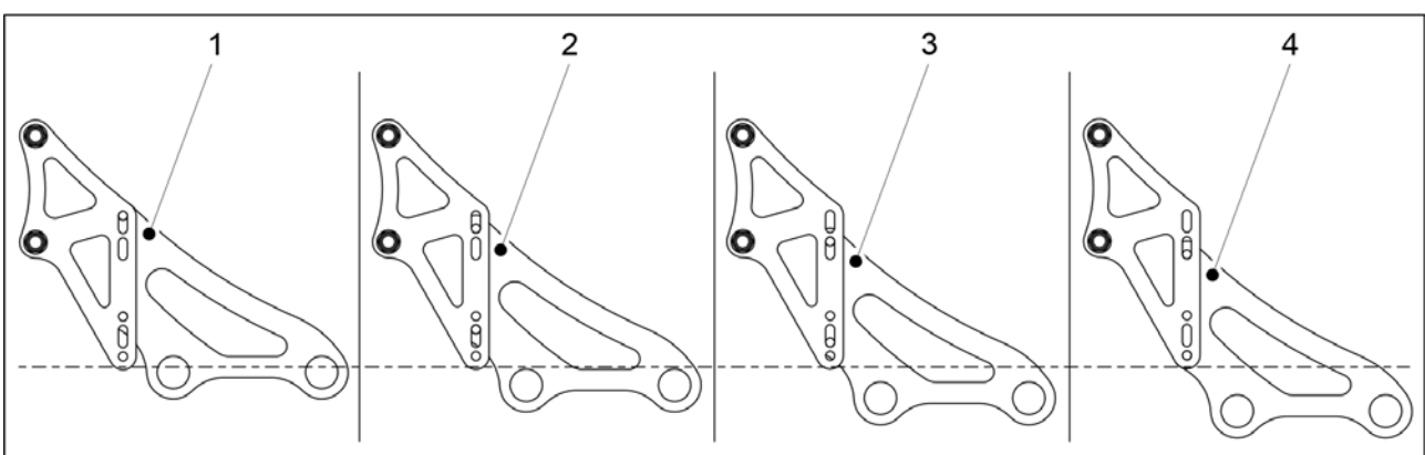
Kuva. 6.16 - 226. Etuharan korkeus - vaihtoehdot
