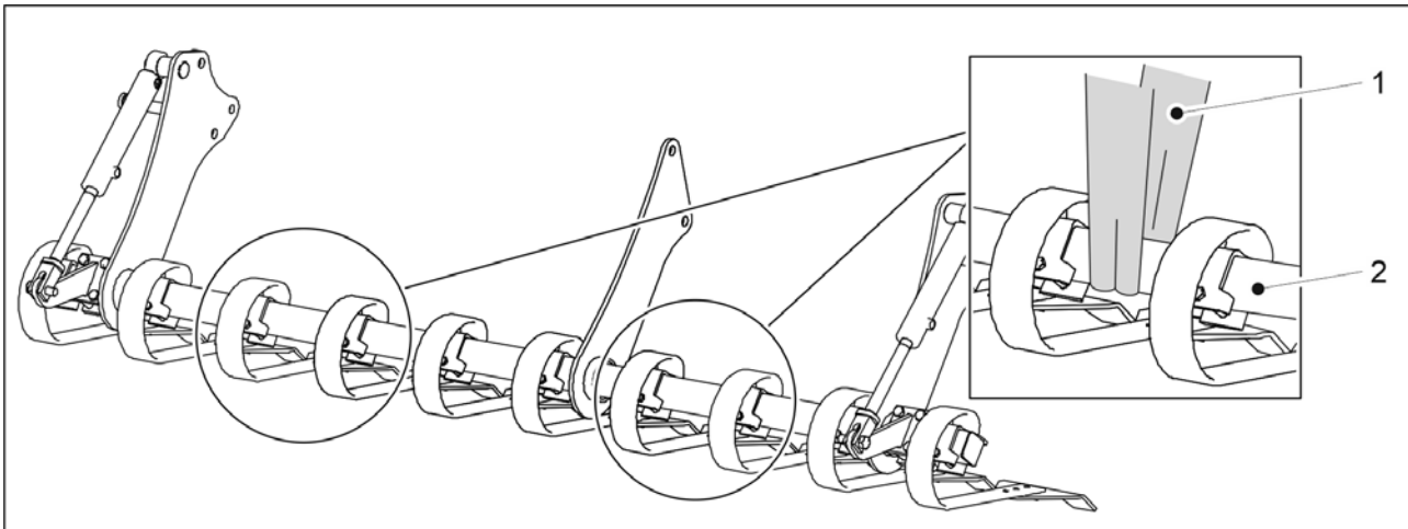
Kuva. 5.1.4 - 59. Etuladan nostaminen
