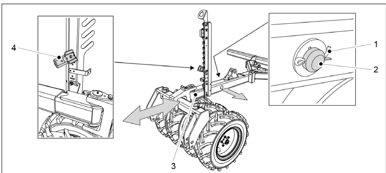
Kuva. 5.3.1 - 115. Aisan pituuden säätäminen
