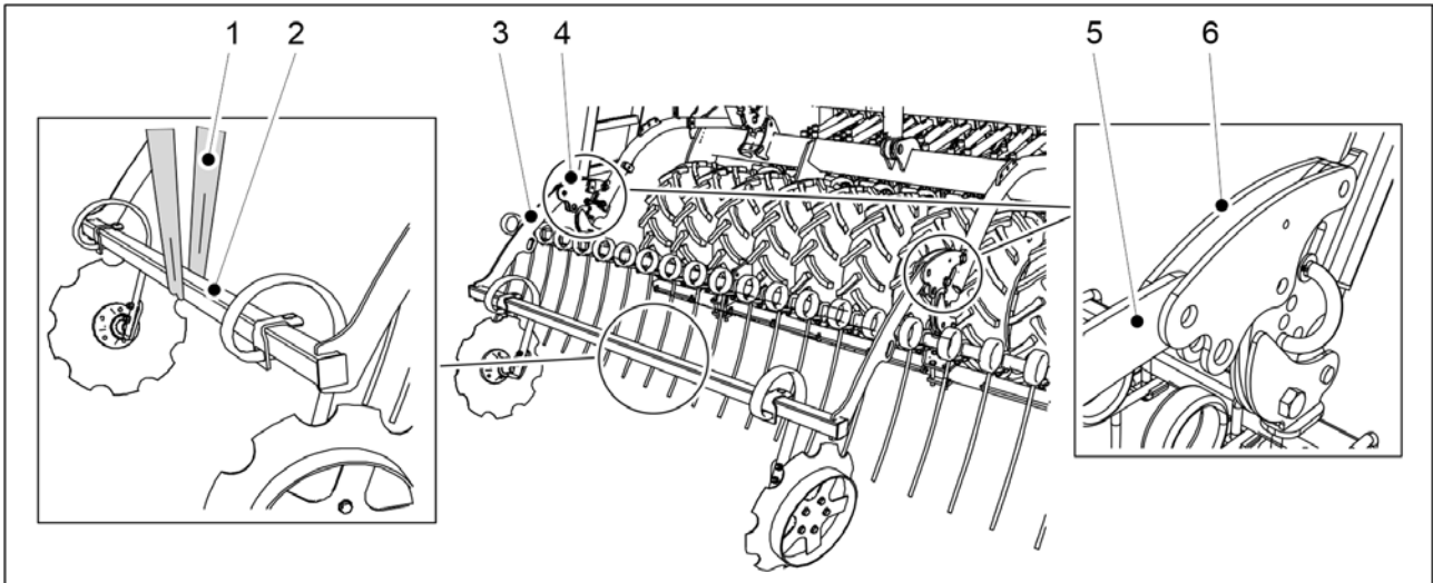
Kuva. 5.1.14 - 86. Takamerkkarien nostaminen
