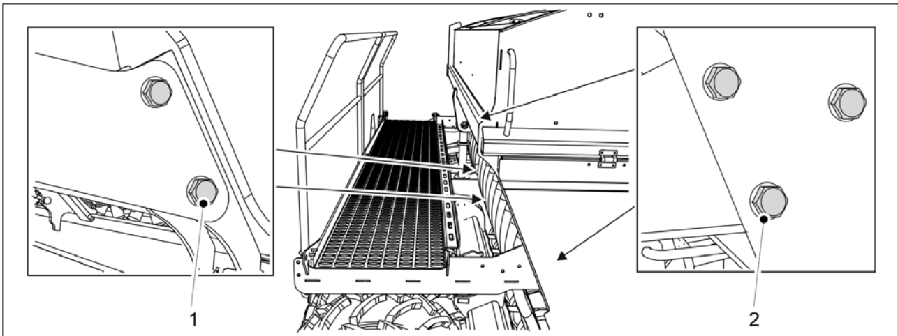
Kuva. 7.1.2.5 - 256. Hoitotason pultit
