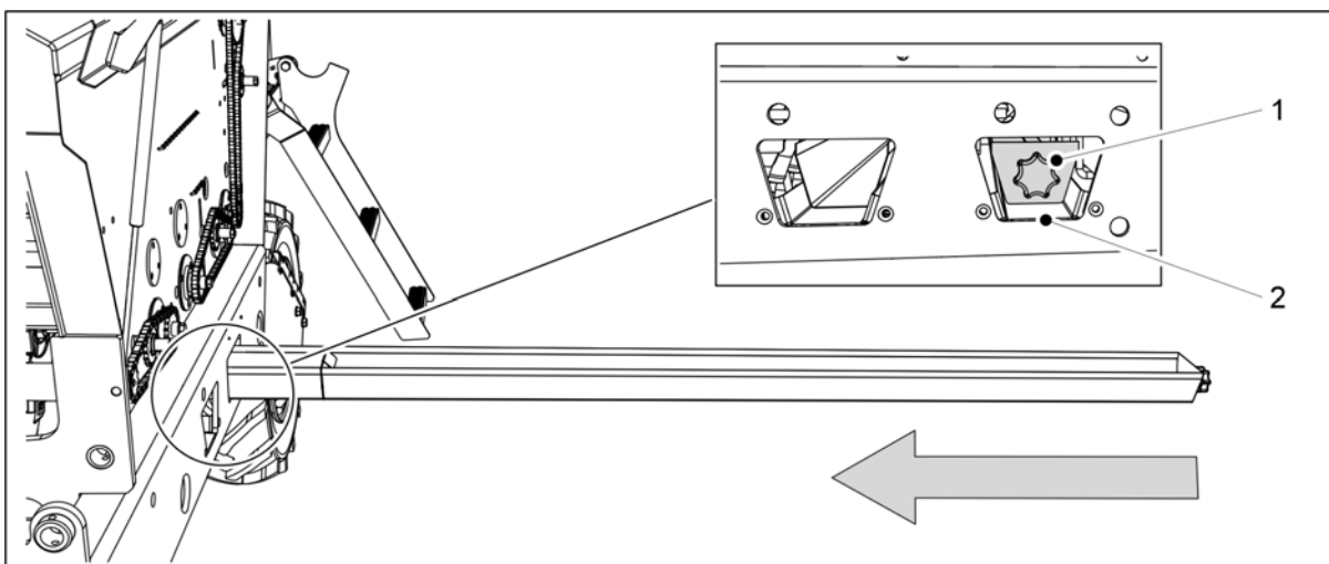
Kuva. 6.8.3 - 193. Kiertokokeakaukaloiden asettaminen
