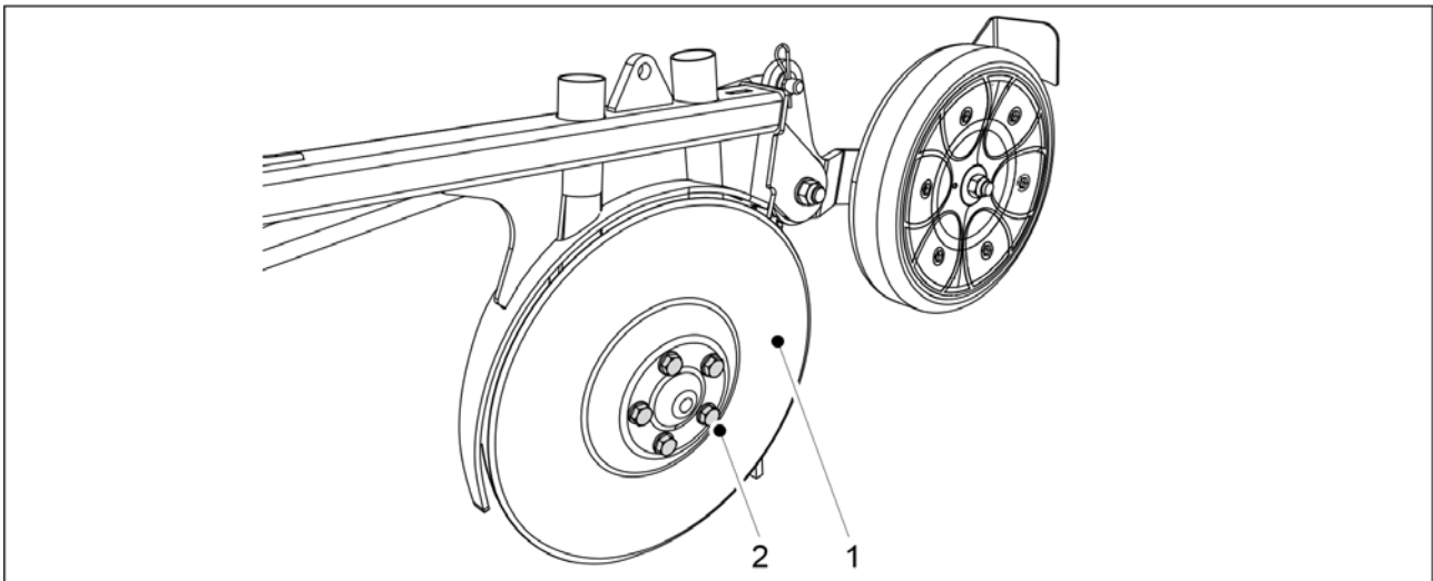
Kuva. 7.8.2.1 - 318. Kiekon irrotus
