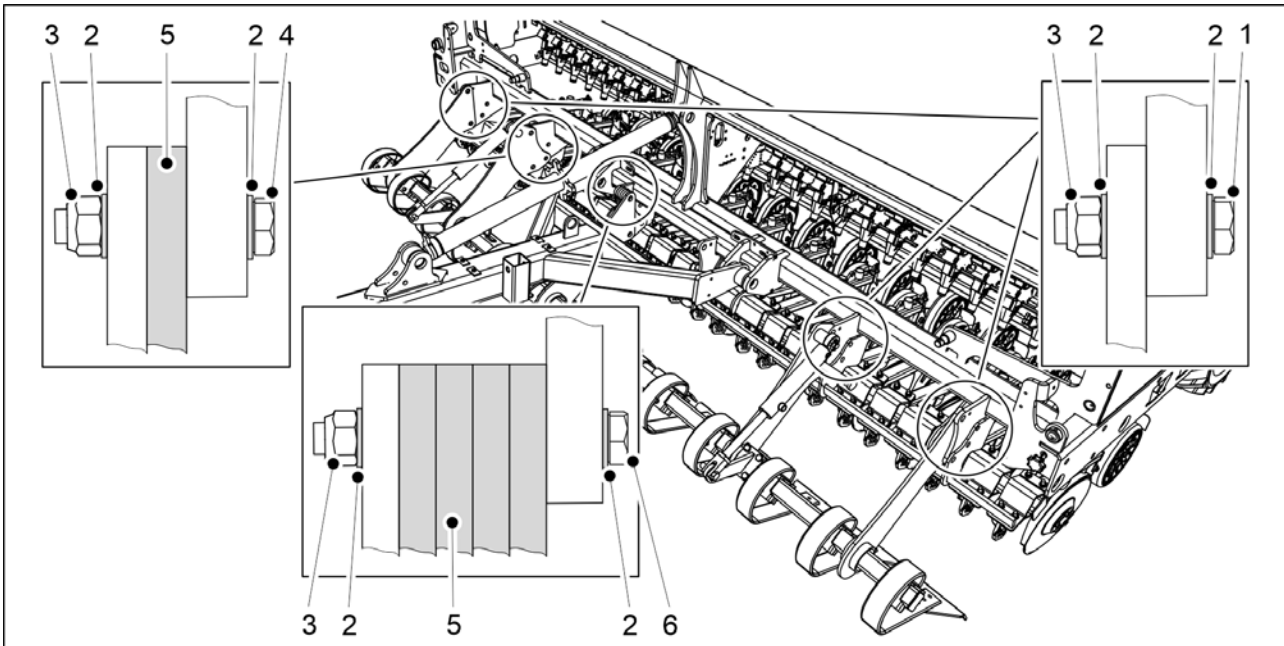
Kuva. 5.1.4 - 61. Etuladan kiinnittäminen eCEREX 400 -koneessa
