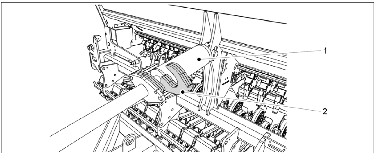
Kuva. 5.3.4 - 120. Sylinterin säätölamellit
