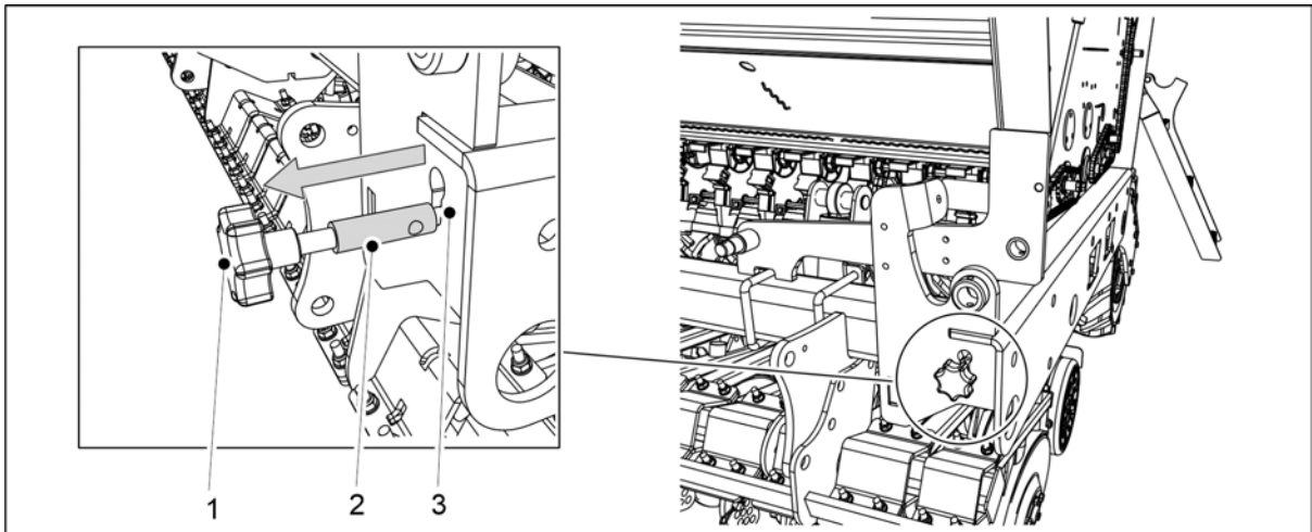
Kuva. 6.8.2 - 183. Kiertokokeen säätötangon ulosveto
