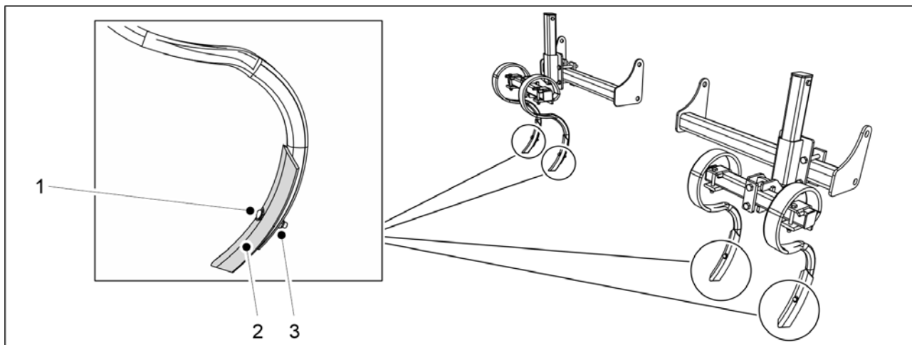
Kuva. 6.18.2 - 233. Joustopiikin kärkilapun vaihtaminen
