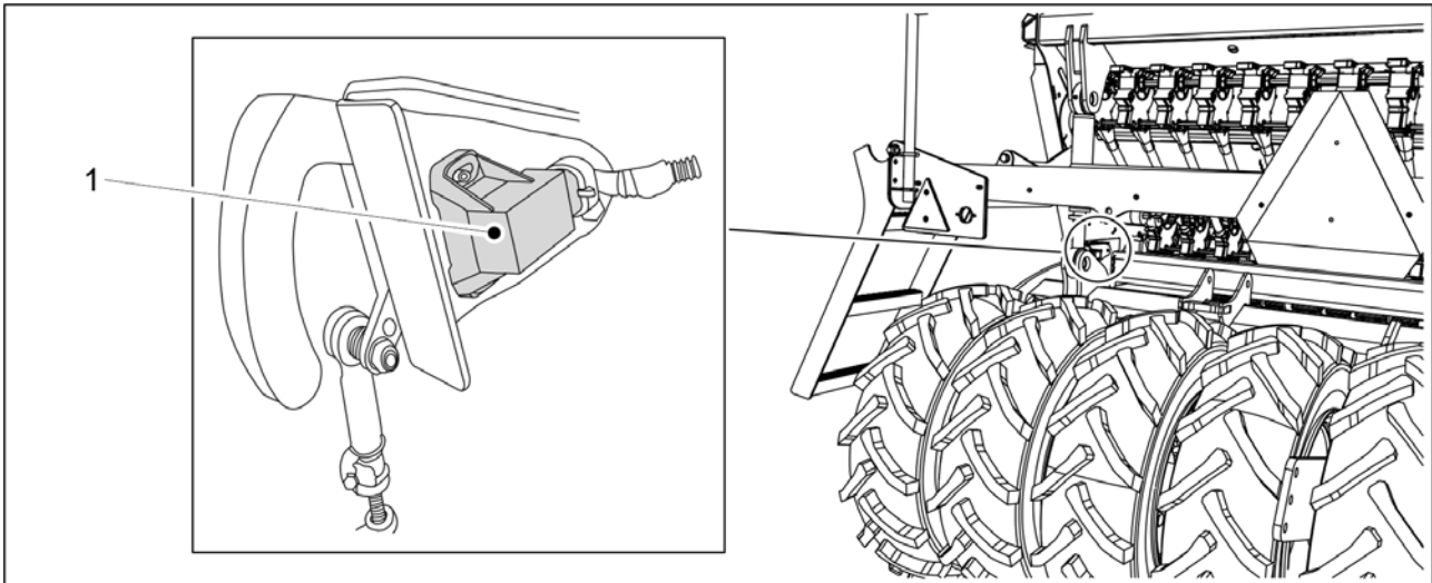
Kuva. 4.1.1.3 - 15. Kylvöasentoanturi
