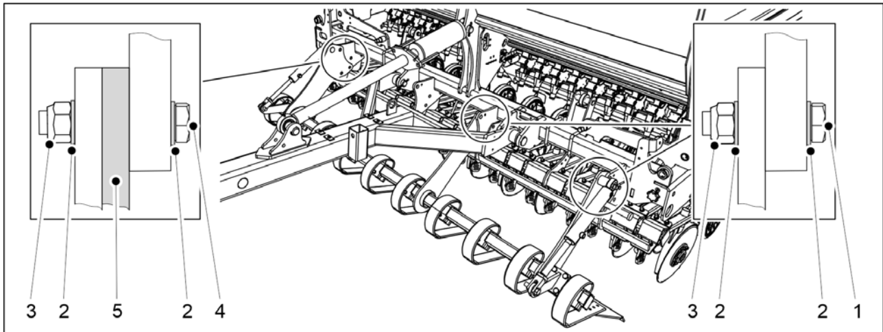
Kuva. 5.1.4 - 60. Etuladan kiinnittäminen eCEREX 300 -koneessa
