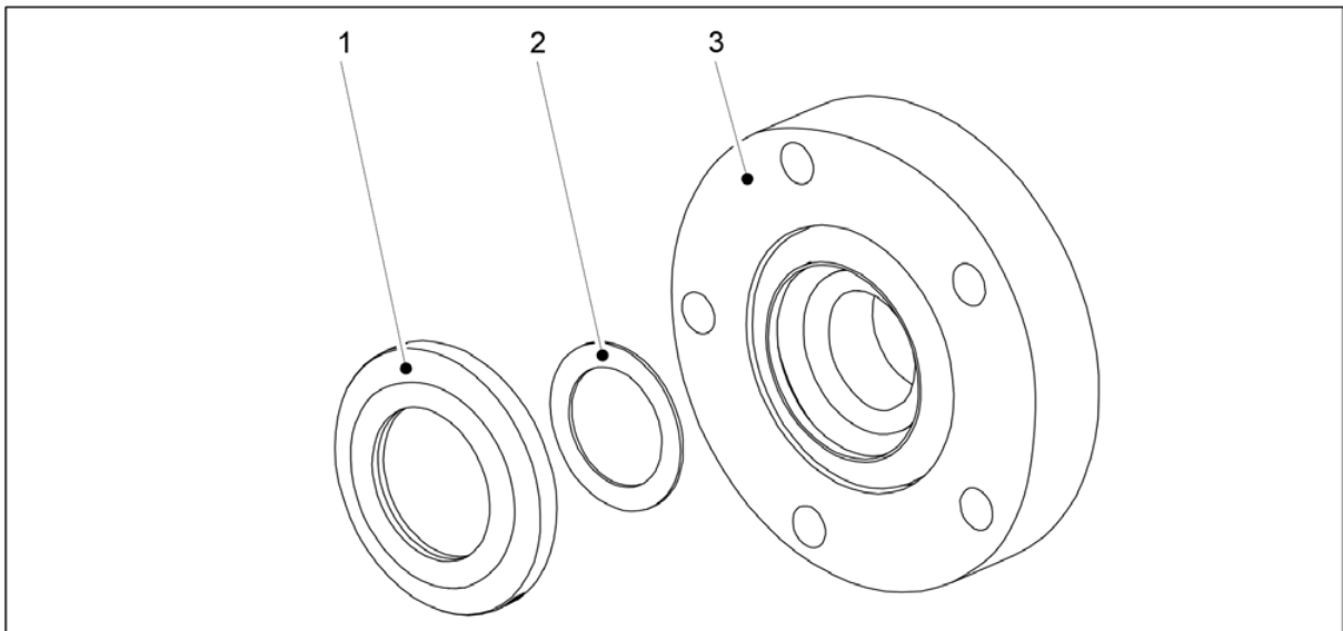
Kuva. 7.8.3.2 - 325. Laakerin tiiviste ja soviterengas
