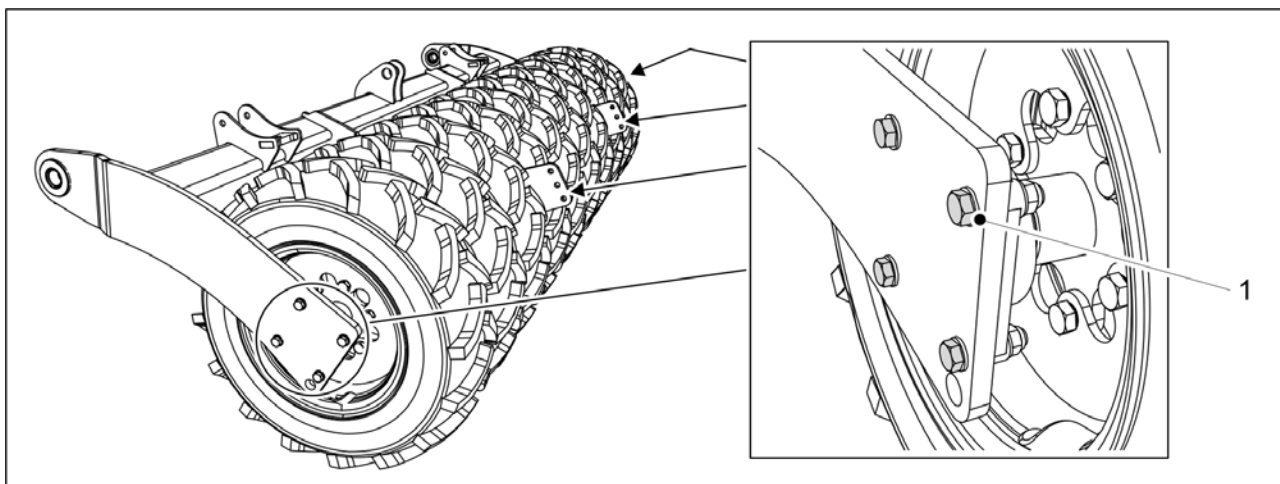
Kuva. 7.1.2.2 - 250. Kuljetuspyörien laippalaakereiden pultit
