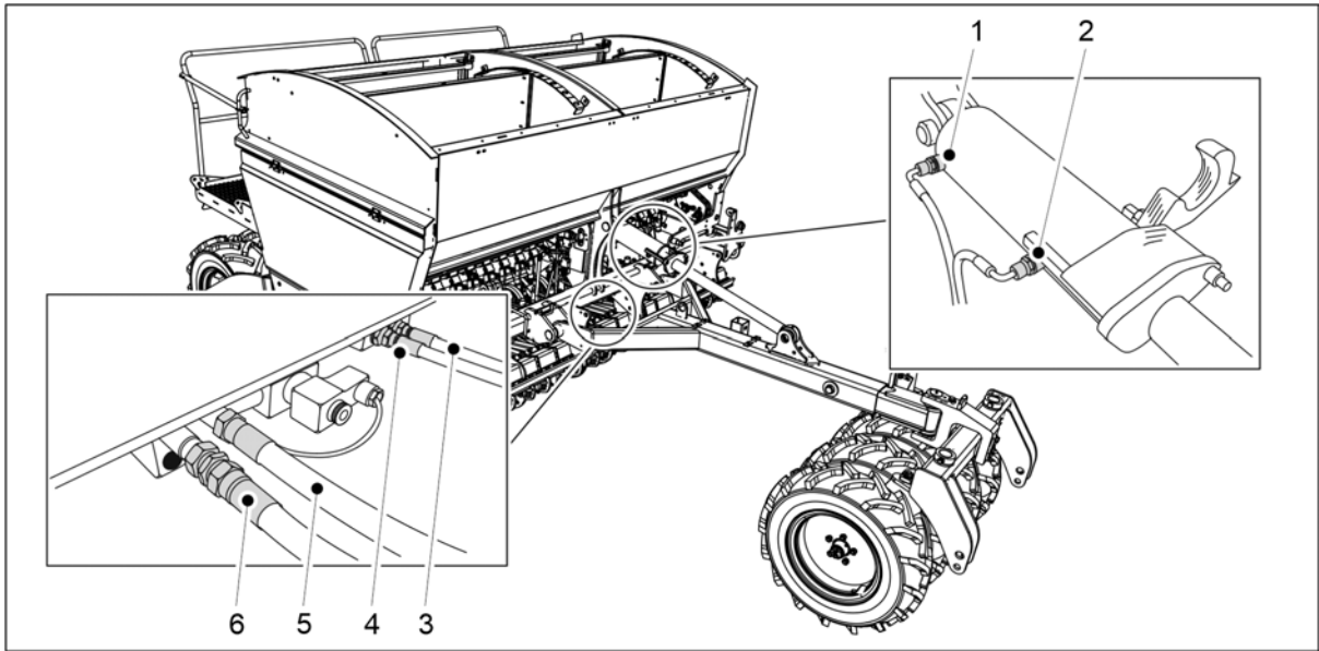
Kuva. 5.1.1 - 56. Hydrauliletkujen kytkentä
