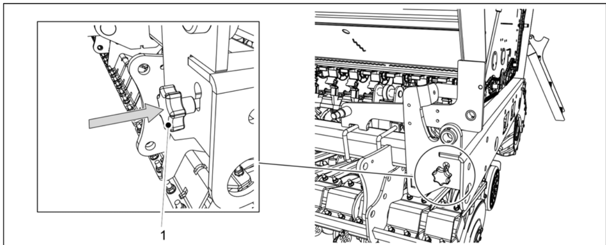
Kuva. 6.8.1 - 182. Kiertokokeen säätötangon sisääntyöntö
