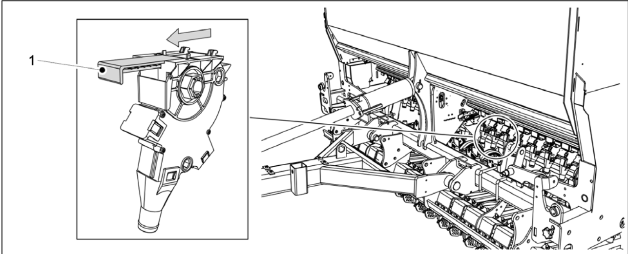
Kuva. 6.6.6.2 - 163. Sulkuluukku lannoitteen syöttöyksikössä
