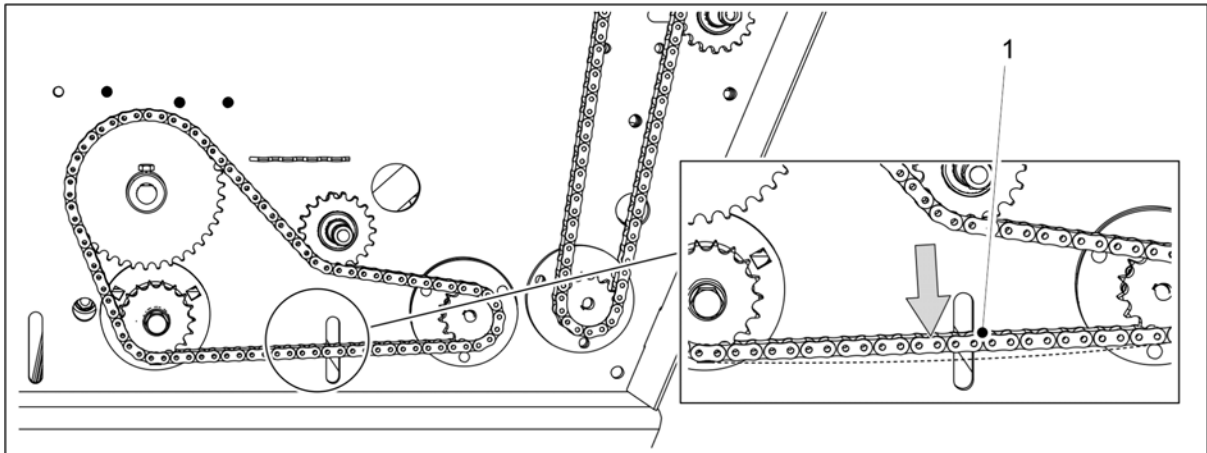
Kuva. 7.1.5.4 - 263. Ketjujen kireyden tarkastus, siemenen karistaja-akselin voimansiirto
