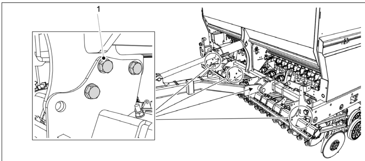
Kuva. 7.1.2.4 - 253. Vannasvarren pultit
