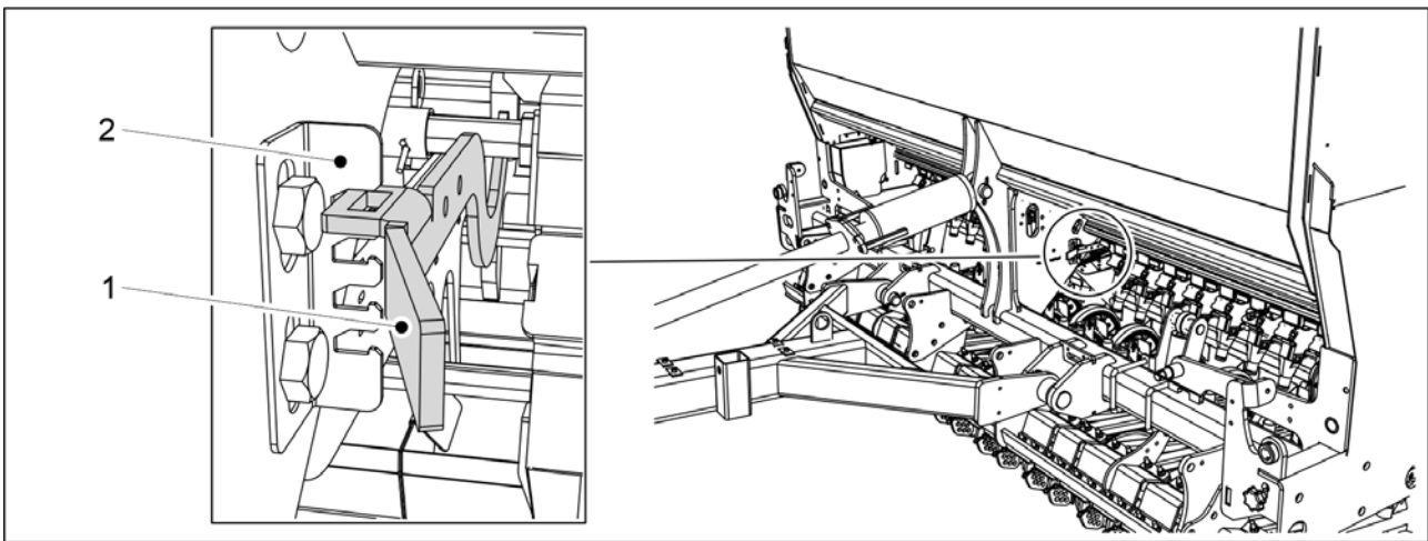
Kuva. 6.6.6.1 - 161. Syöttöyksiköiden pohjaläppien säätövipu, lannoitesäiliö
