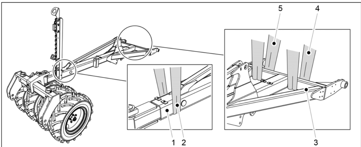
Kuva. 5.1.6 - 64. Vetopuomi ja pyöränvälilyrä
