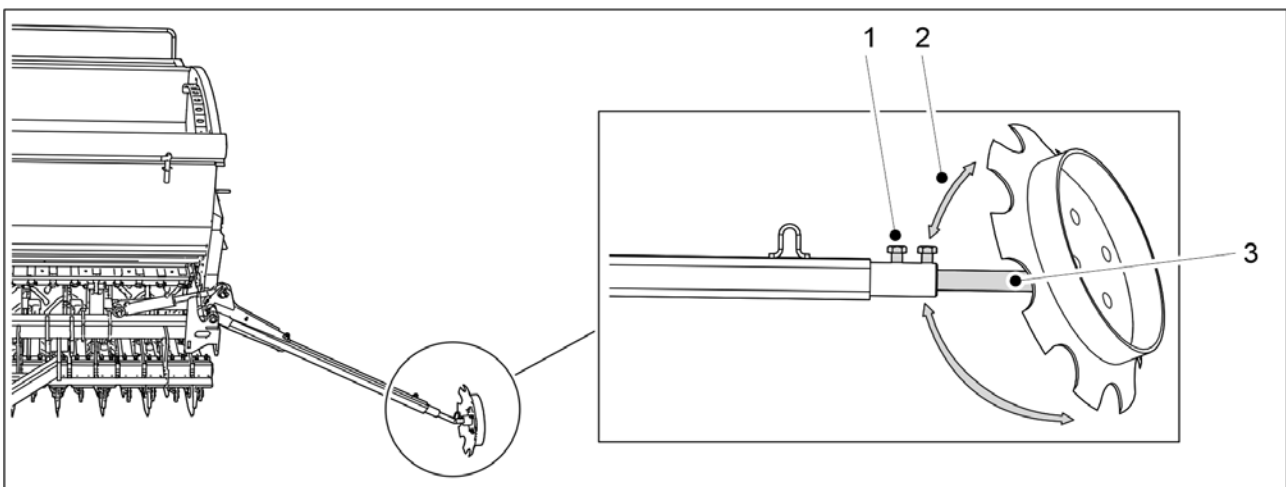
Kuva. 5.3.7 - 123. Keskimerkkarien säätäminen
