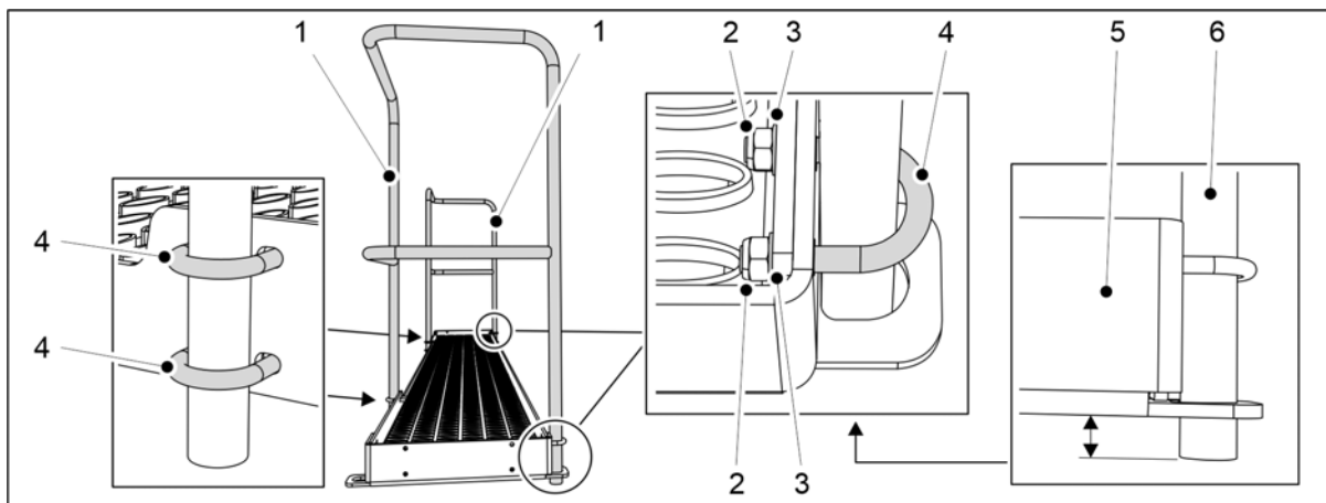
Kuva. 5.1.16 - 101. Kaiteiden kiinnittäminen 400-koneessa
