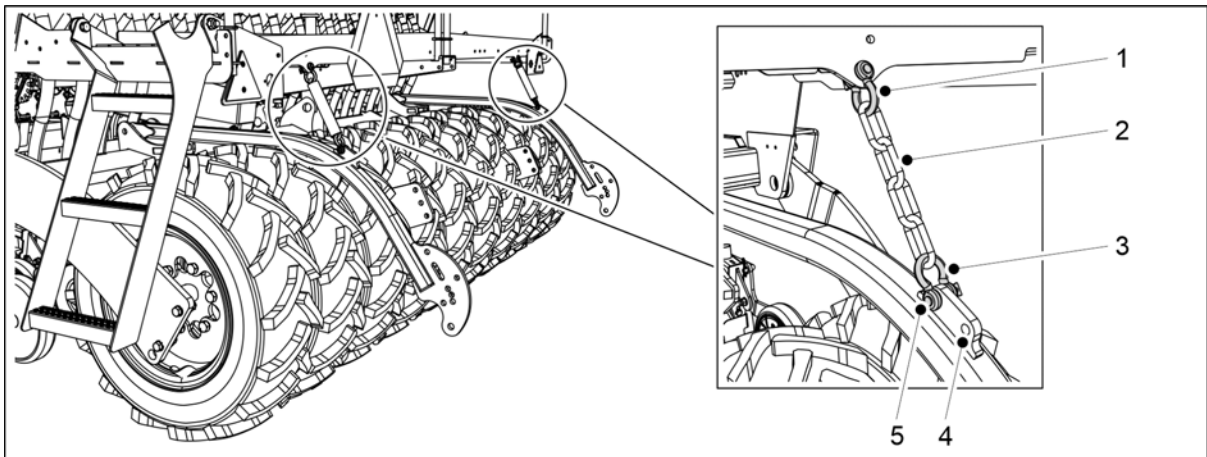
Kuva. 5.1.13 - 83. Jälkiharan ketjujen kiinnittäminen
