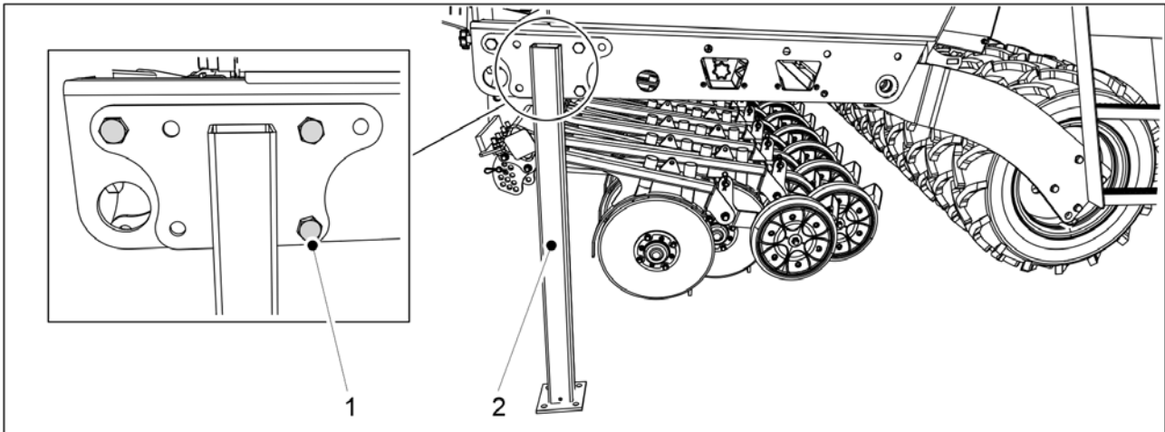
Kuva. 5.1.9 - 73. Kuljetustuki
