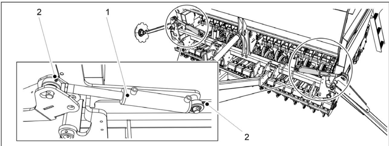
Kuva. 7.2.8 - 273. Keskimerkkarisylinterit
