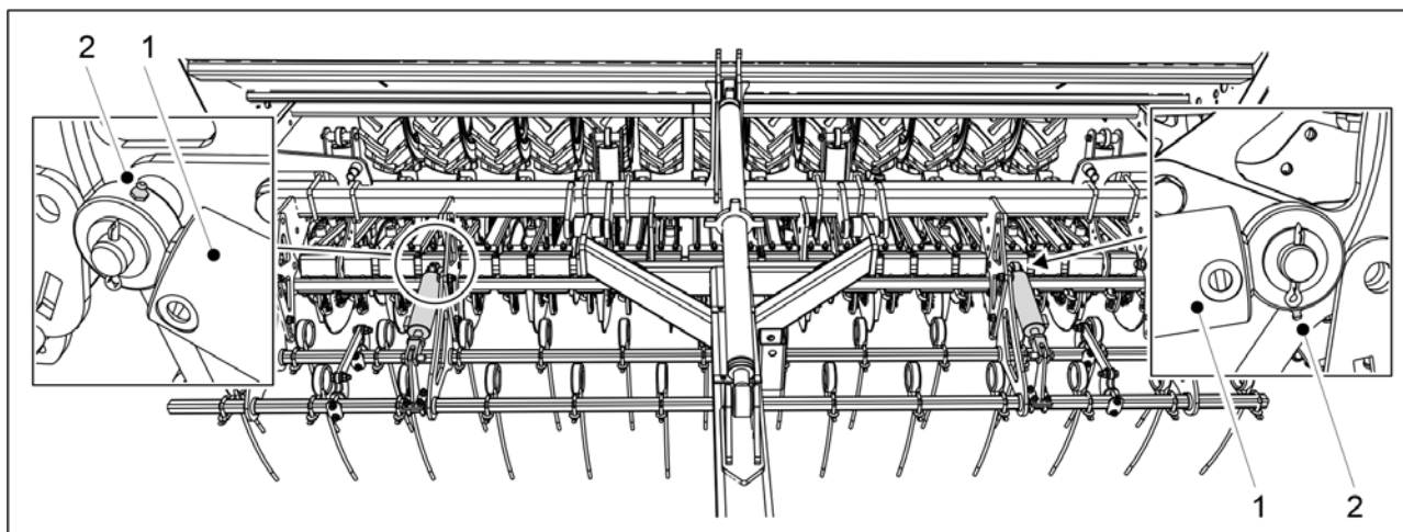
Kuva. 7.2.12 - 279. Etuharan sylinterit
