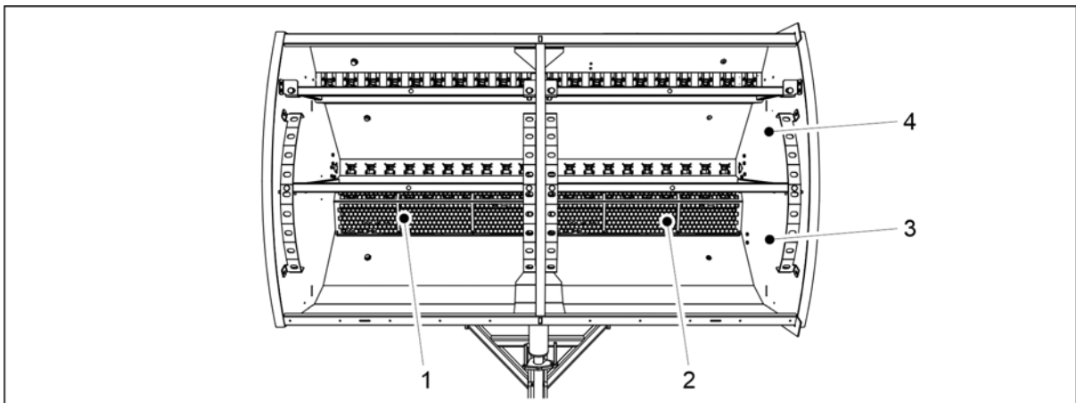
Kuva. 7.3.1 - 286. Säiliöiden puhdistus
