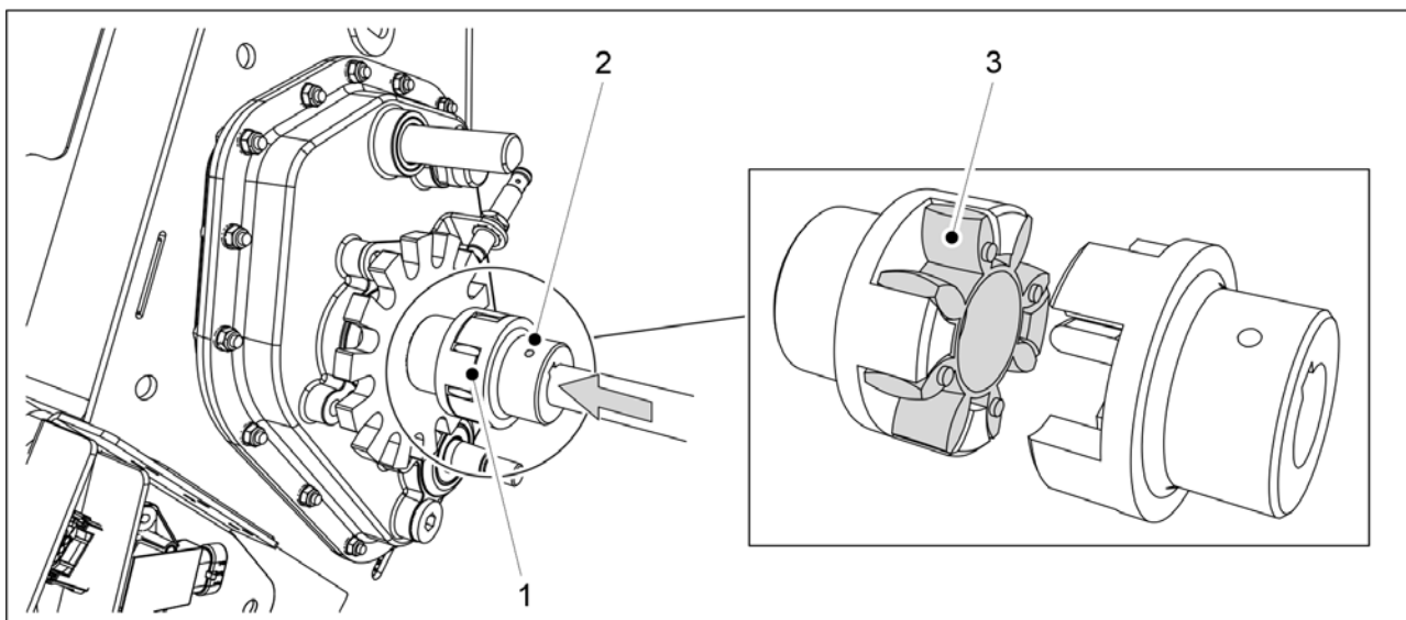
Obrázek. 7.7.2.2 - 350. Montáž spojky
