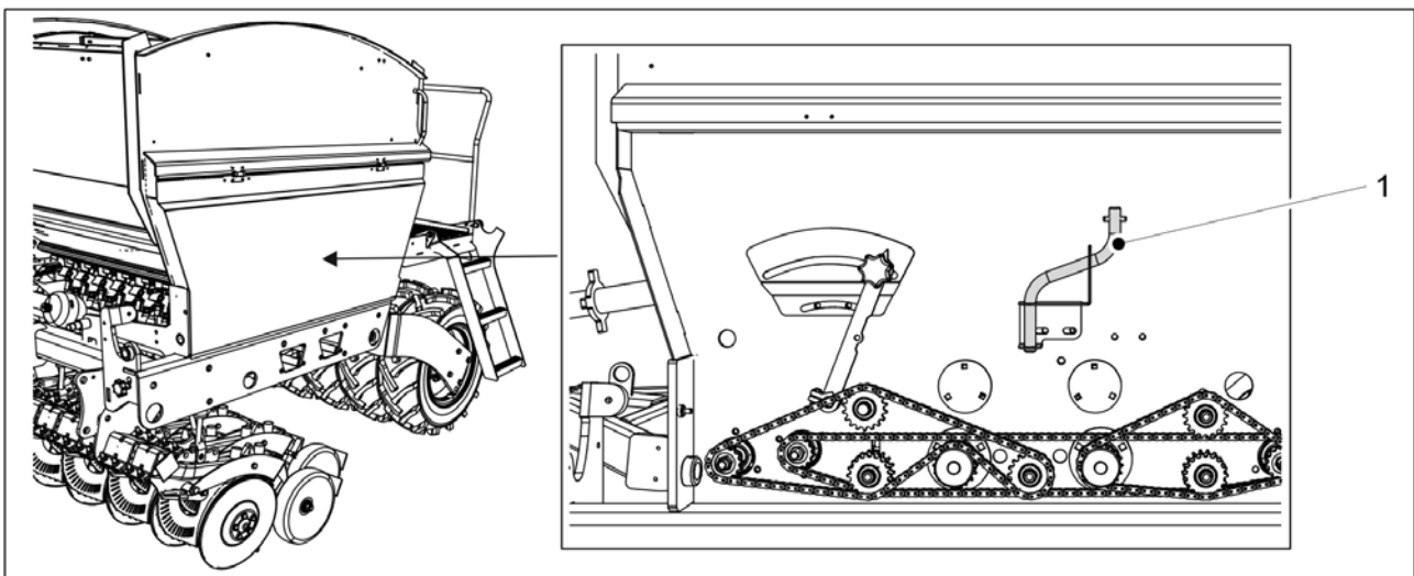
Obrázek. 6.8 - 185. Umístění kliky na kalibrační zkoušku
