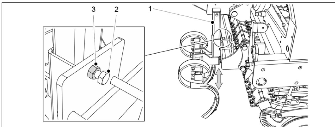
Obrázek. 6.15.1 - 256. Regulace výšky odstraňovače dráhy
