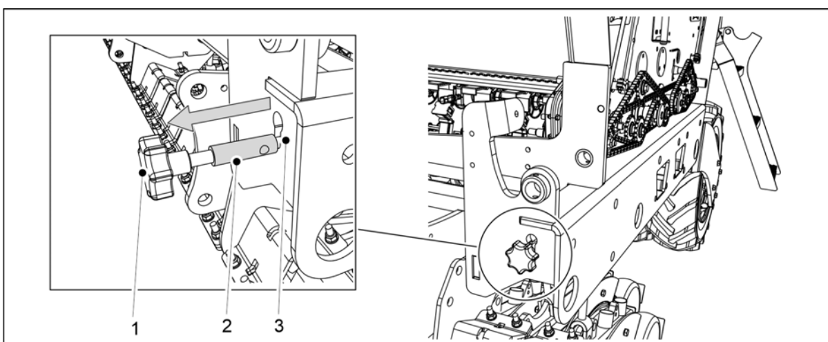
Obrázek. 6.8.4 - 211. Vytáhněte regulační tyč kalibrační zkoušky.
