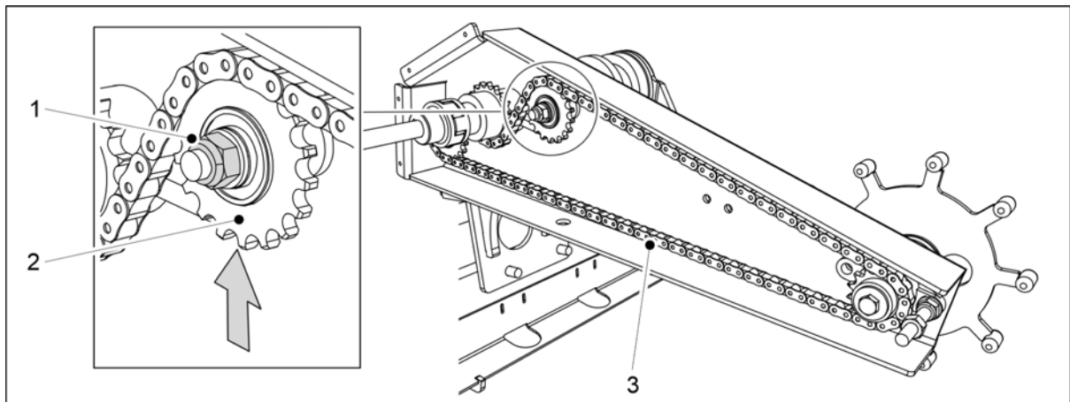
Obrázek. 7.7.1 - 348. Dotahování řetězu pohonu kola
