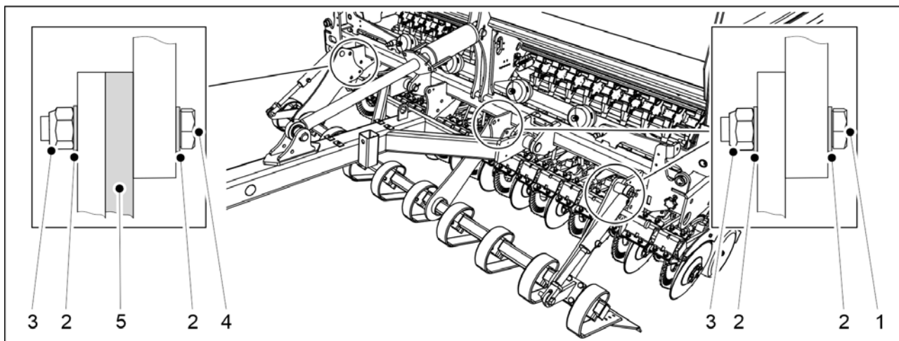
Obrázek. 5.1.4 - 68. Montáž přední nivelační desky na model FORTE 300 EVO
