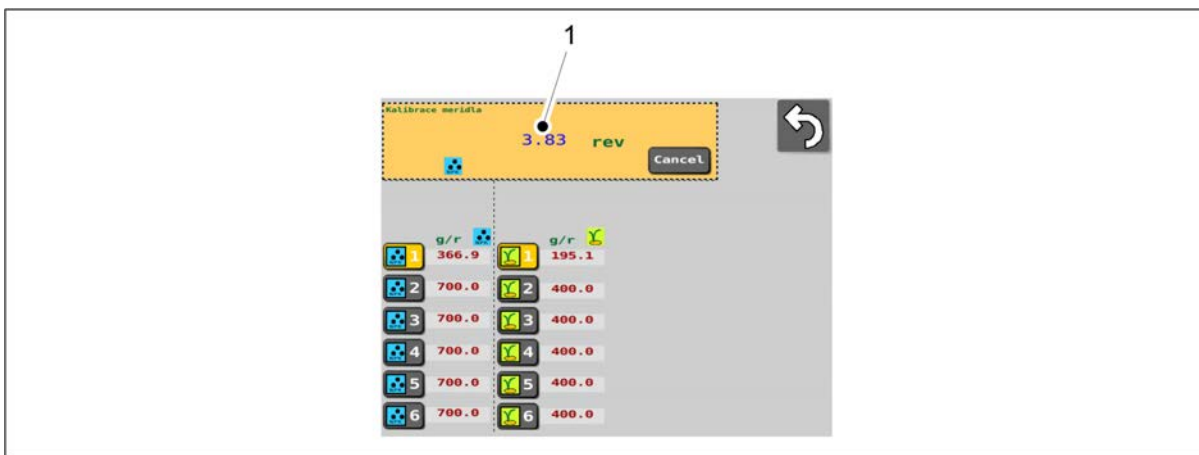
Obrázek. 6.8.4 - 220. Otáčky hřídele podavače provedené klikou kalibrační zkoušky
