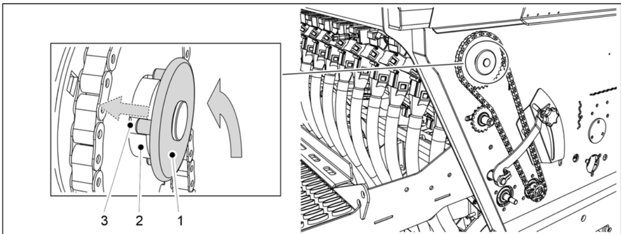
Obrázek. 6.8.2 - 200. Návrat podavače malého osiva do provozní polohy
