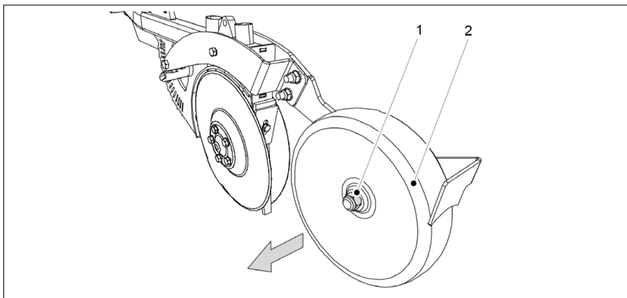
Obrázek. 7.9.4.1 - 367. Demontáž uzavíracího kola
