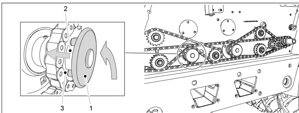
Obrázek. 6.8.2 - 199. Návrat podavače hnojiva do provozní polohy
