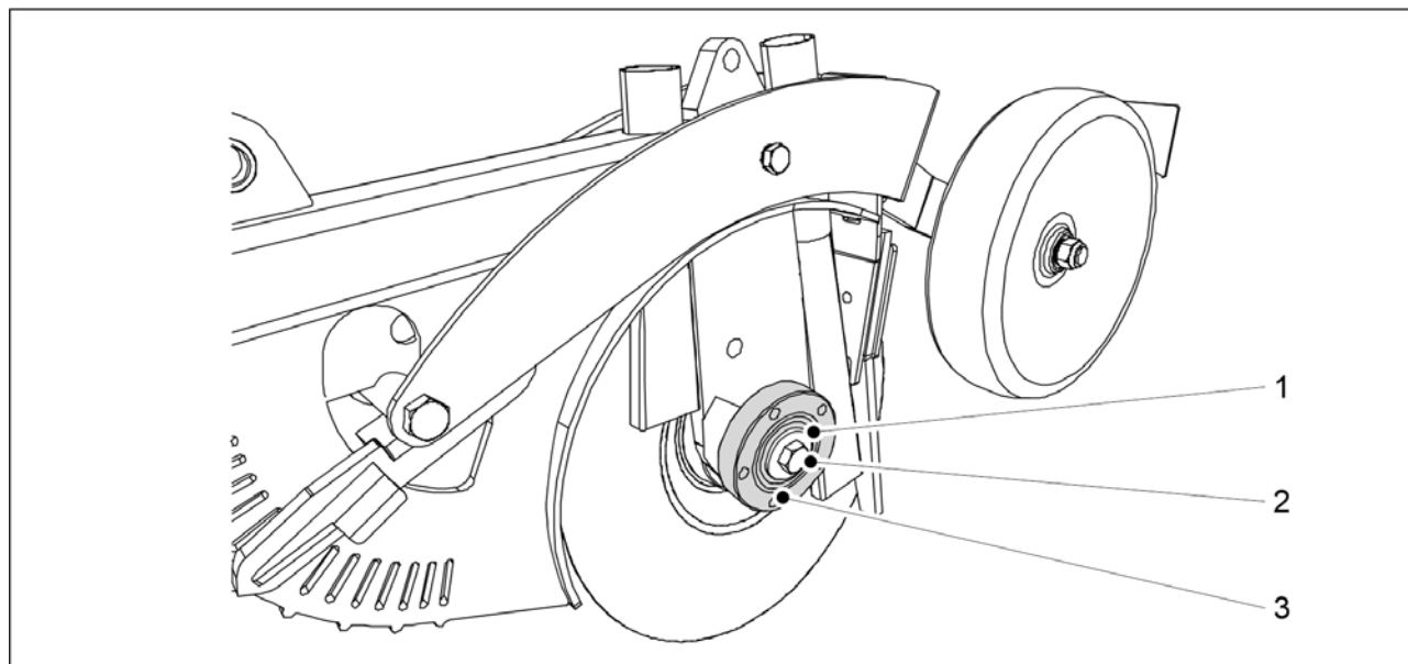
Obrázek. 7.9.2.2 - 361. Montáž pouzdra ložiska
