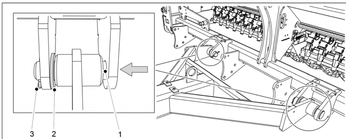
Obrázek. 5.1.1 - 62. Montáž kolového pěchu
