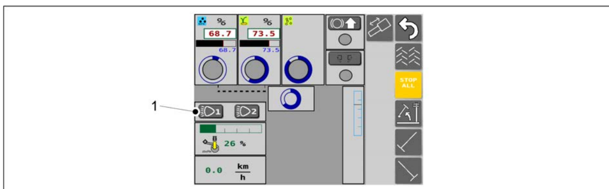
Obrázek. 6.3.12 - 160. Obrazovka Manuálního režimu
