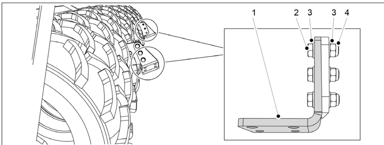
Obrázek. 5.1.11 - 85. Montáž závěsných desek stěrky
