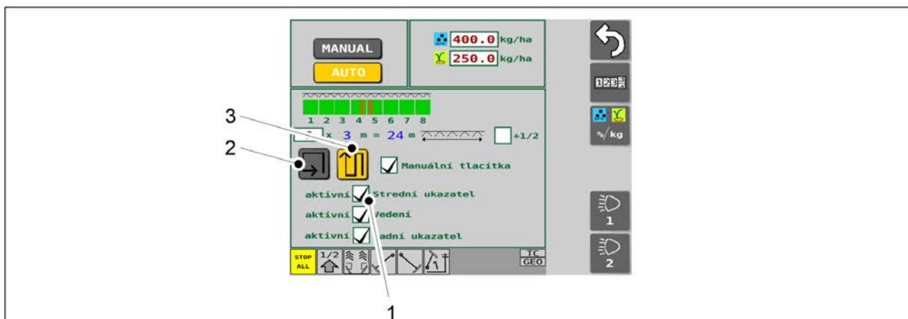
Obrázek. 6.3.6 - 149. Volba středních značkovačů a režimu jízdy
