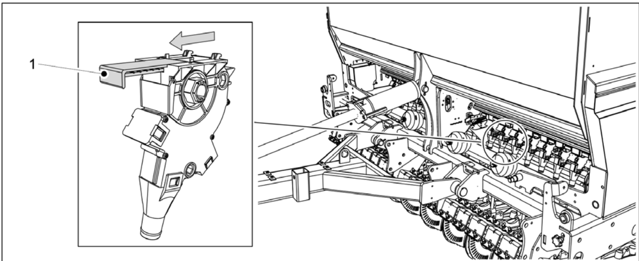
Obrázek. 6.6.7.2 - 173. Uzavírací deska podávací jednotky hnojiva
