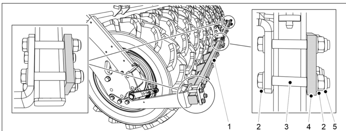
Obrázek. 5.1.12 - 90. Montáž stěrky
