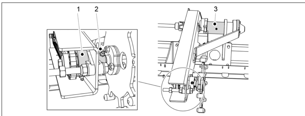
Obrázek. 7.2.3.2 - 300. Mazání ložisek nápravy kol
