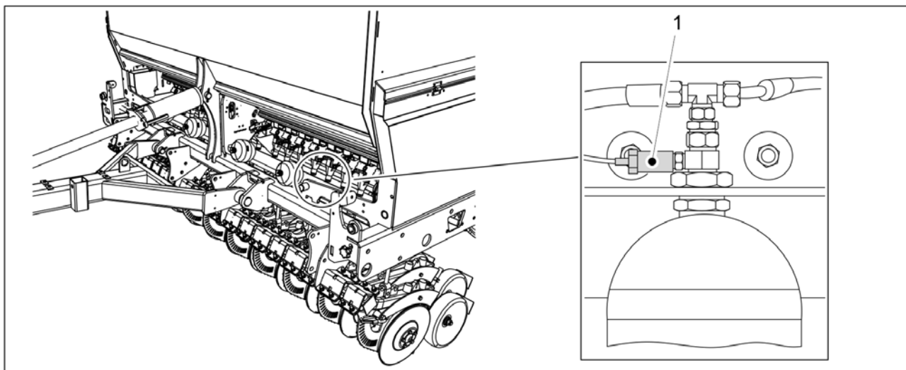
Obrázek. 4.1.1.10 - 28. Snímač tlaku radličky
