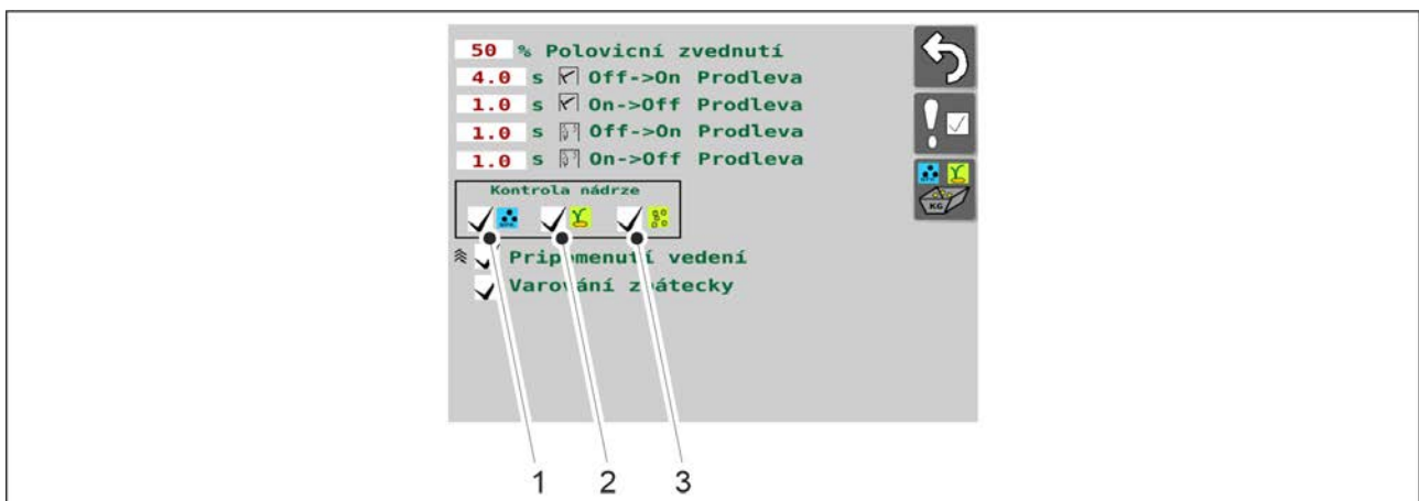
Obrázek. 6.3.9 - 154. Volba snímačů hladiny v násypce
