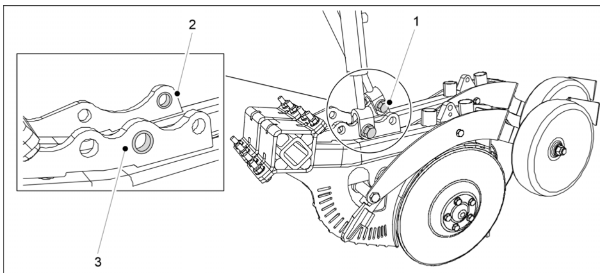
Obrázek. 7.9.1.2 - 357. Montáž válce radličky
