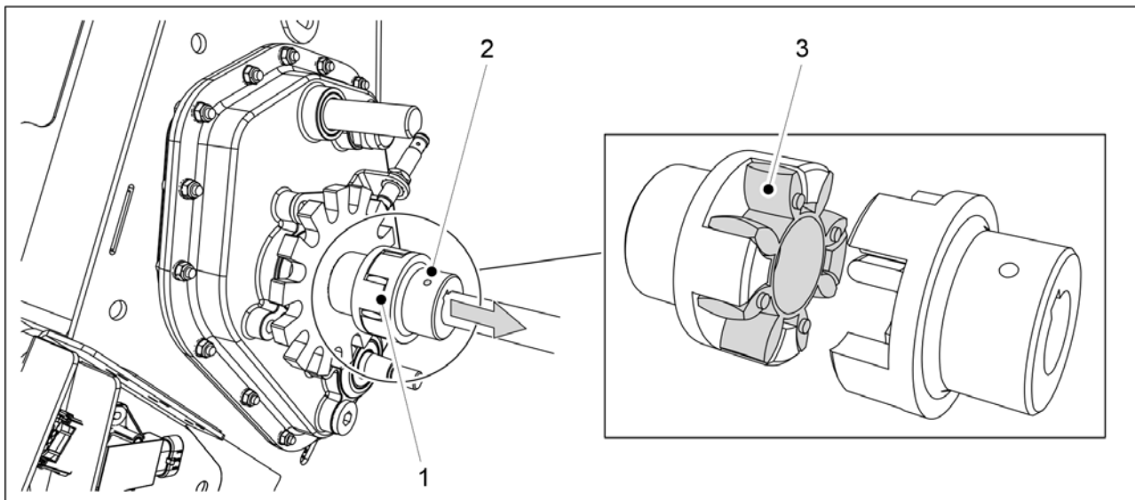
Obrázek. 7.7.2.1 - 349. Demontáž pružného spojovacího prvku spojky
