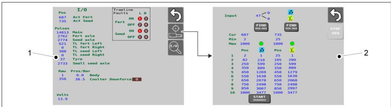
Obrázek. 7.10.3 - 376. Diagnostická data z kalibrace vstupů a výstupů a data lineárního ovladače.
