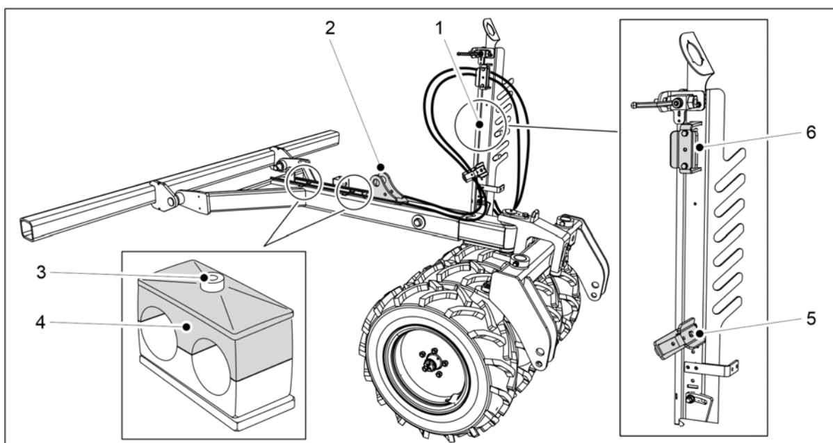
Obrázek. 5.1.1 - 63. Hydraulické hadice a elektrické vedení
