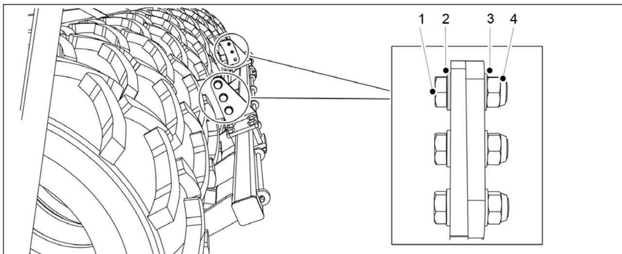
Obrázek. 7.4.1 - 324. Demontáž stěrky
