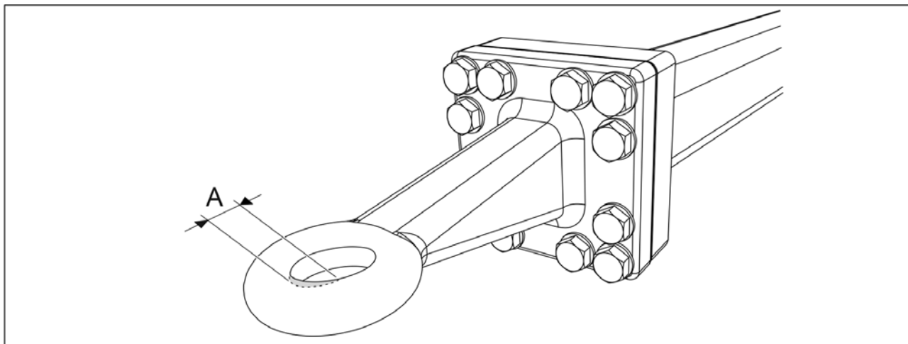
Obrázek. 7.1.11 - 289. Opotřebení tažného oka
