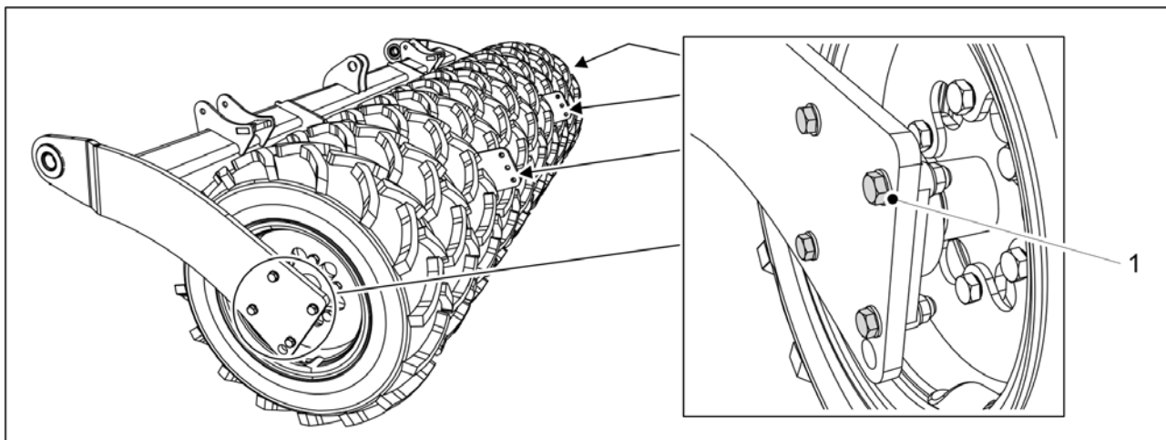
Obrázek. 7.4.4 - 336. Montáž sestavy kola
