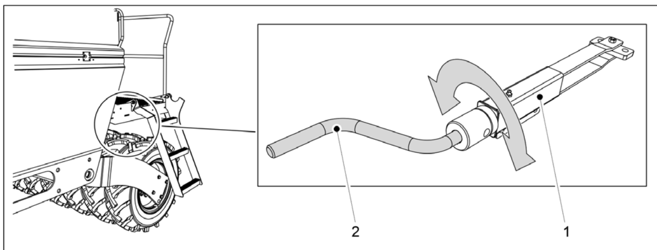
Obrázek. 6.19.1 - 261. Parkovací brzda
