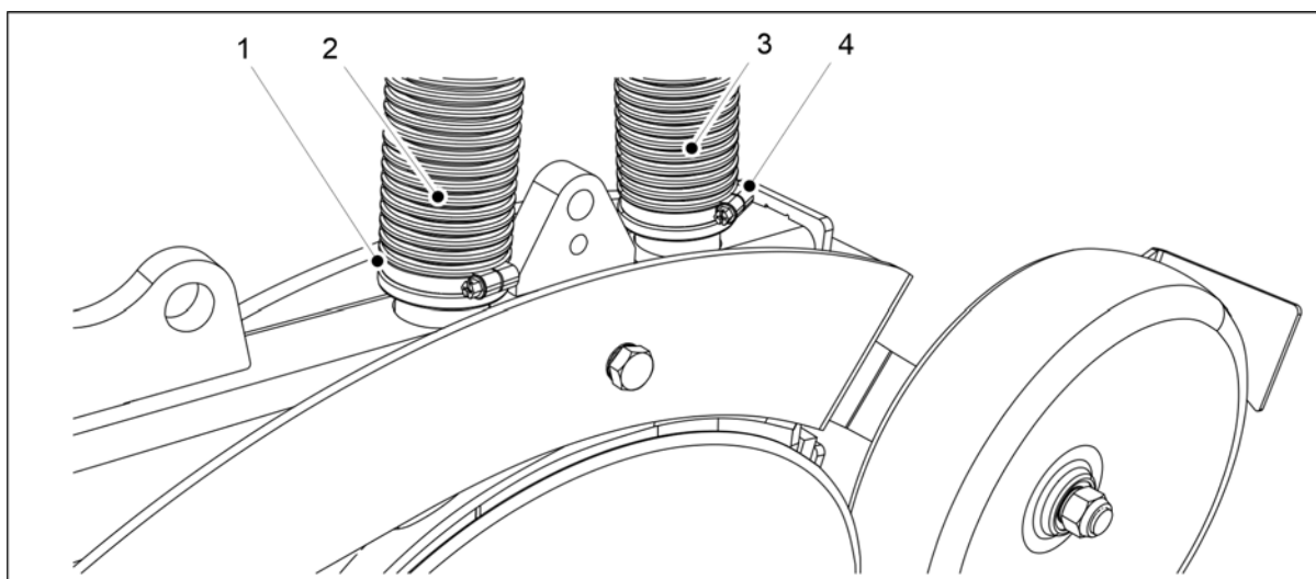
Obrázek. 7.9.1.2 - 358. Připojení hadic radličky
