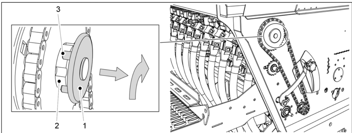
Obrázek. 6.8.2 - 197. Deaktivace malého podavače osiva
