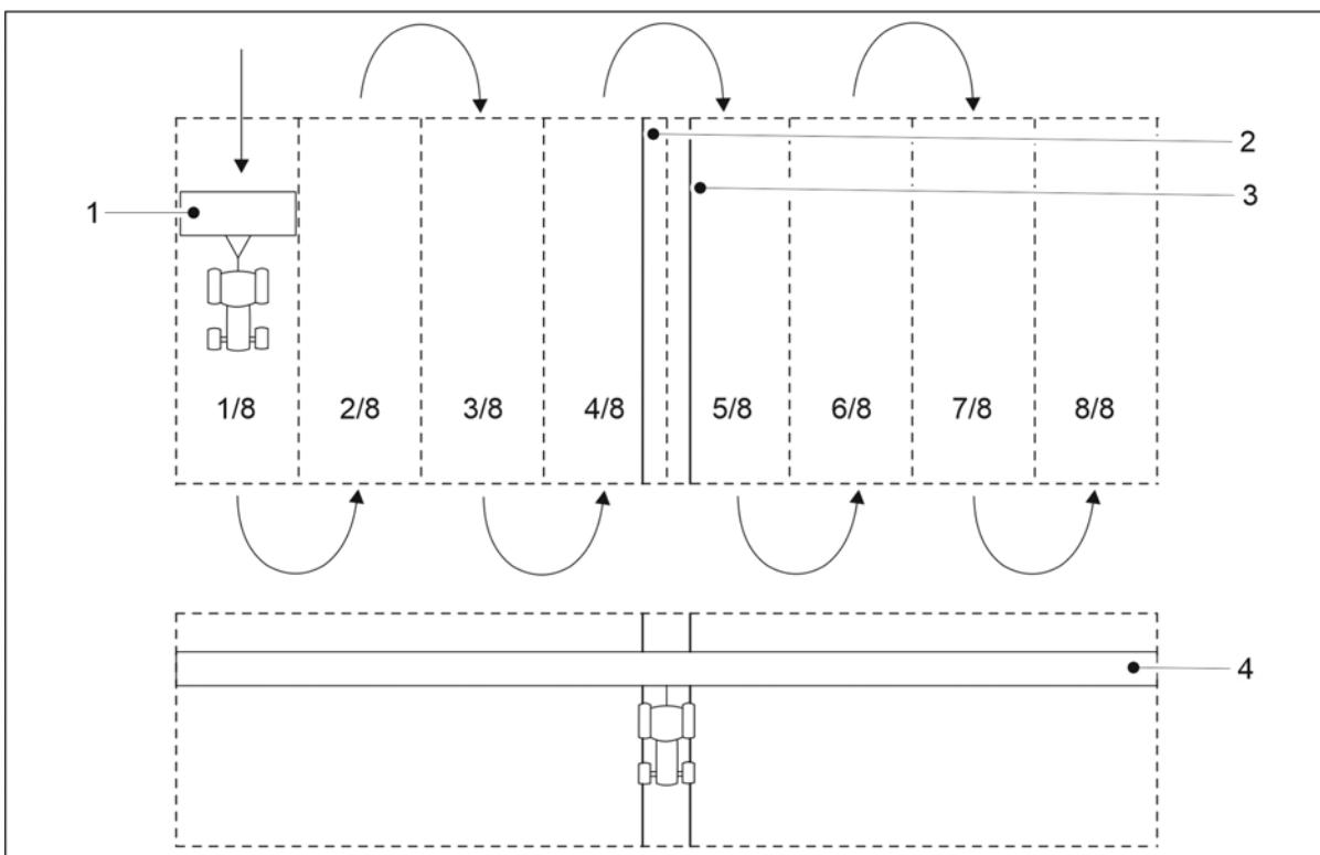
Obrázek. 5.2.2.1 - 116. Asymetrické kolejové řádky
