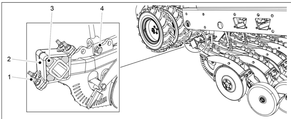
Obrázek. 7.9.1.1 - 355. Demontáž radličky
