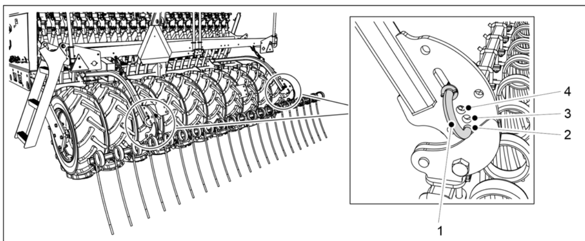
Obrázek. 6.11 - 248. Regulace úhlu zadních bran
