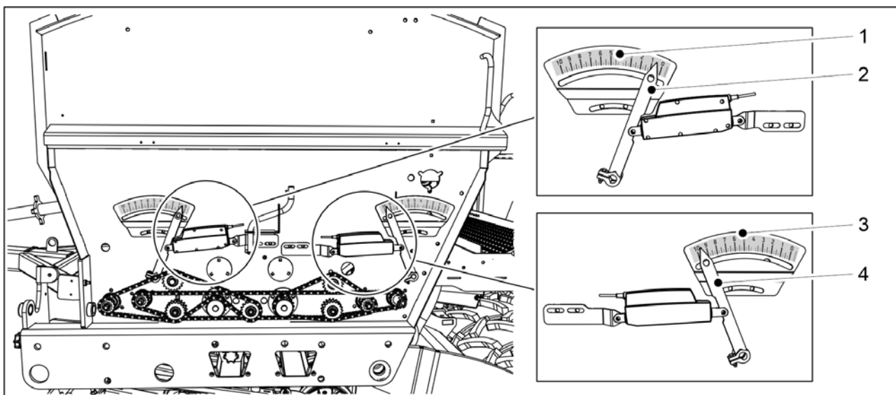
Obrázek. 7.1.14 - 292. Kontrola fungování regulace cílové dávky
