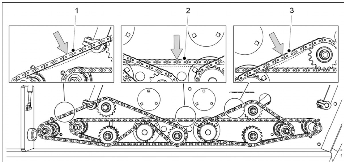
Obrázek. 7.1.5.1 - 281. Kontrola napnutí řetězu, převodovka hnojiva a osiva
