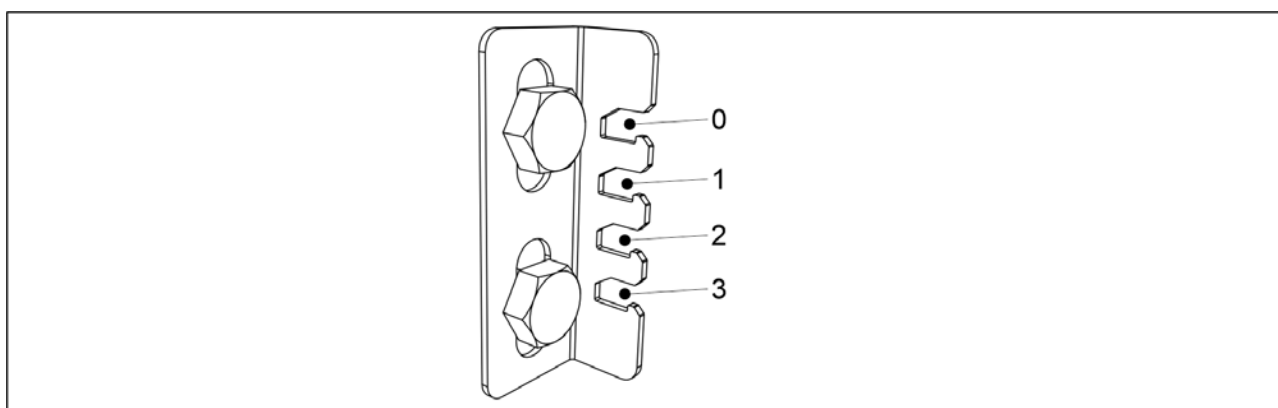
Obrázek. 6.6.7.1 - 172. Pozice ovládací páky / materiál k vysetí
