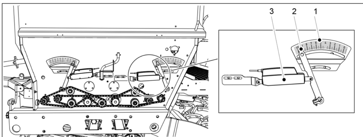
Obrázek. 6.8.5 - 233. Lineární ovladač
