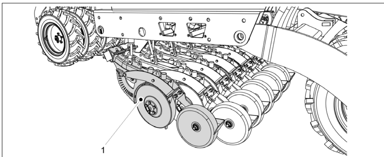
Obrázek. 7.9.1.1 - 353. Spouštění radličky na zem
