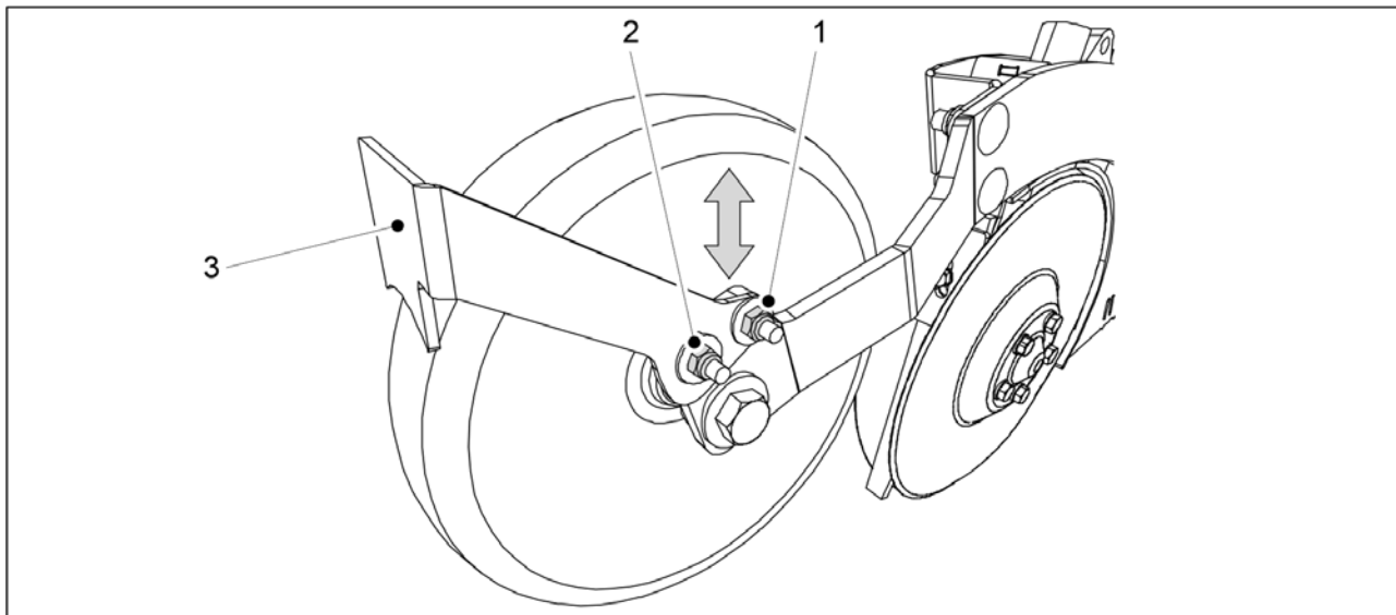
Obrázek. 7.9.5.2 - 370. Stěrka uzavíracího kolečka
