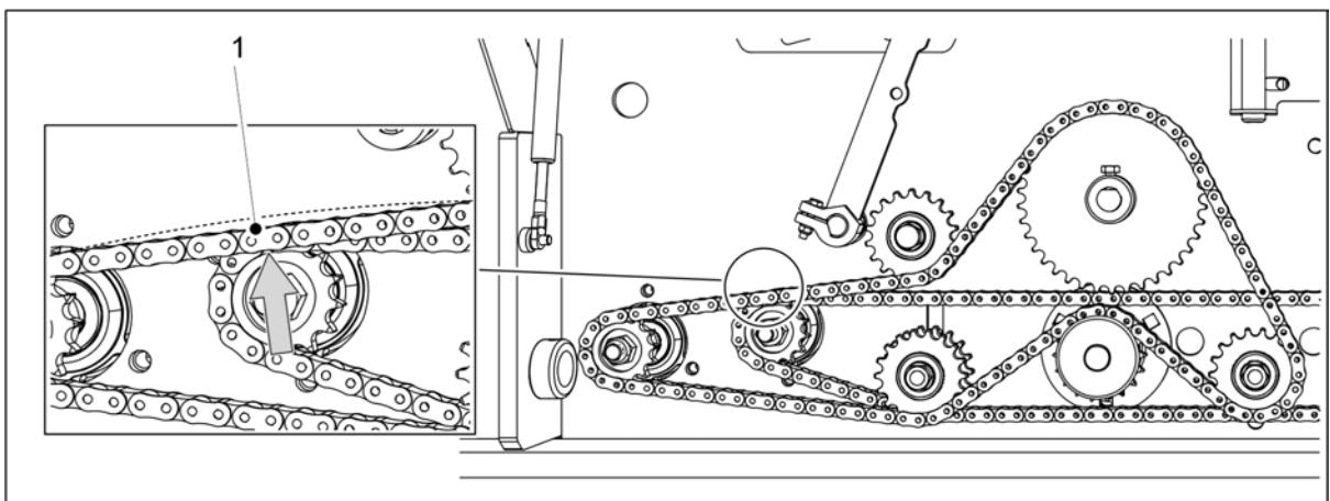
Obrázek. 7.1.5.3 - 283. Kontrola napnutí řetězu, převodovka dávkovací osy hnojiva
