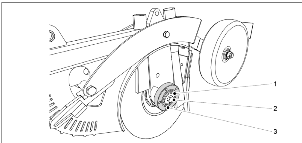
Obrázek. 7.9.2.1 - 360. Demontáž pouzdra ložiska
