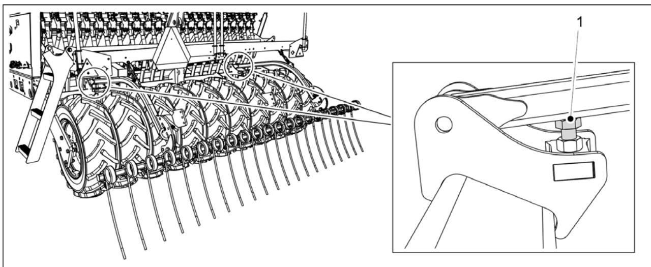
Obrázek. 6.11 - 247. Regulace výšky zadních bran
