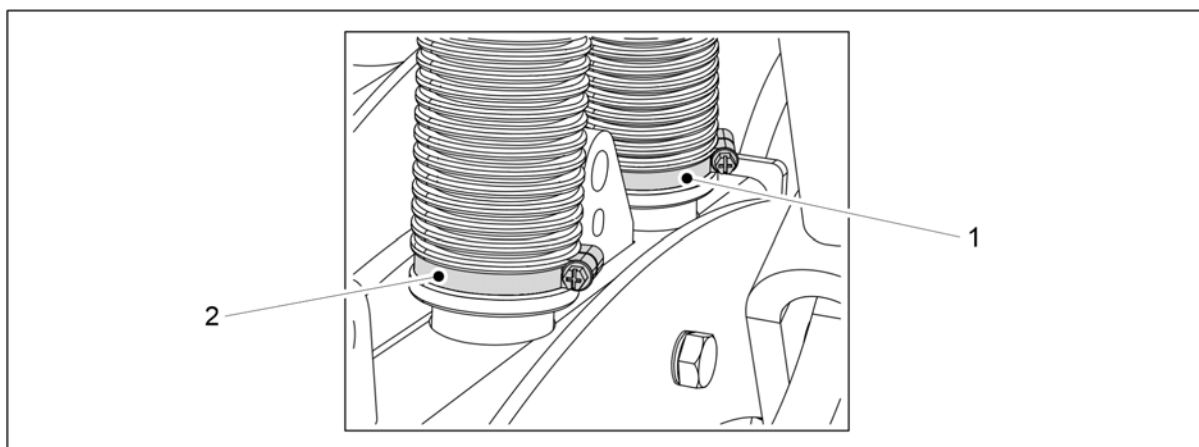
Obrázek. 5.1.10 - 84. Upevnění secí a hnojící hadice k radličce
