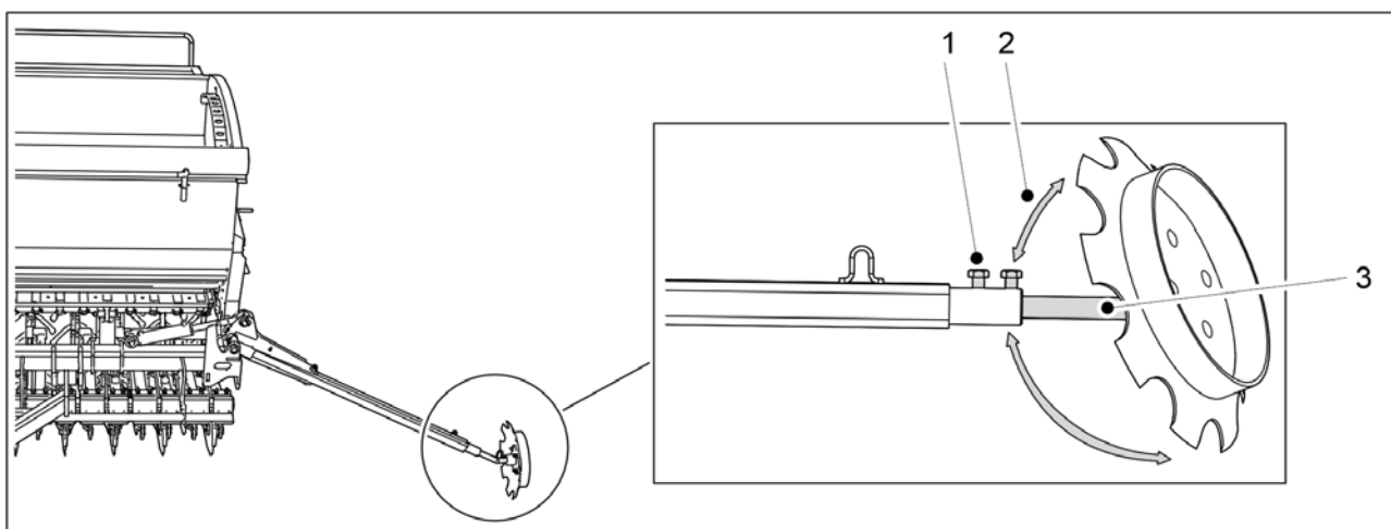
Obrázek. 5.3.7 - 132. Úprava středních značkovačů
