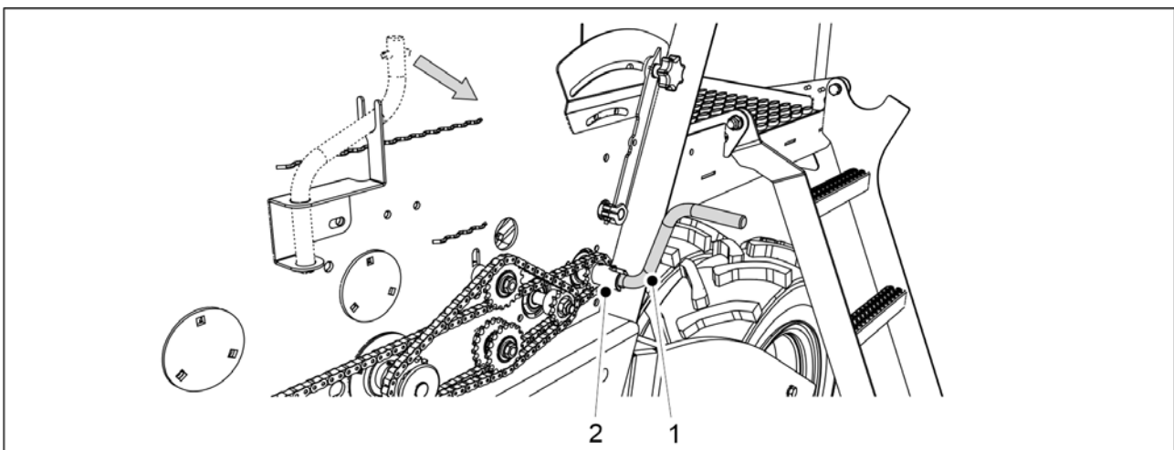
Obrázek. 6.8.4 - 218. Upevnění kliky pro kalibrační zkoušku
