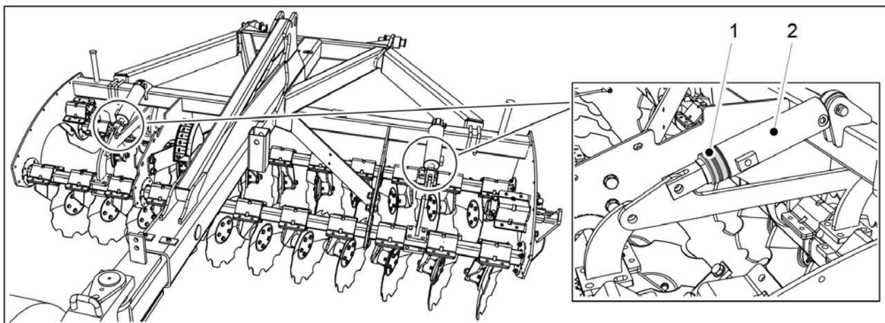
Obrázek. 6.14 - 252. Regulace hloubky orby předního diskového kultivátoru
