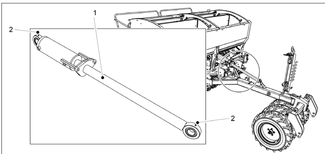
Obrázek. 7.2.14 - 313. Válec táhla
