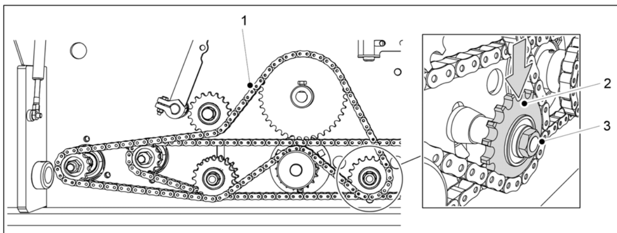
Obrázek. 7.5.3 - 342. Dotážení řetězu dávkovací osy hnojiva
