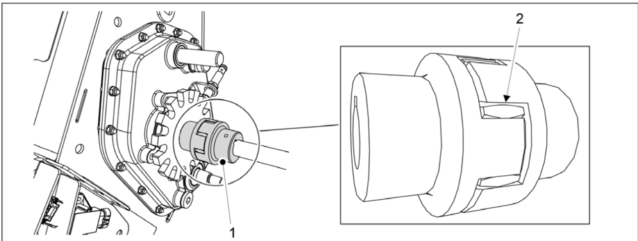
Obrázek. 7.1.7 - 287. Kontrola spojky
