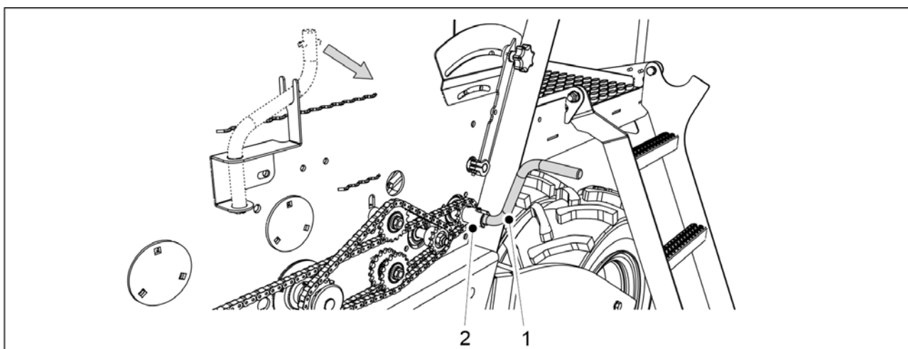
Obrázek. 6.8.5 - 234. Upevnění kliky pro kalibrační zkoušku
