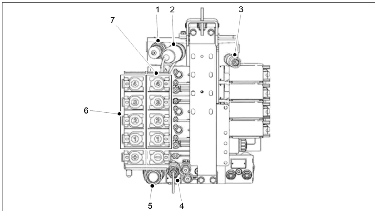
Obrázek. 5.3 - 120. Jako spojovací model jsou dodány hydraulické spoje série T Valtra.
