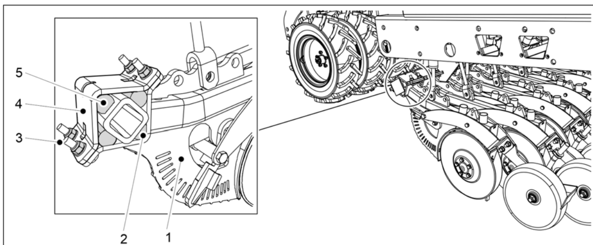
Obrázek. 7.9.1.2 - 356. Utažení radličky
