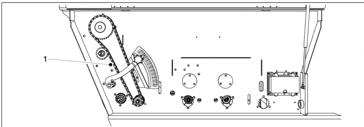
Obrázek. 7.2.2.2 - 296. Mazání řetězu, převodovka násypky malého osiva
