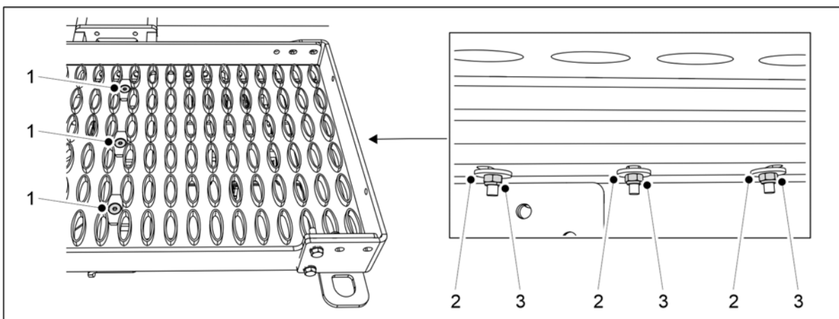
Obrázek. 5.1.16 - 108. Montáž lávky na držáky
