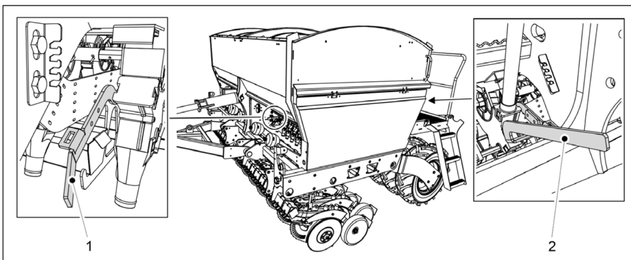
Obrázek. 7.3.1 - 317. Spodní klapky otevřeny
