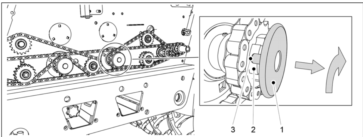
Obrázek. 6.8.4 - 213. Deaktivace podavače osiva
