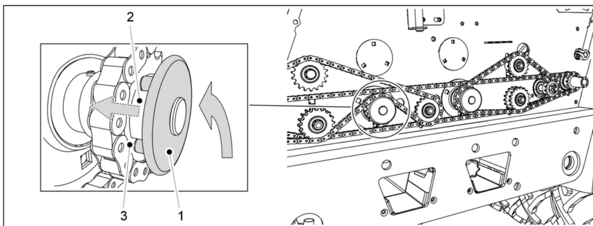
Obrázek. 6.8.5 - 240. Návrat podavače hnojiva do provozní polohy
