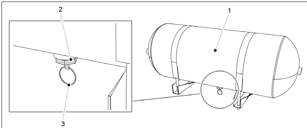
Obrázek. 7.1.15.2 - 293. Vypuštění vody z pneumatické nádrže
