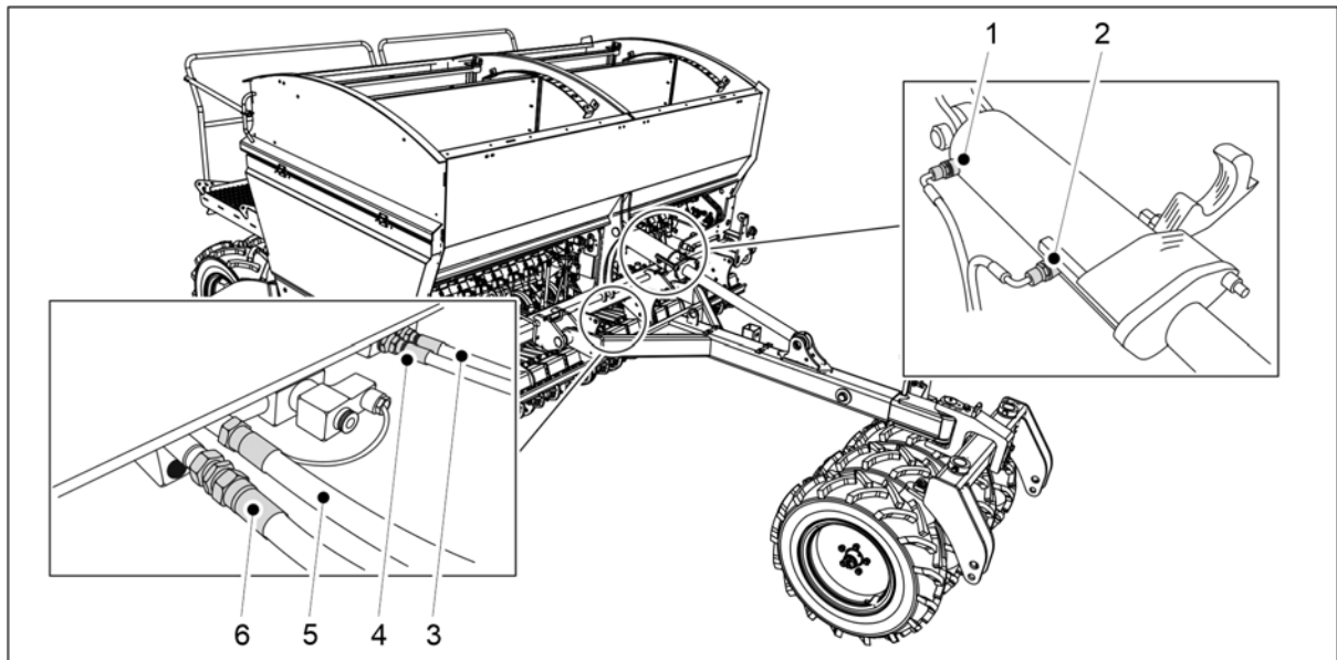
Obrázek. 5.1.1 - 64. Zapojení hydraulických hadic
