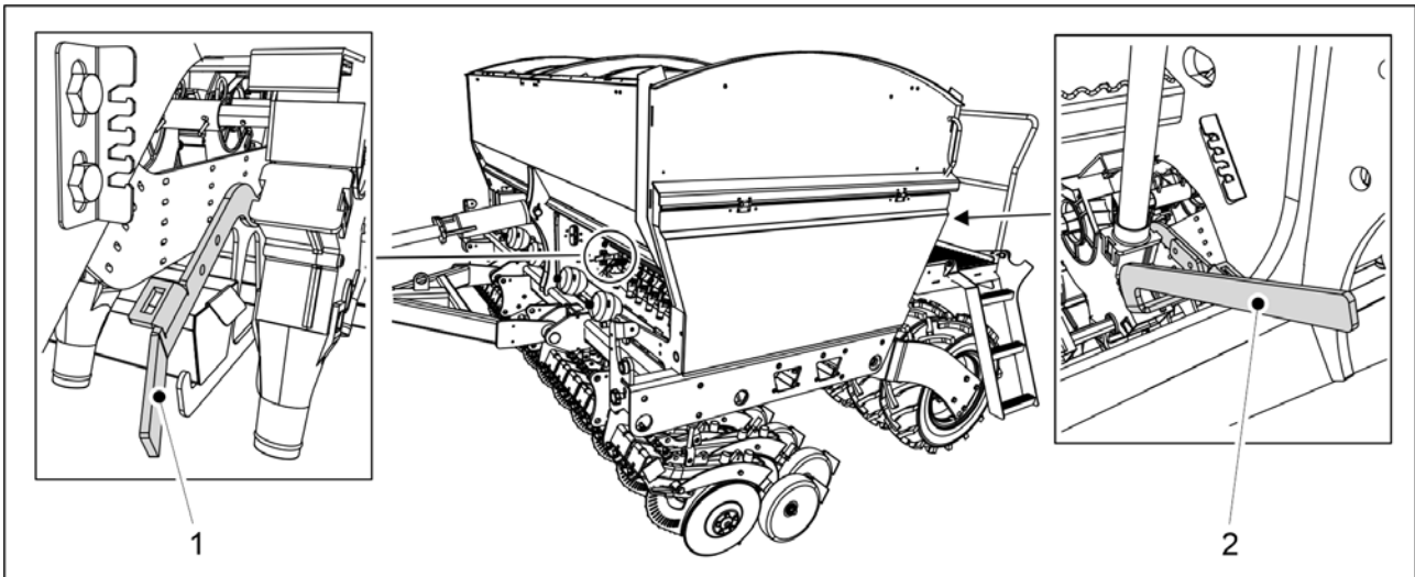
Obrázek. 6.20.2 - 265. Otevření spodních klapek násypek
