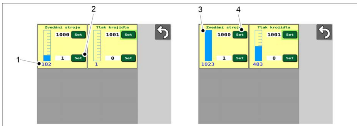
Obrázek. 7.10.1.1 - 371. Kalibrace snímače secí pozice stroje
