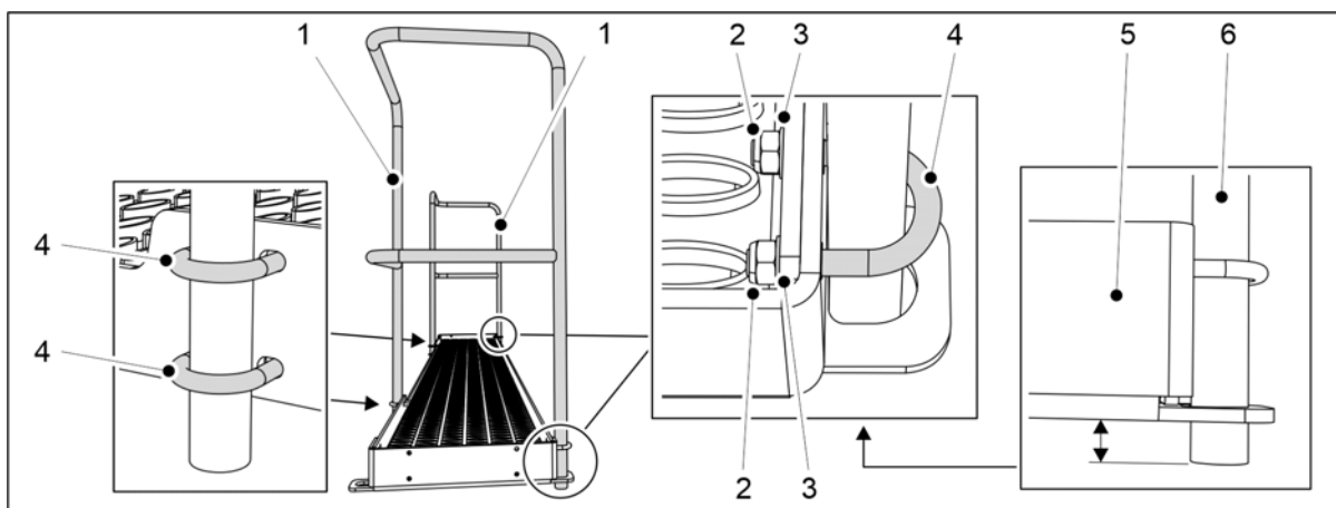
Obrázek. 5.1.15 - 103. Montáž zábradlí na model FORTE 400 EVO
