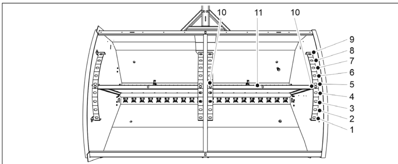
Obrázek. 6.6.5 - 168. Úprava rozdělovače násypky
