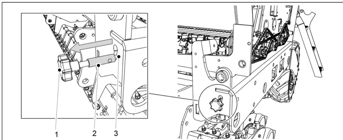
Obrázek. 6.8.1 - 186. Vytáhněte regulační tyč kalibrační zkoušky.
