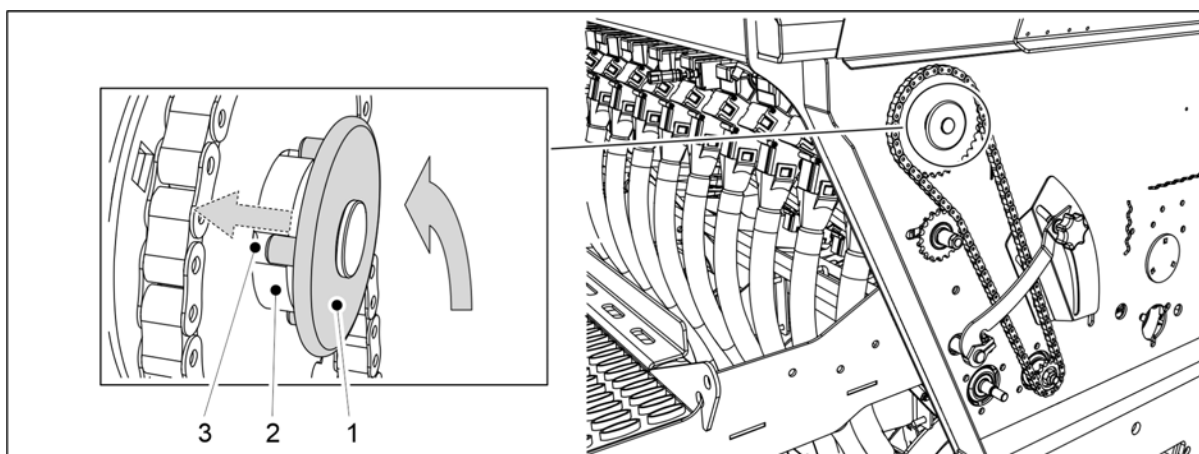
Obrázek. 6.8.5 - 241. Návrat podavače malého osiva do provozní polohy
