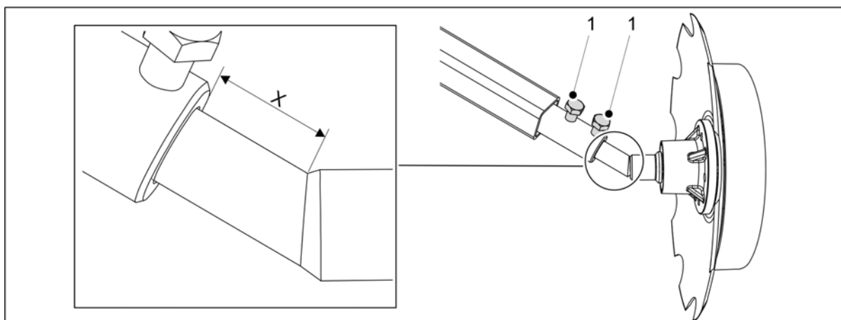
Obrázek. 5.3.7 - 133. Měření výchozí úpravy šířky
