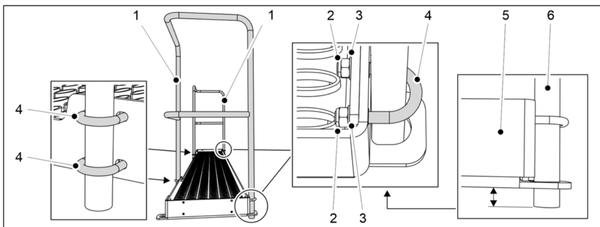
Obrázek. 5.1.16 - 110. Montáž zábradlí na stroj 400
