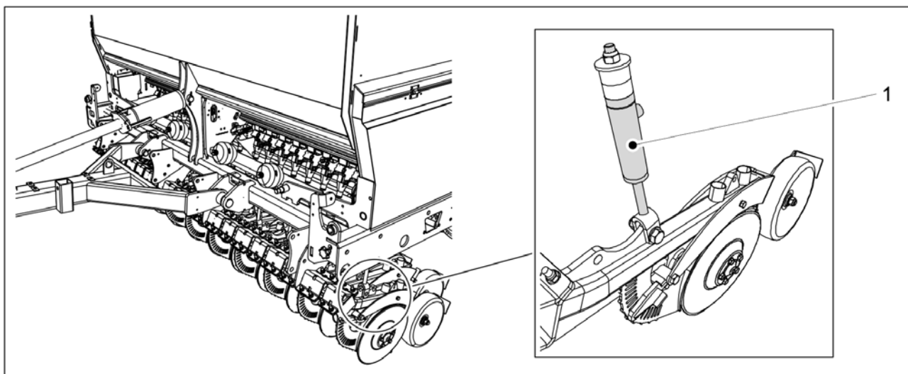
Obrázek. 6.10 - 246. Úprava tlaku radličky
