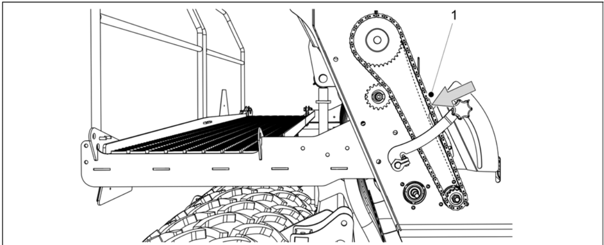
Obrázek. 7.1.5.2 - 282. Kontrola napnutí řetězu, převodovka malého osiva
