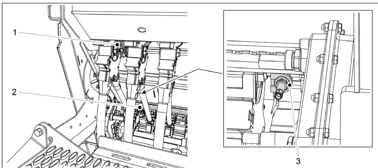
Obrázek. 4.1.1.5 - 21. Umístění otočných krytů hřídele
