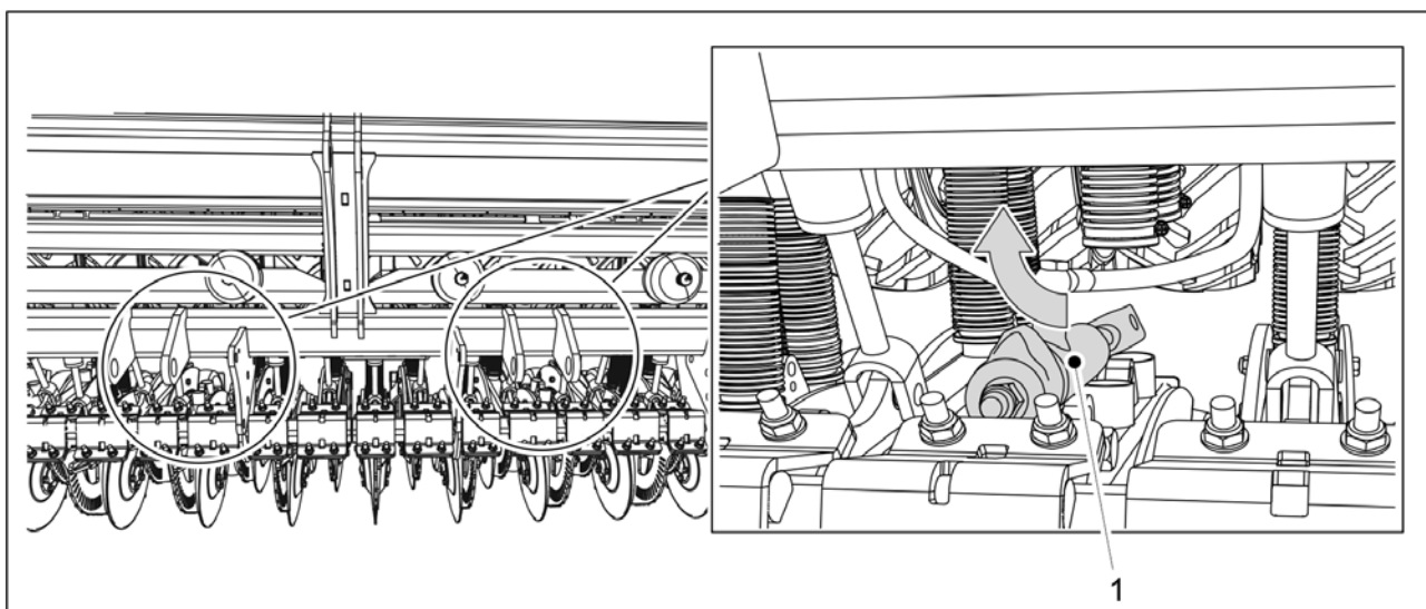
Obrázek. 5.1.10 - 82. Montáž válce
