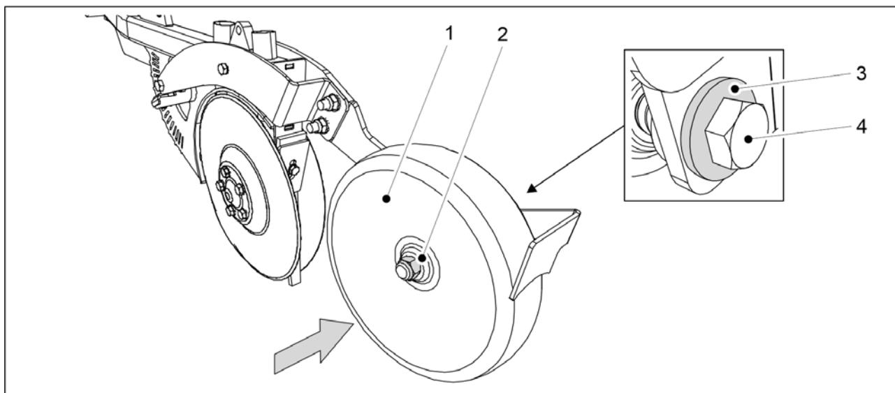
Obrázek. 7.9.4.2 - 368. Instalace uzavíracího kola
