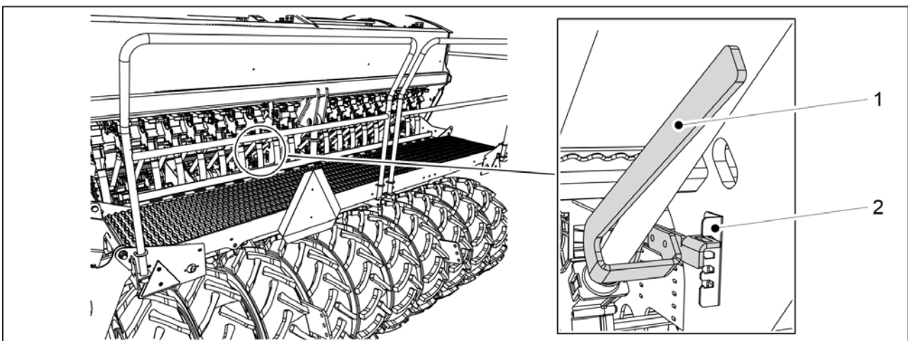
Obrázek. 6.6.8.1 - 174. Ovládací páka pro spodní klapky podavačů, zásobník osiva
