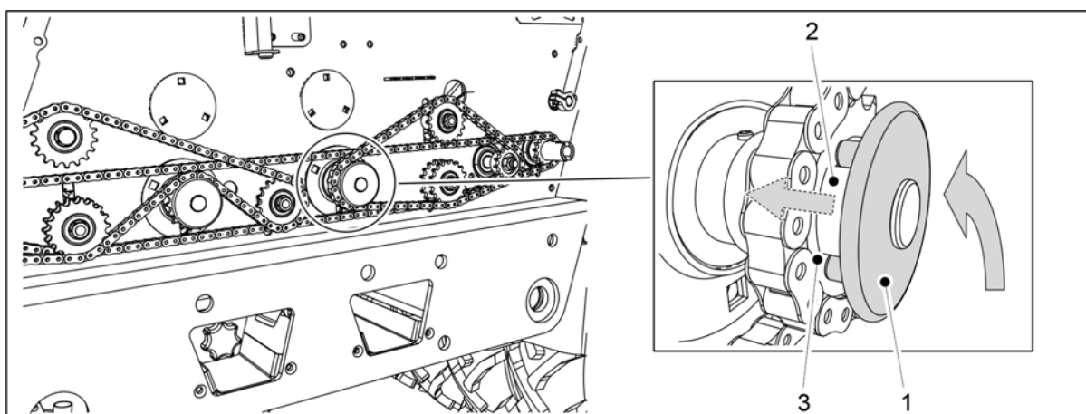
Obrázek. 6.8.1 - 191. Návrat podavače osiva do provozní polohy
