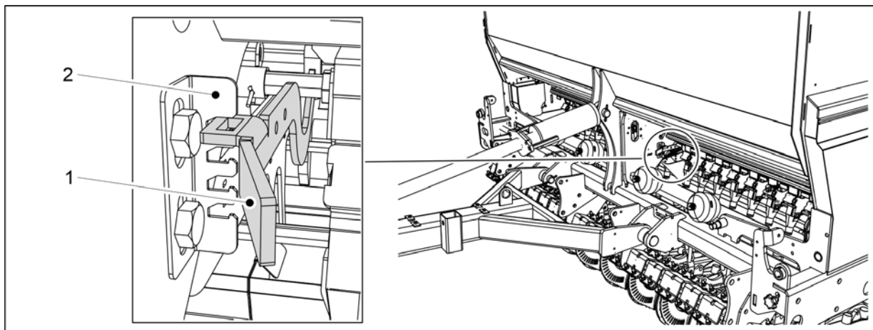
Obrázek. 6.6.7.1 - 171. Ovládací páka pro spodní klapky podavačů, zásobník hnojiva
