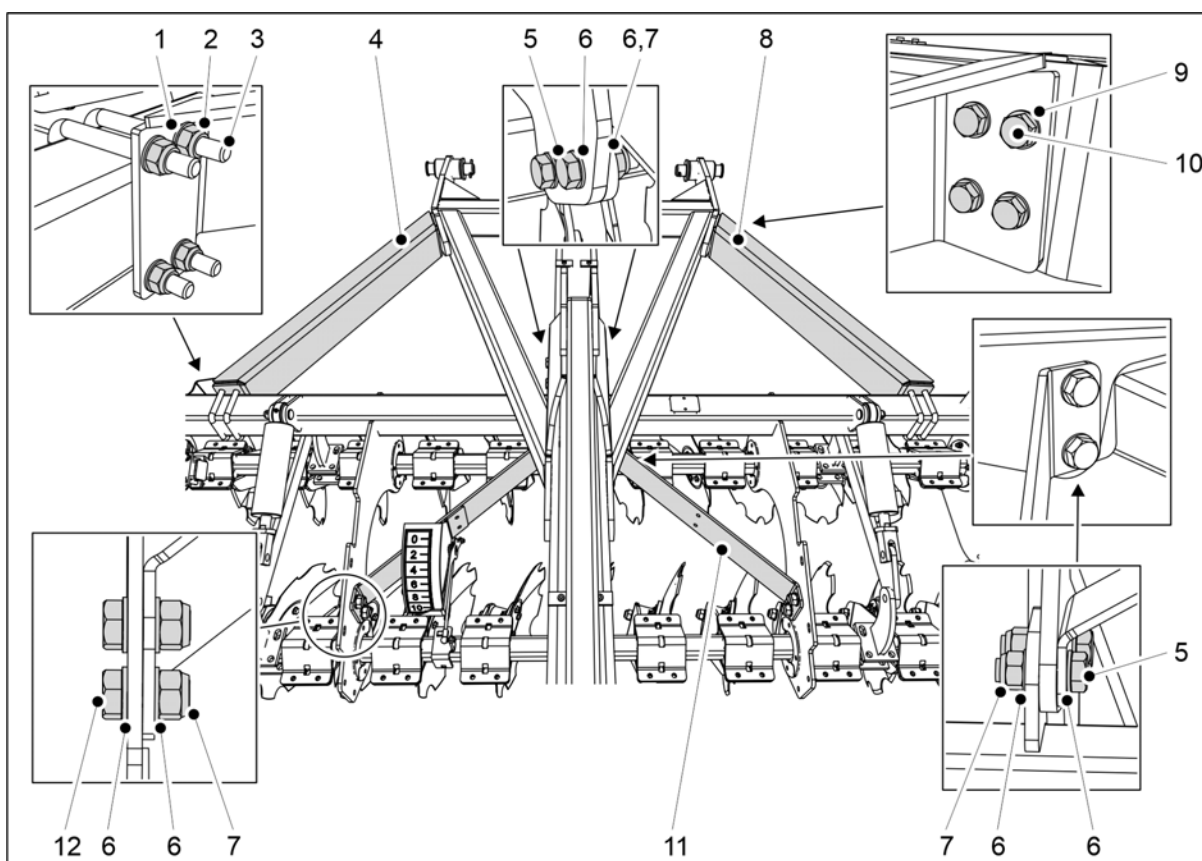
Obrázek. 5.1.6 - 74. Upevnění předního diskového kultivátoru k táhlu
