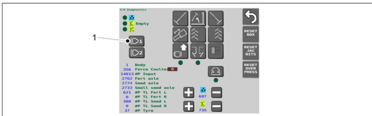
Obrázek. 6.3.12 - 162. Obrazovka režimu diagnostiky vstupů a výstupů
