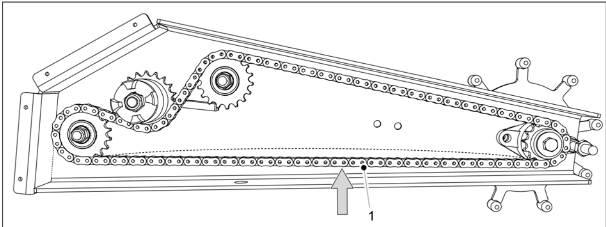
Obrázek. 7.1.6 - 286. Řetěz pohonu kola
