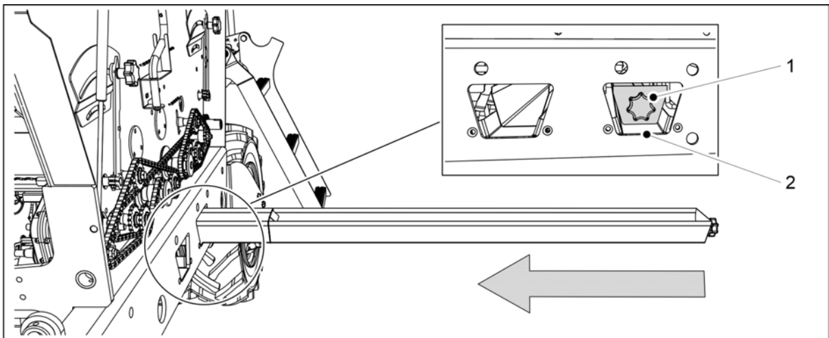
Obrázek. 6.8.5 - 228. Nastavení kalibračních misek
