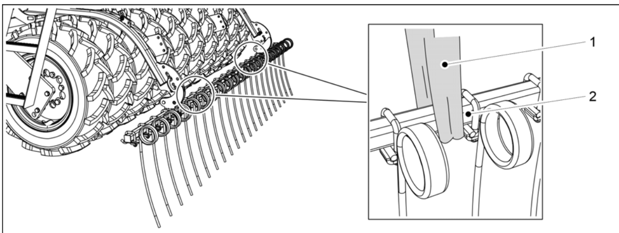
Obrázek. 7.4.1 - 327. Zvednutí zadních bran
