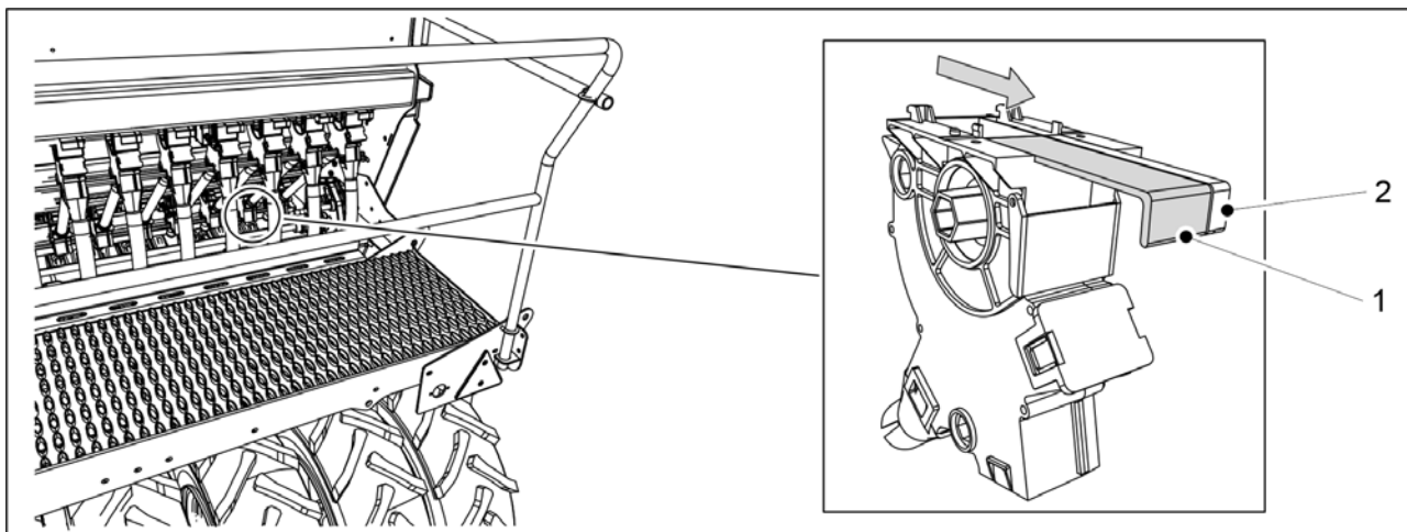
Obrázek. 6.6.8.2 - 176. Uzavírací deska na podavači osiva
