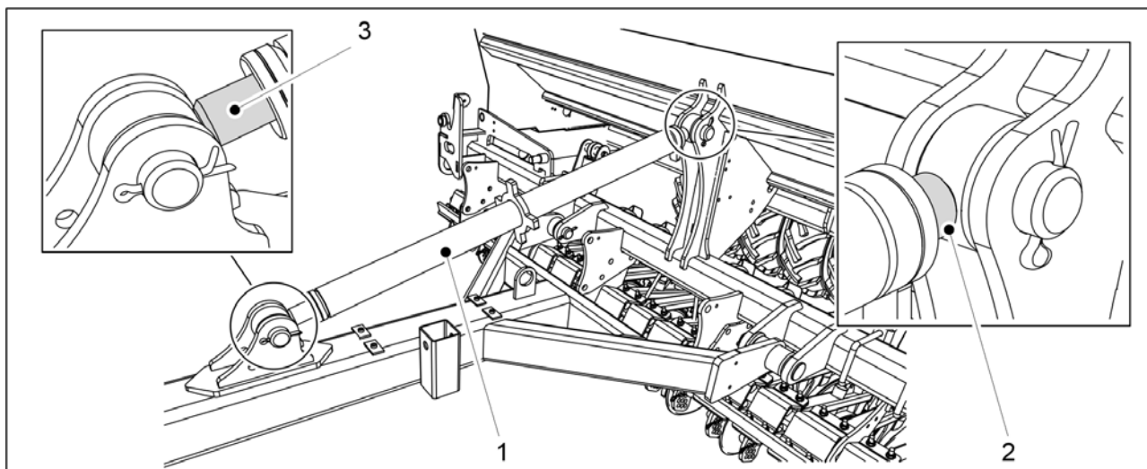
Obrázek. 7.2.15 - 314. Napínák
