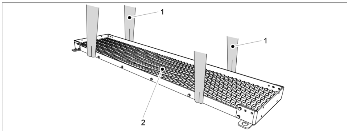
Obrázek. 5.1.15 - 99. Zvedání lávky
