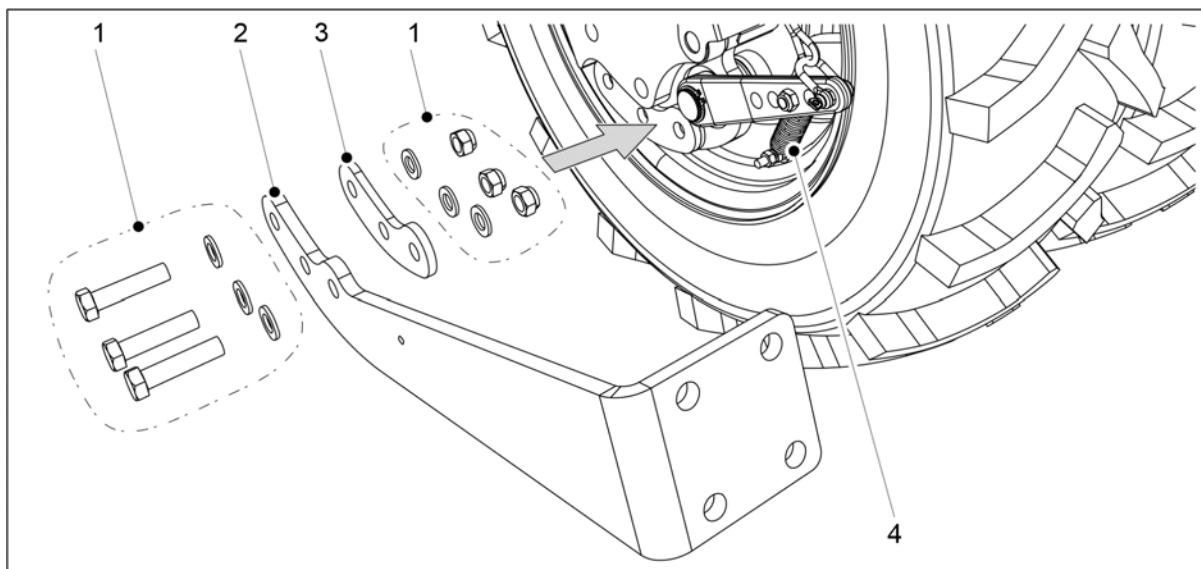
Obrázek. 5.1.12 - 88. Montáž stěrky k nastavci držáku
