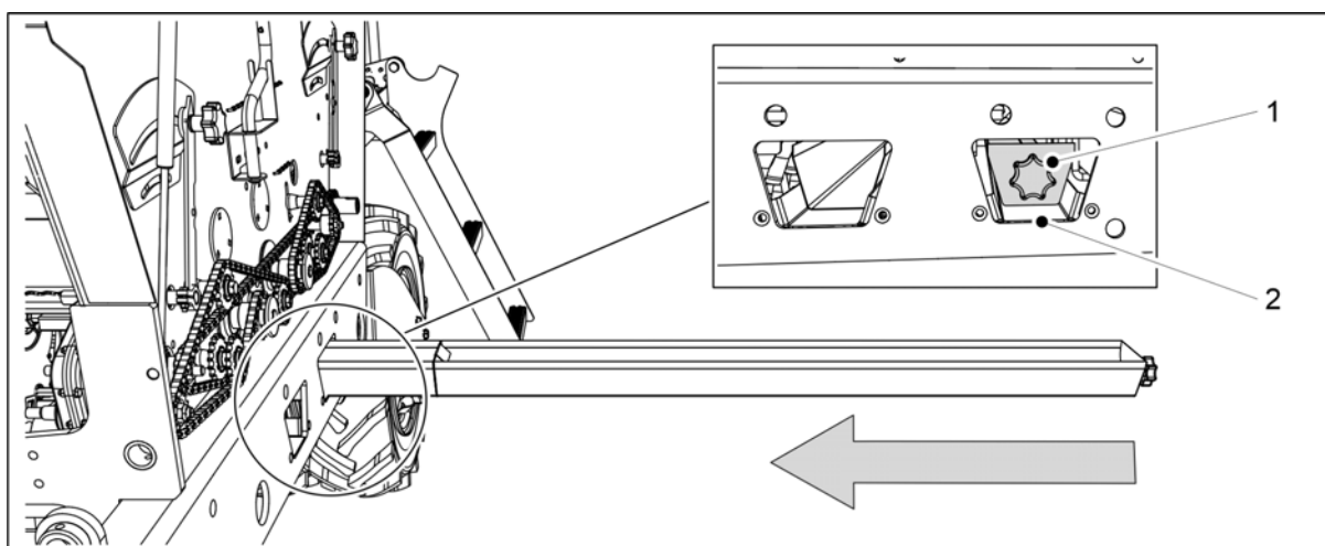
Obrázek. 6.8.2 - 195. Nastavení kalibračních misek
