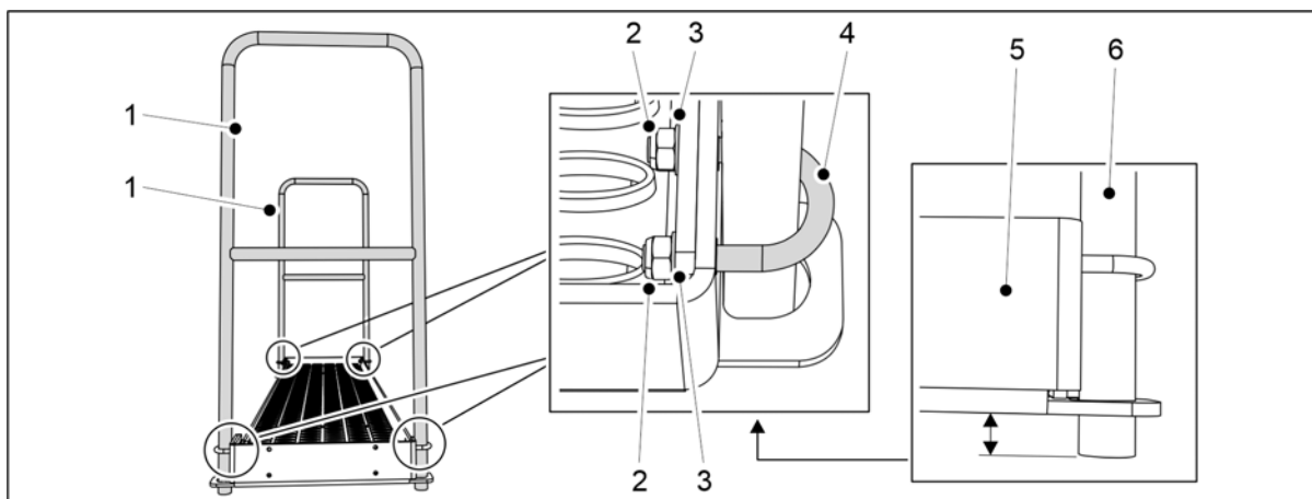
Obrázek. 5.1.15 - 102. Montáž zábradlí na model FORTE 300 EVO
