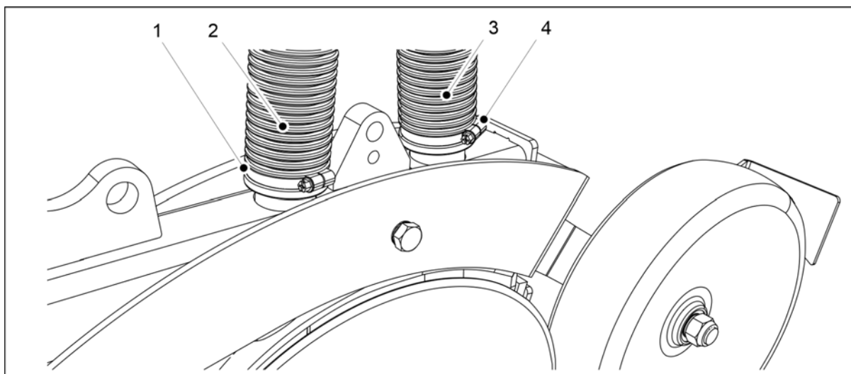
Obrázek. 7.9.1.1 - 354. Odpojení hadic radličky
