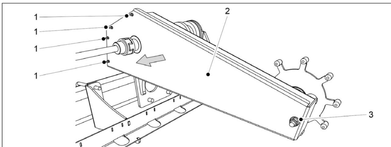
Obrázek. 7.2.3.2 - 299. Kryt pláště pohonu kola
