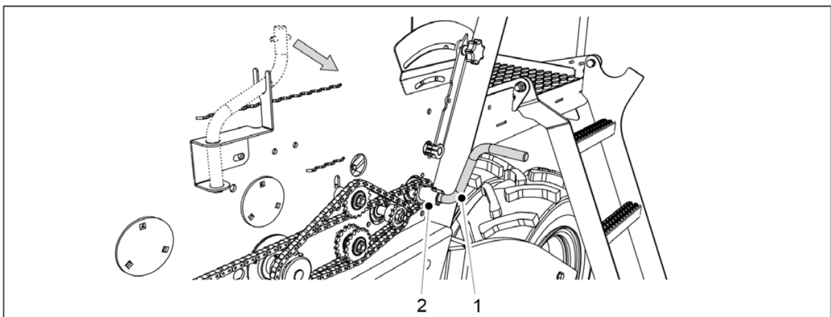
Obrázek. 6.8.2 - 198. Upevnění kliky pro kalibrační zkoušku
