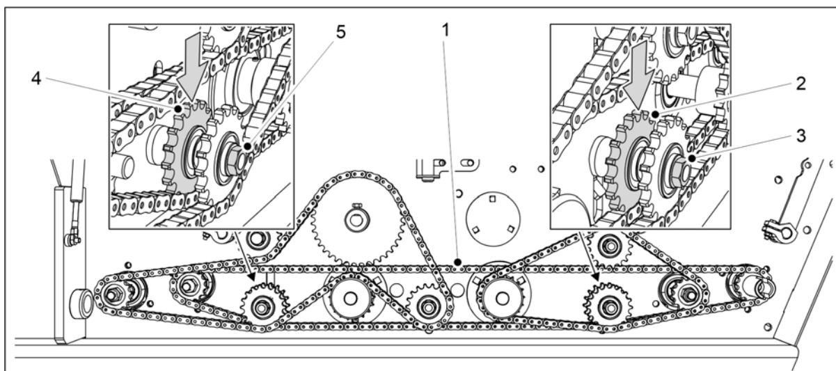
Obrázek. 7.5.3 - 341. Napnutí převodového řetězu
