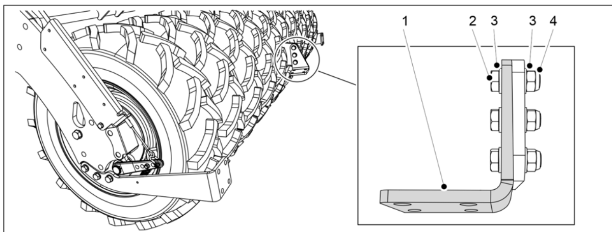
Obrázek. 5.1.12 - 89. Montáž závěsných desek stěrky
