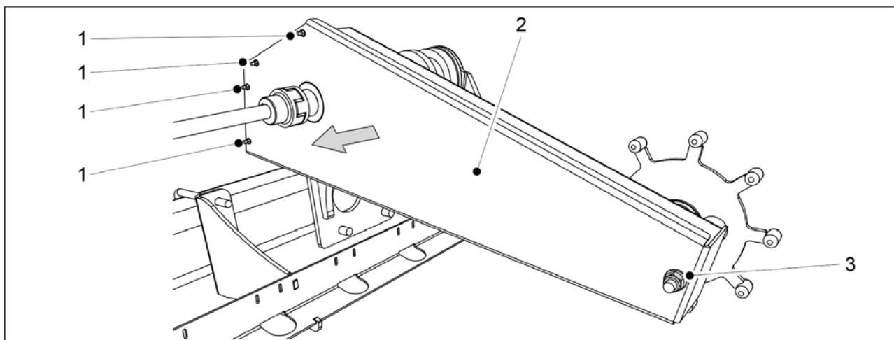
Obrázek. 7.2.3.1 - 297. Řetěz pohonu kola
