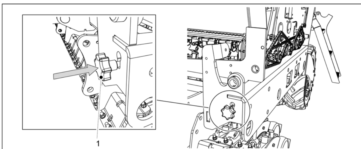
Obrázek. 6.8.5 - 242. Vložení regulační tyče kalibrační zkoušky
