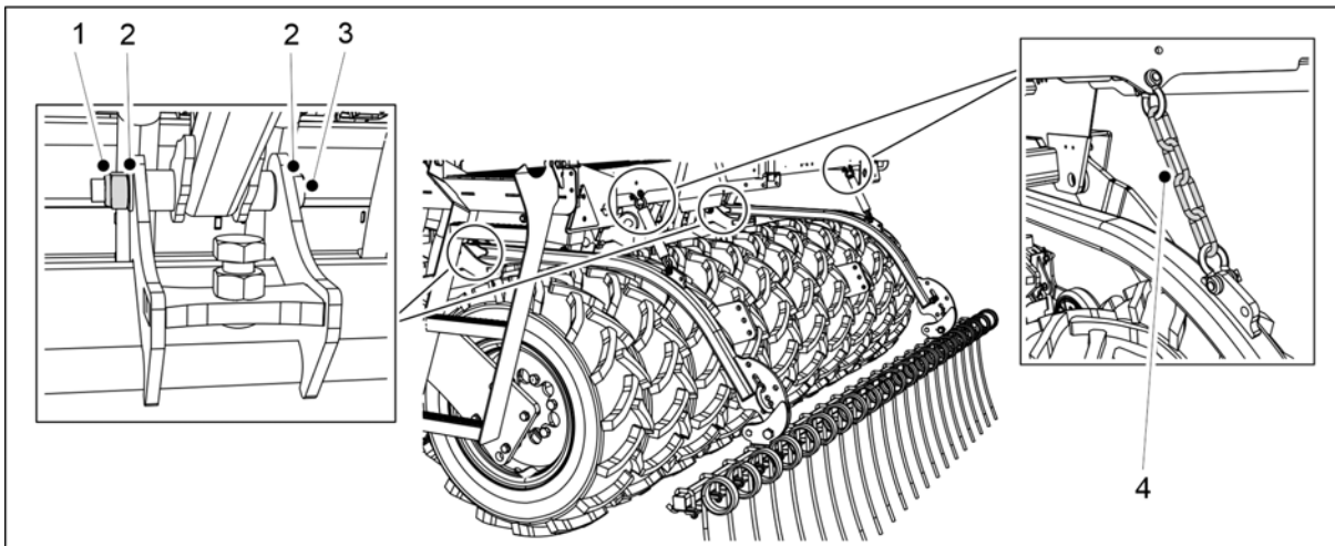
Obrázek. 7.4.1 - 326. Demontáž zadních bran
