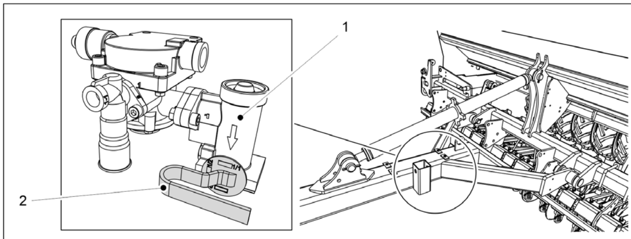
Obrázek. 6.19.3 - 263. Řídicí ventil brzdné síly
