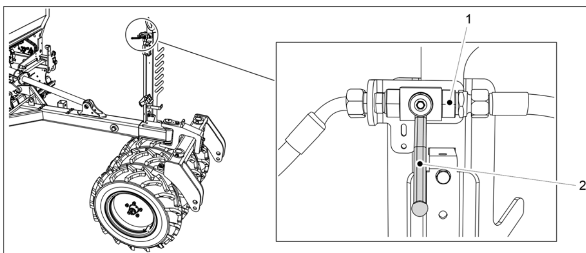
Obrázek. 5.3.5 - 131. Uzavření kulového ventilu zdvihacího obvodu
