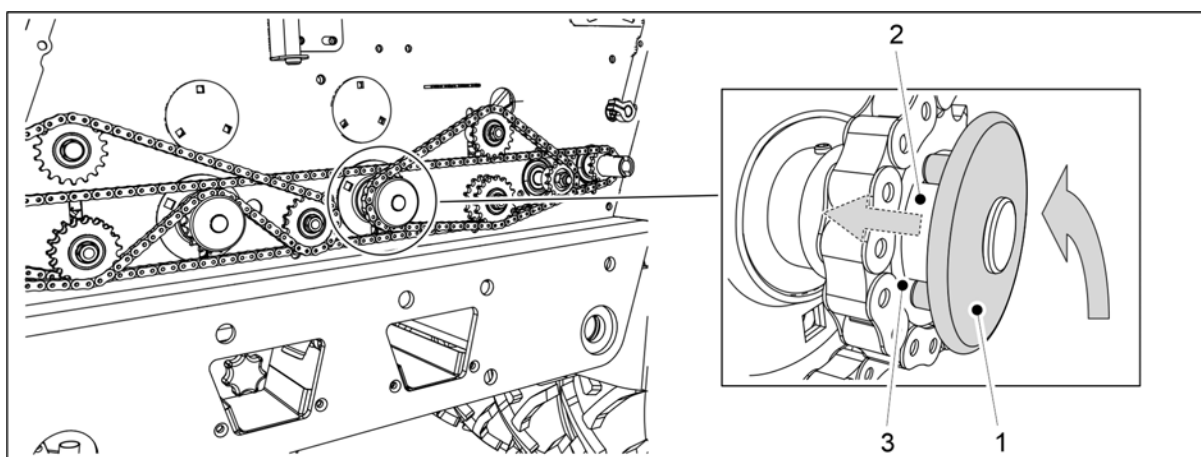
Obrázek. 6.8.4 - 224. Návrat podavače osiva do provozní polohy
