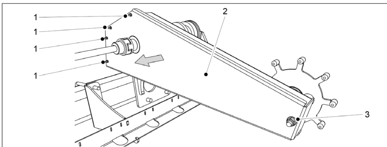
Obrázek. 7.1.6 - 285. Kryt pláště pohonu kola
