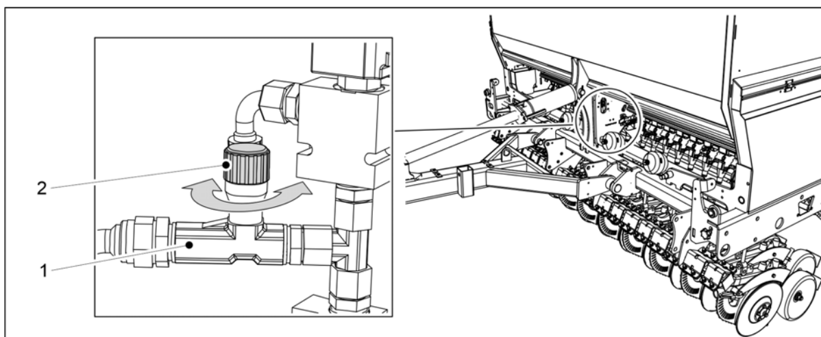
Obrázek. 5.3.7 - 134. Úprava rychlosti zdvihu středních značkovačů
