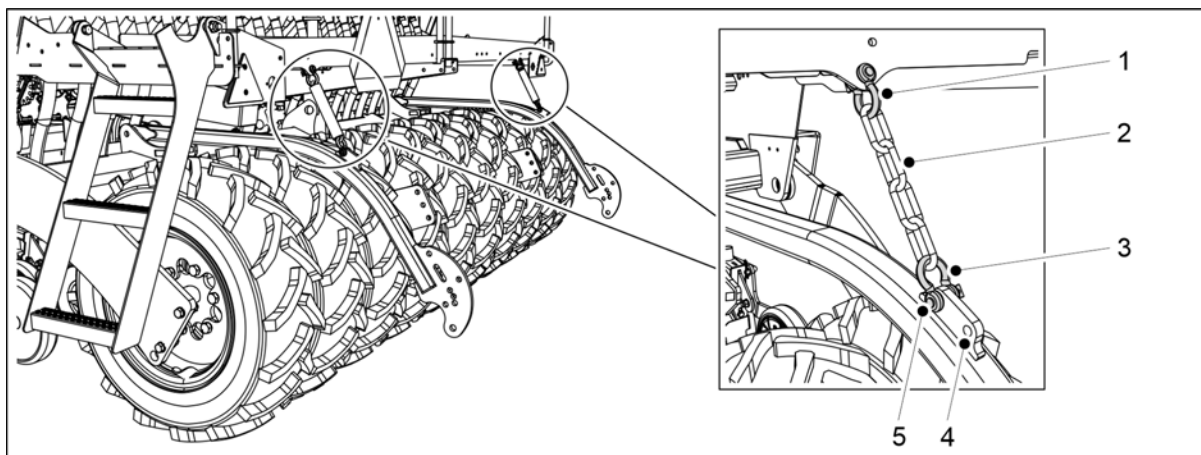
Obrázek. 5.1.13 - 92. Montáž řetězů zadních bran
