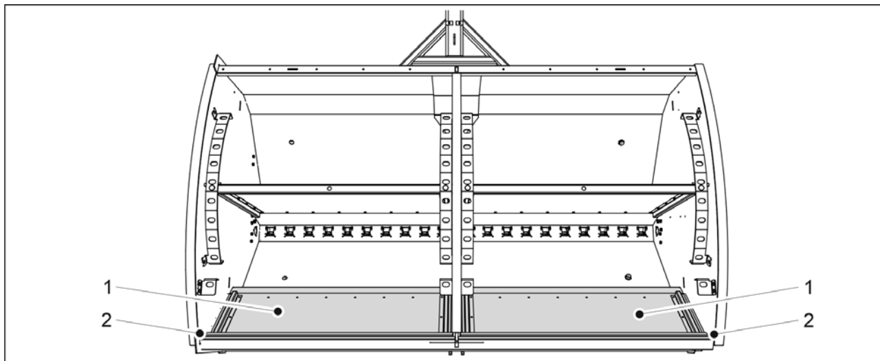
Obrázek. 6.6.4.1 - 167. Rozdělovače násypky malého osiva otočené vzad
