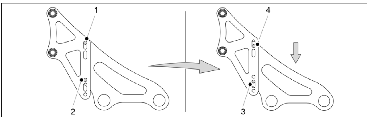
Obrázek. 6.13 - 251. Regulace výšky předních bran
