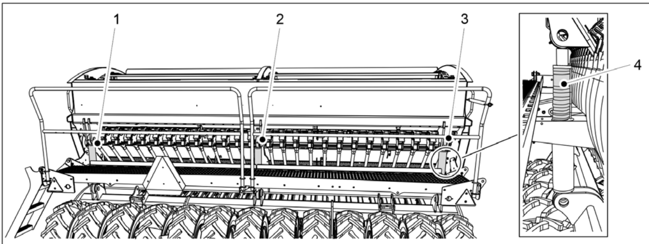
Obrázek. 7 - 270. Dorazy válců
