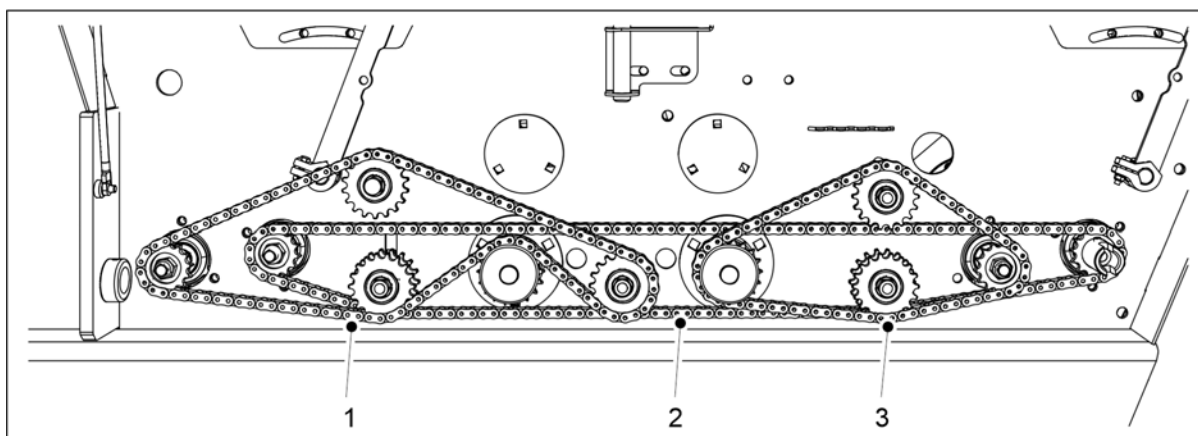
Obrázek. 7.2.2.1 - 295. Mazání řetězu, převodovka násypky hnojiva a osiva
