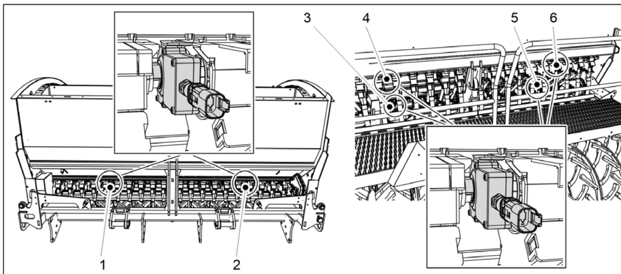
Obrázek. 4.1.1.7 - 24. Pozice spojky kolejových řádků
