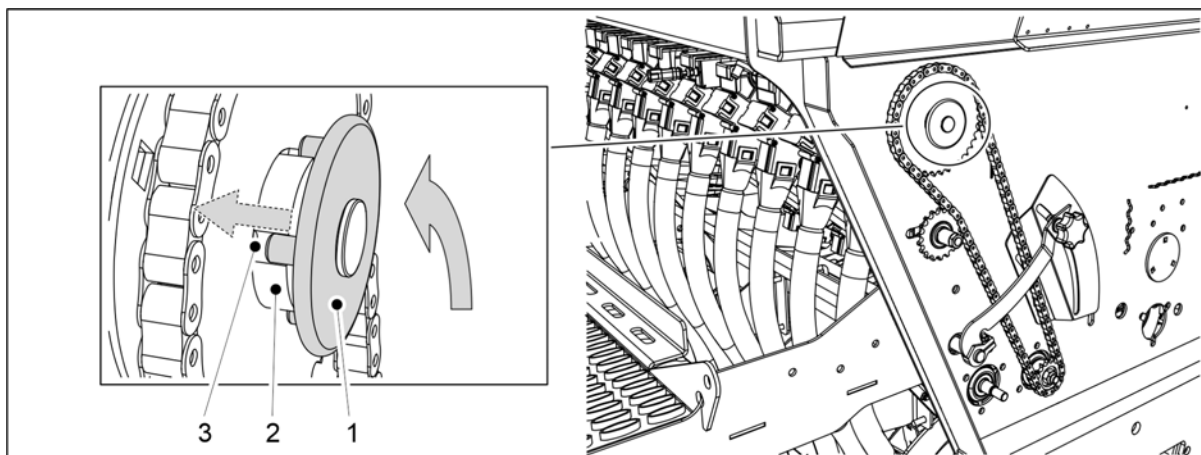
Obrázek. 6.8.4 - 225. Návrat podavače malého osiva do provozní polohy
