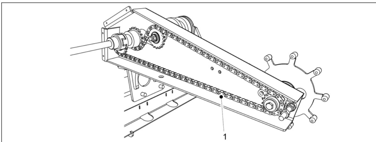
Obrázek. 7.2.3.1 - 298. Mazání řetězu pohonu kola
