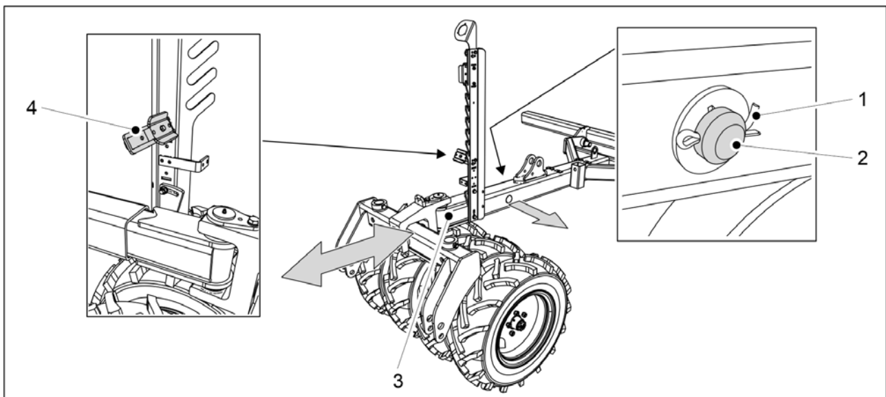
Obrázek. 5.3.1 - 124. Úprava délky nosníku
