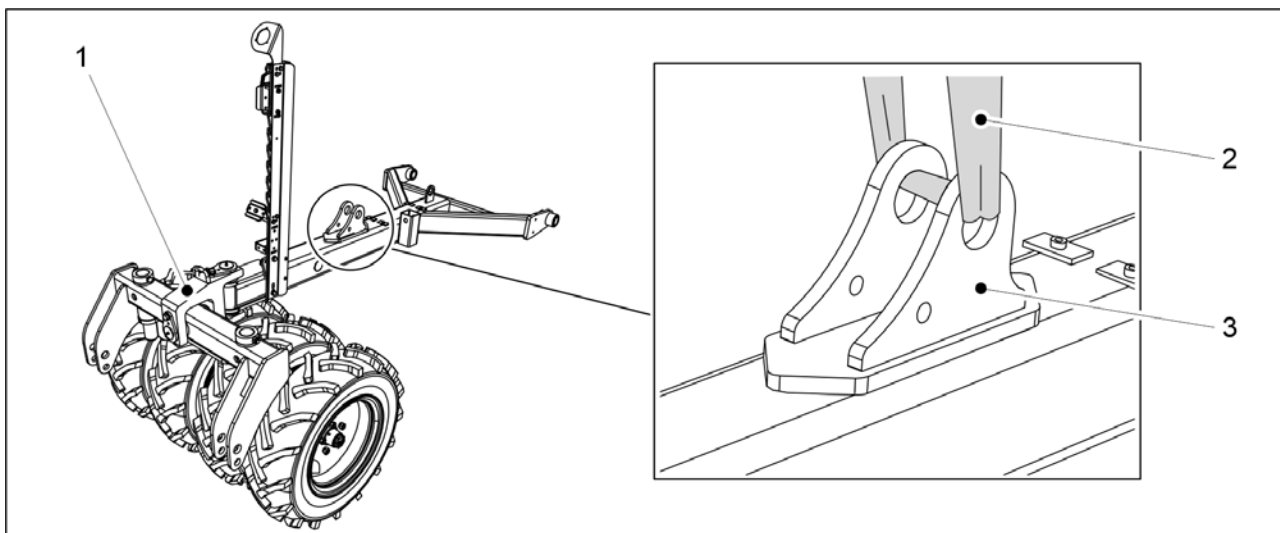
Obrázek. 5.1.1 - 61. Zvedání kolového pěchu
