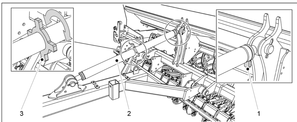
Obrázek. 5.3.3 - 127. Úprava pomocí napínáku
