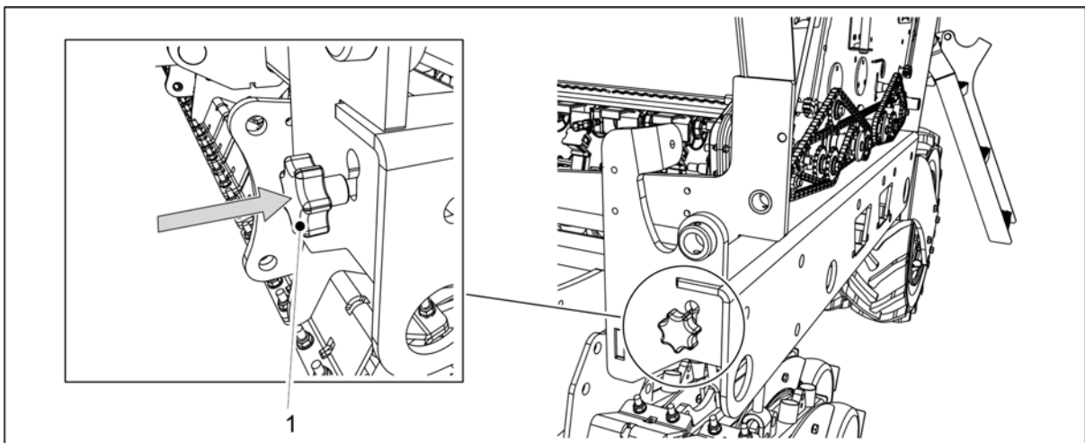
Obrázek. 6.8.2 - 201. Vložení regulační tyče kalibrační zkoušky
