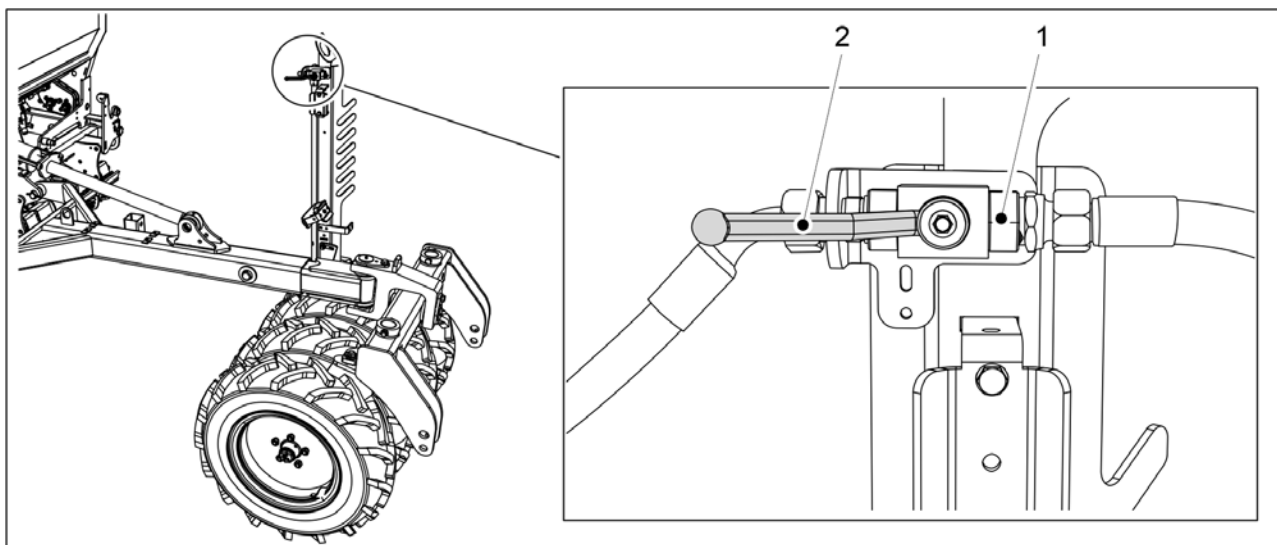
Obrázek. 5.3.5 - 130. Otevření kulového ventilu zdvihacího obvodu
