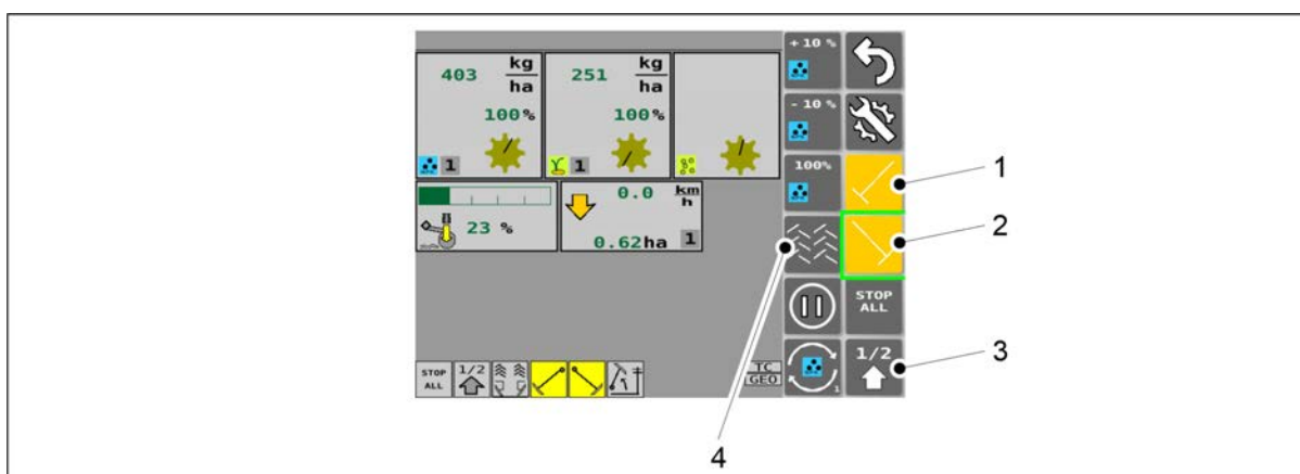
Obrázek. 6.3.11 - 158. Obrazovka jízdy v manuálním režimu
