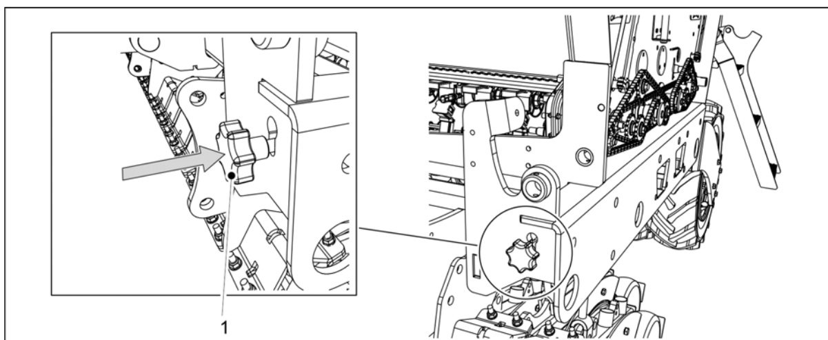
Obrázek. 6.8.4 - 226. Vložení regulační tyče kalibrační zkoušky
