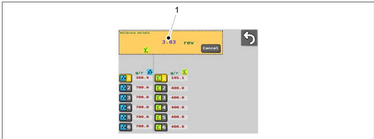
Obrázek. 6.8.5 - 236. Otáčky hřídele podavače provedené klikou kalibrační zkoušky
