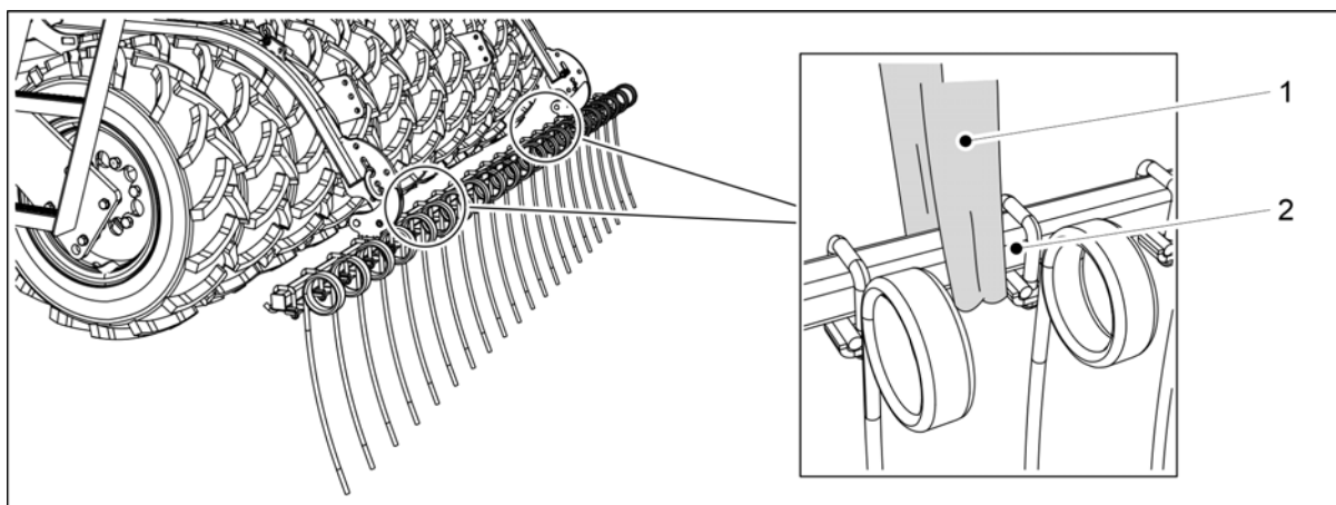
Obrázek. 5.1.13 - 93. Zvednutí zadních bran
