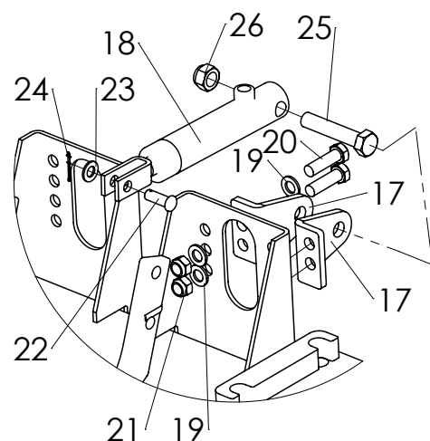
Jarrusylinterin kiinnikkeet, kiinteä akseli The brake cylinder brackets of the rigid axle
