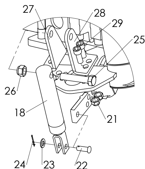
Jarrusylinterin kiinnikkeet, kääntyvä akseli The brake cylinder brackets of the steering axle
