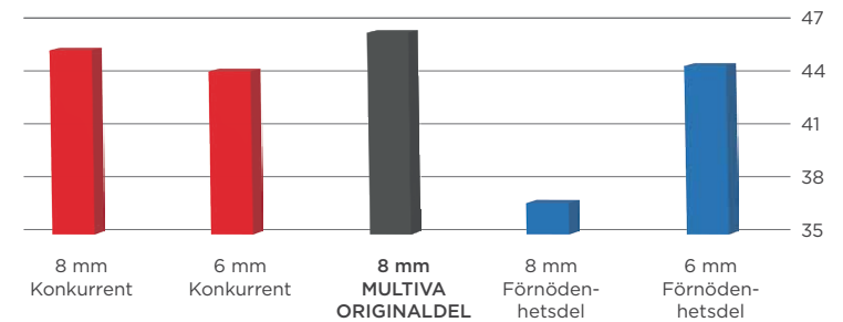
Spetsarnas hårdhet i medeltal* (HRC)
